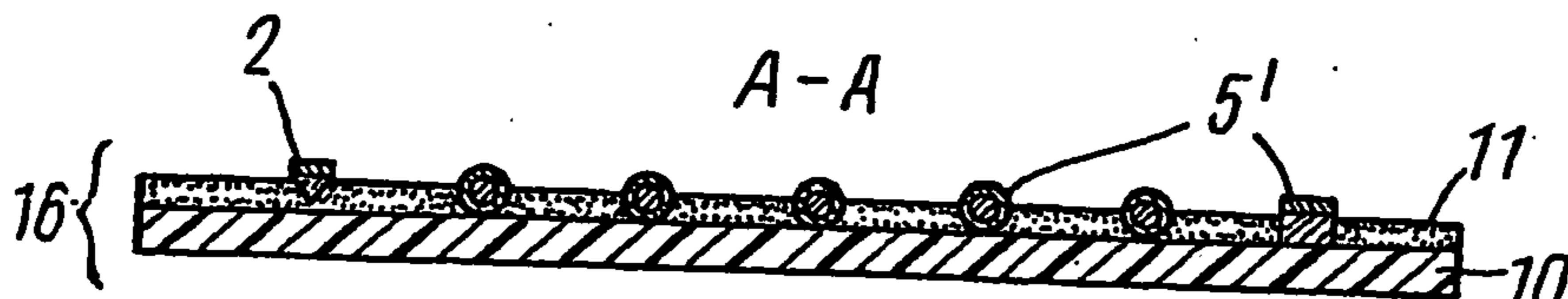
A-A FIG. 5B
