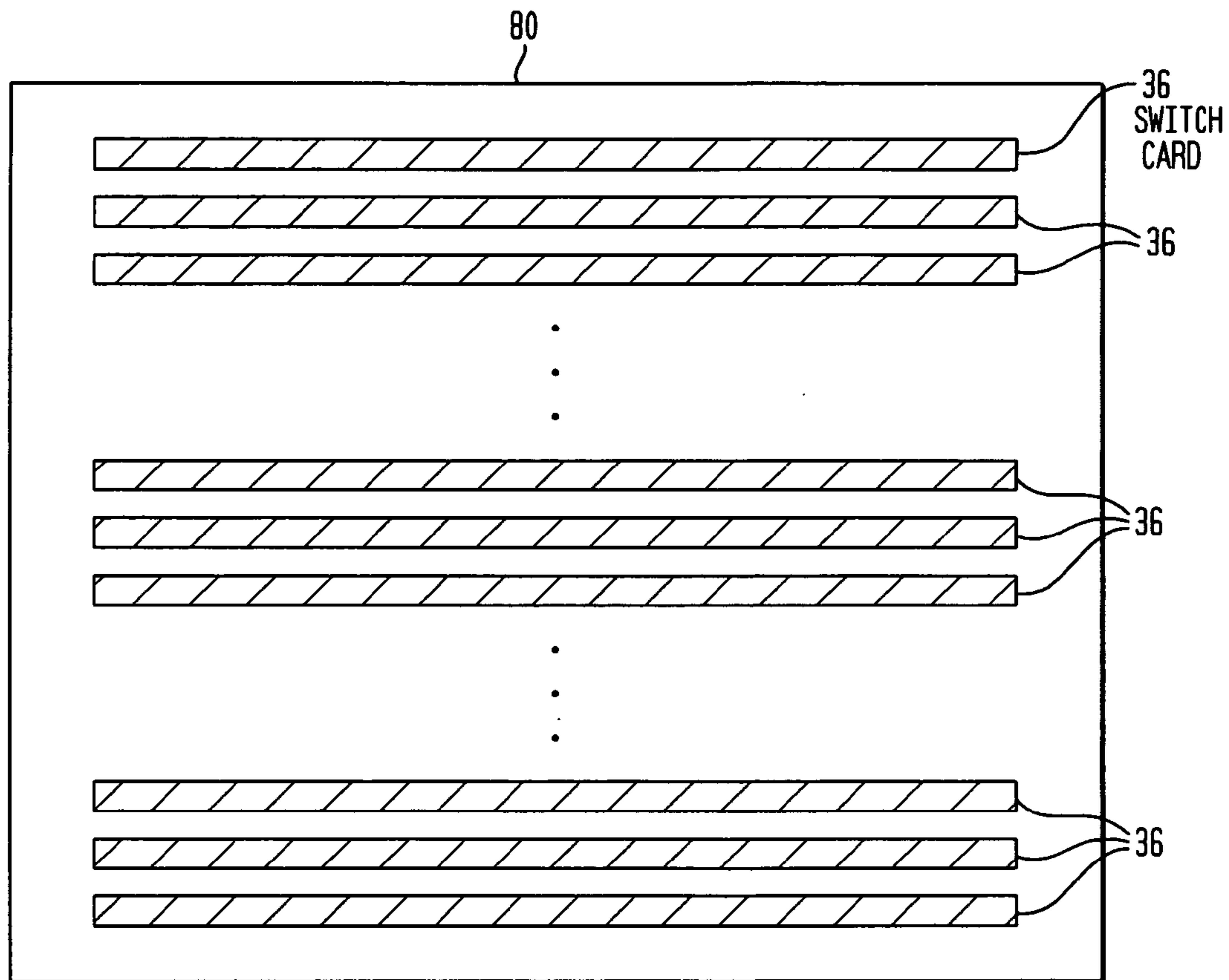
FIG. 8 SWITCH MIDPLANE
