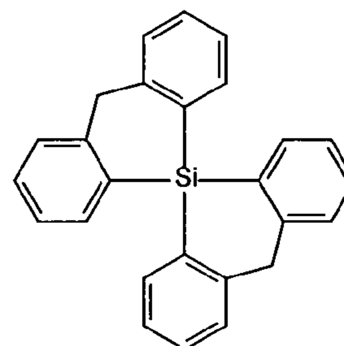
9,9-spirobissilaanthracene
