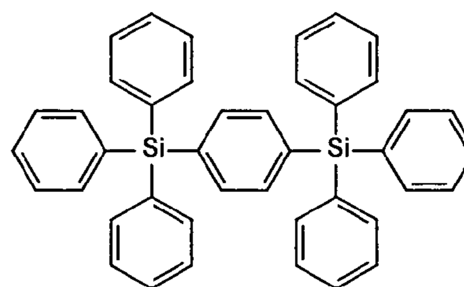
p\text{-(SiPh}_3)_2\text{Ph}
