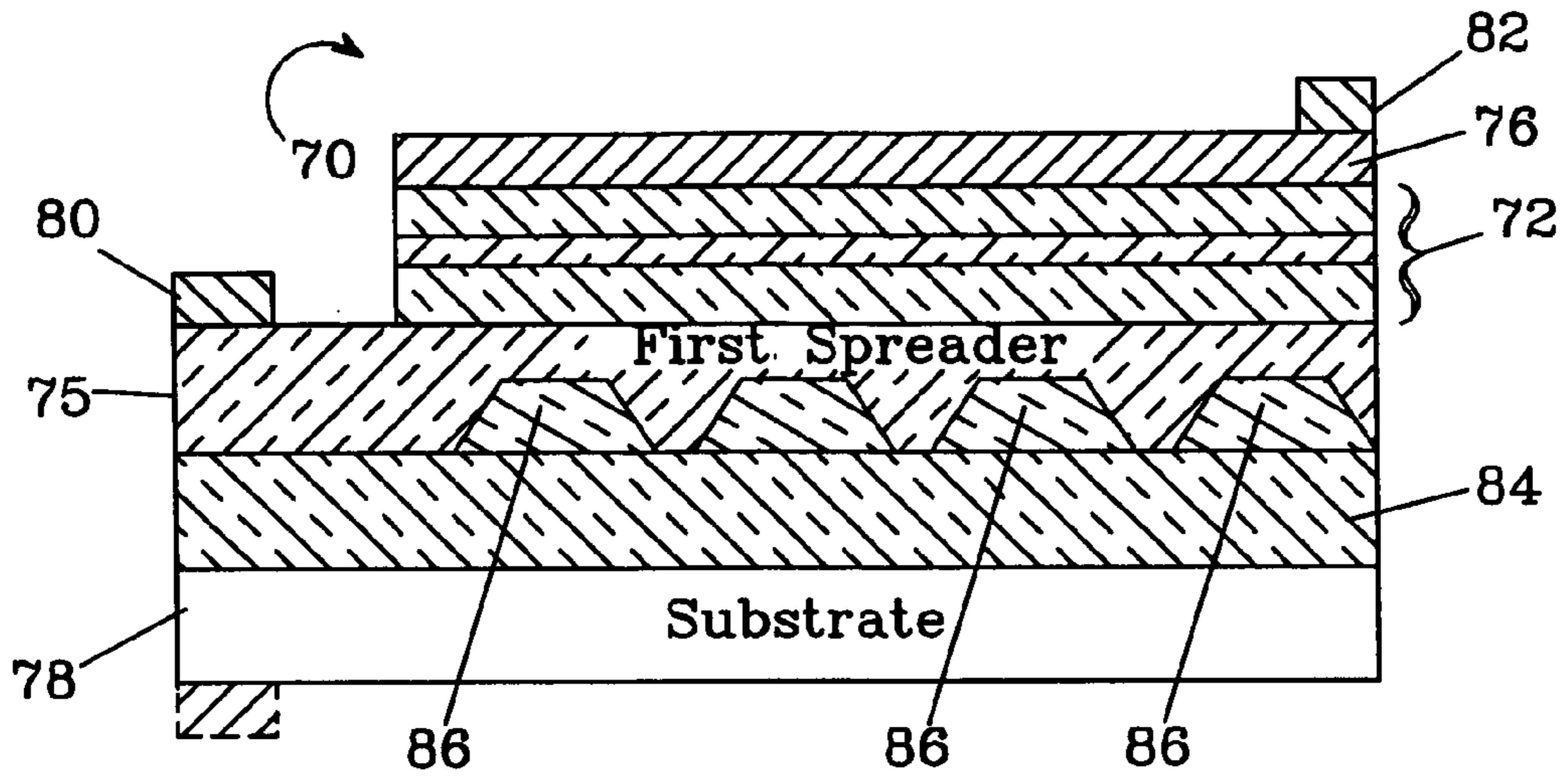
FIG. 5
