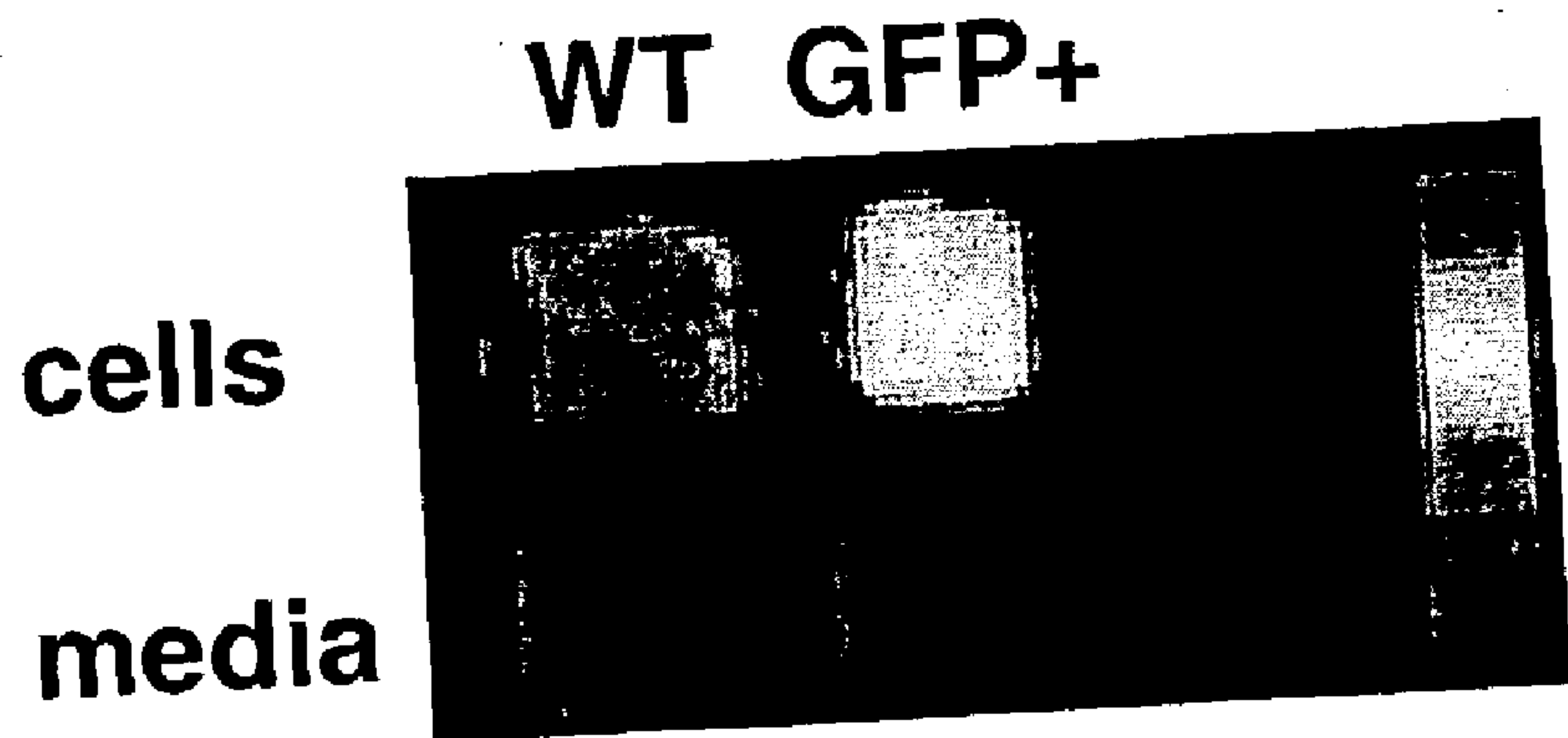
FIG. 9B WT GFP+
