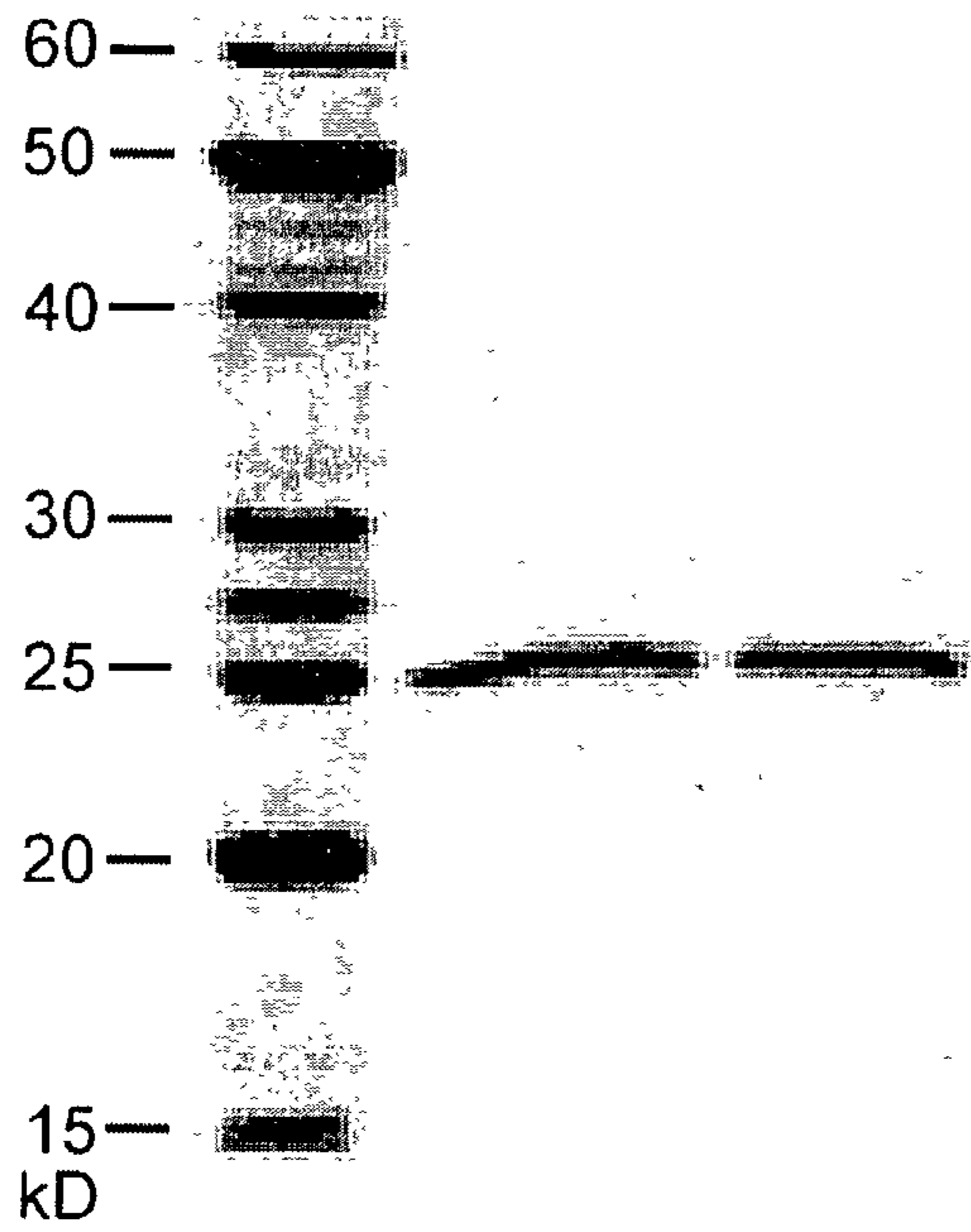
Fig. 4A mutRNA Tyr CUA + + + - + TyrRS wt SS12 SS12 SS12 - L-3-(2-naphthyl)-Ala - + - + +
