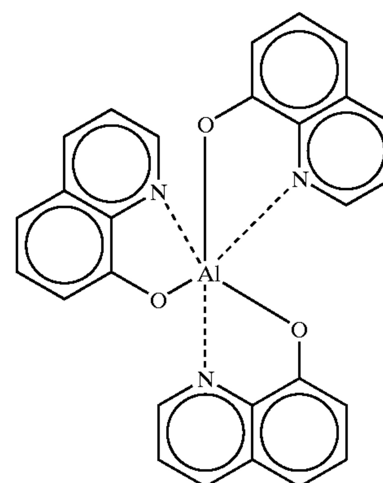
Alq3
