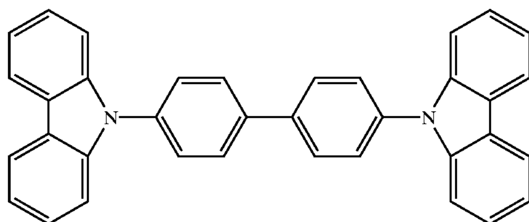
CBP
