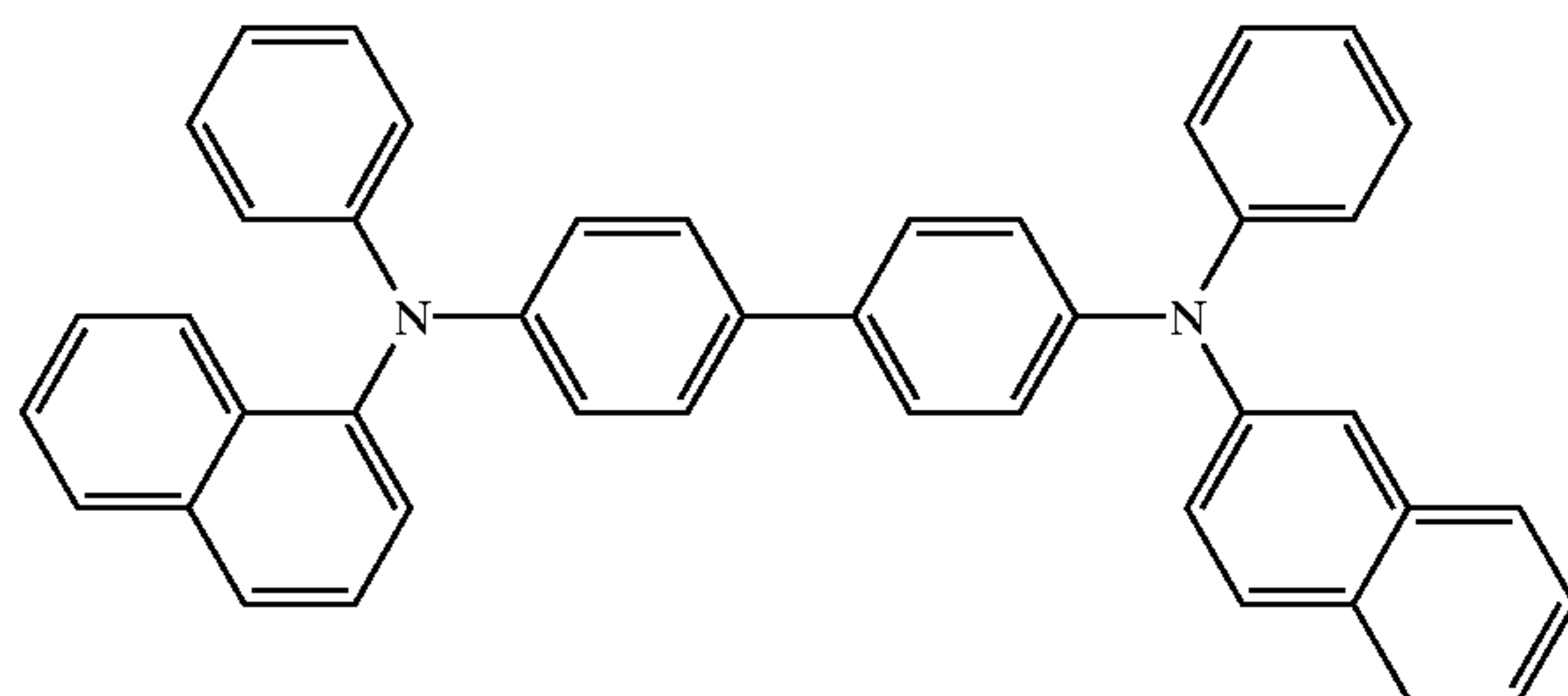
\alpha -NPD
