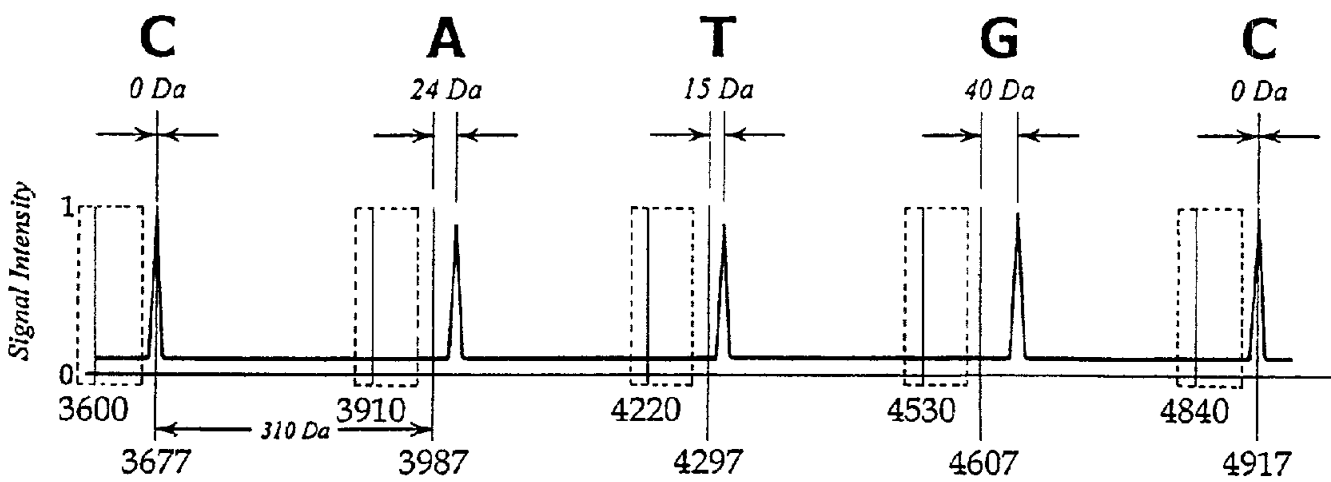
Mass (daltons) FIG. 2b
