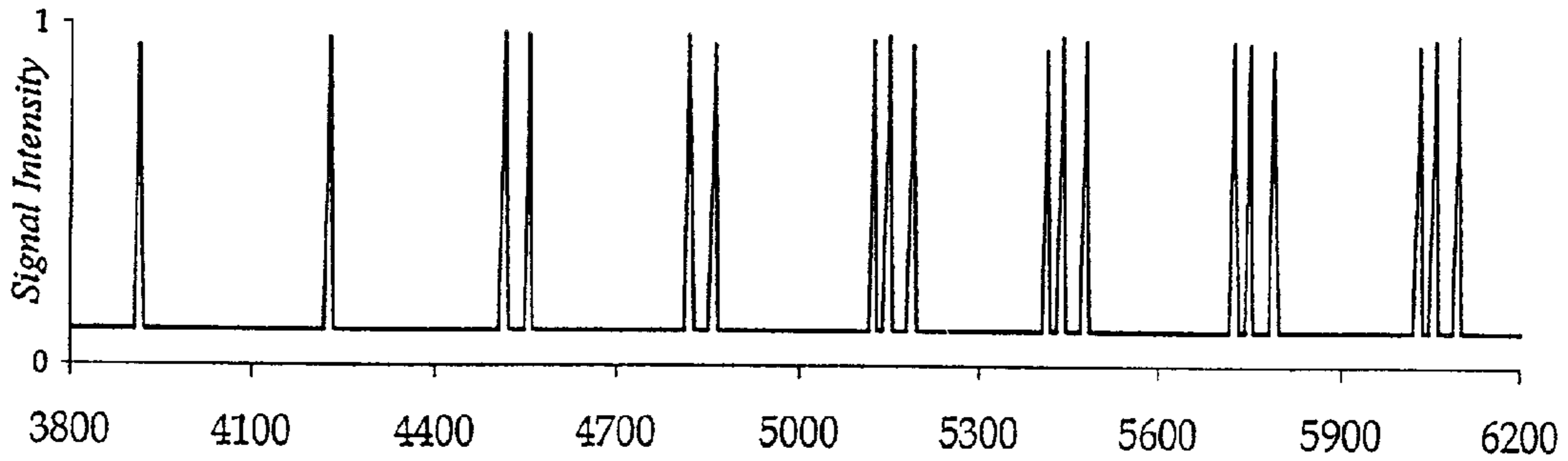
FIG. 6b Mass (daltons)
