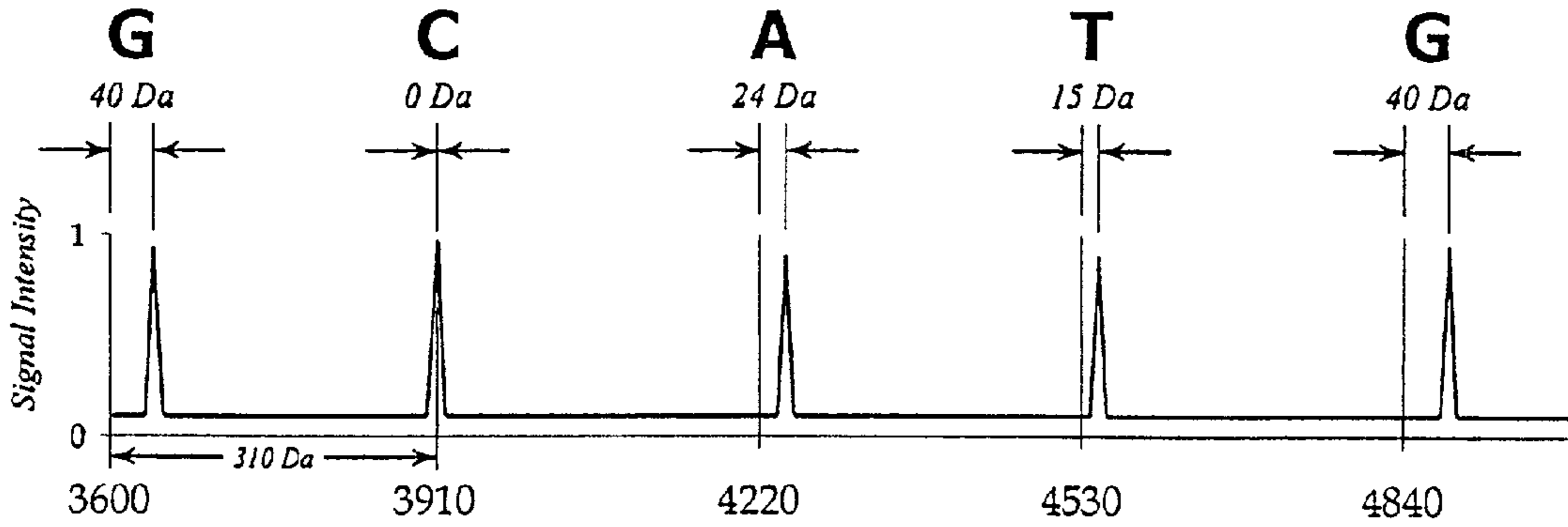
Mass (daltons) FIG. 2a
