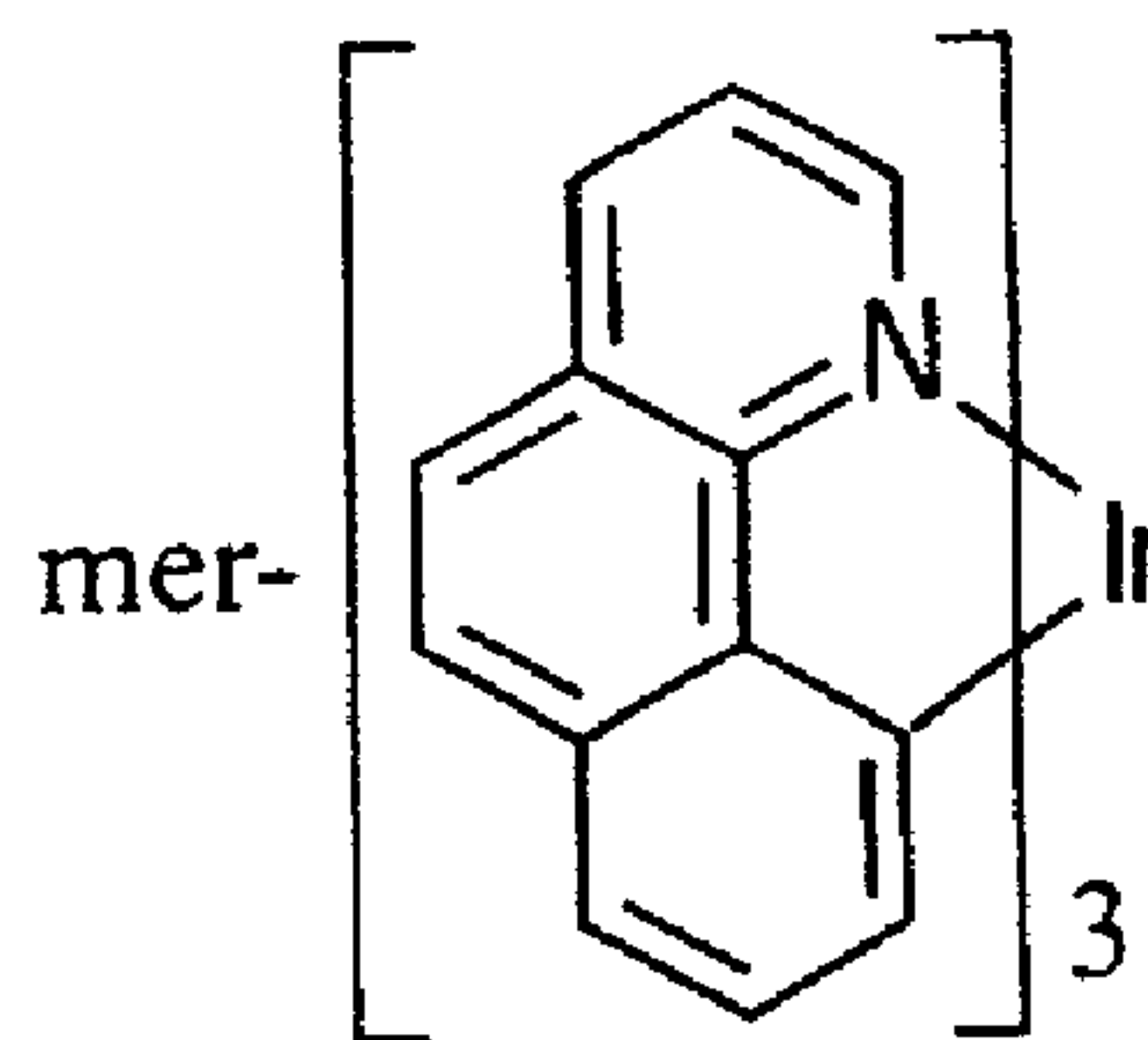
mer-Irbq
