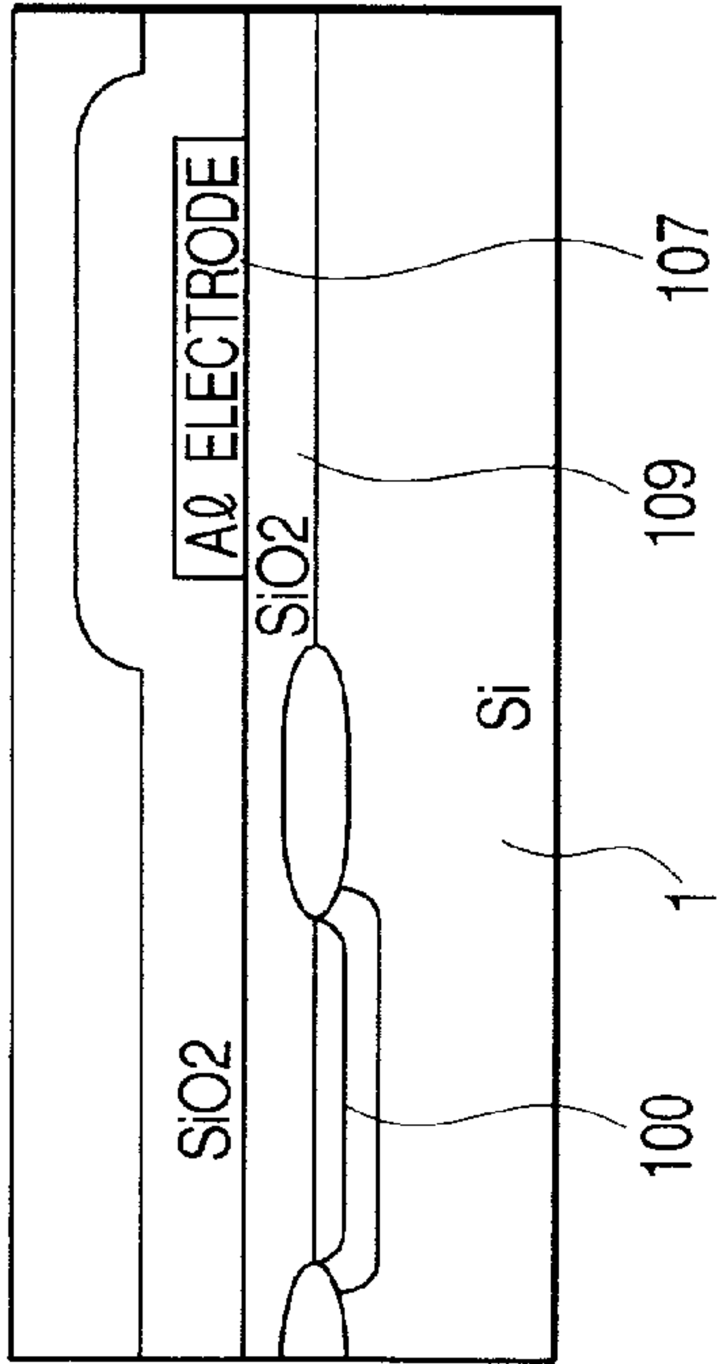
FIG. 19A
