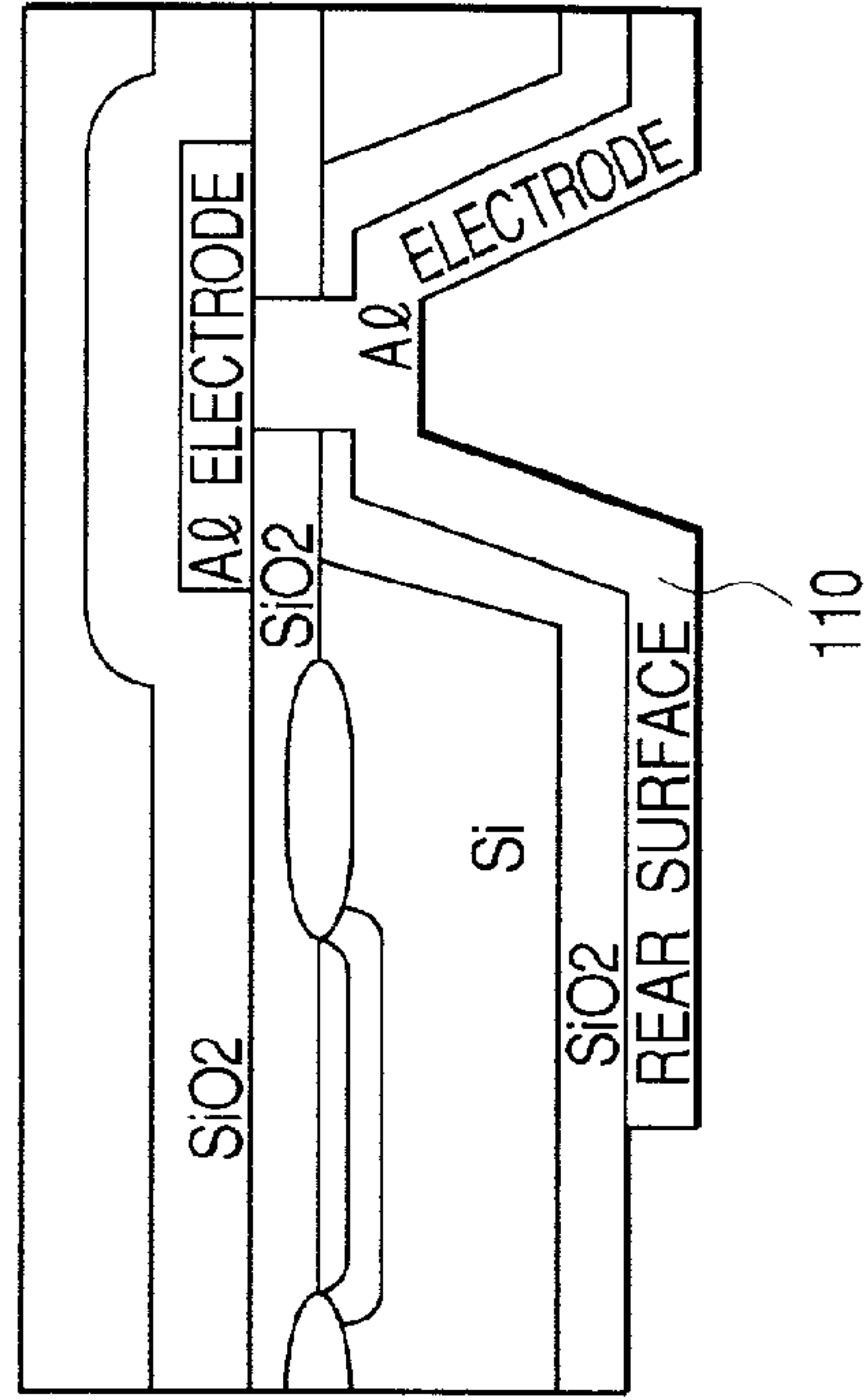
FIG. 19D
