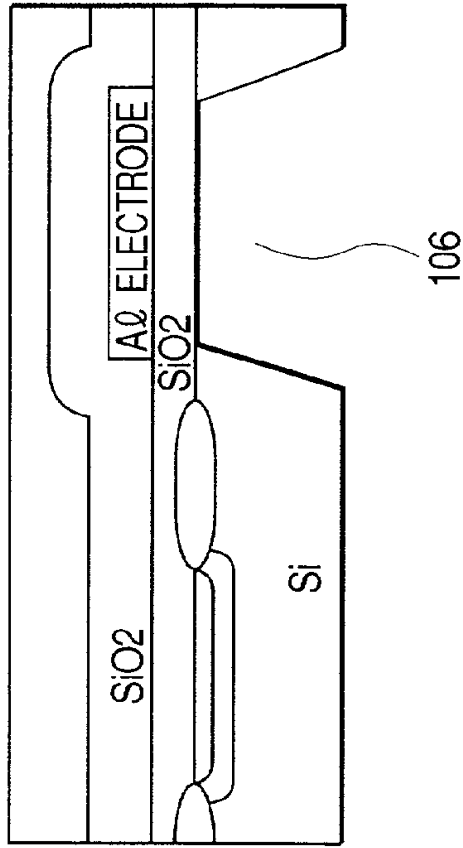
FIG. 19B
