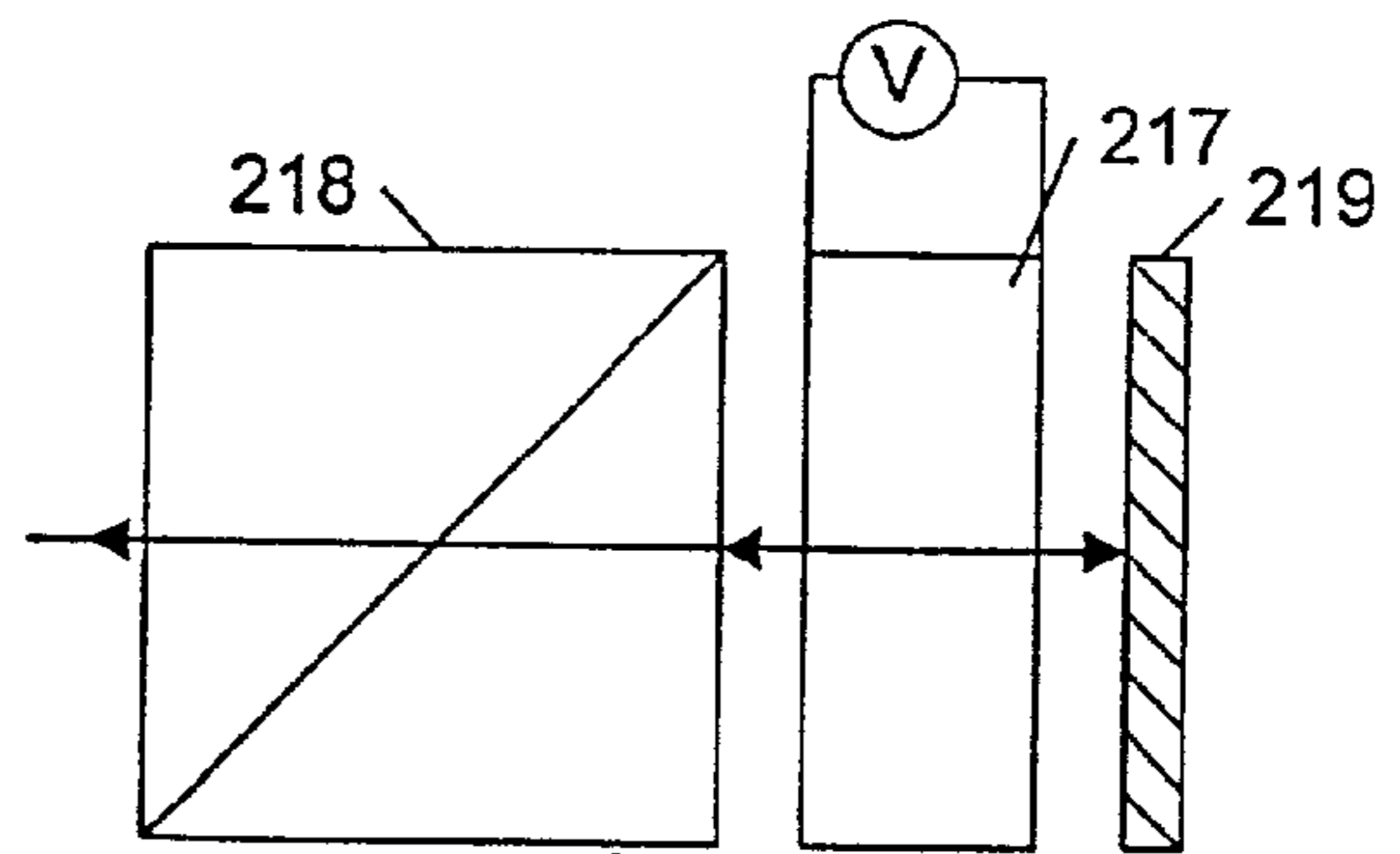
RETRO-REFLECTED
