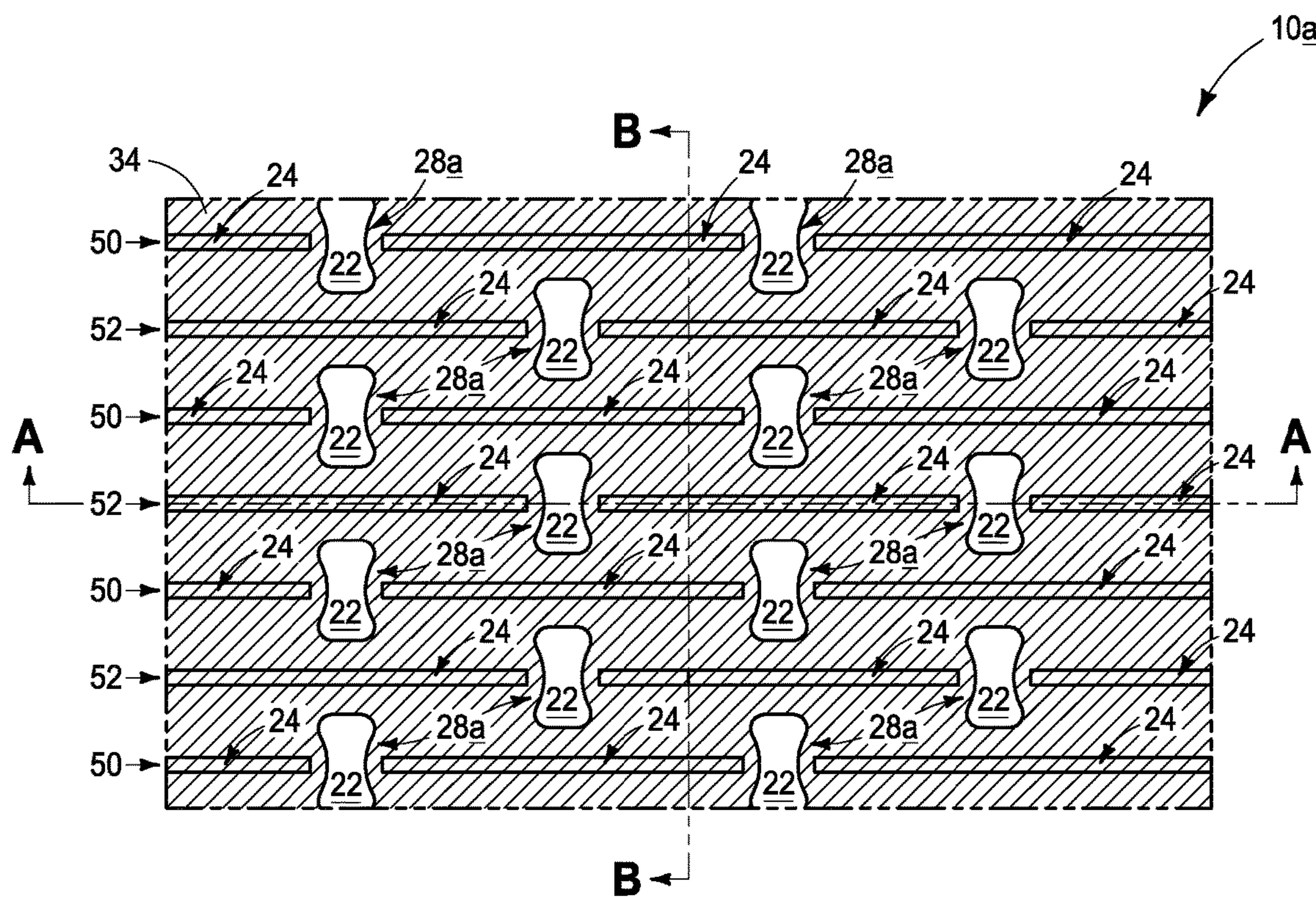
FIG. 28 (C-C)
