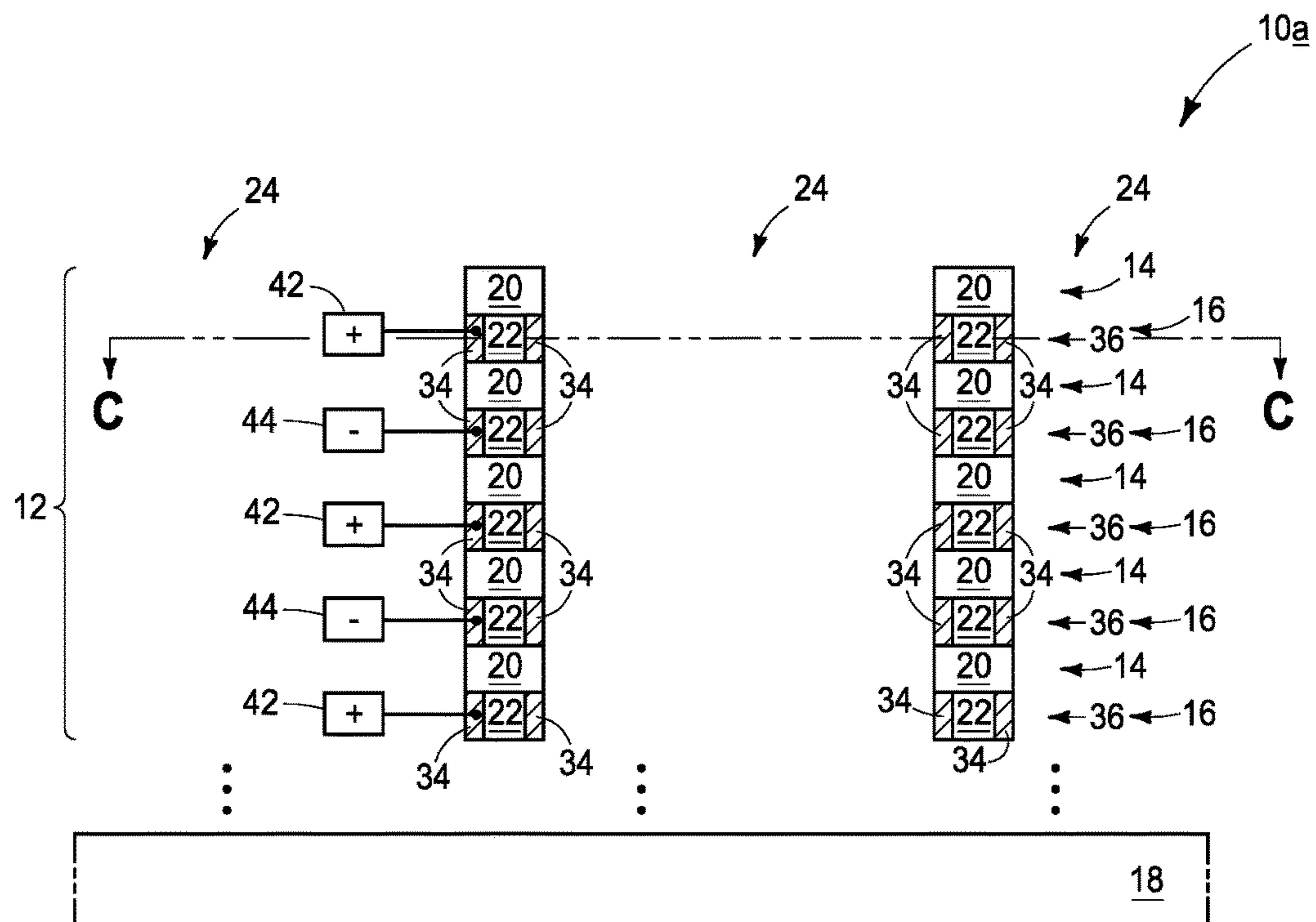
FIG. 35 (A-A)
