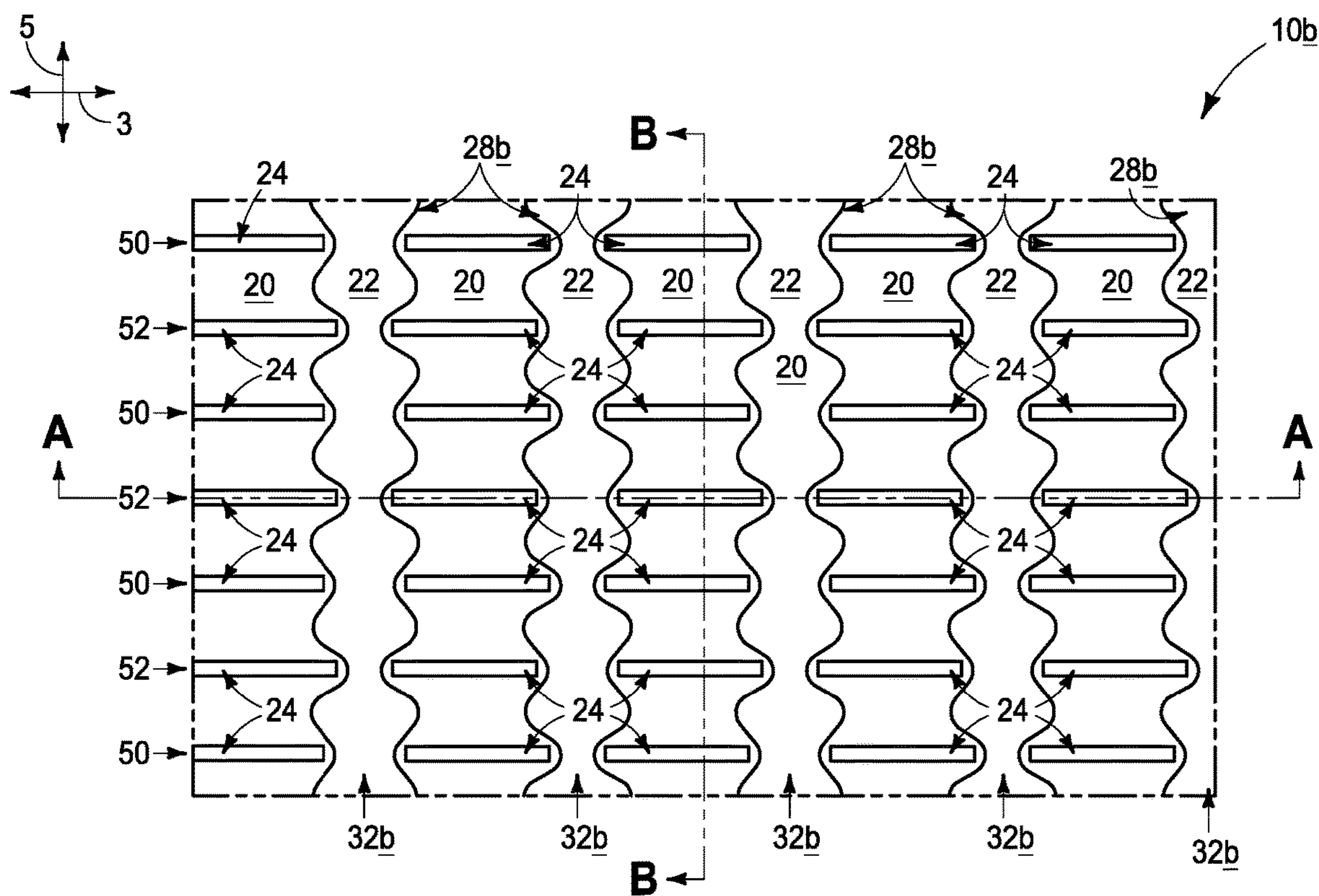
FIG. 40 (C-C)
