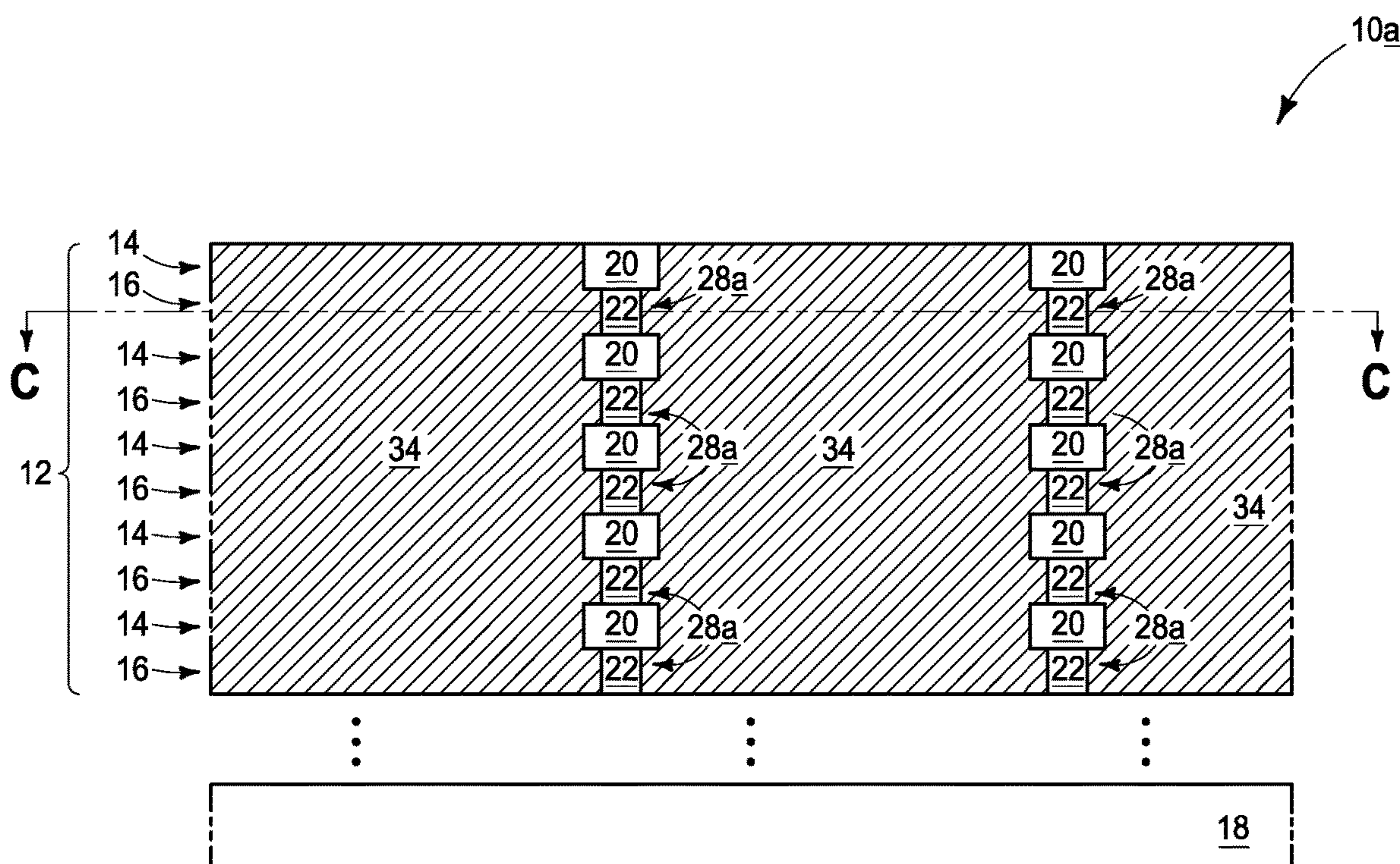
FIG. 29 (A-A)
