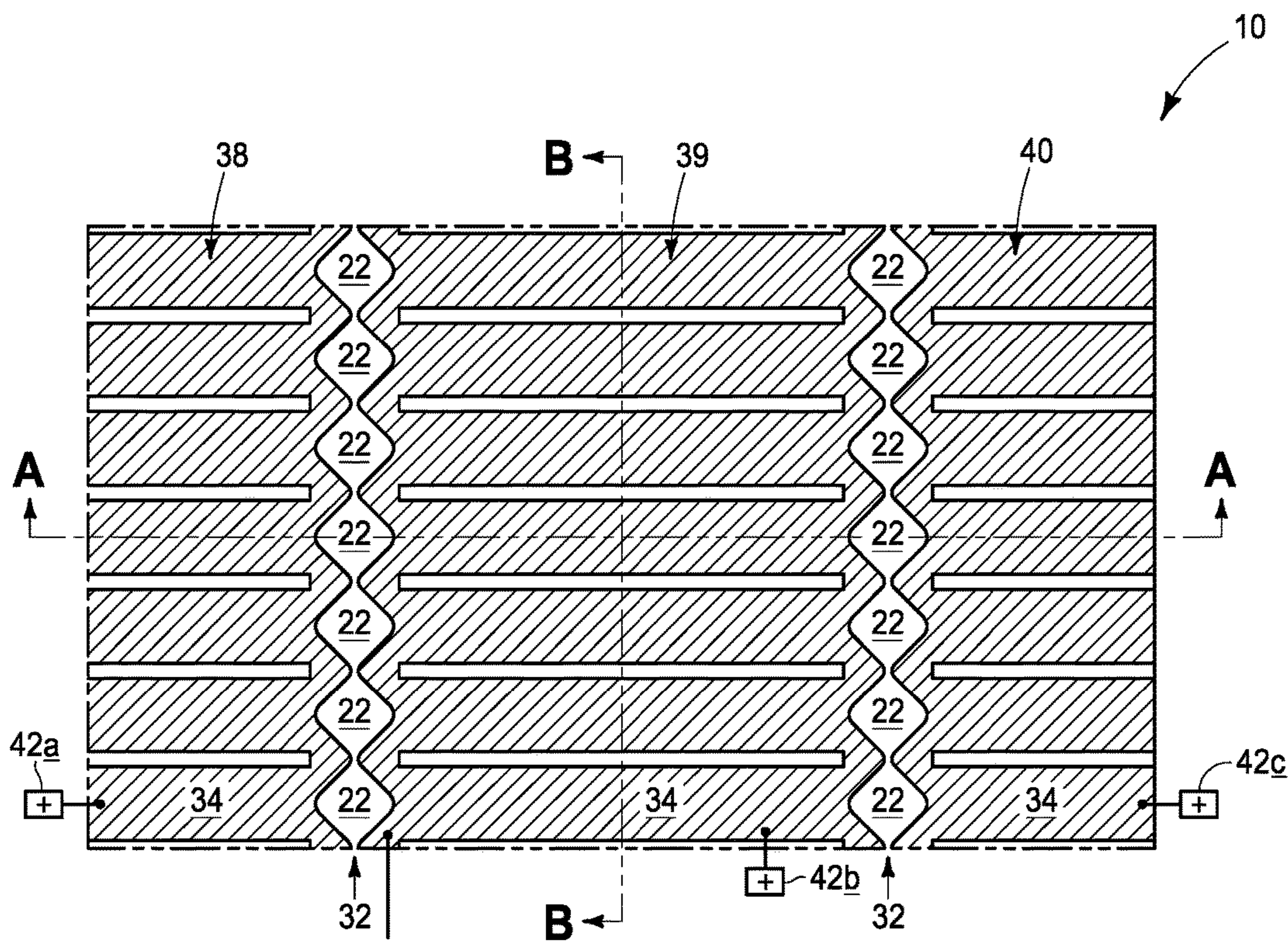
FIG. 19 (C-C)
