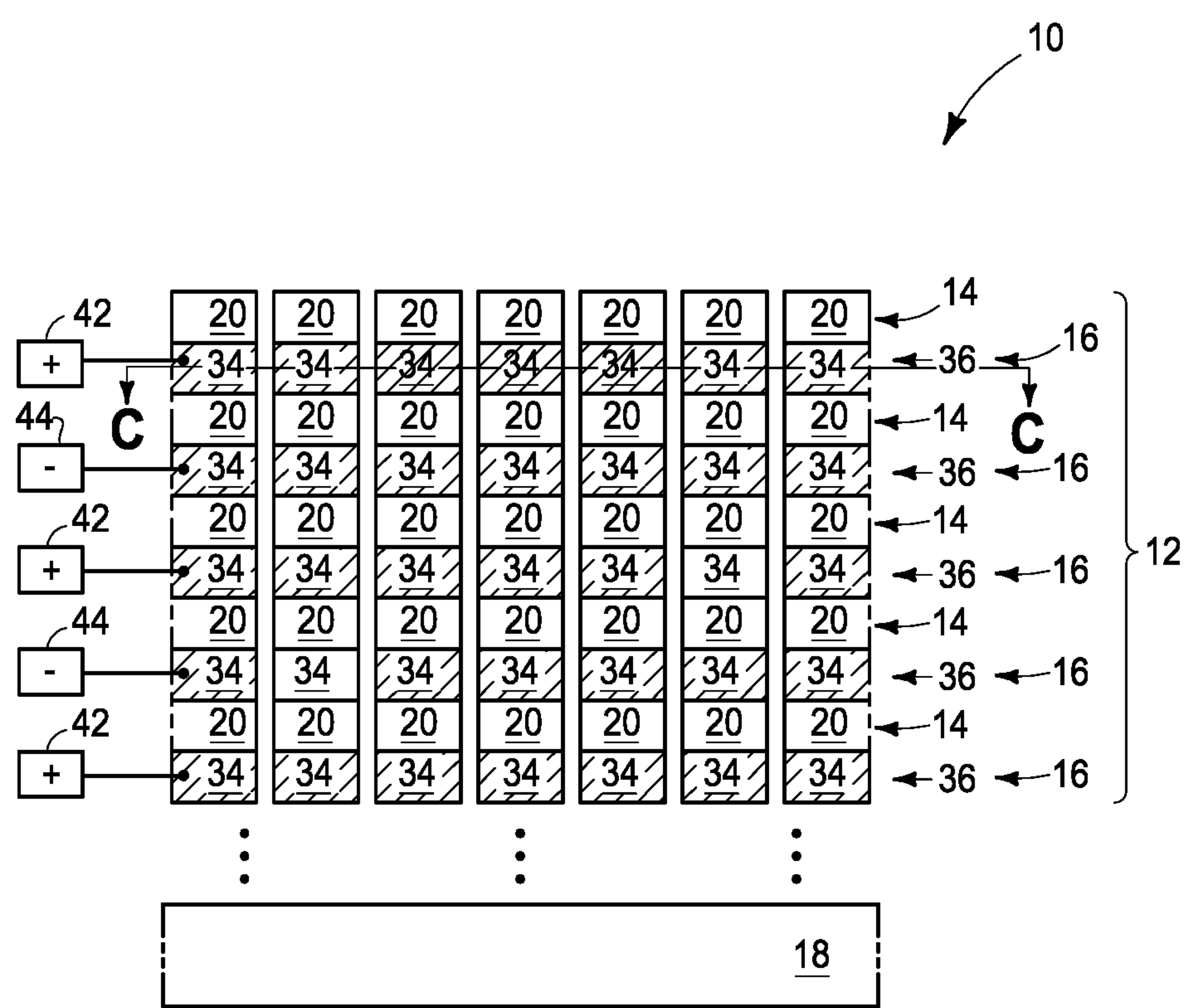
FIG. 18 (B-B)
