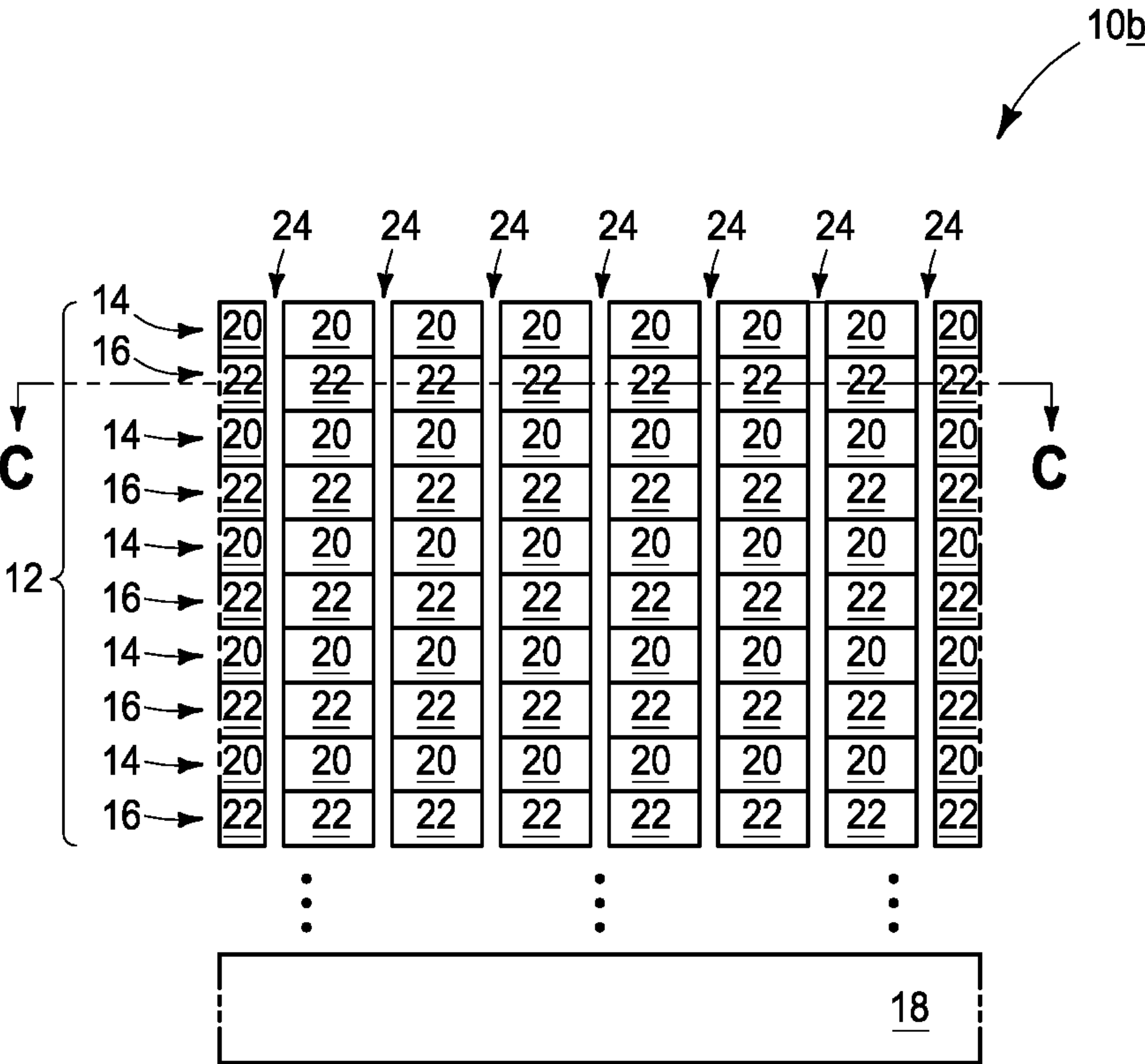
FIG. 42 (B-B)
