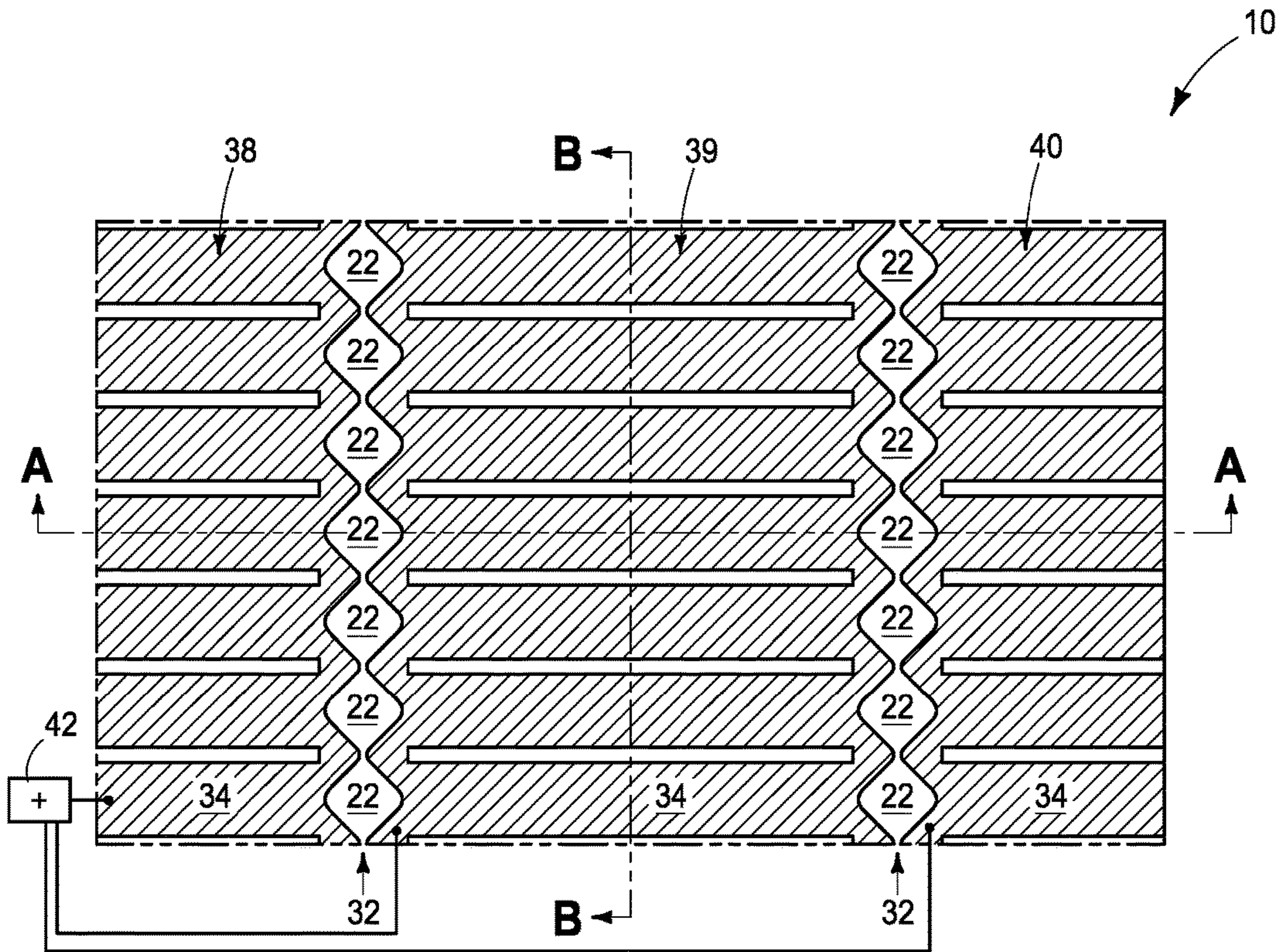
FIG. 16 (C-C)
