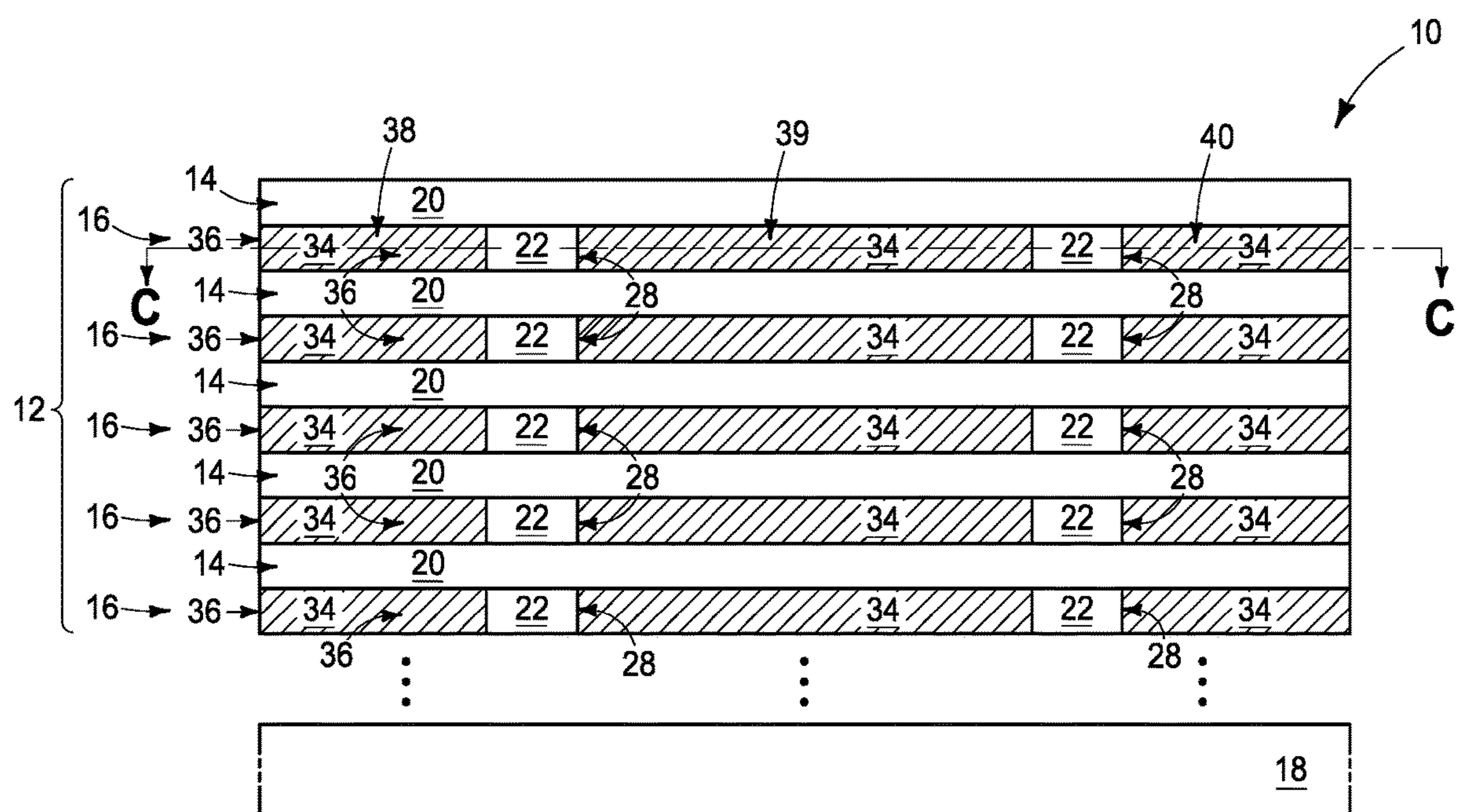
FIG. 14 (A-A)
