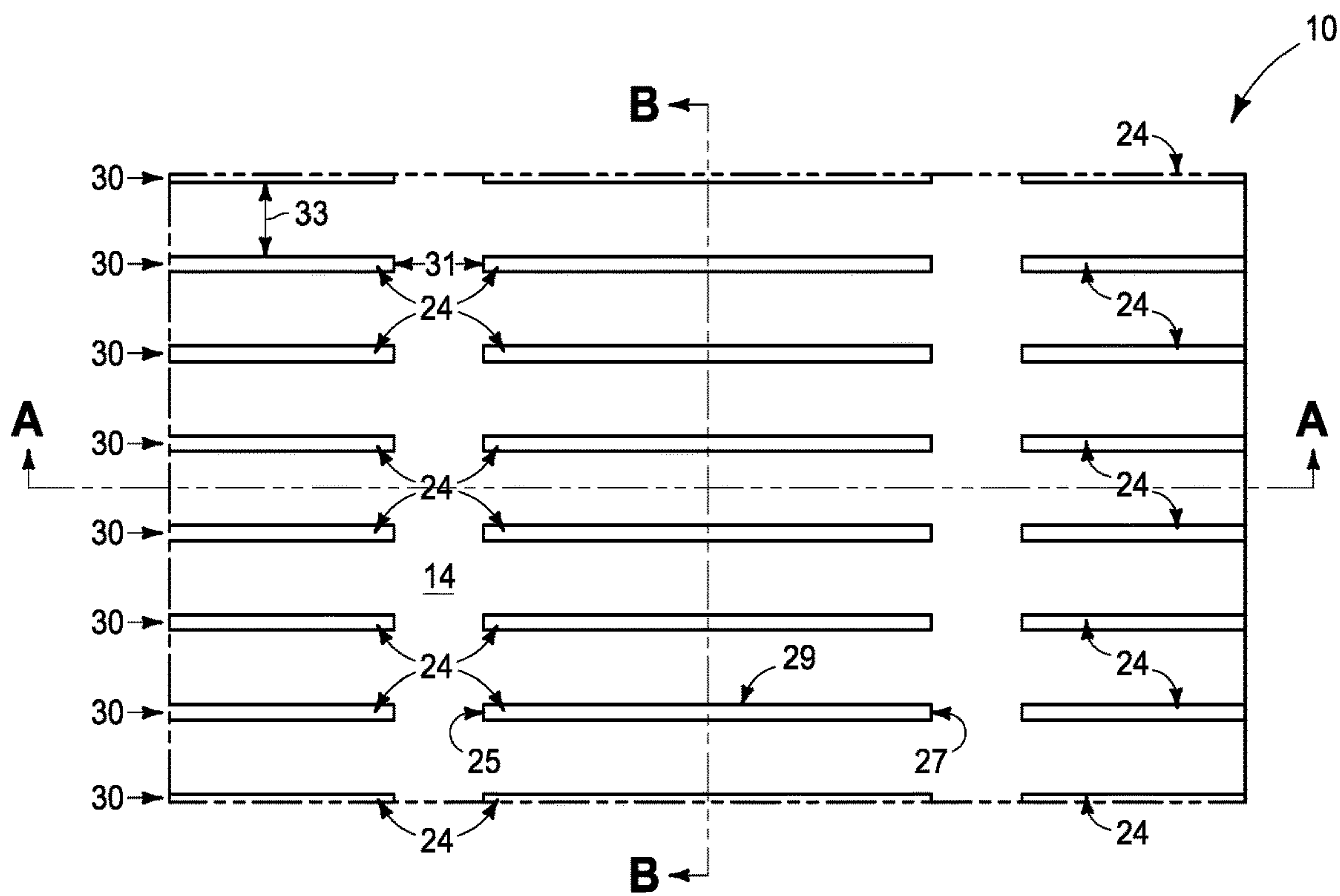
FIG. 4 (C-C)
