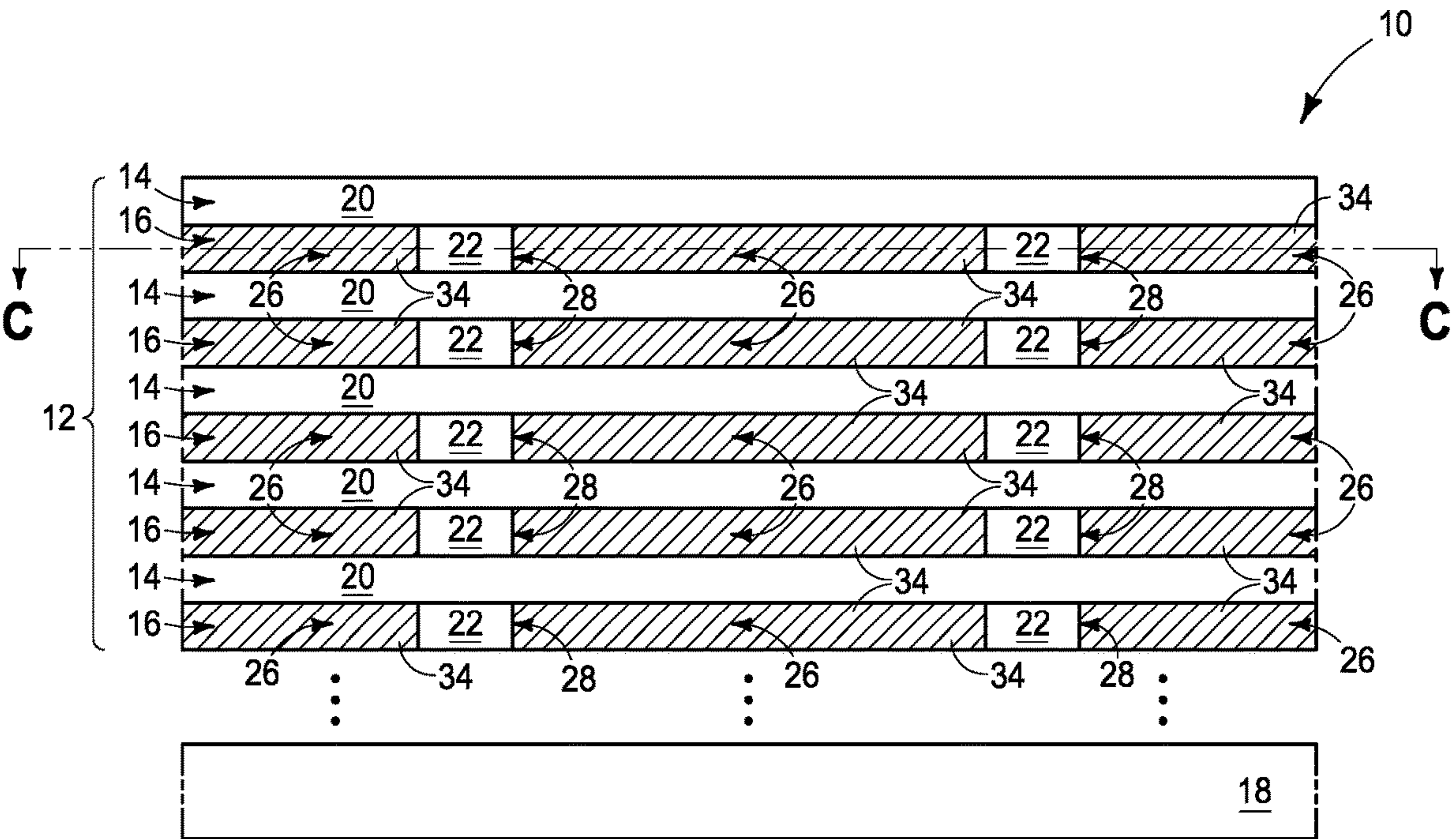
FIG. 11 (A-A)
