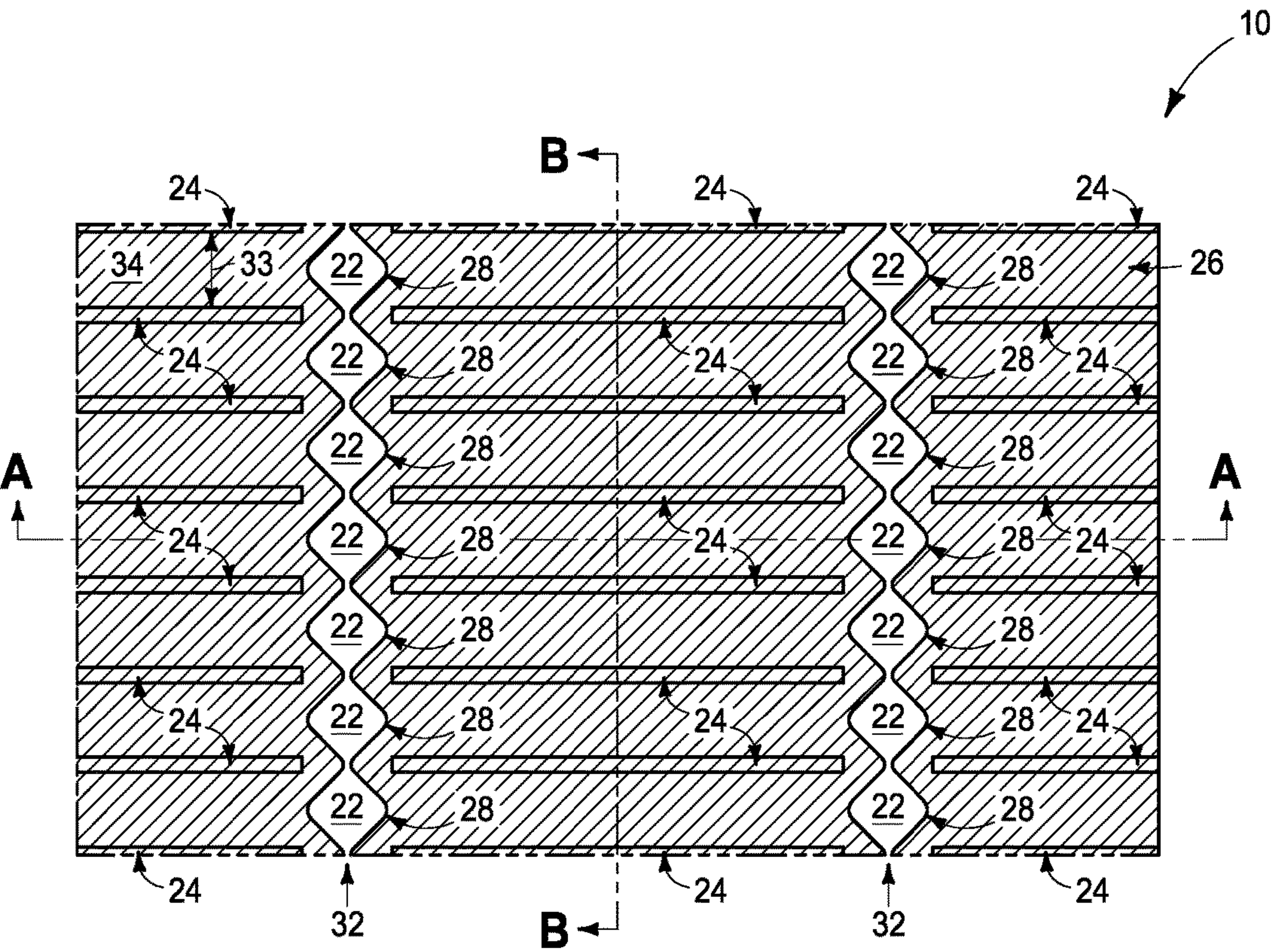
FIG. 10 (C-C)
