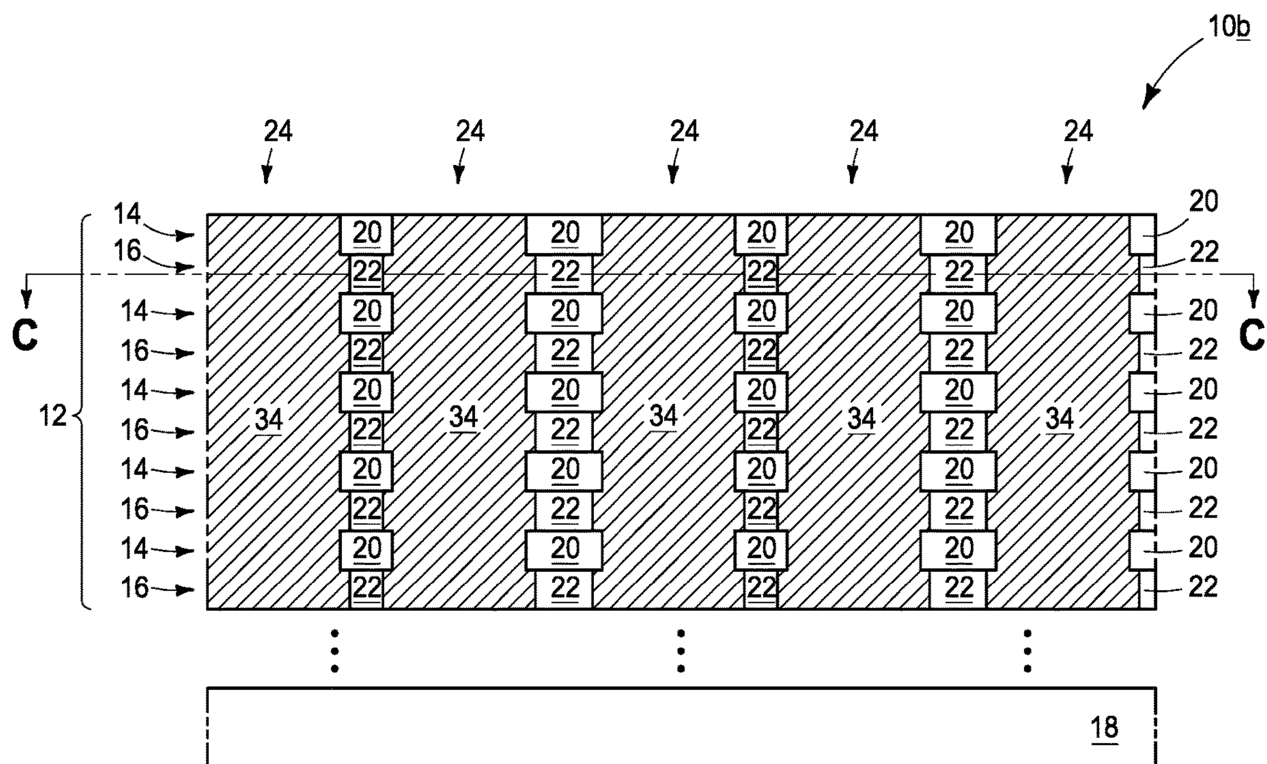
FIG. 44 (A-A)
