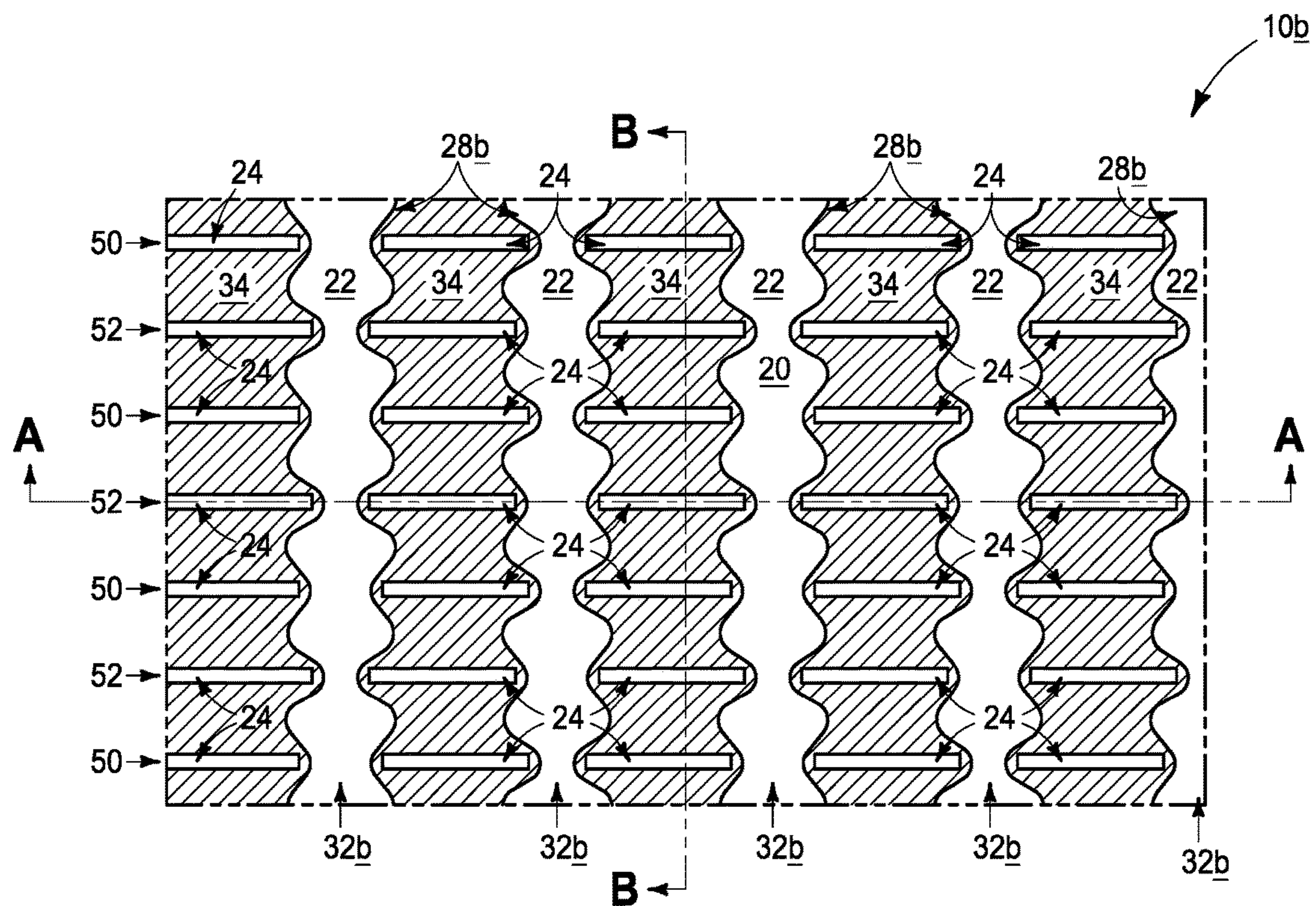
FIG. 43 (C-C)
