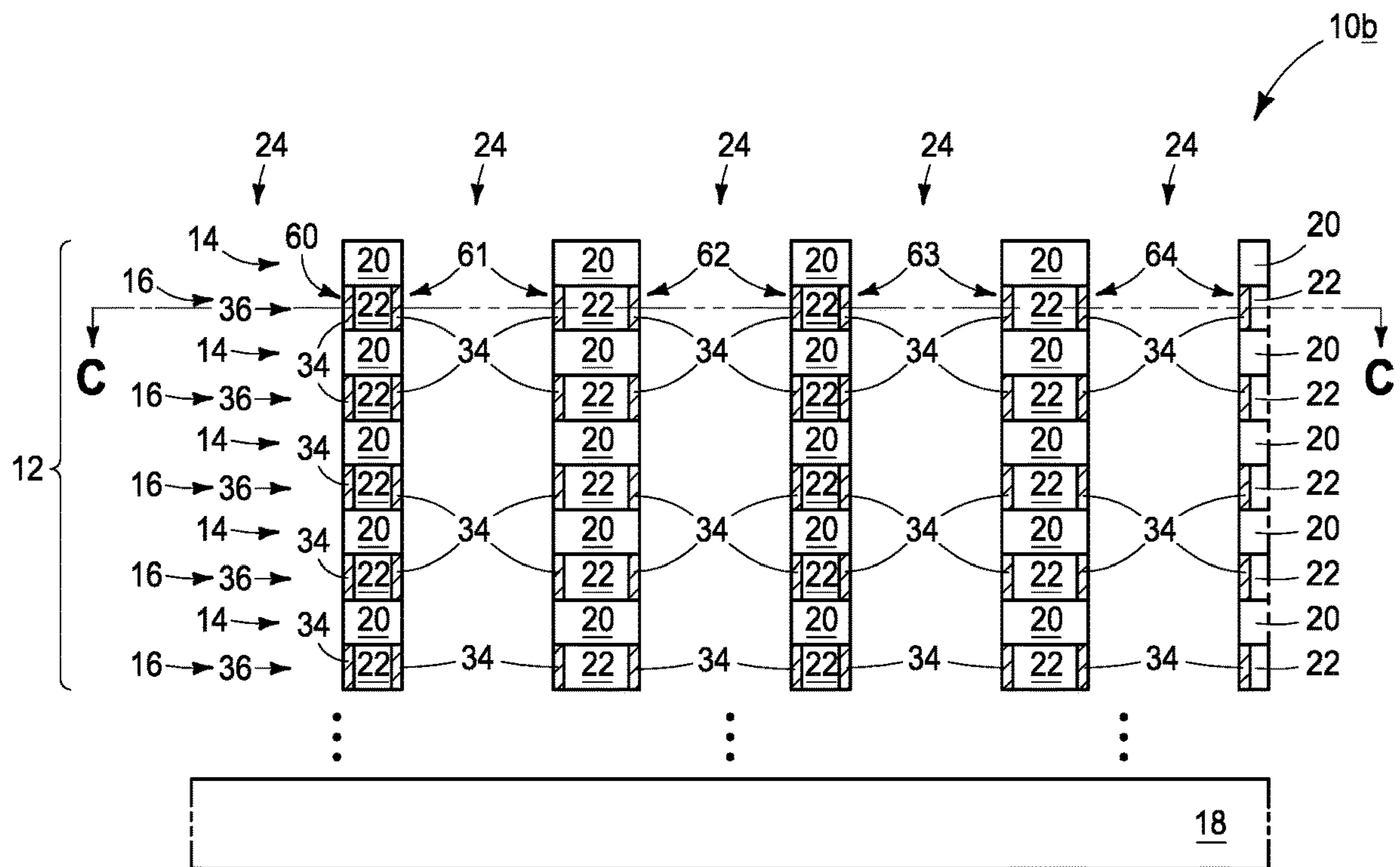
FIG. 47 (A-A)
