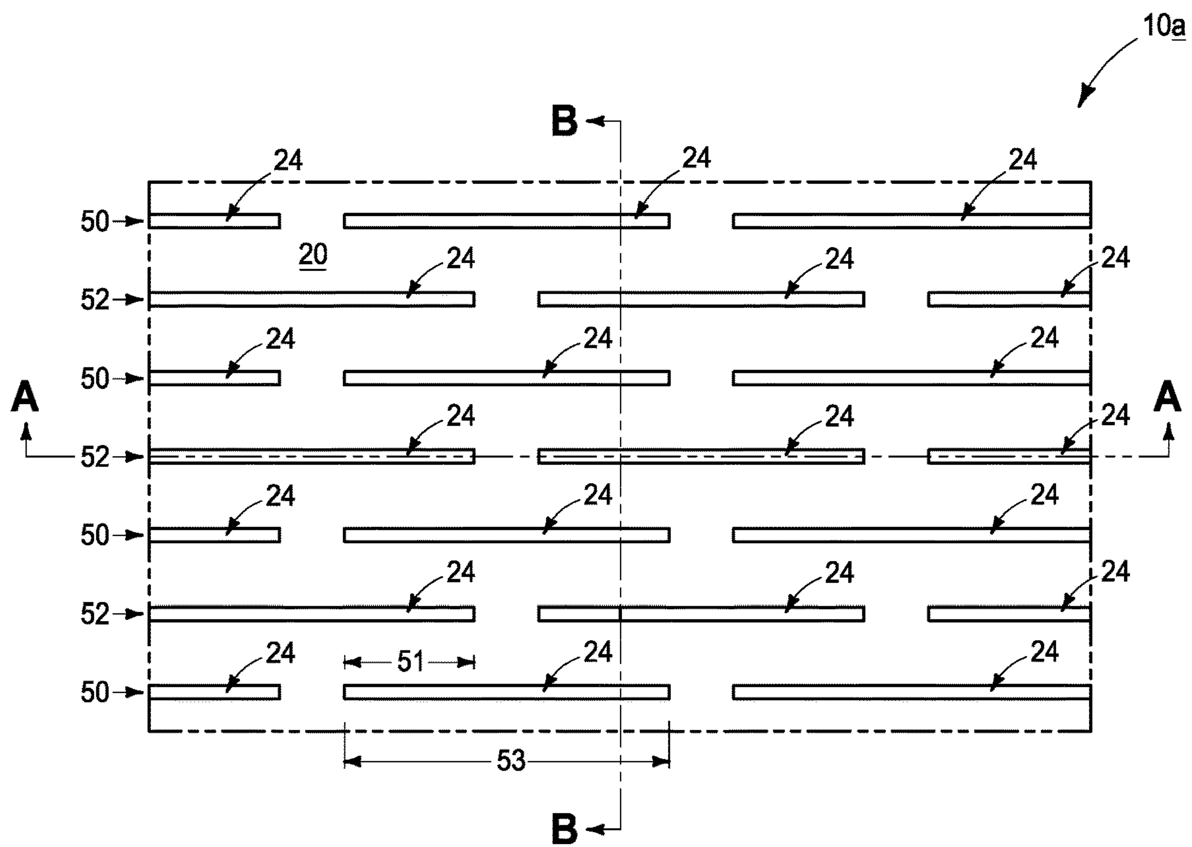
FIG. 22 (C-C)
