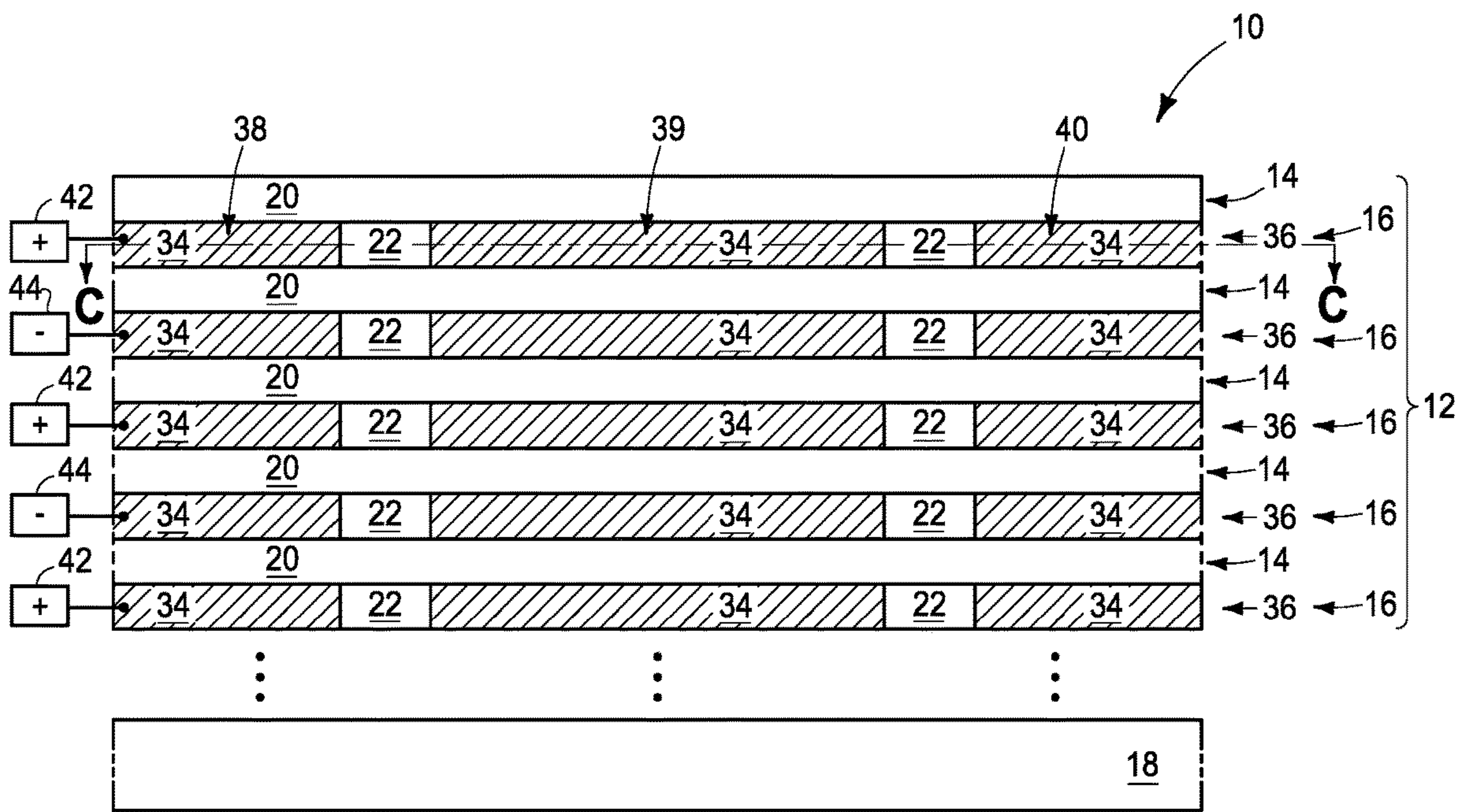
FIG. 17 (A-A)
