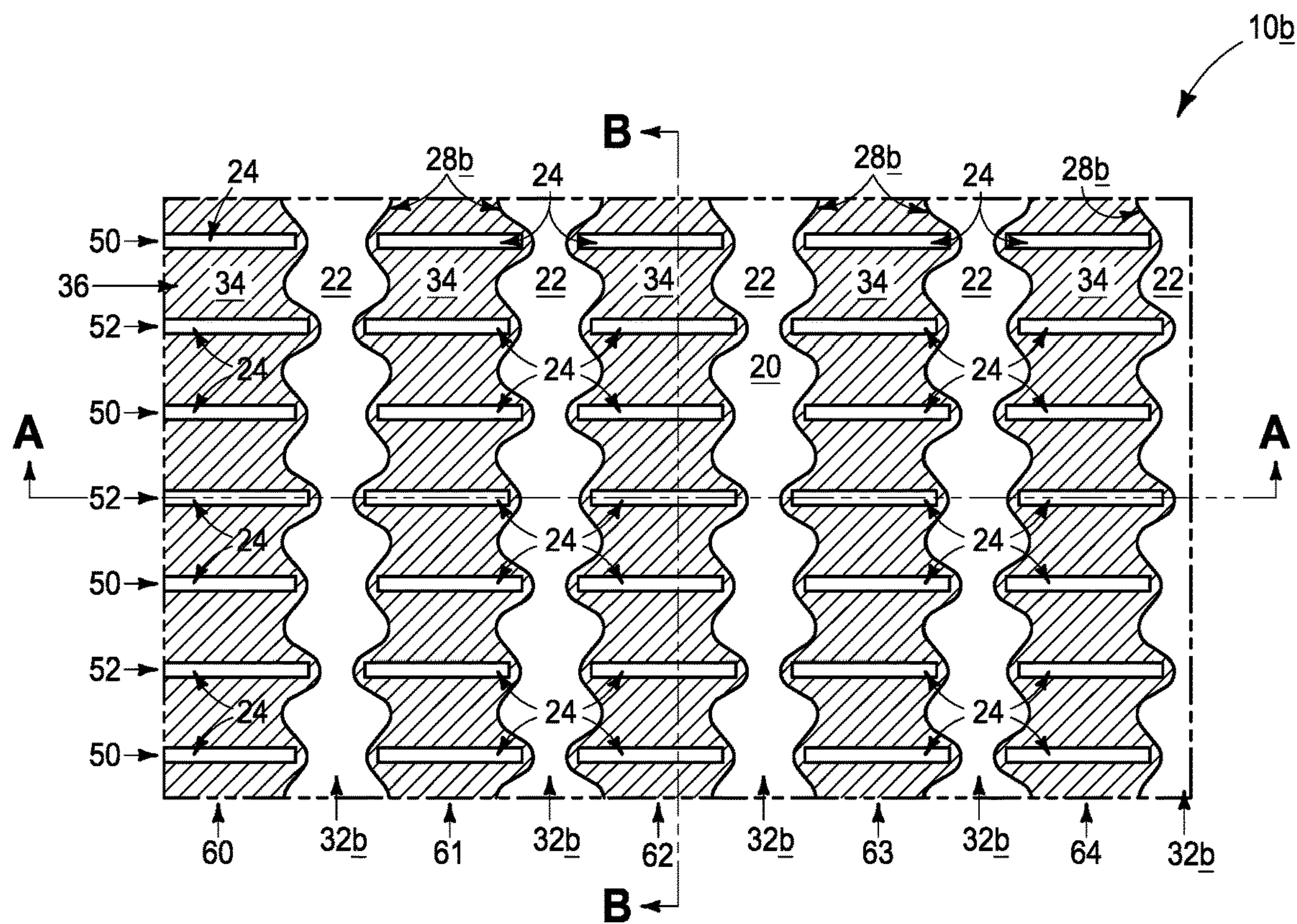
FIG. 46 (C-C)
