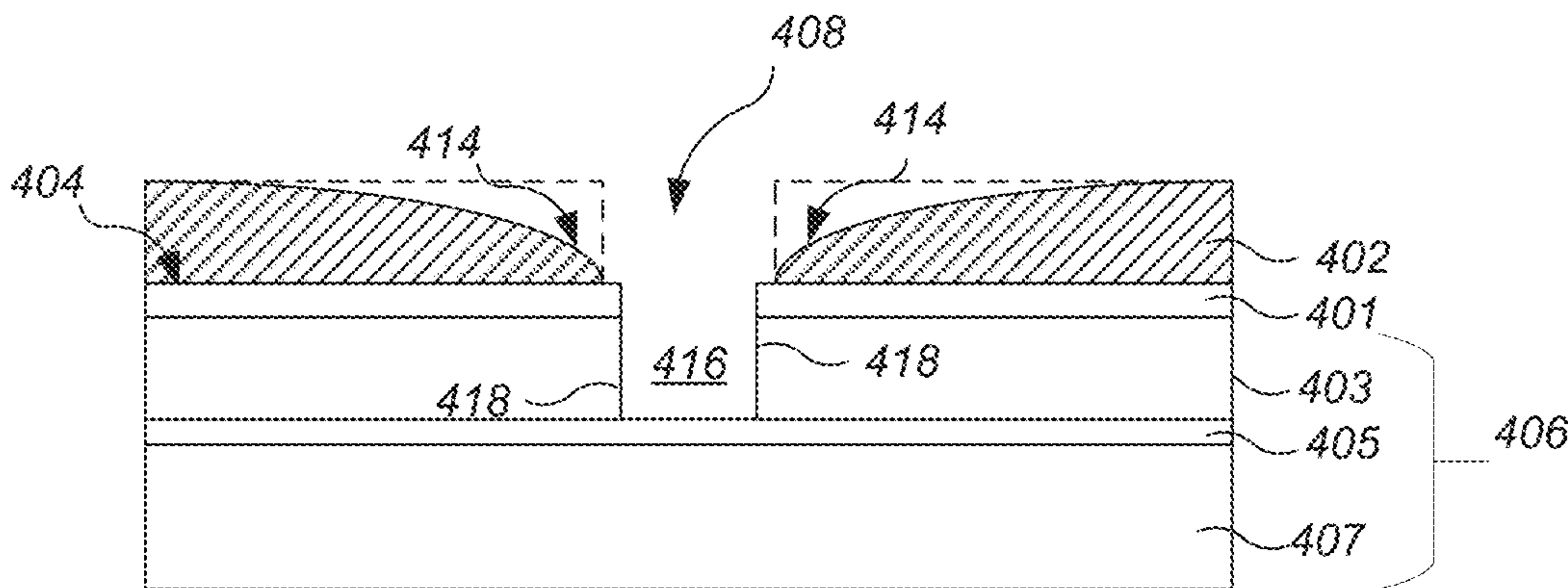
FIG. 4C
