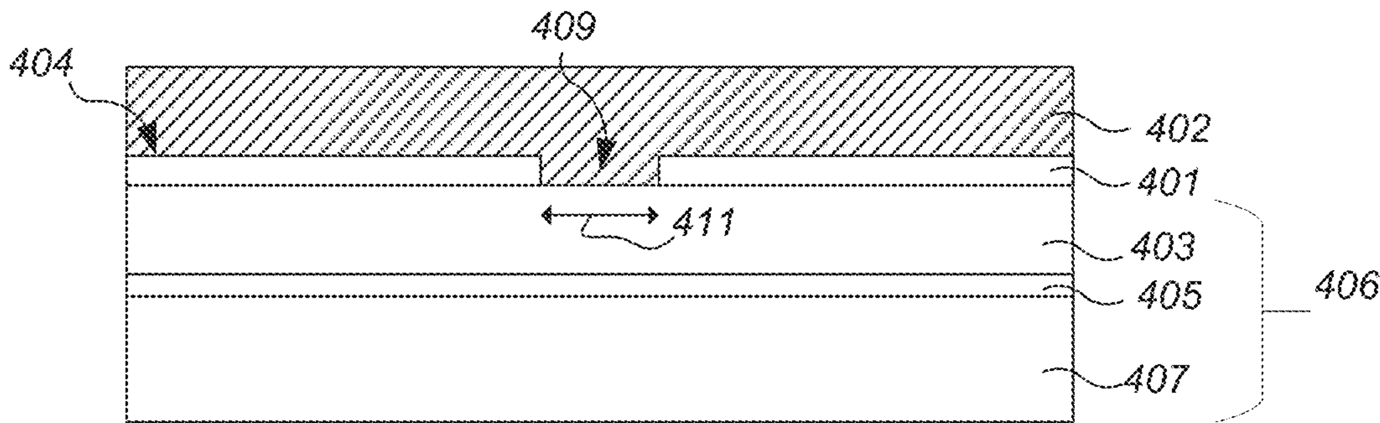
FIG. 4A
