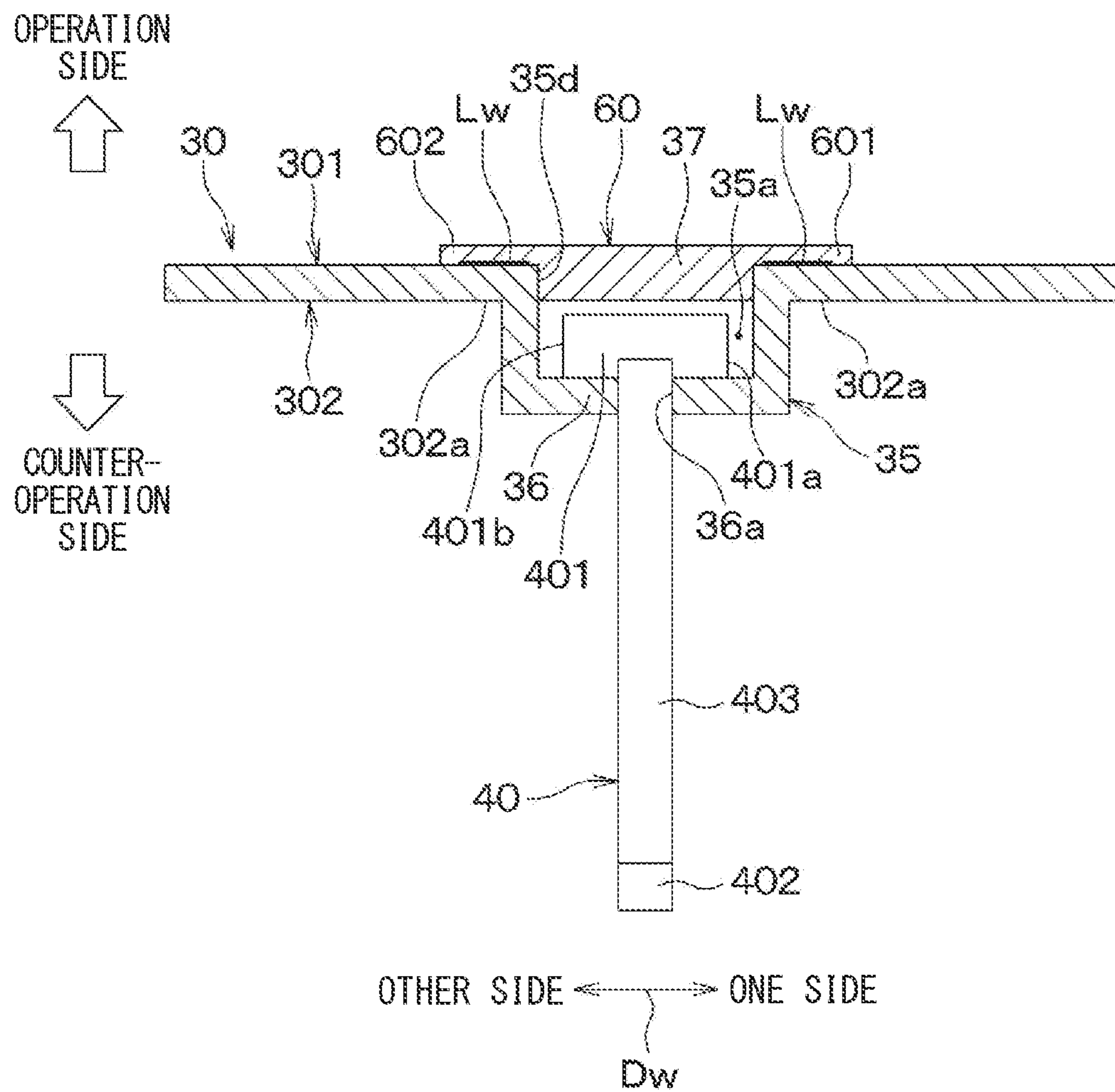
FIG. 16
