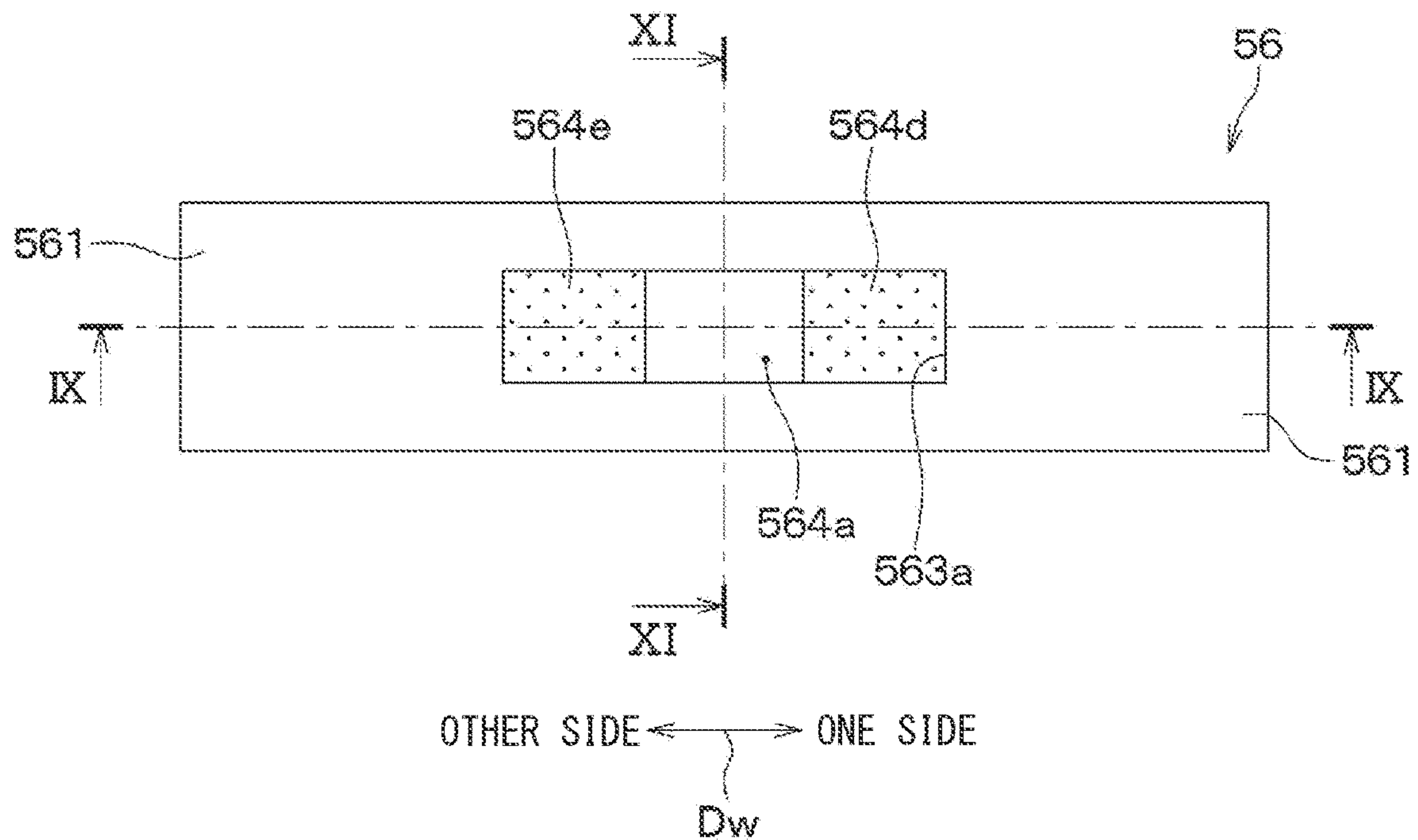
FIG. 8
