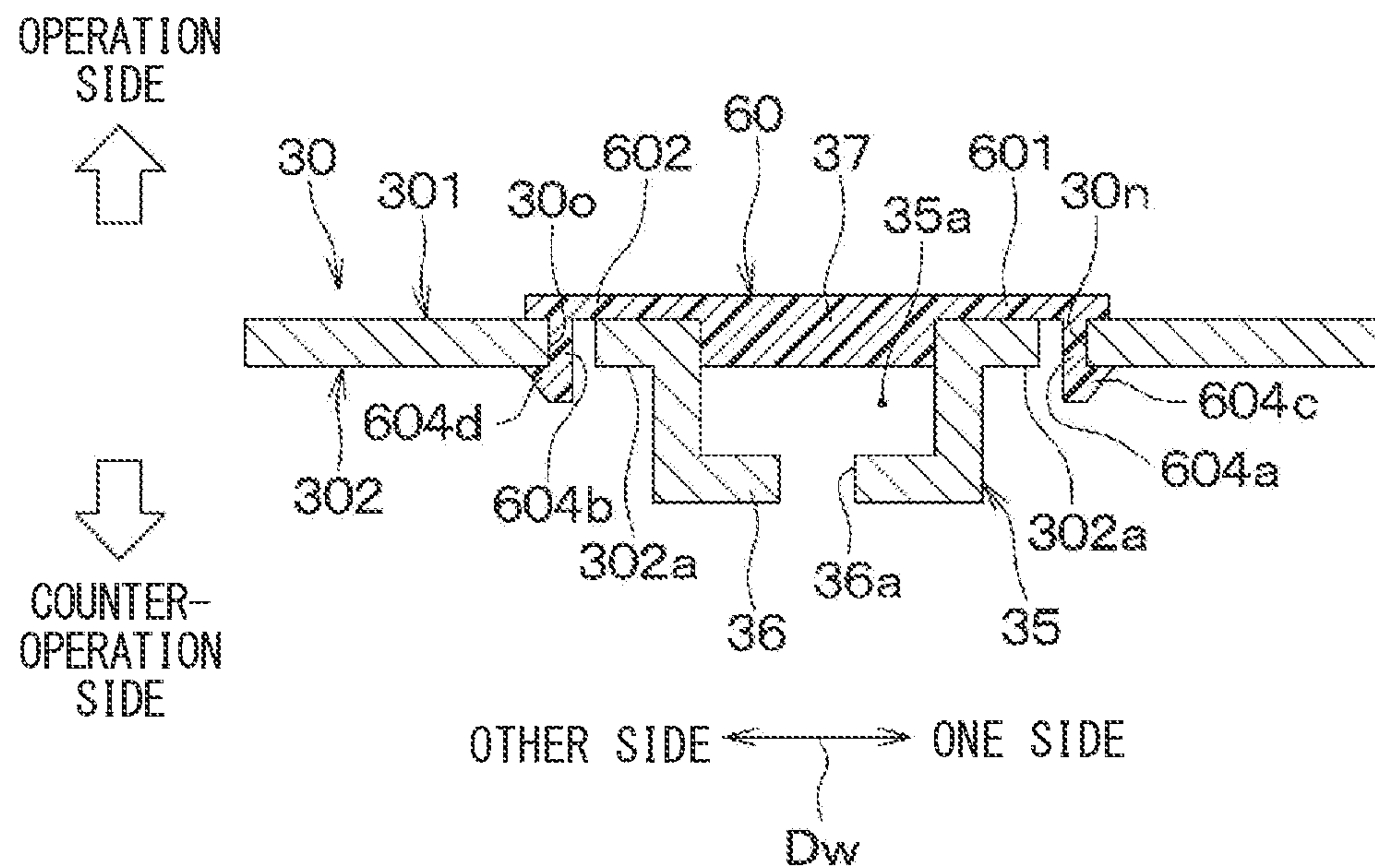
FIG. 35
