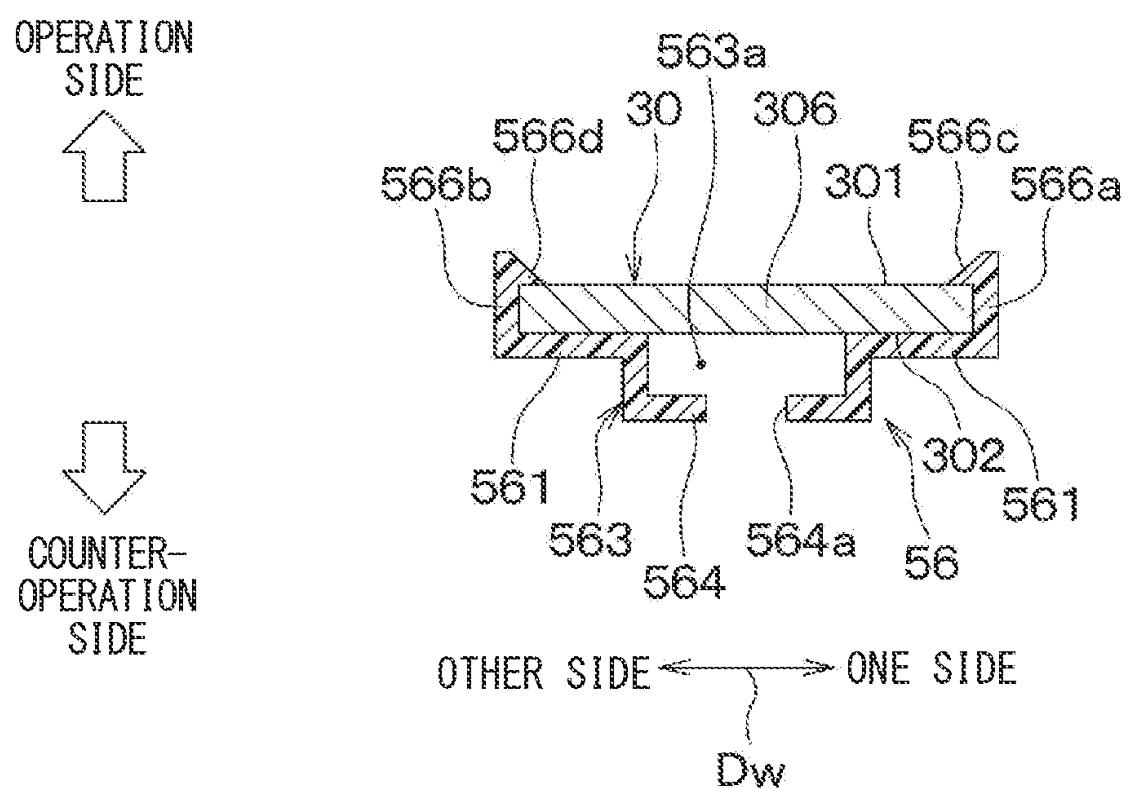
FIG. 32
