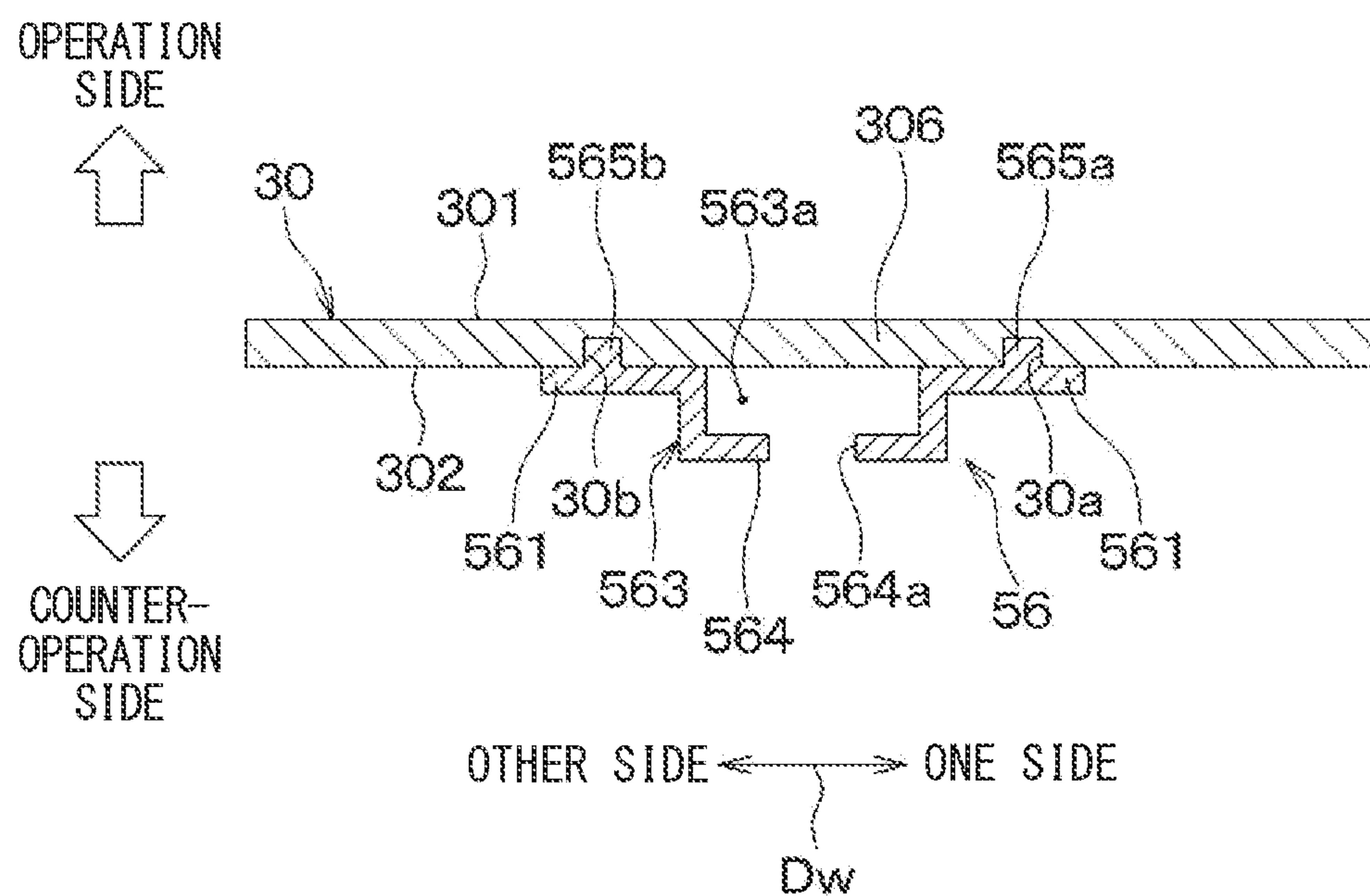
FIG. 20
