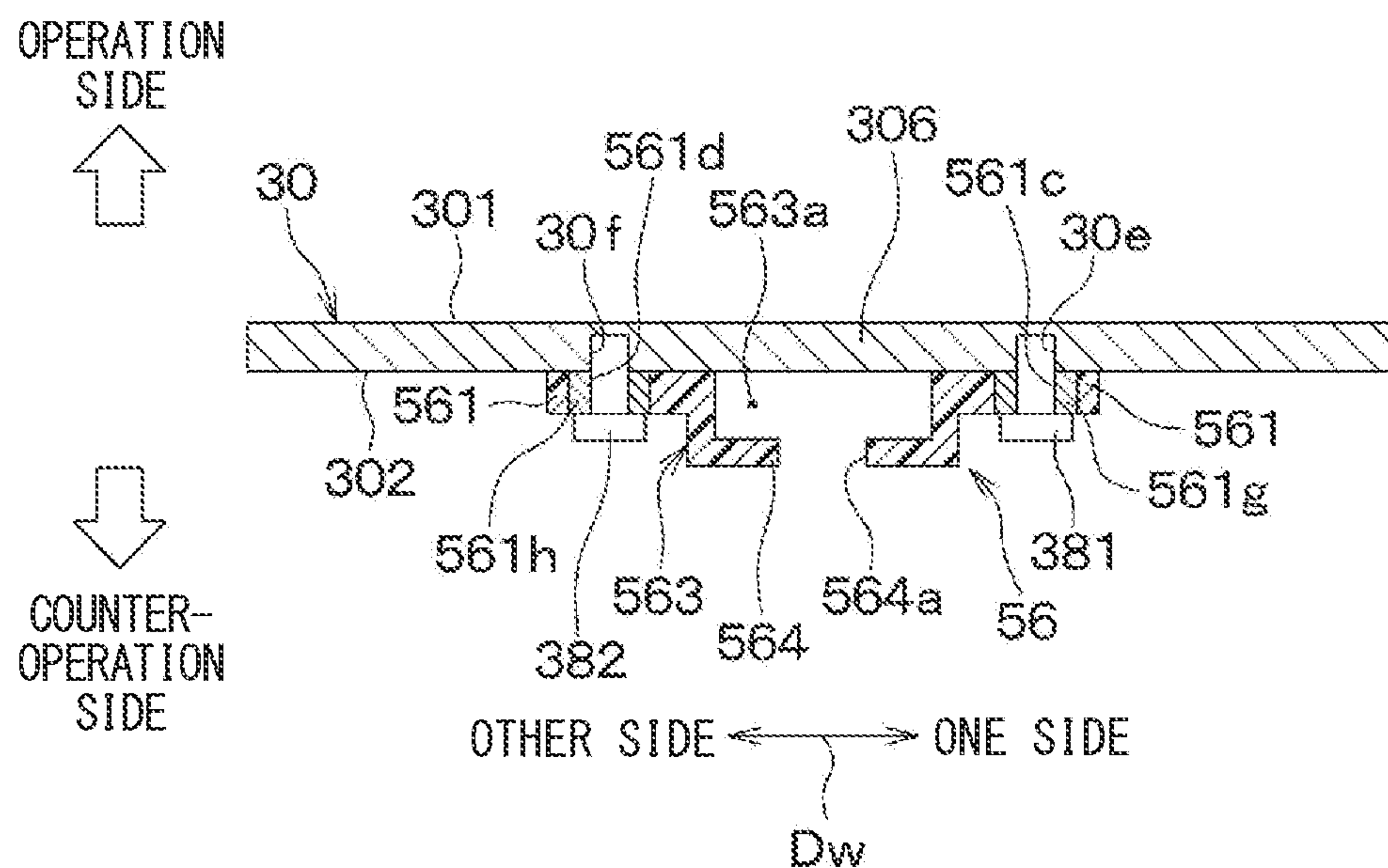
FIG. 30
