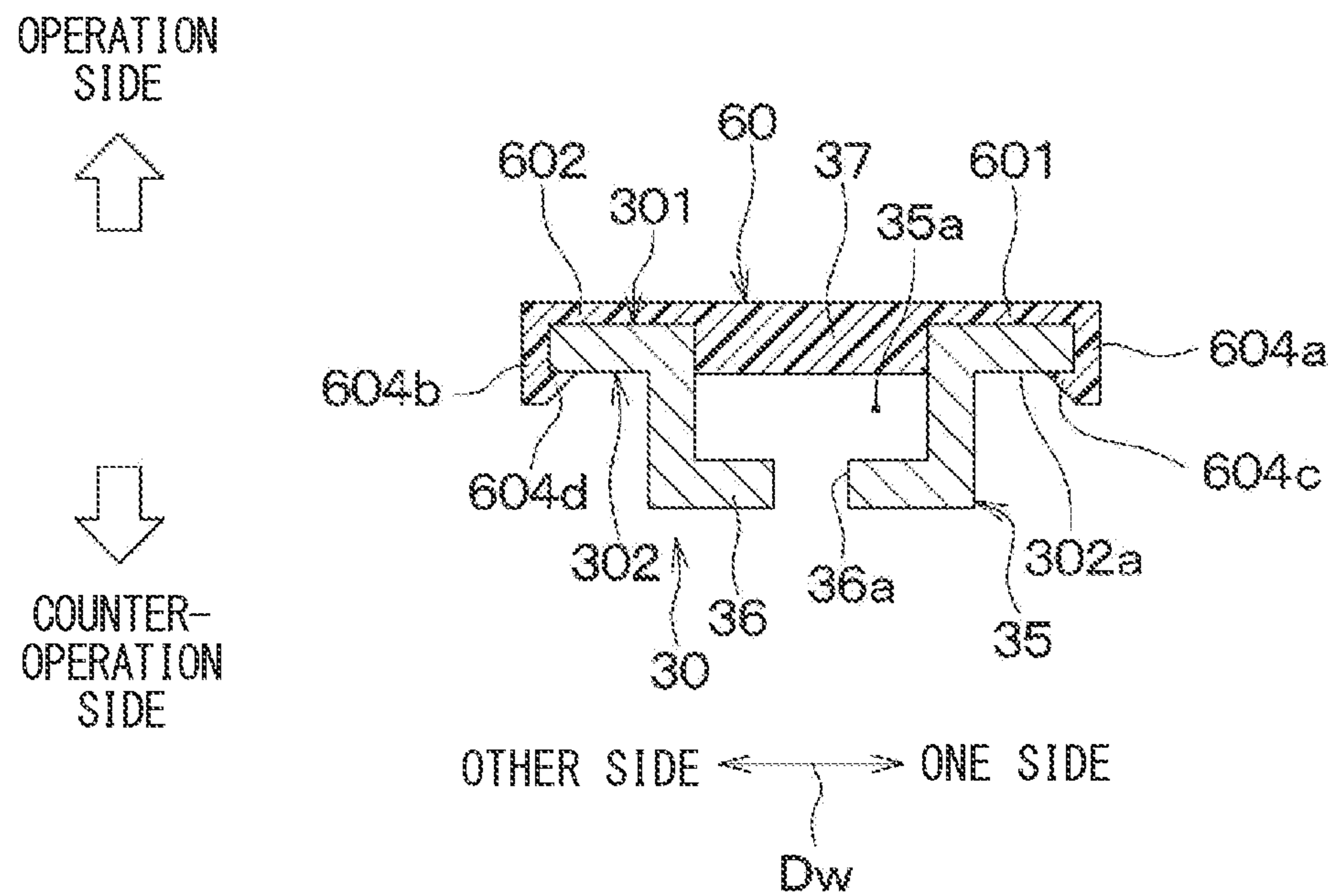
FIG. 33
