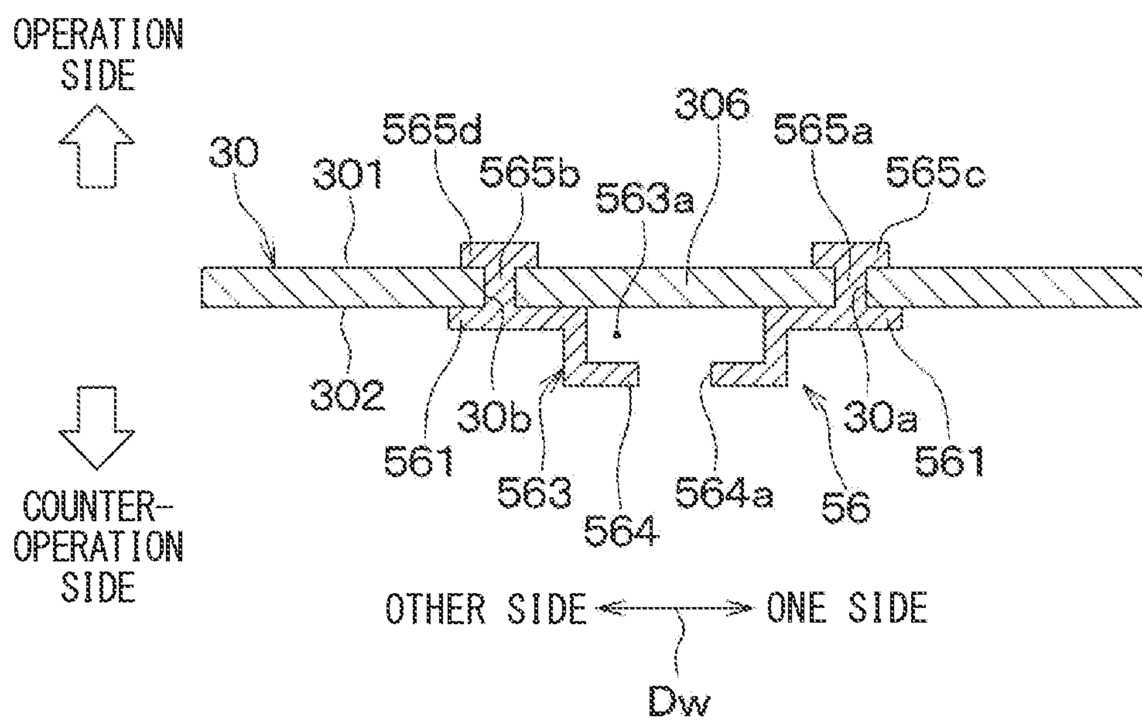
FIG. 22
