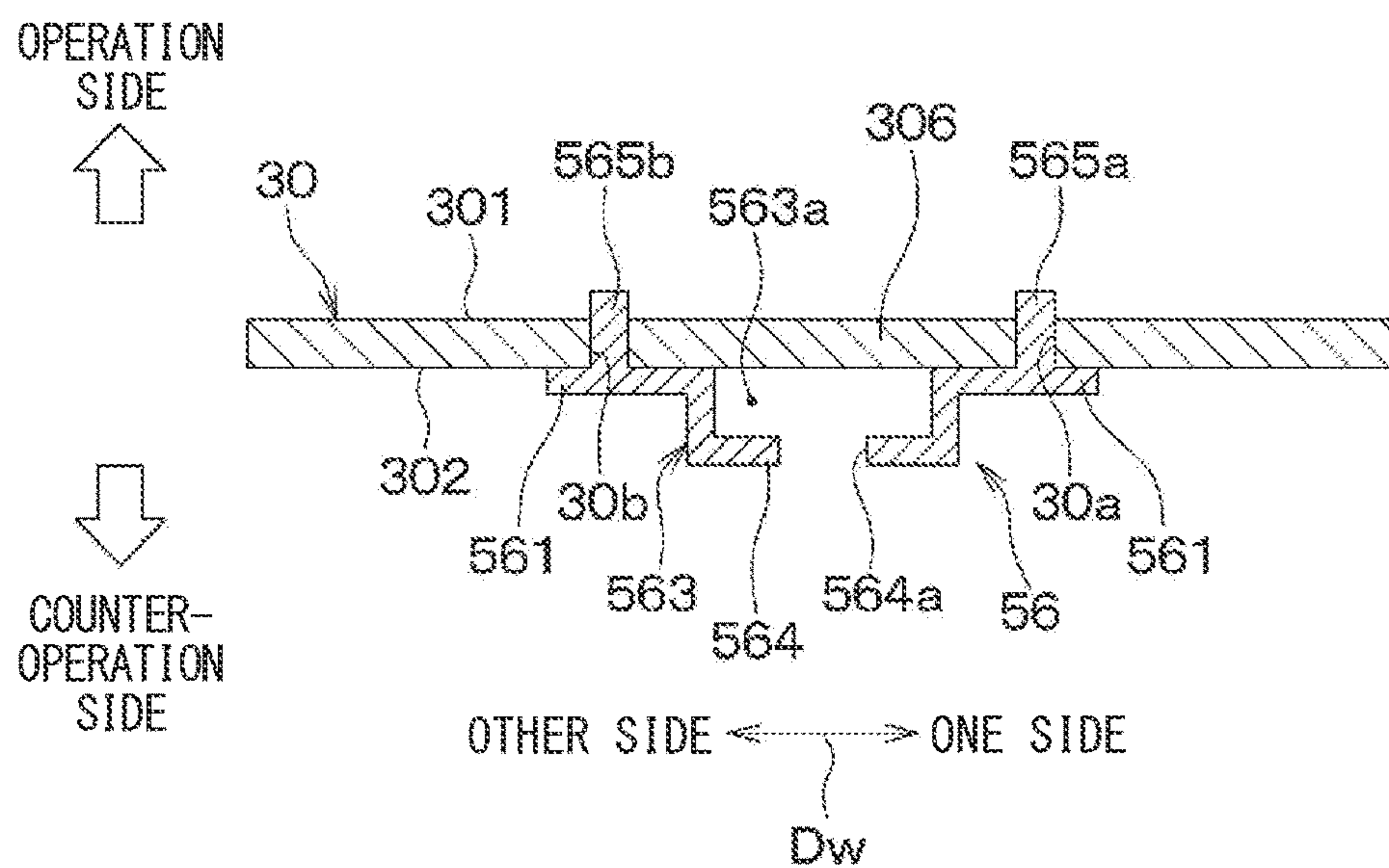
FIG. 18
