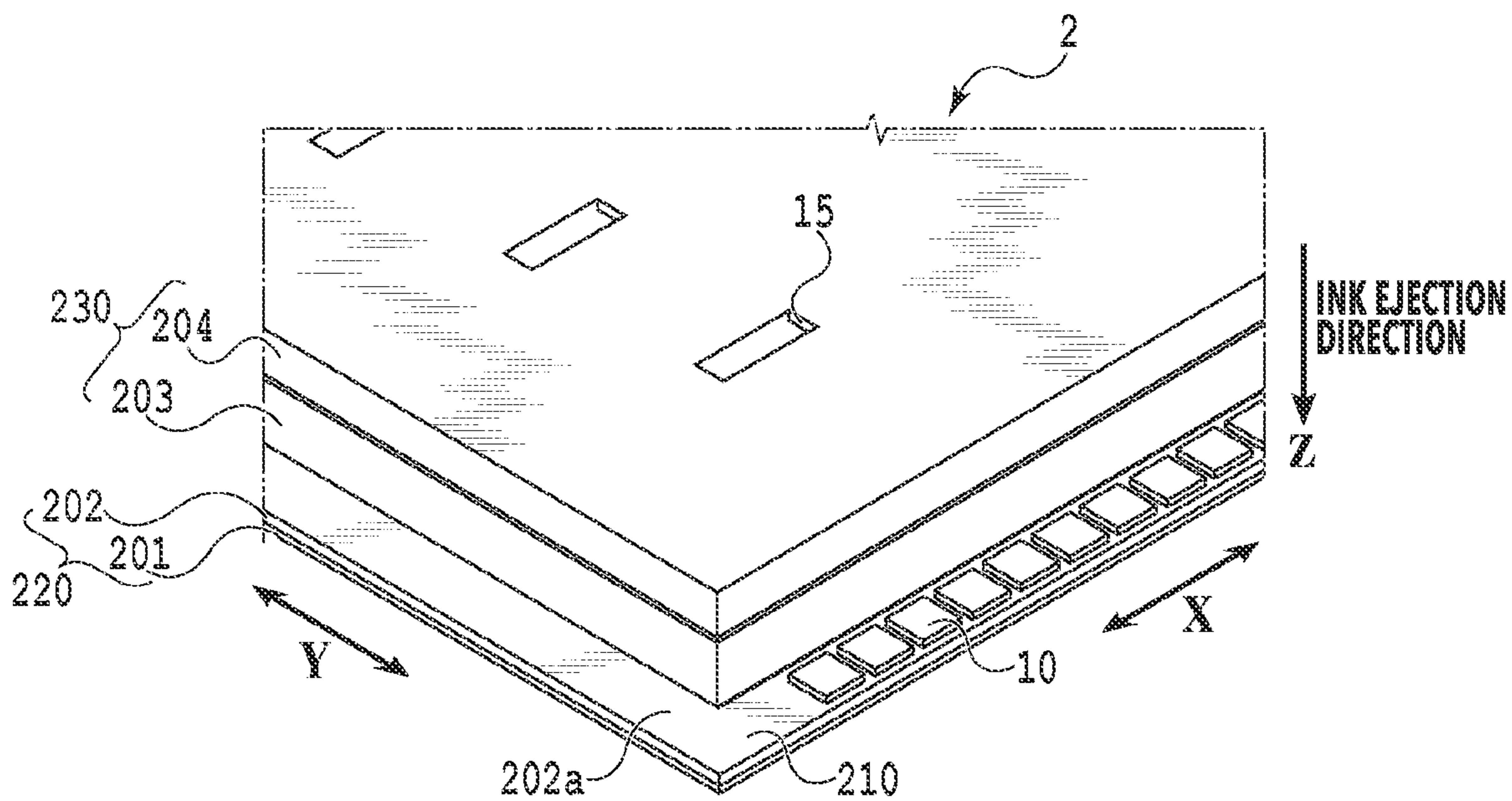
FIG. 5B
