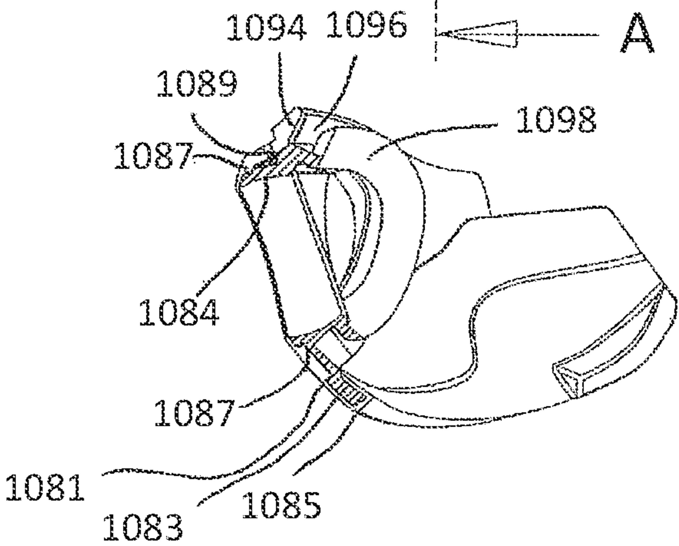
SECTION A-A
