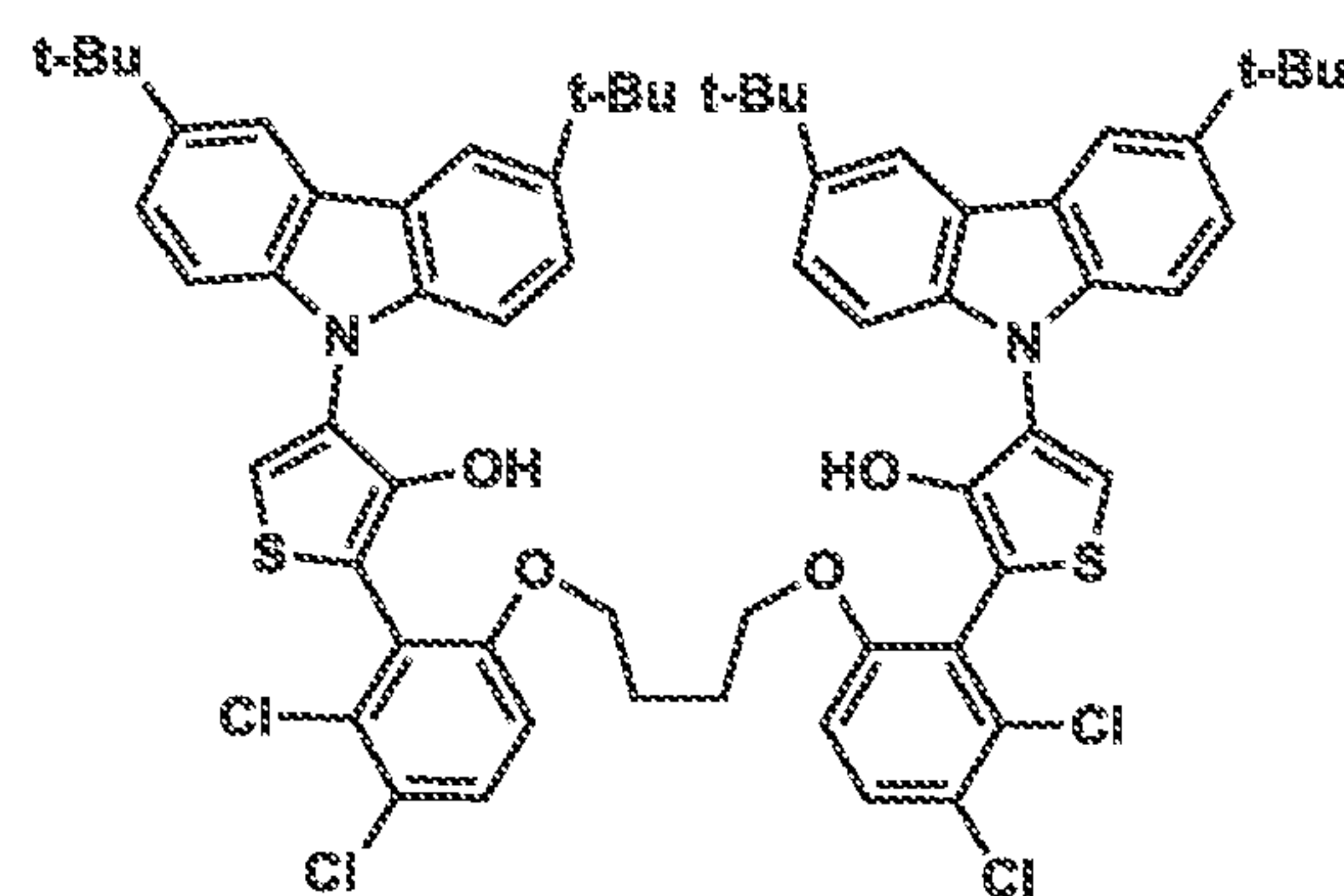
Ligand 23
