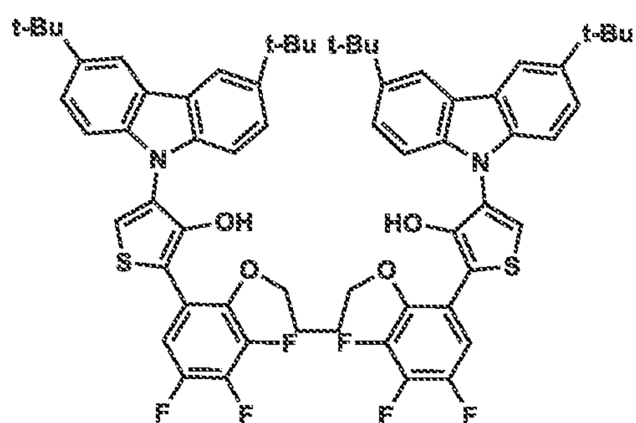
Ligand 20
