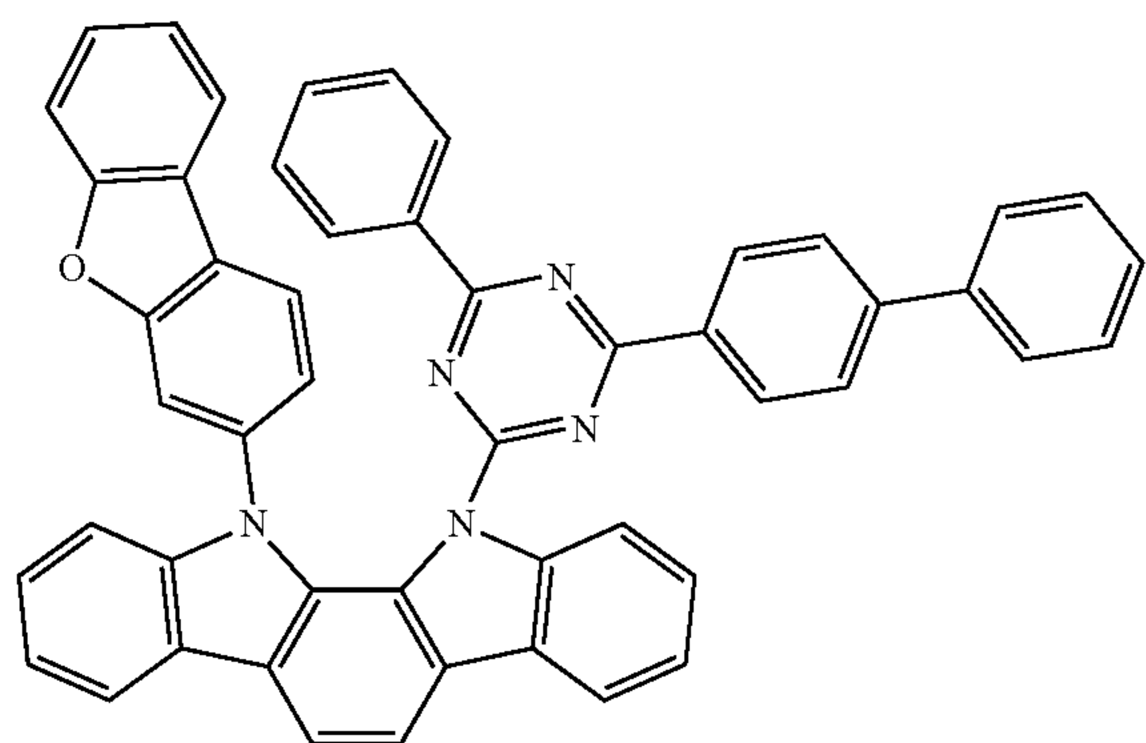
Compound D15
