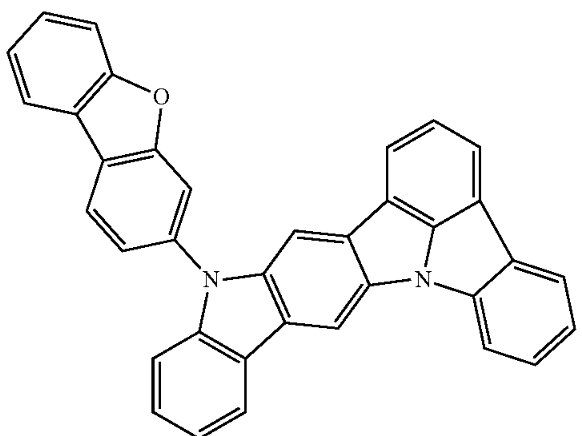
Compound E14
