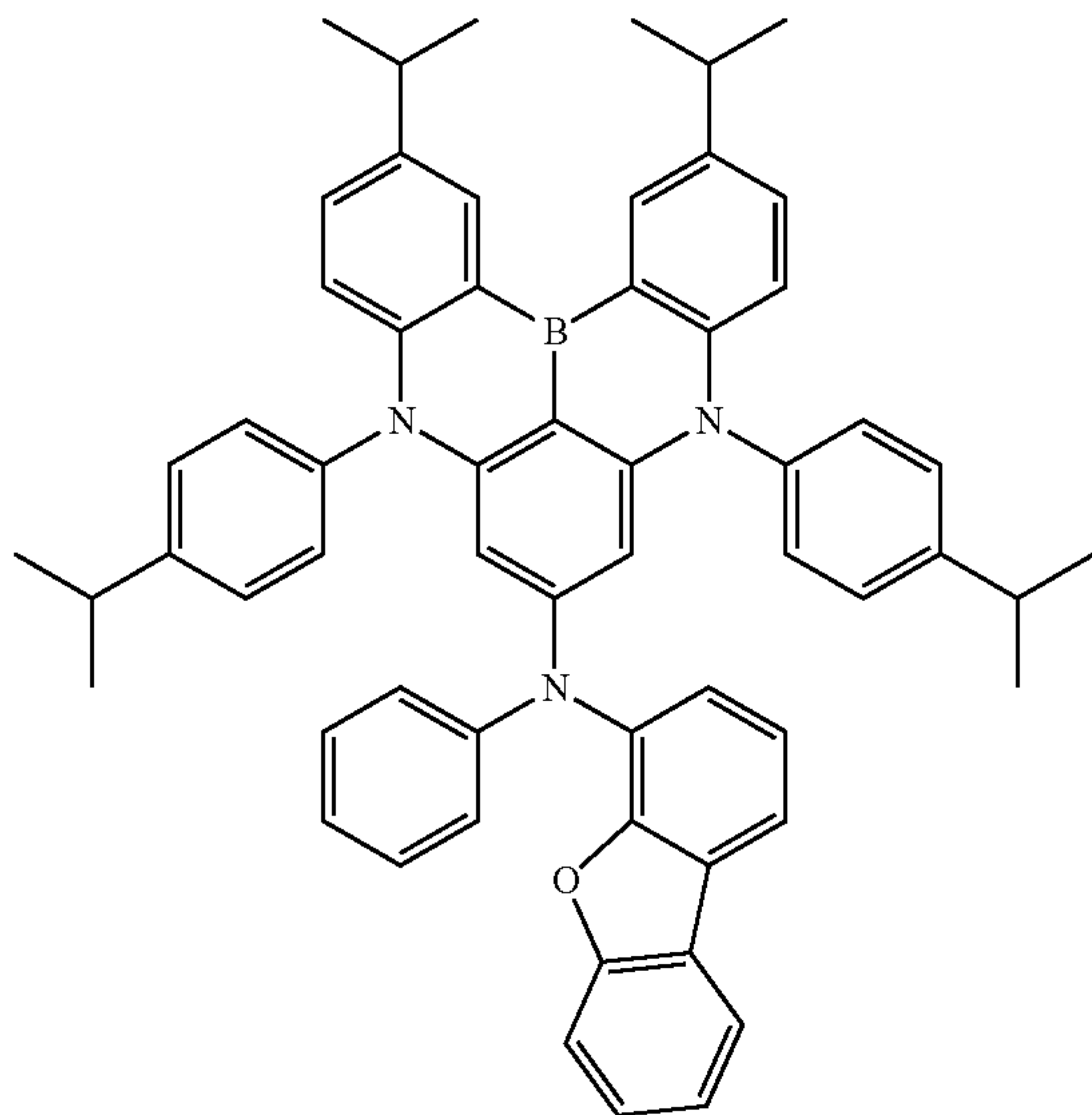
Dopant 117
