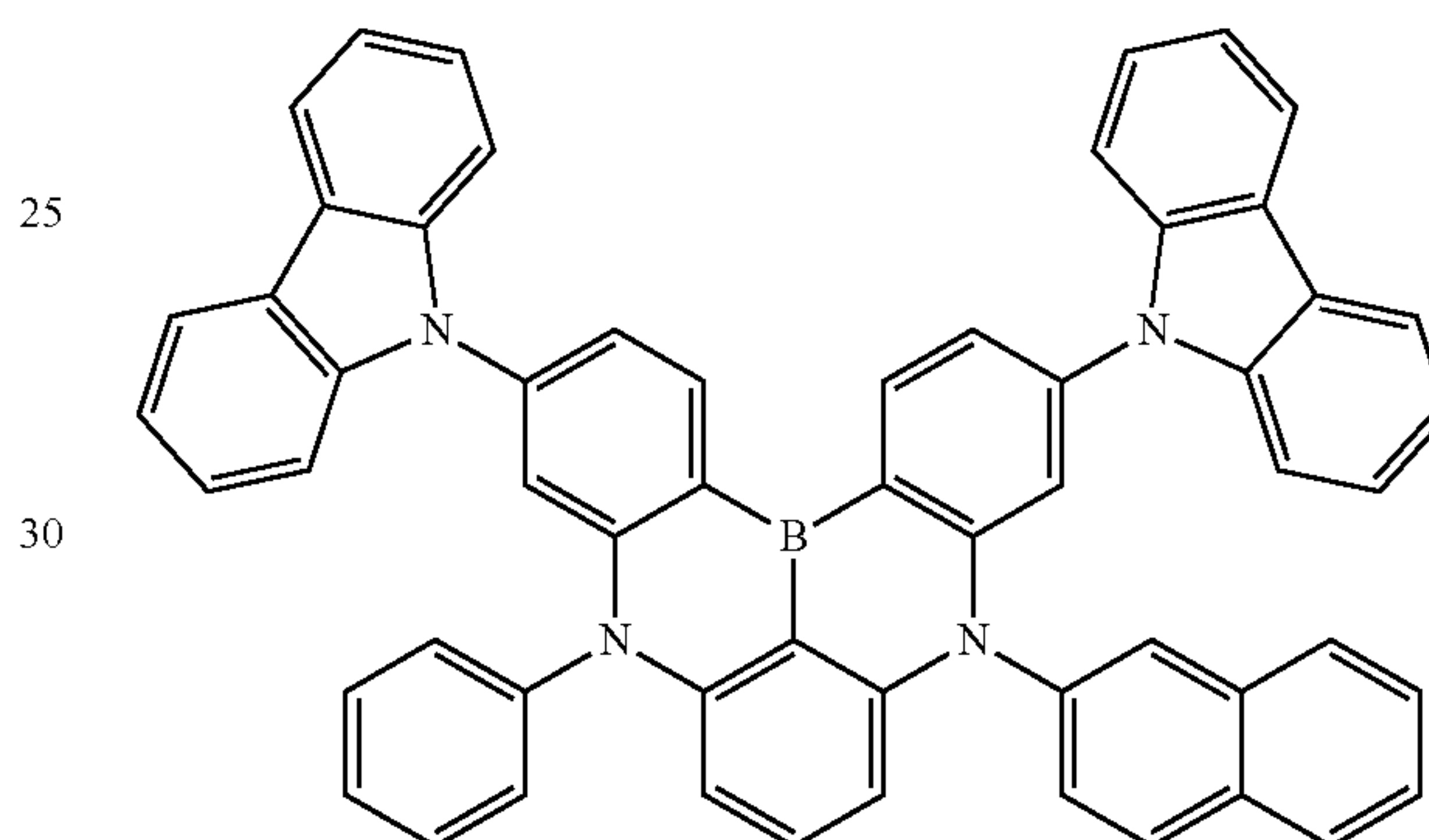
Dopant 106
