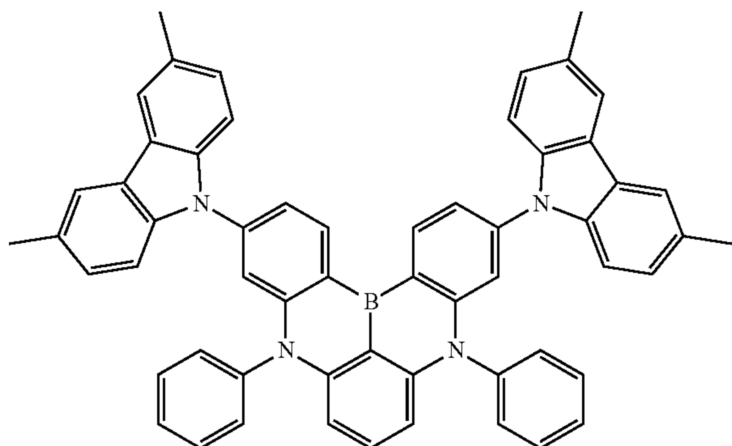
Dopant 73
