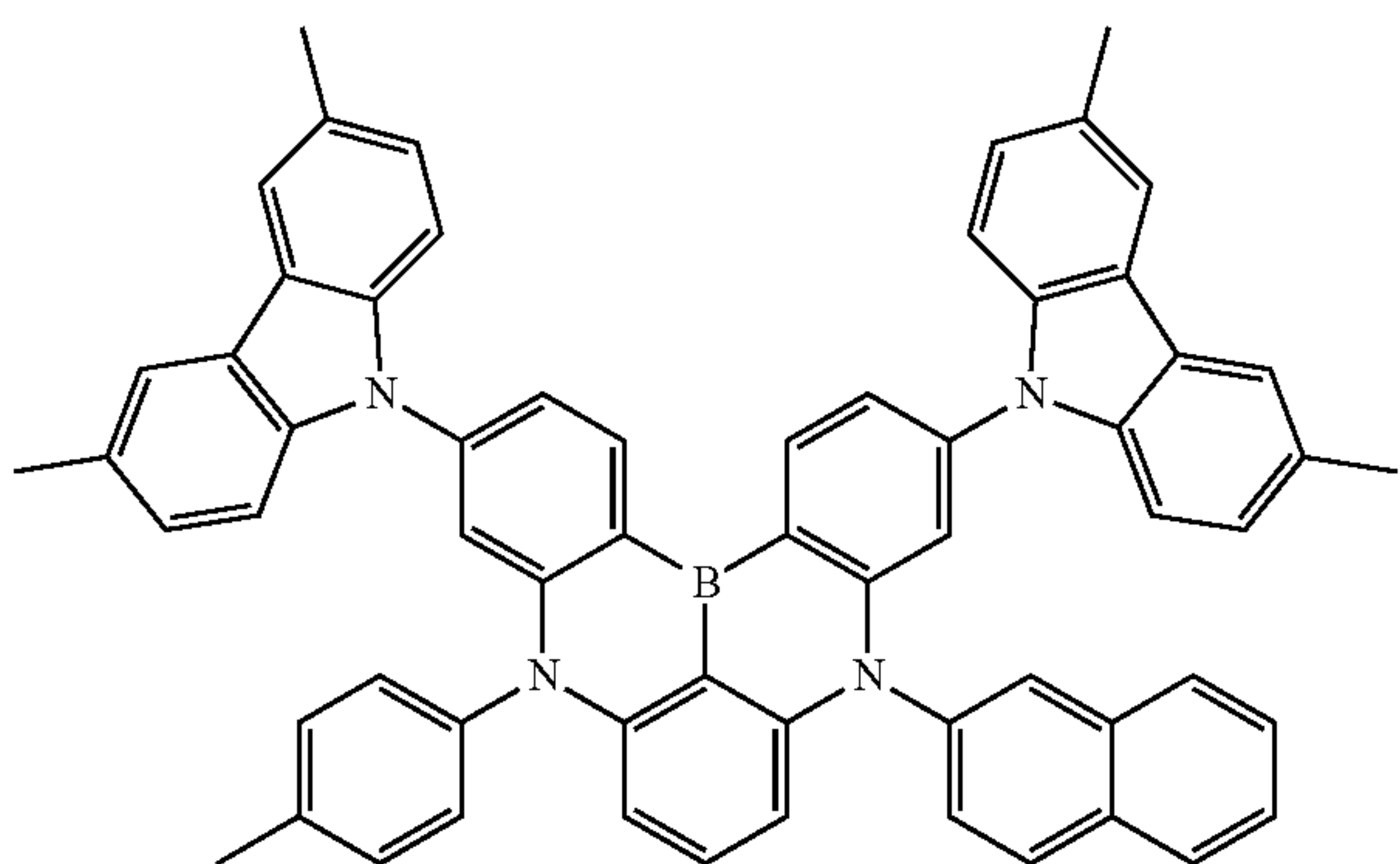
Dopant 108
