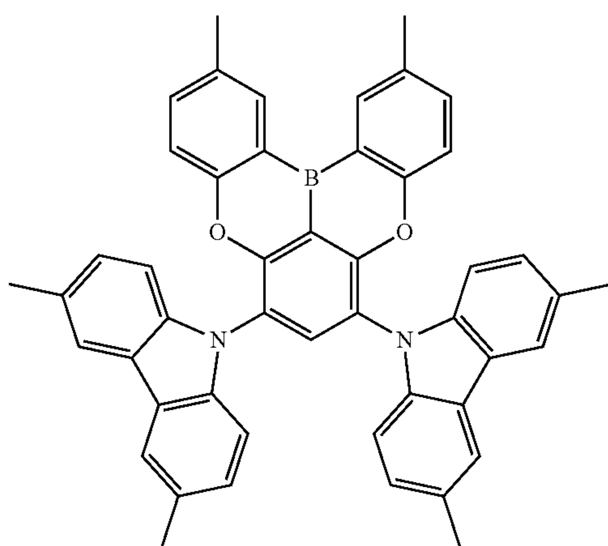
Dopant 227
