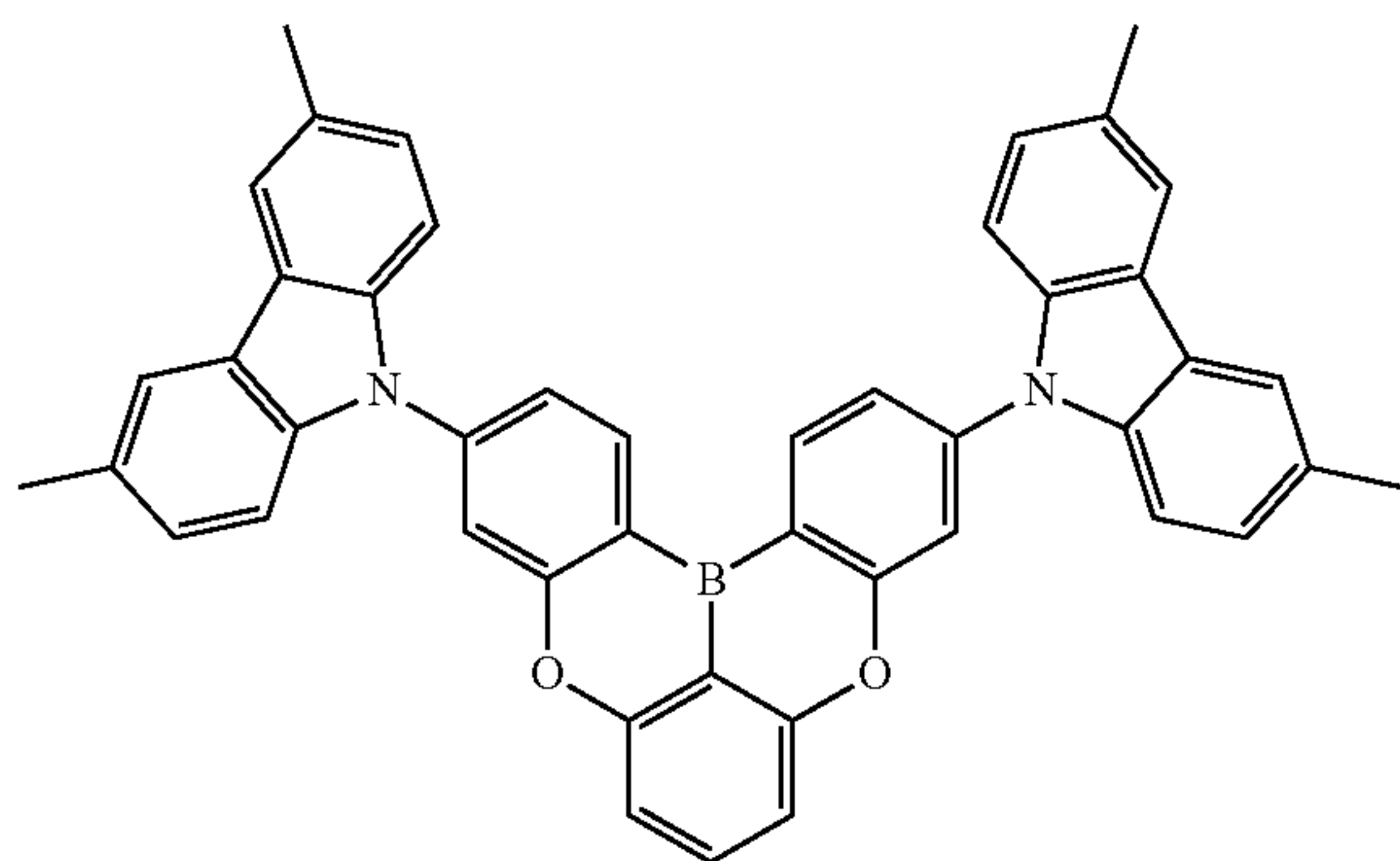
Dopant 194
