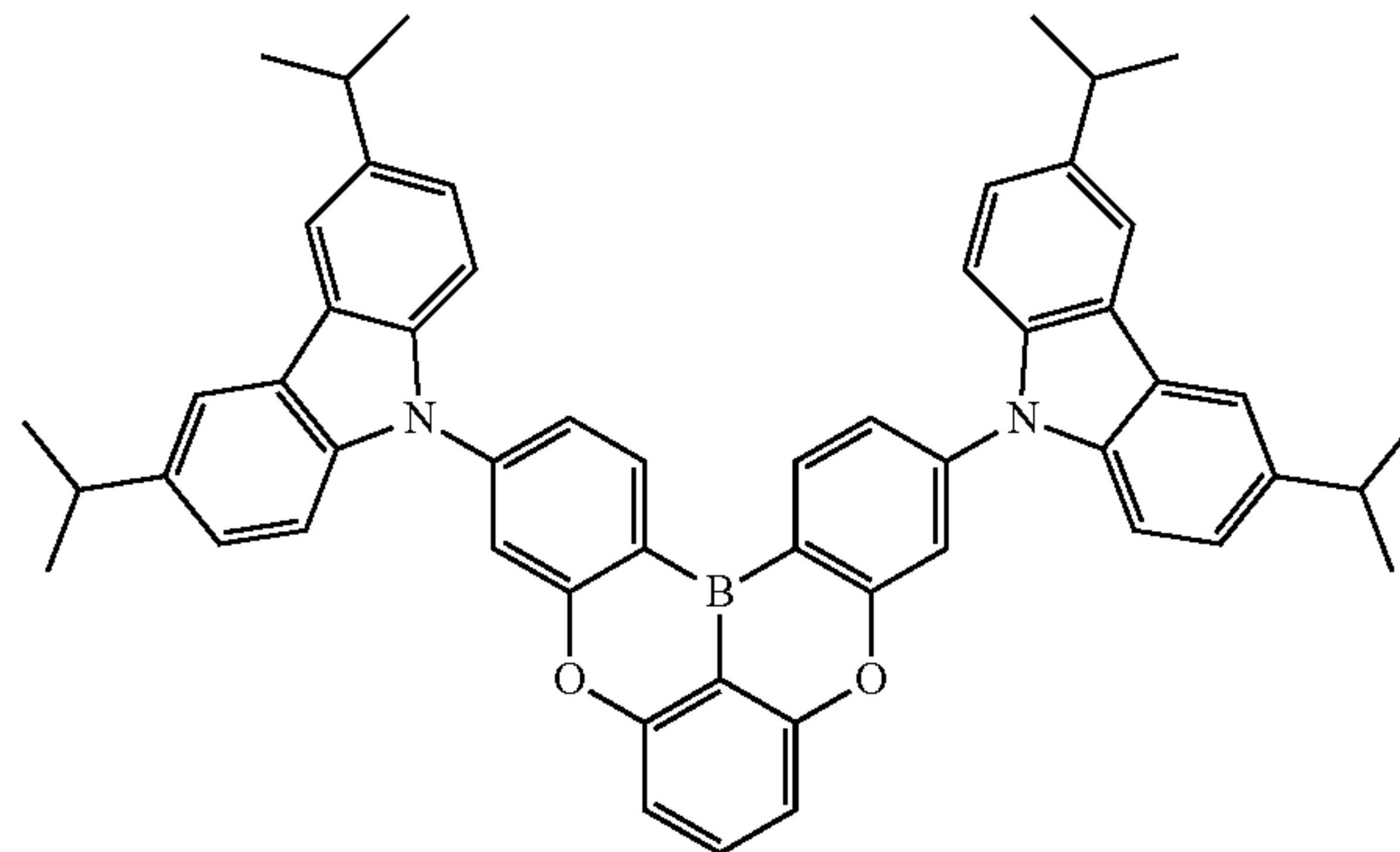
Dopant 200
