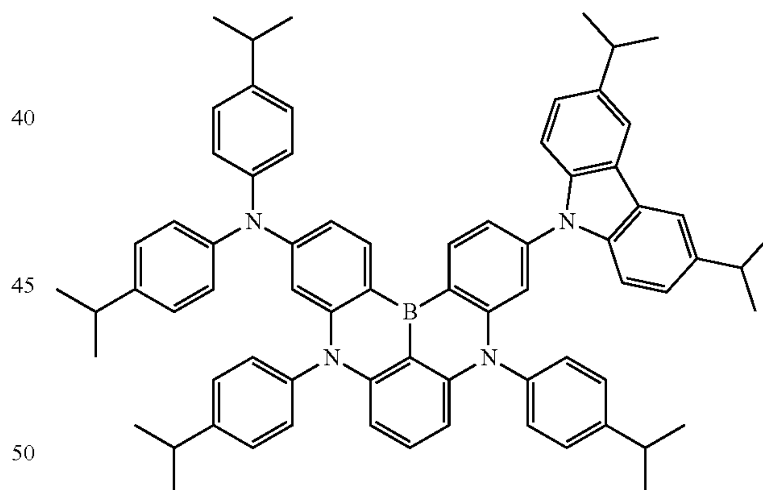
Dopant 80
