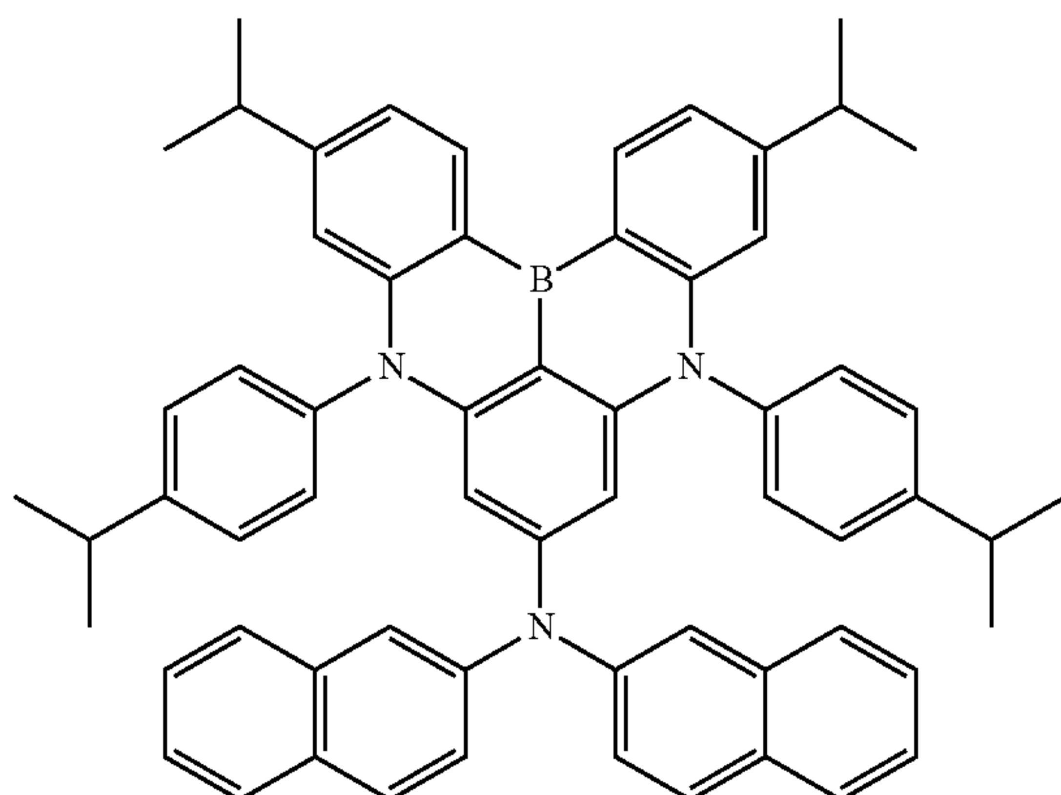
Dopant 142
