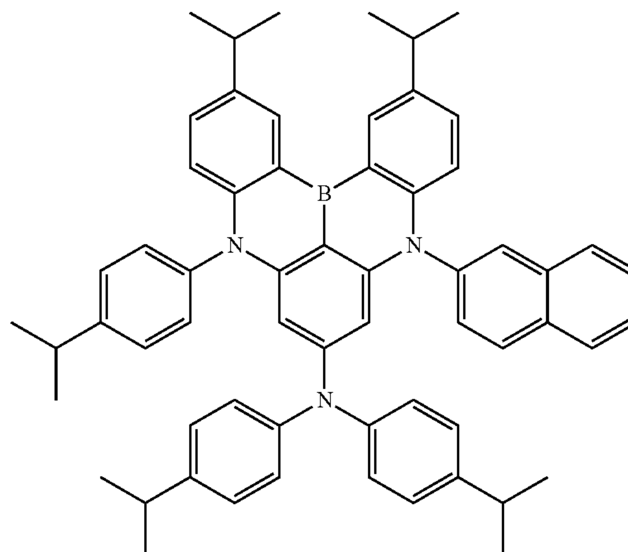
Dopant 84
