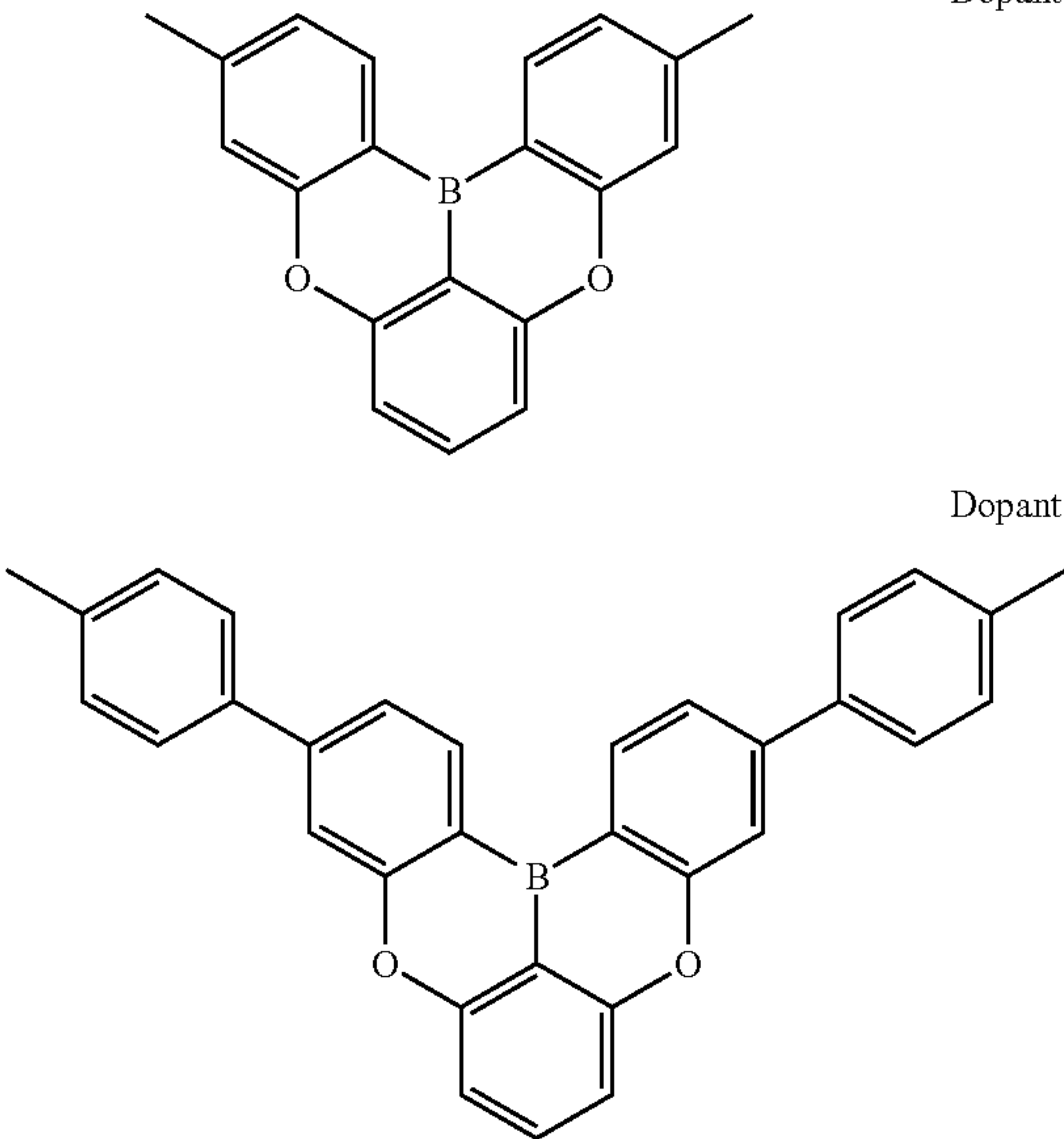
Dopant 171
