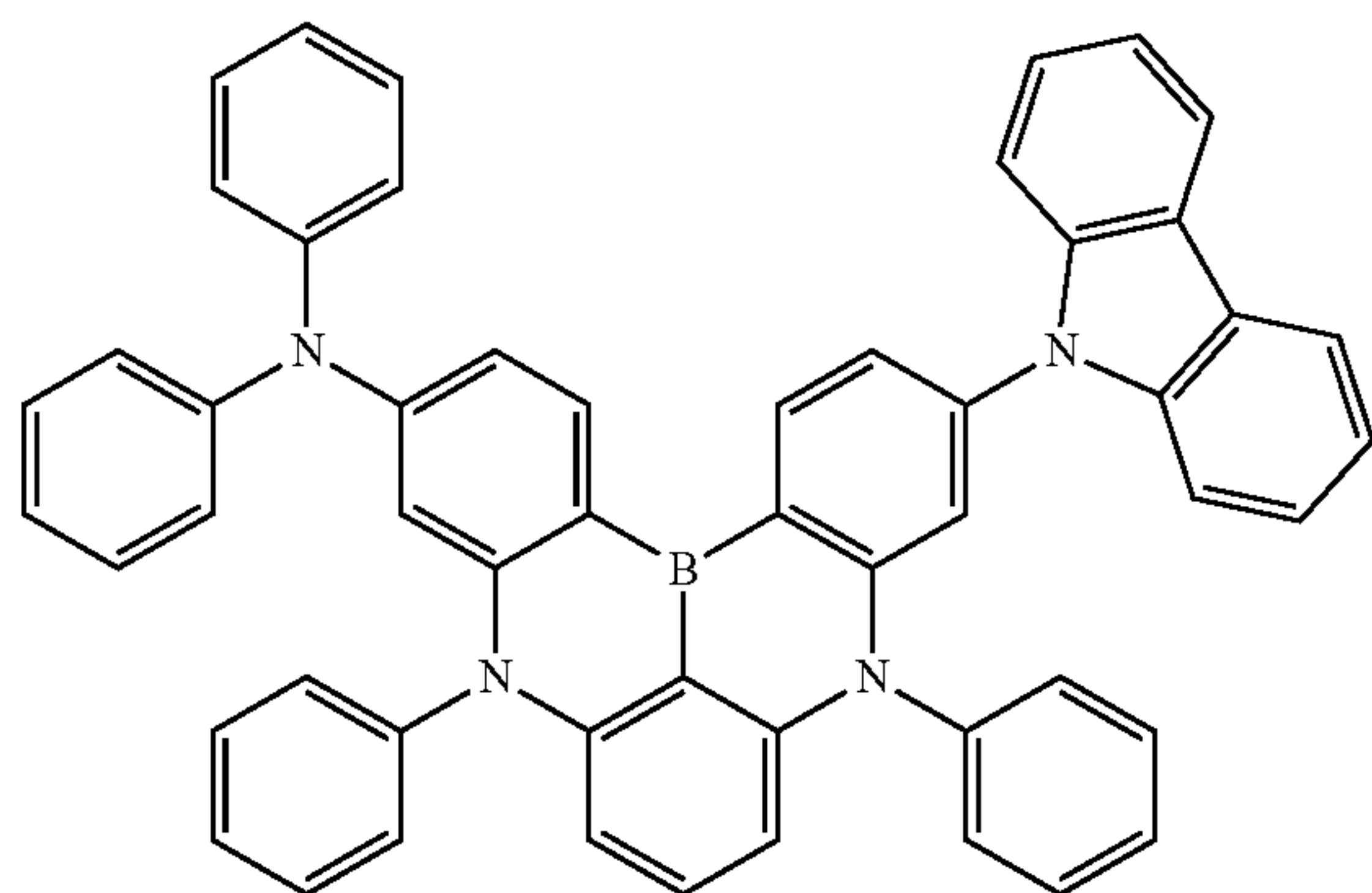
Dopant 76
