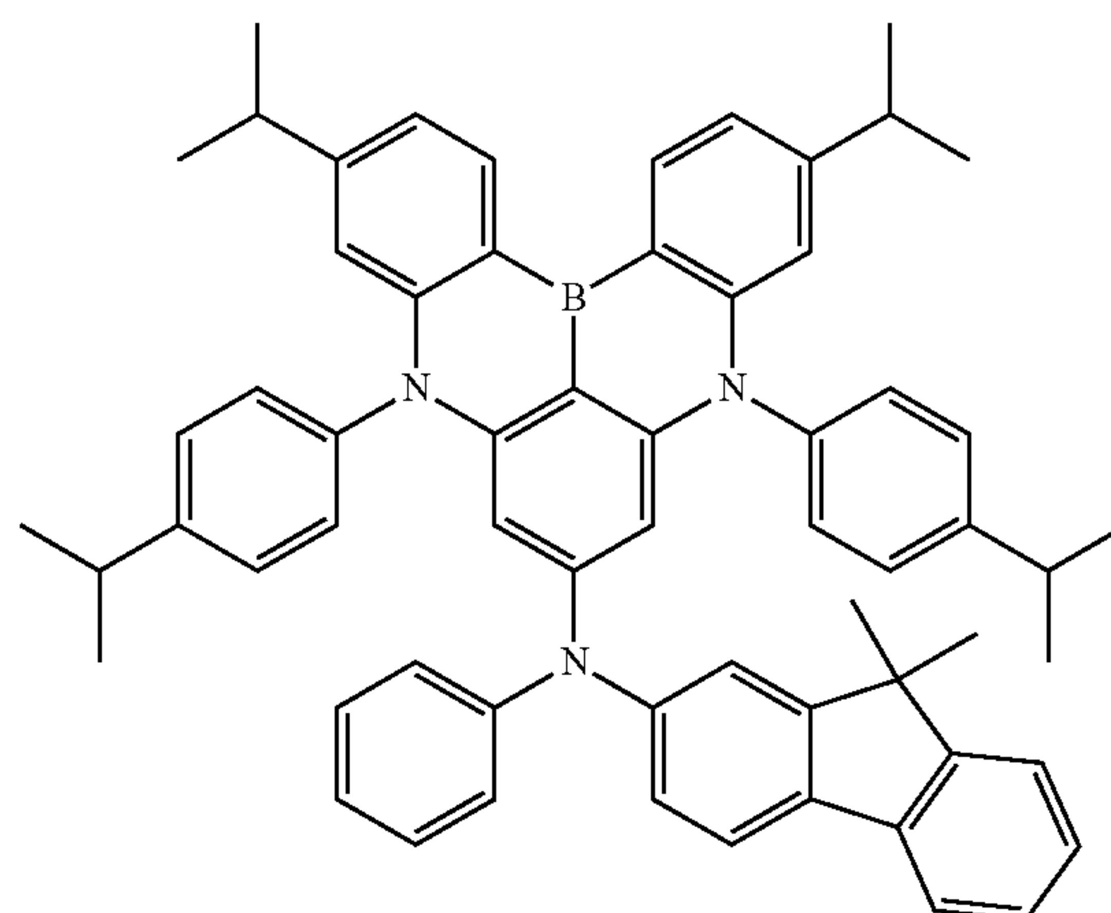
Dopant 121
