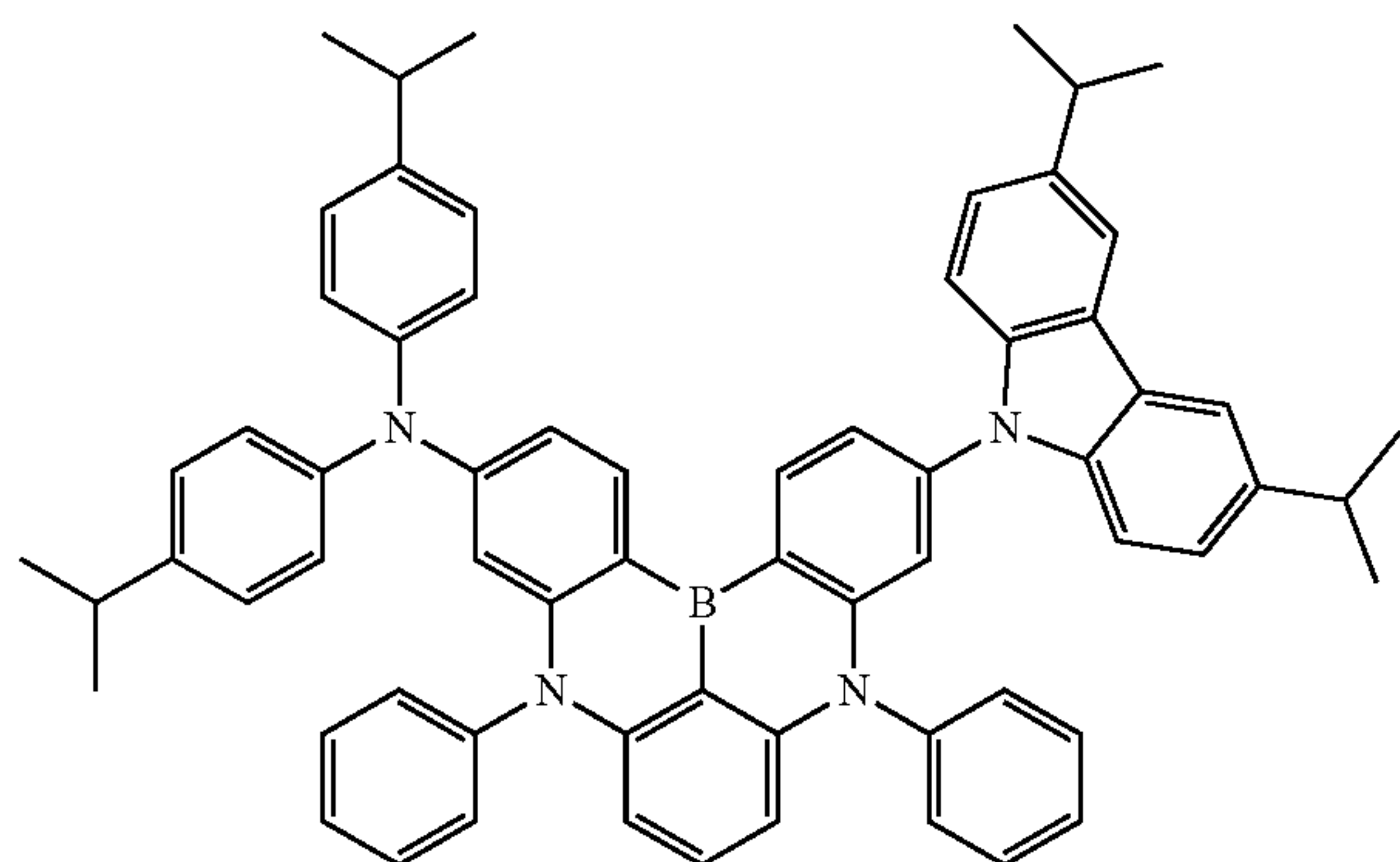
Dopant 81
