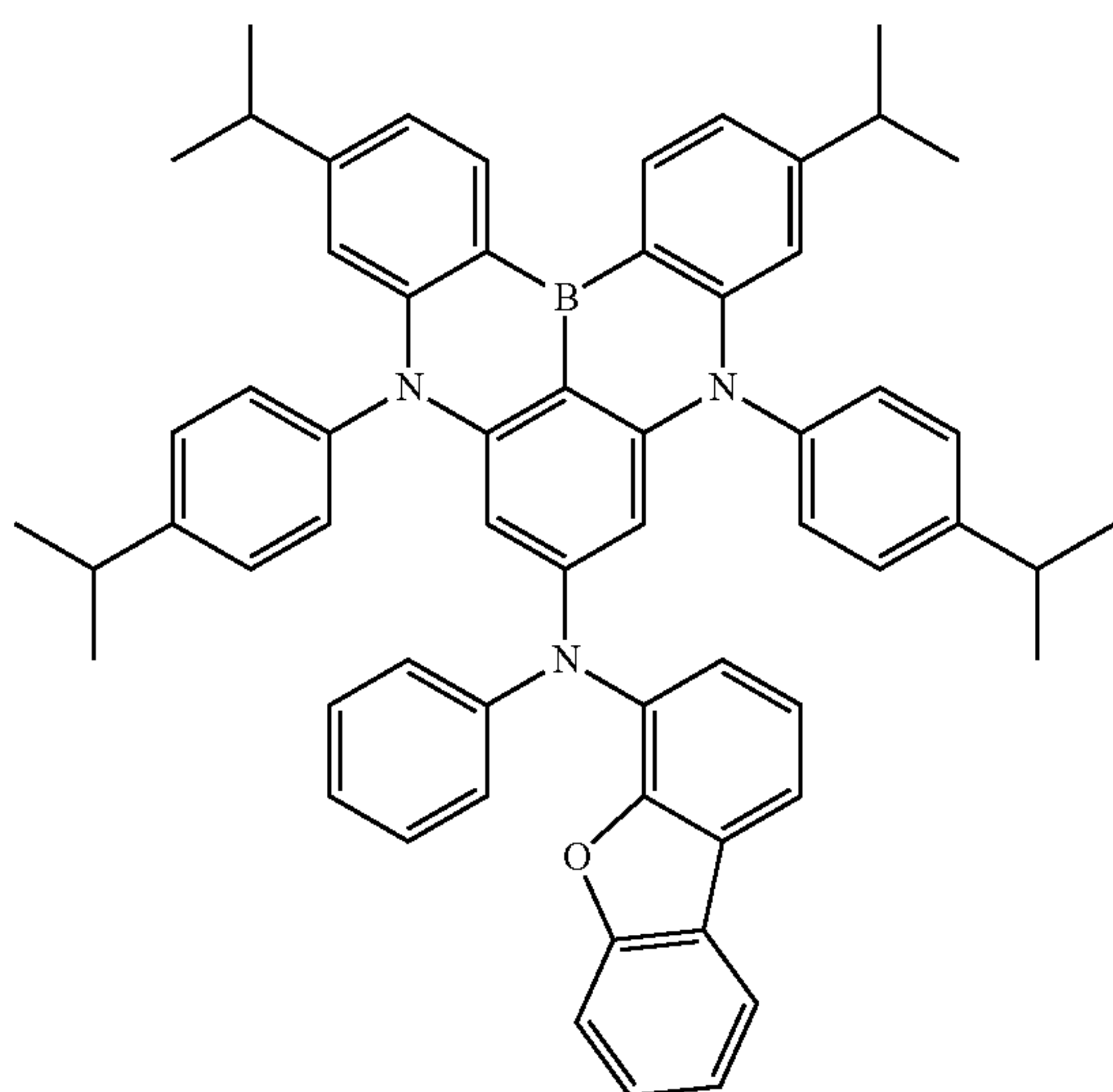
Dopant 118
