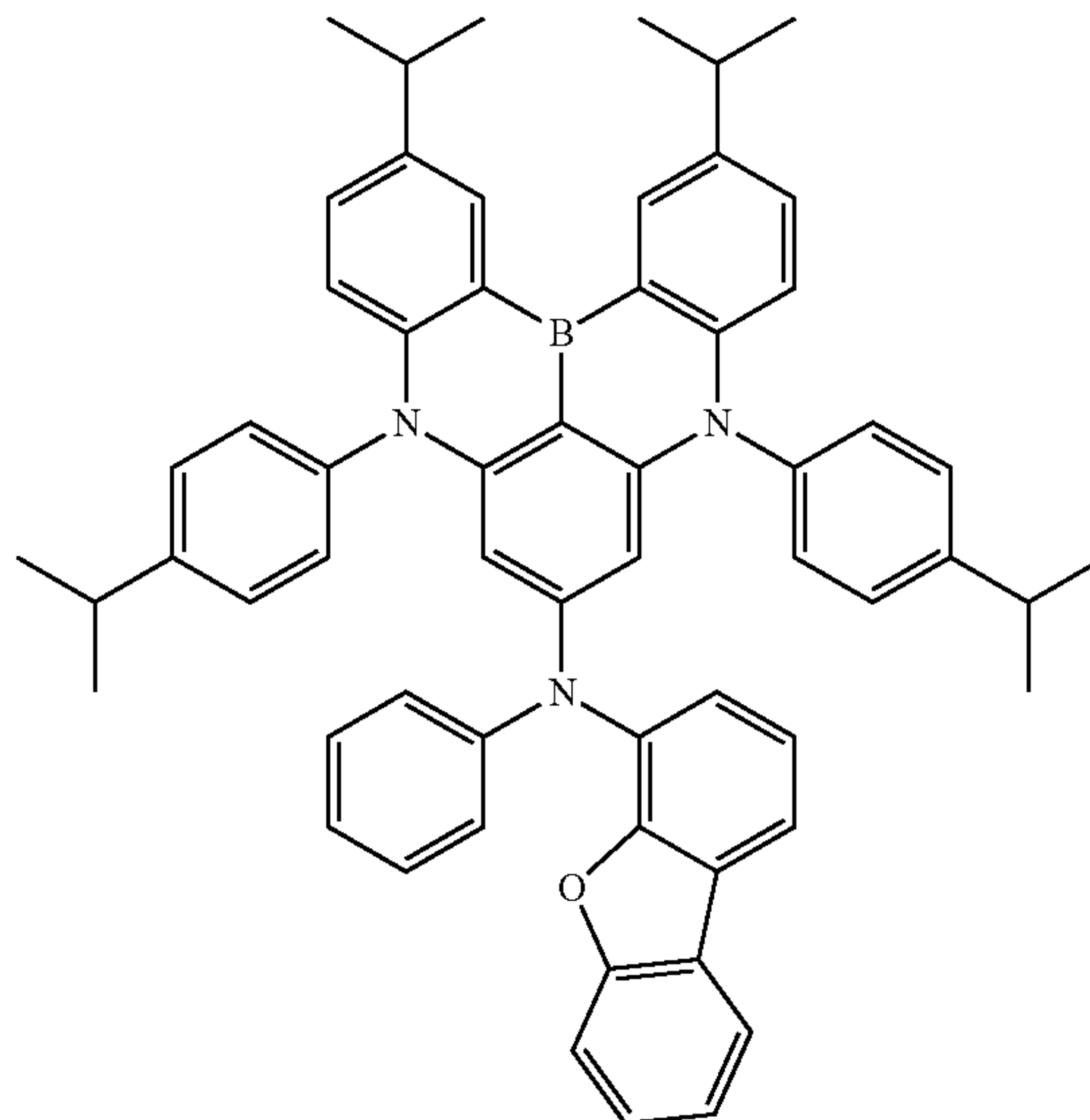
Dopant 117
