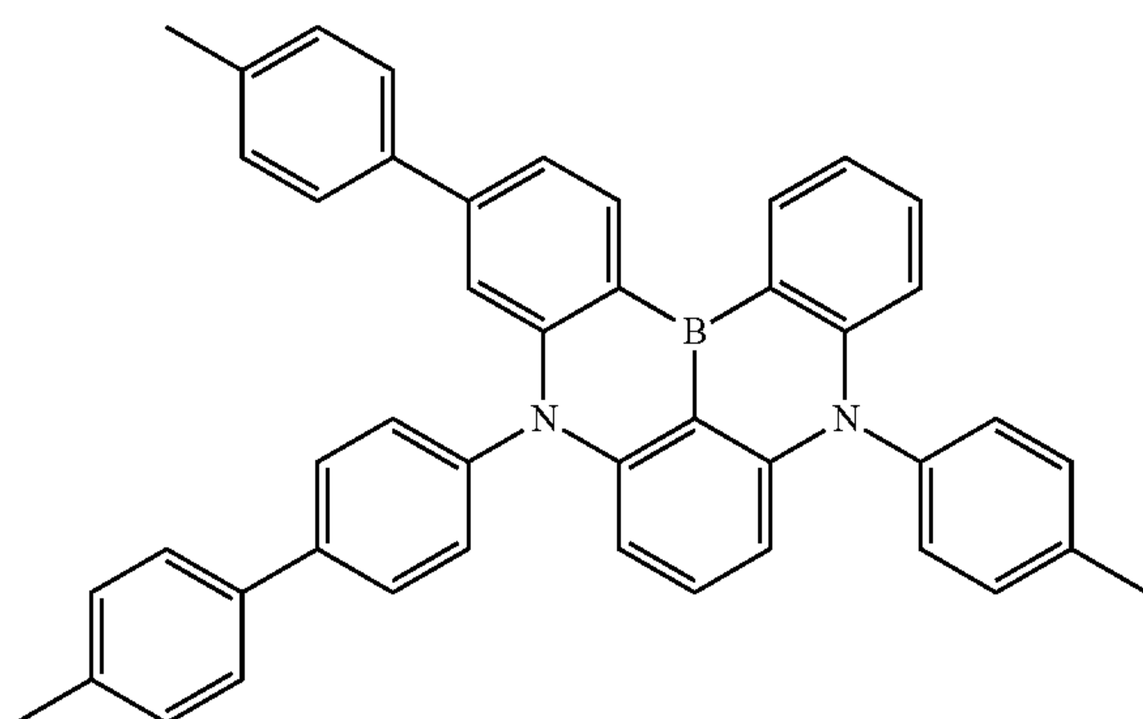
Dopant 27
