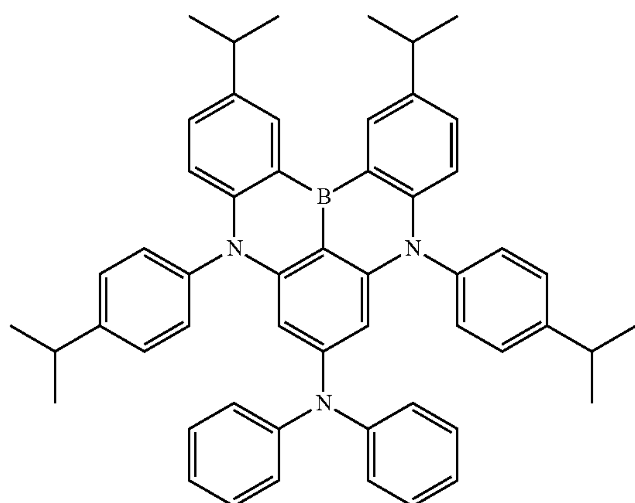
Dopant 51
