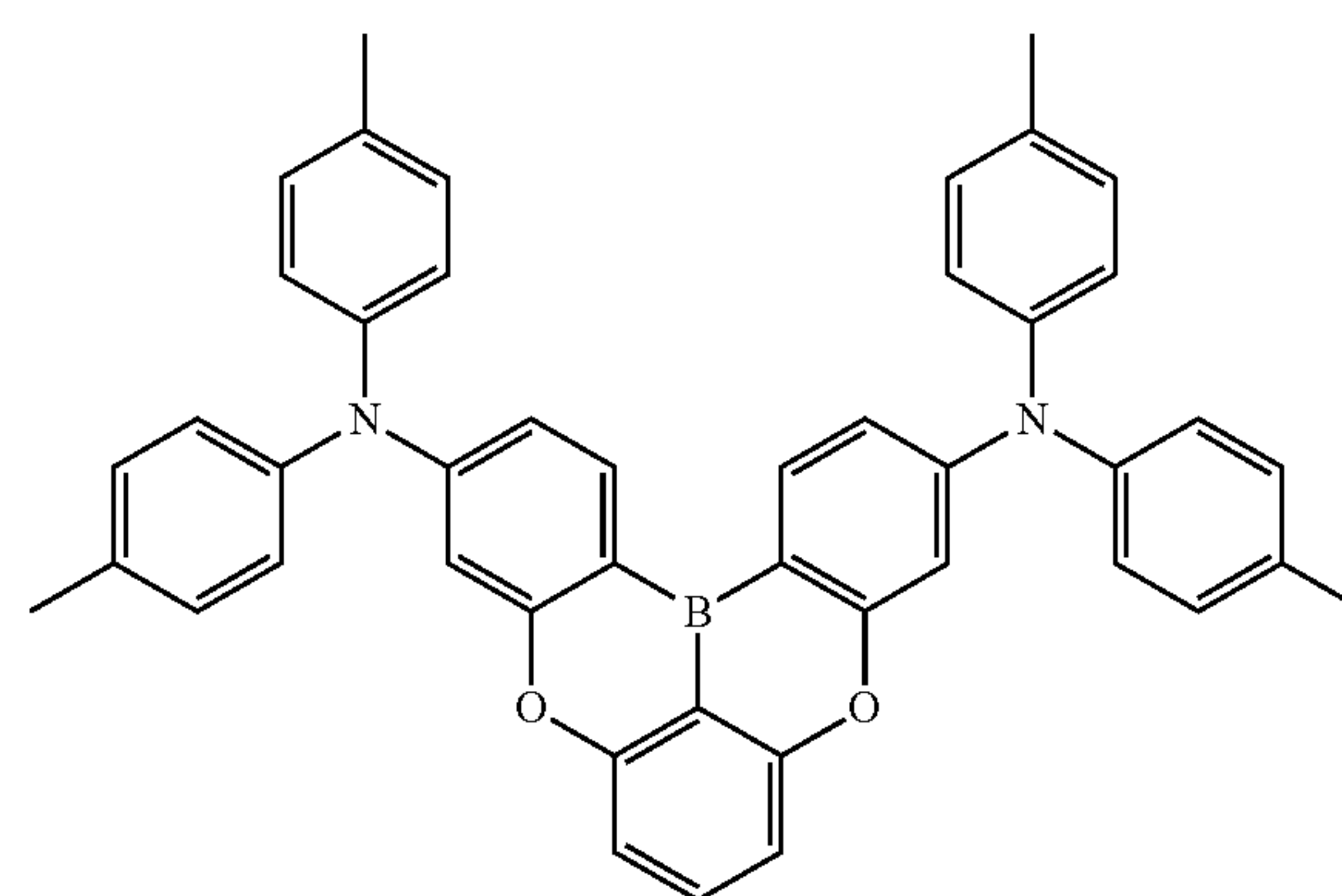
Dopant 191
