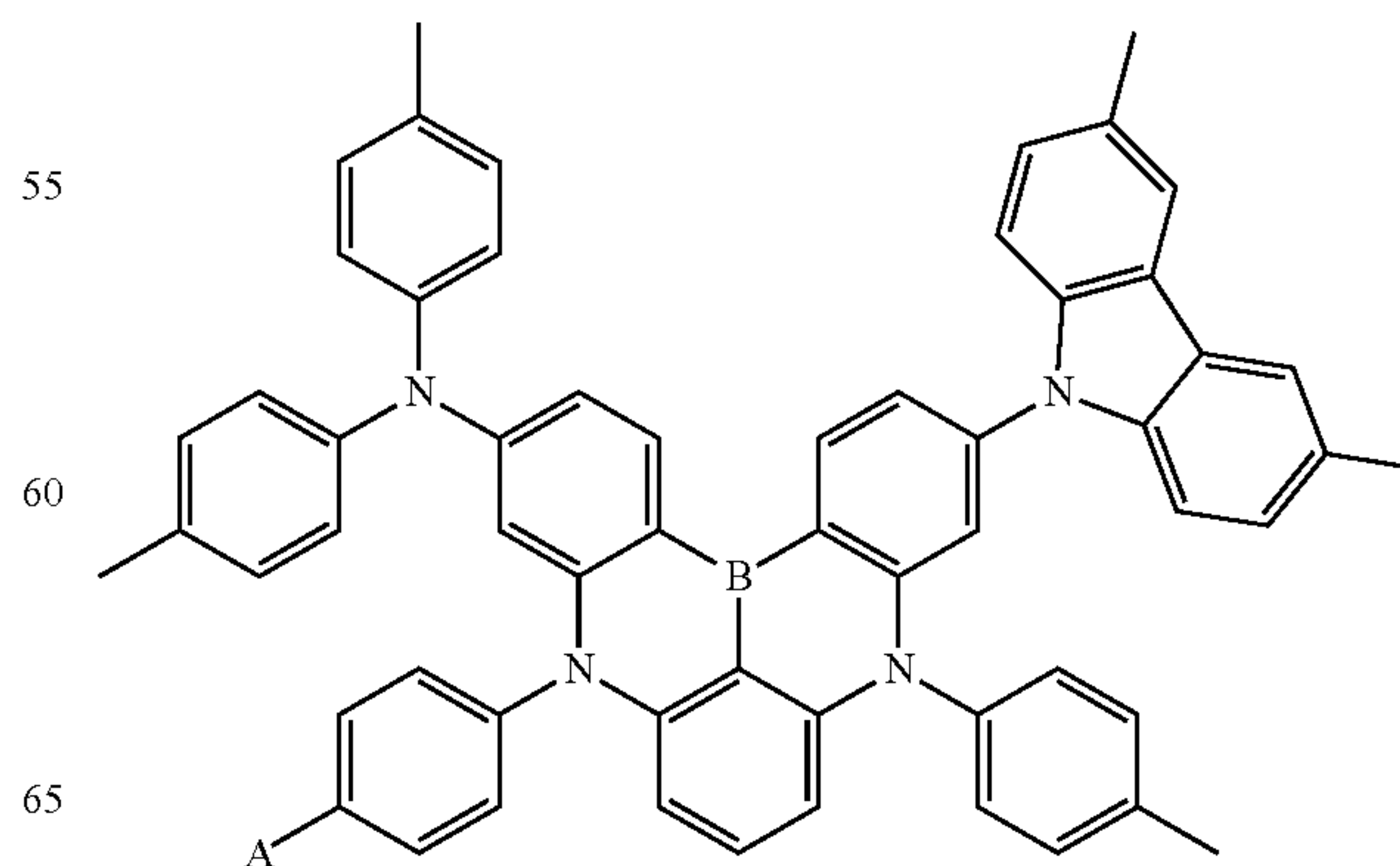
Dopant 77
