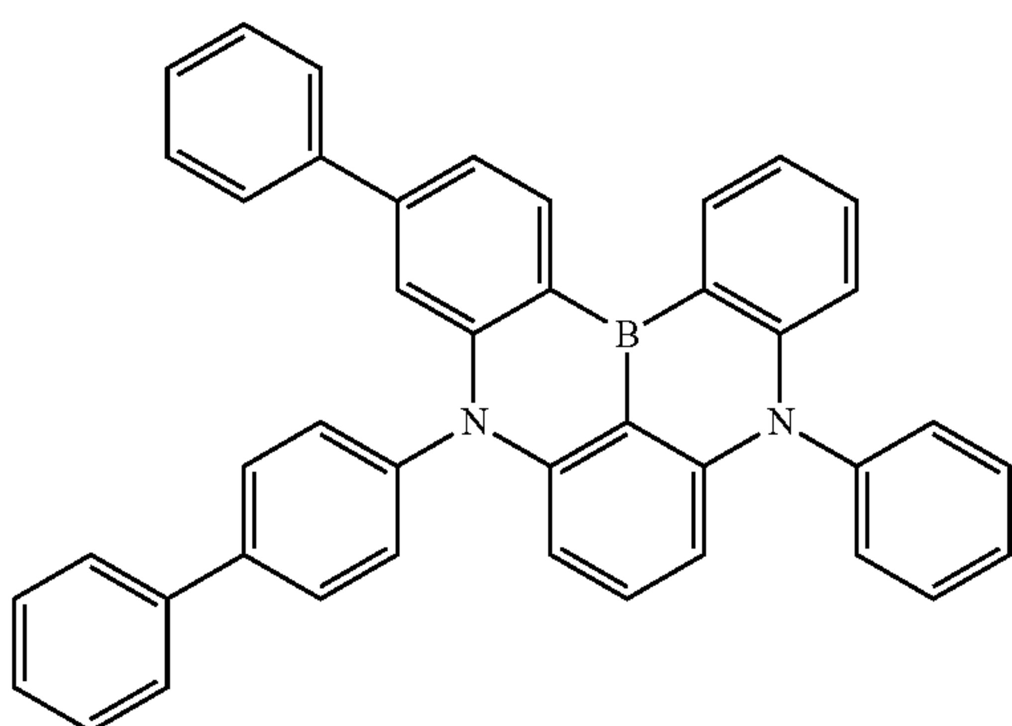
Dopant 26 20
