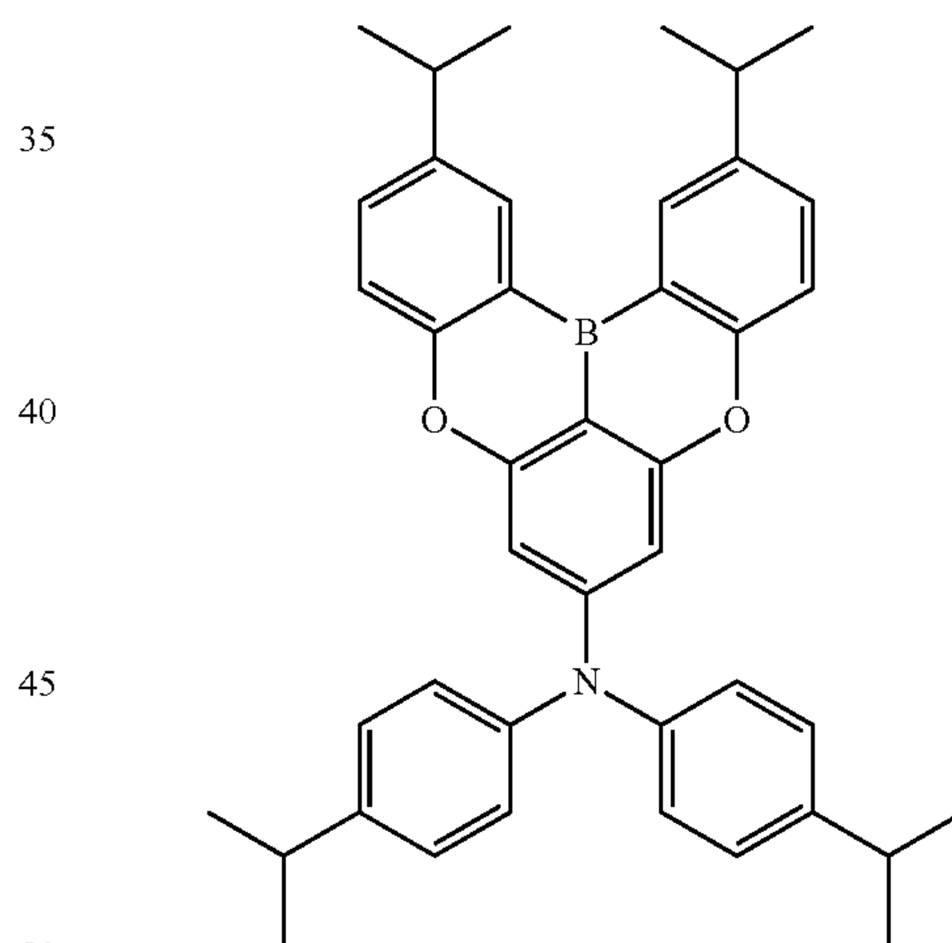
Dopant 191
