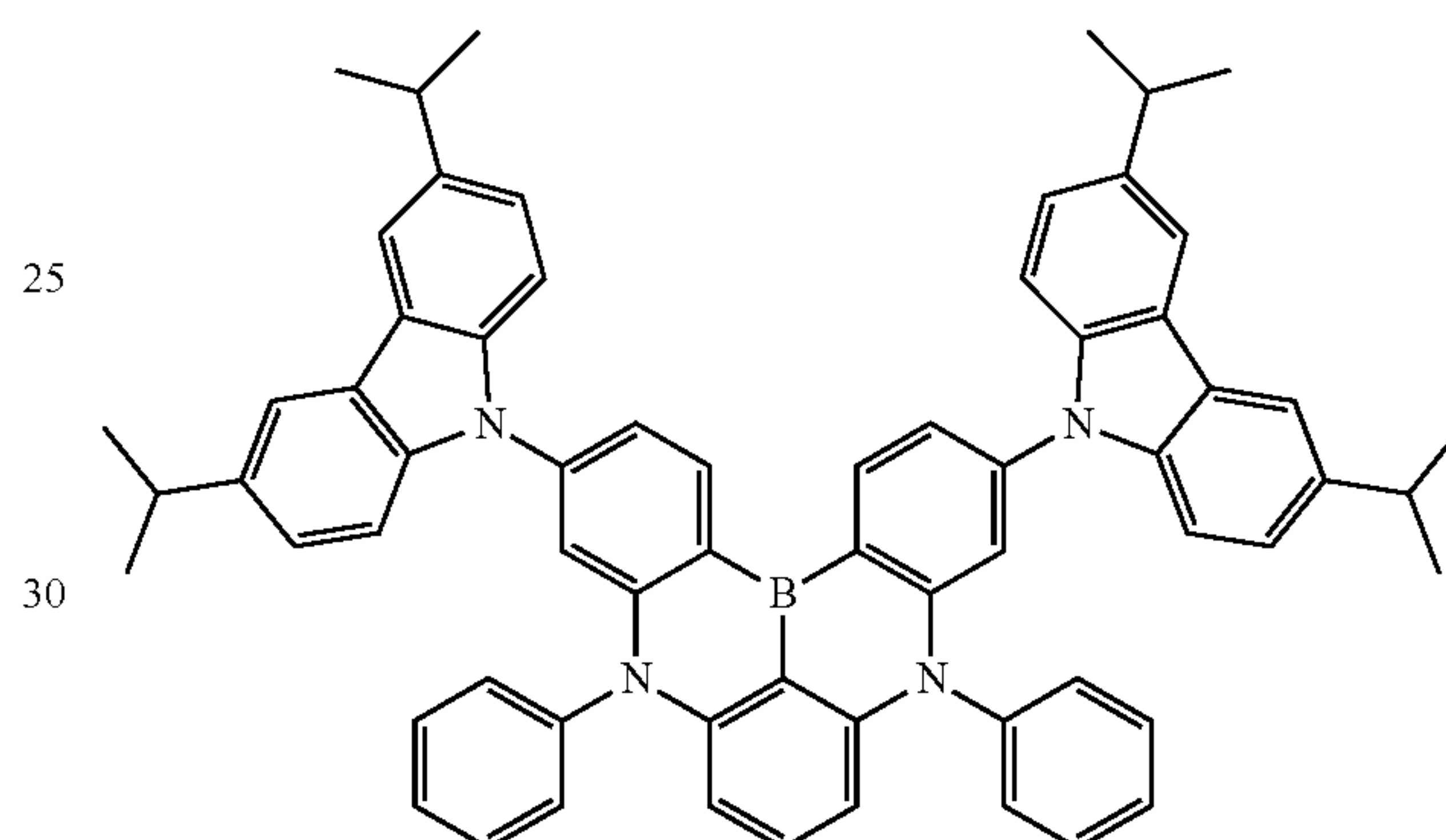
Dopant 75
