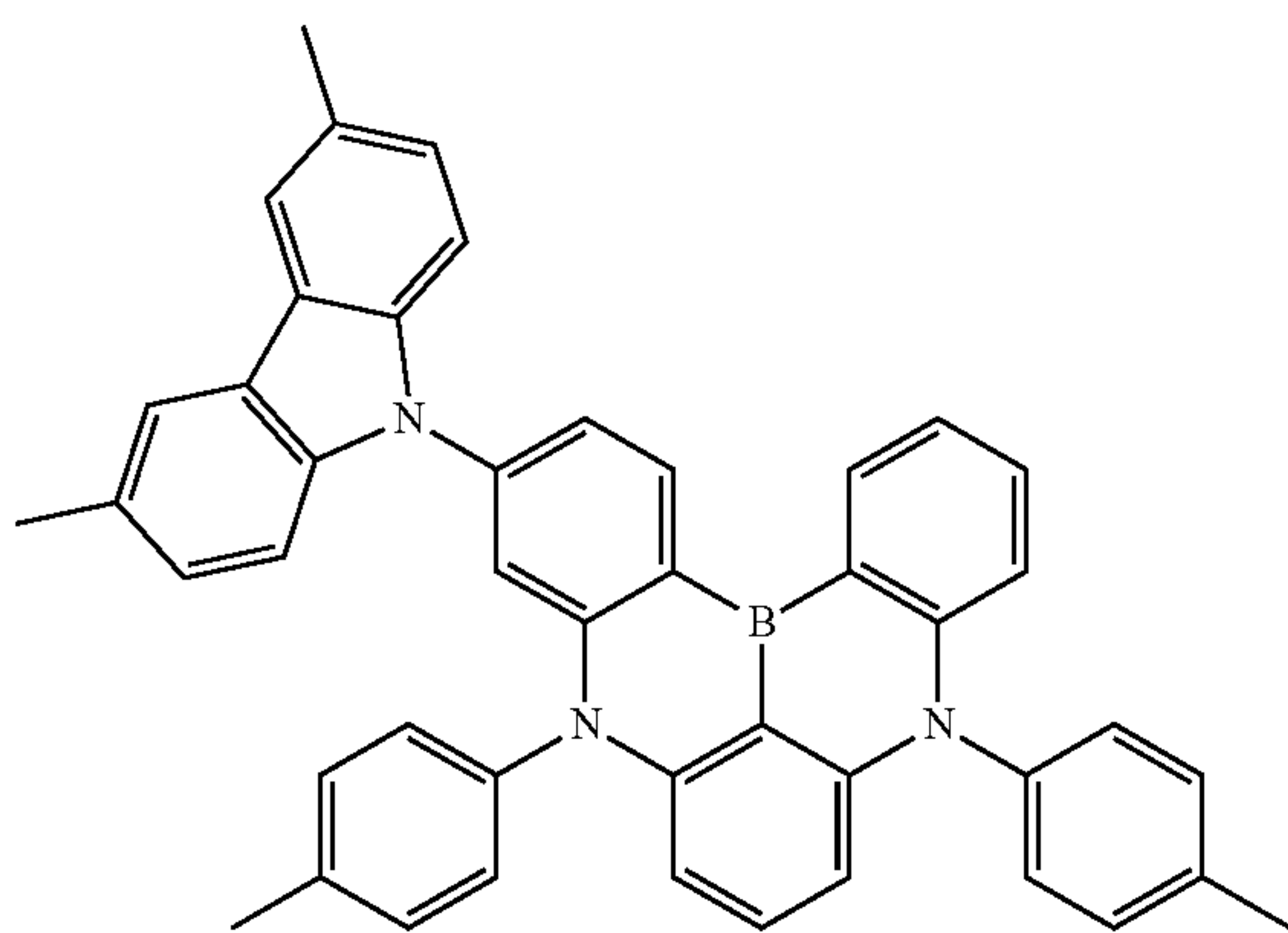
Dopant 68
