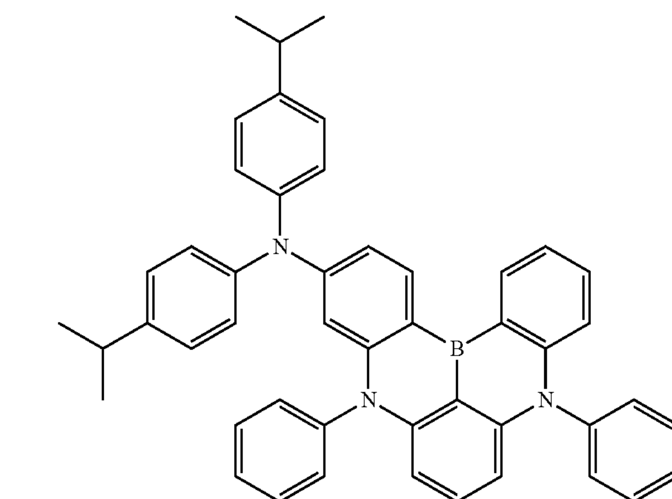
Dopant 56
