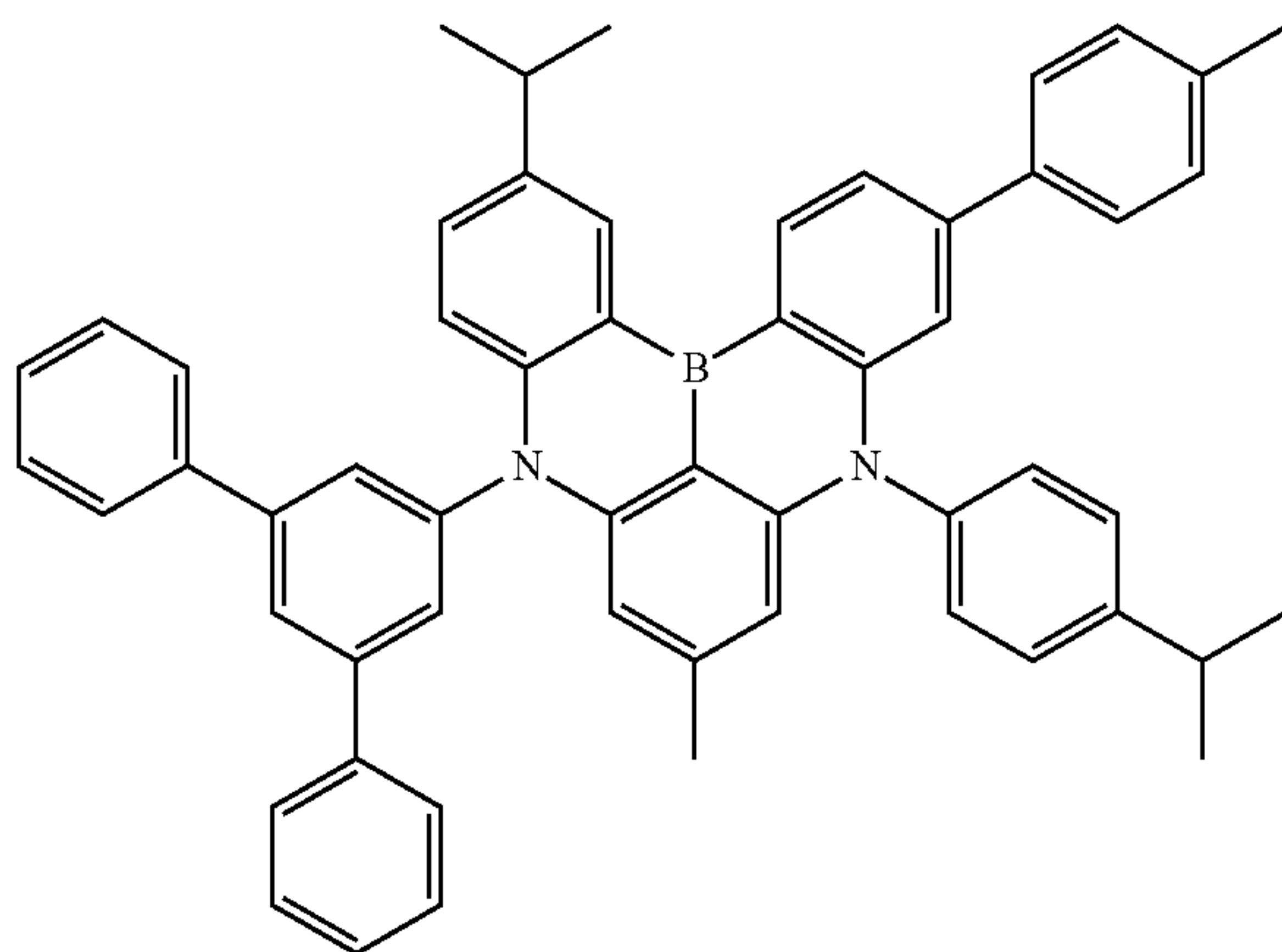
Dopant 160
