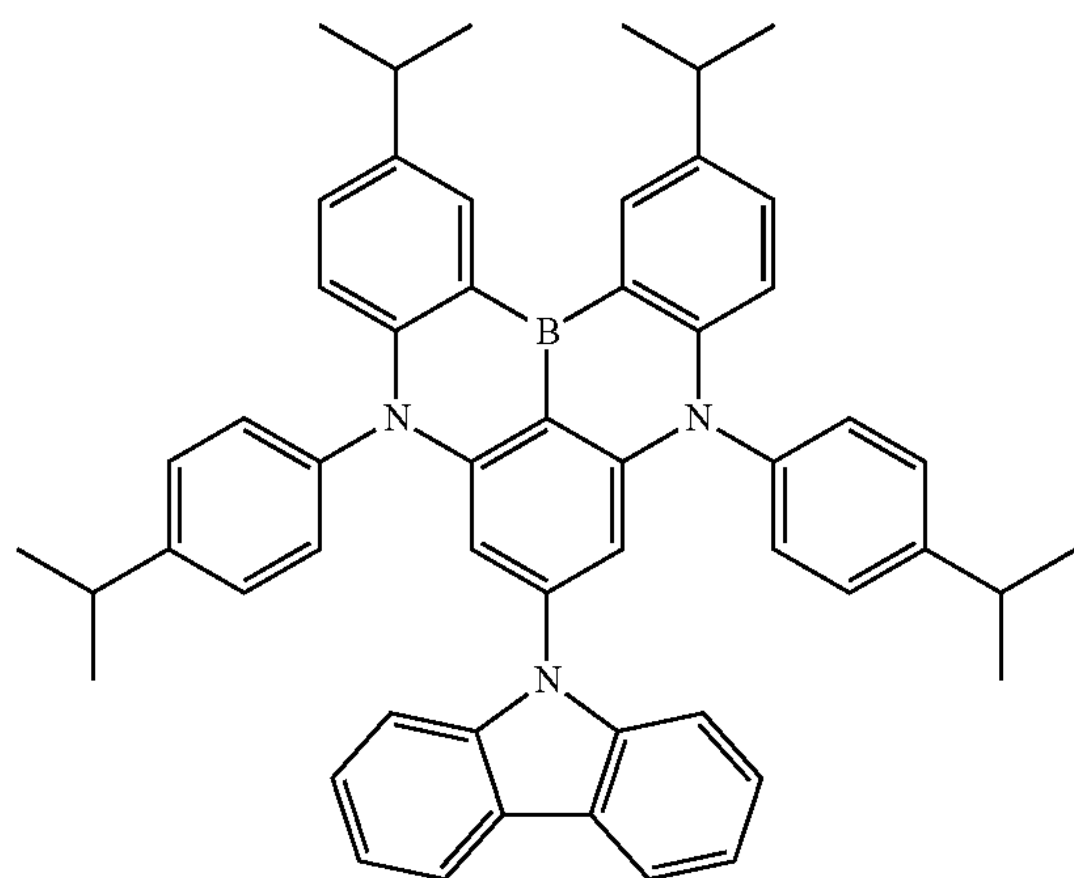
Dopant 66
