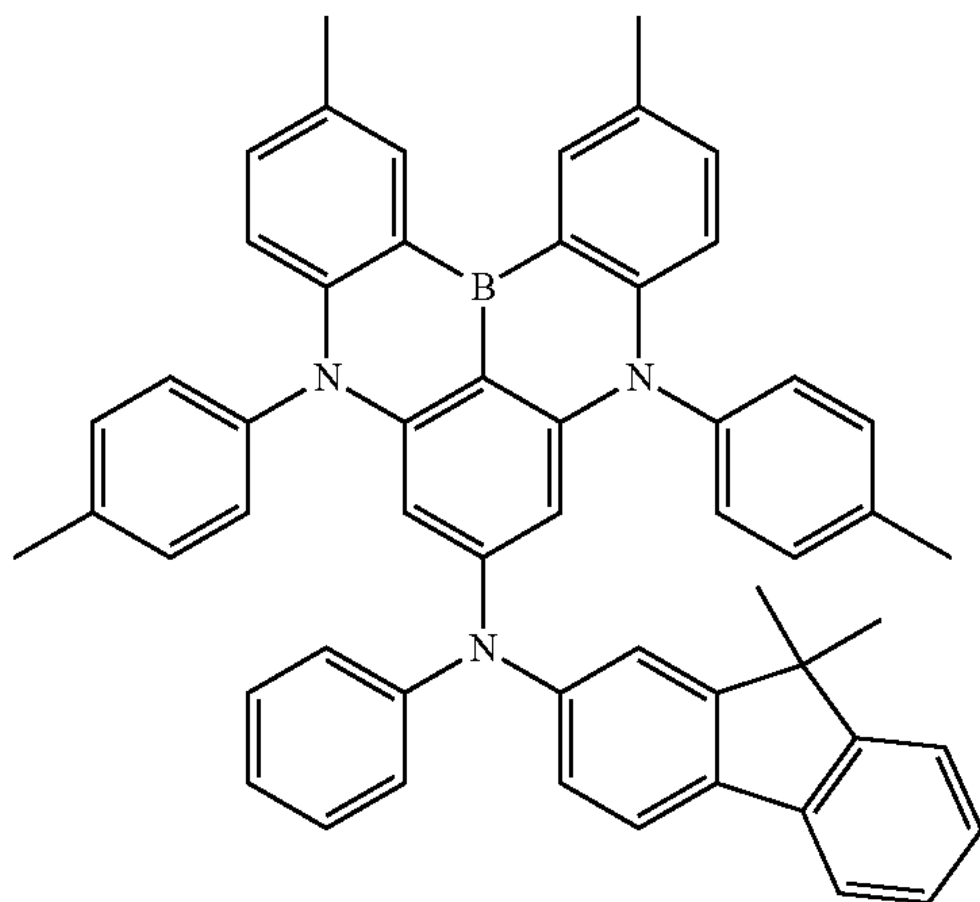
Dopant 128
