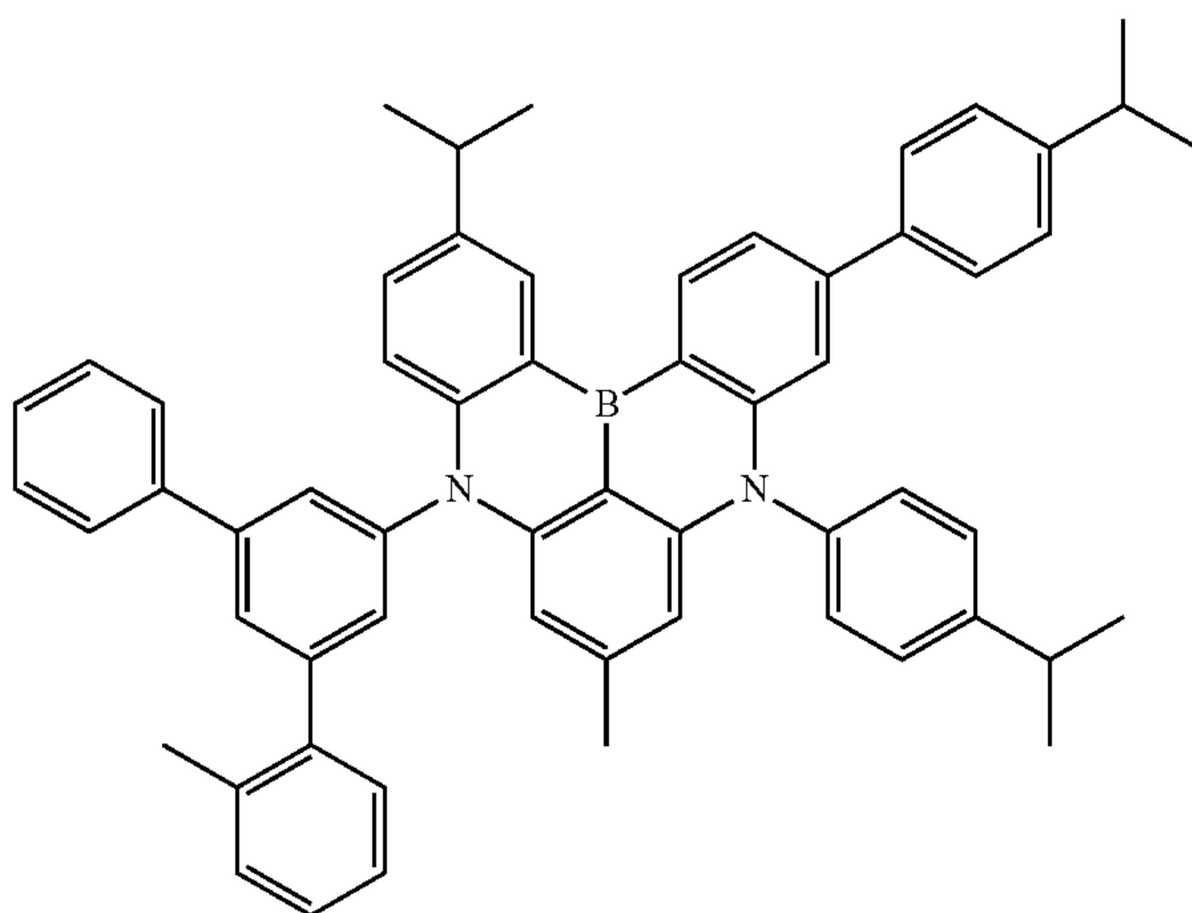
Dopant 158
