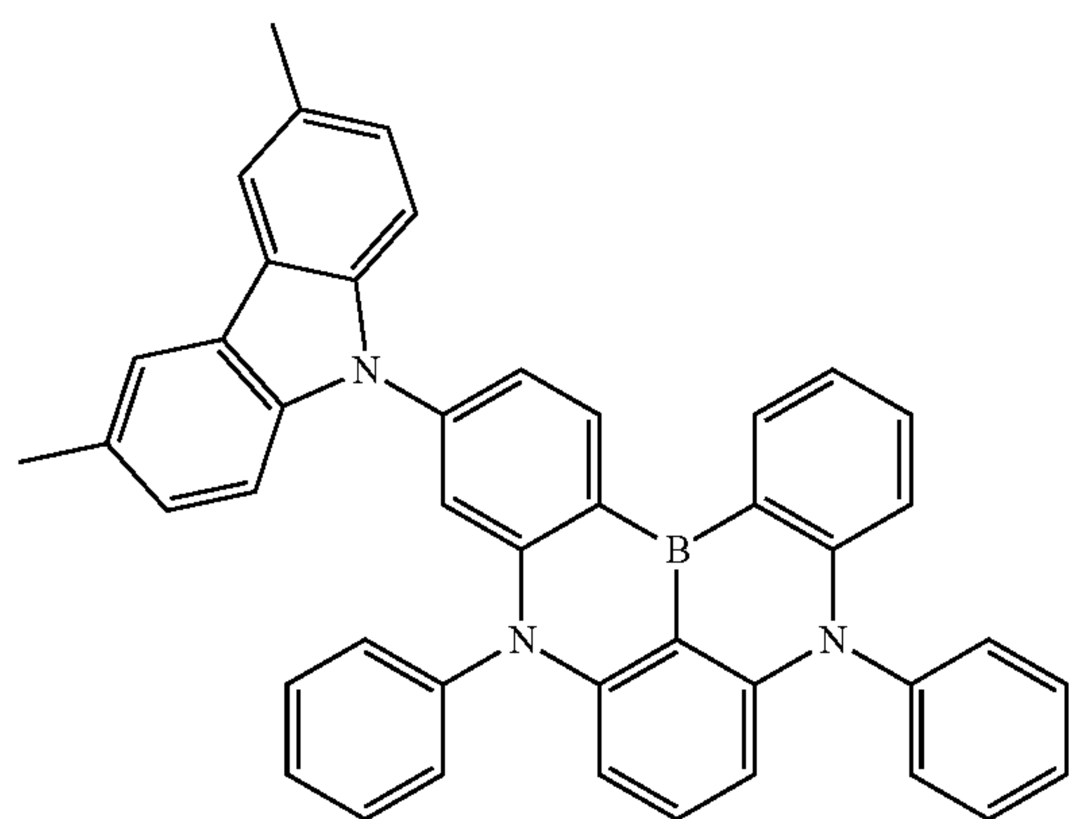
Dopant 68
