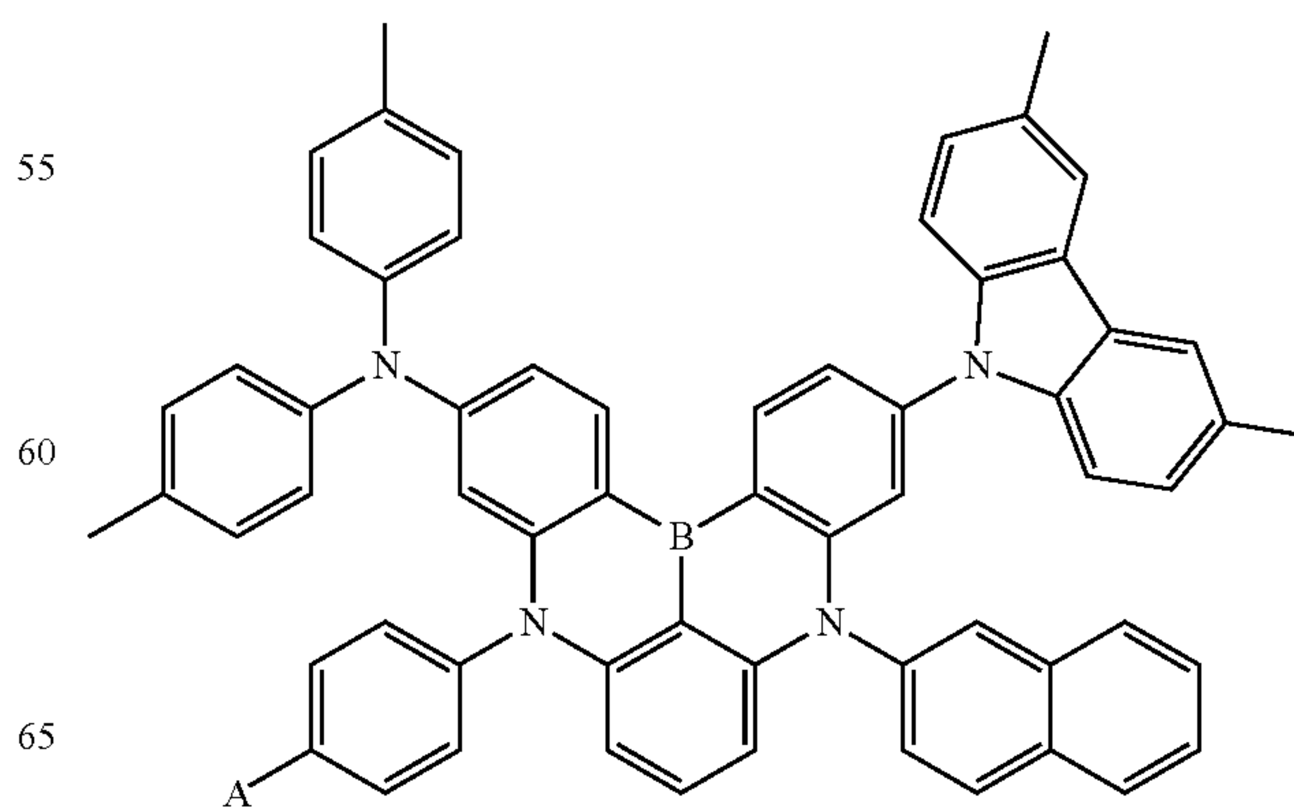
Dopant 112
