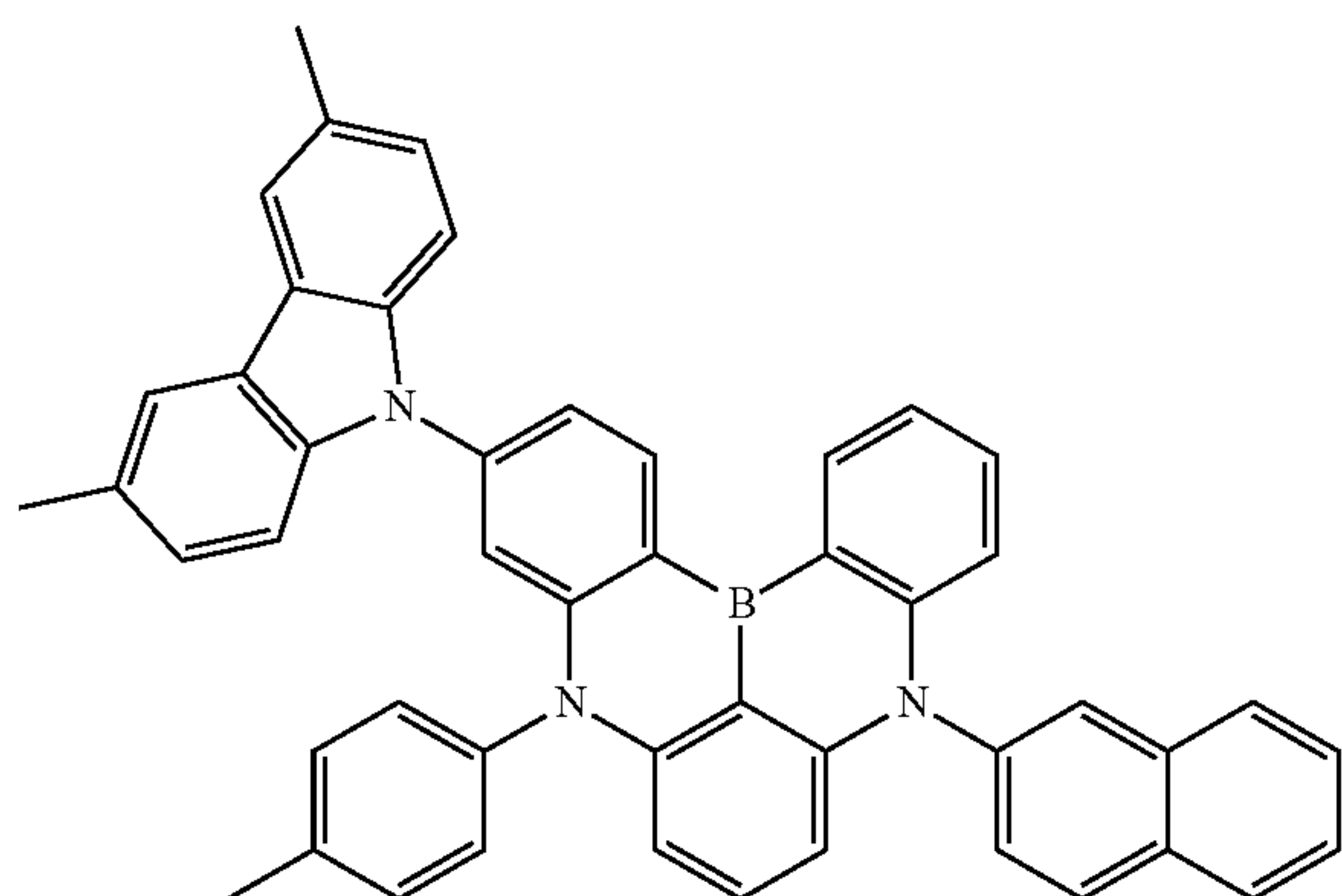
Dopant 103
