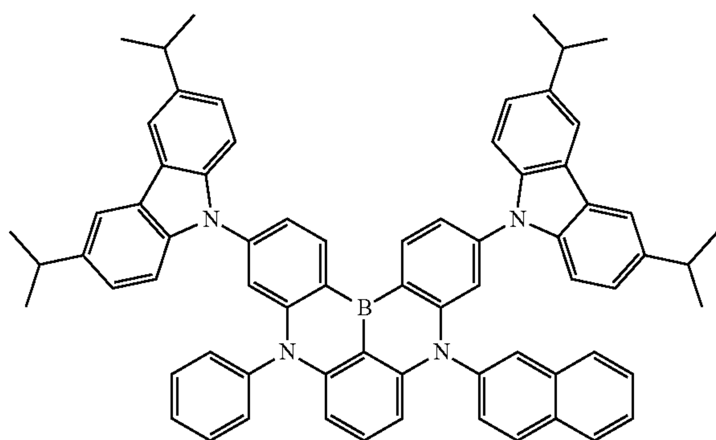
Dopant 110
