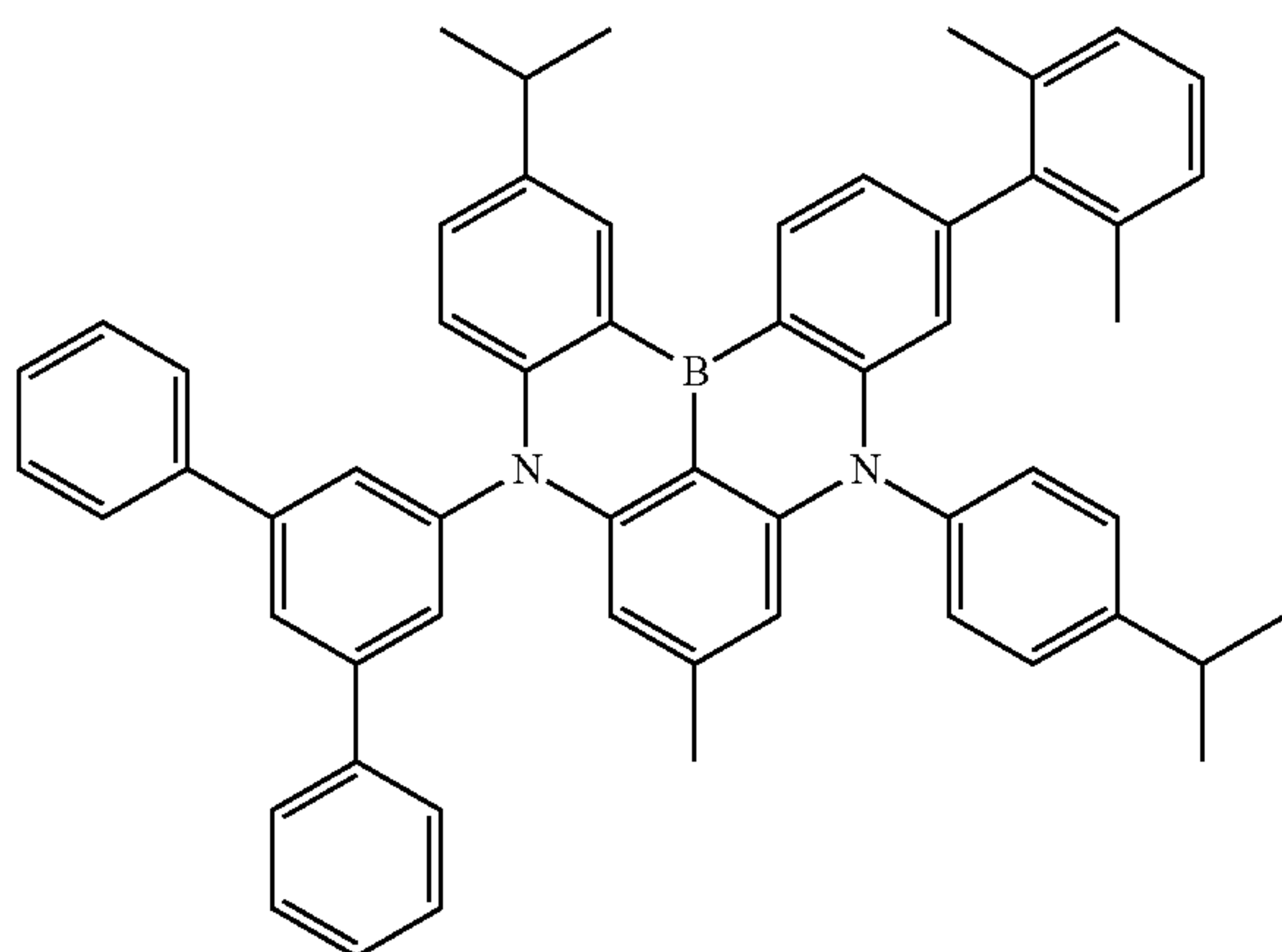
Dopant 161
