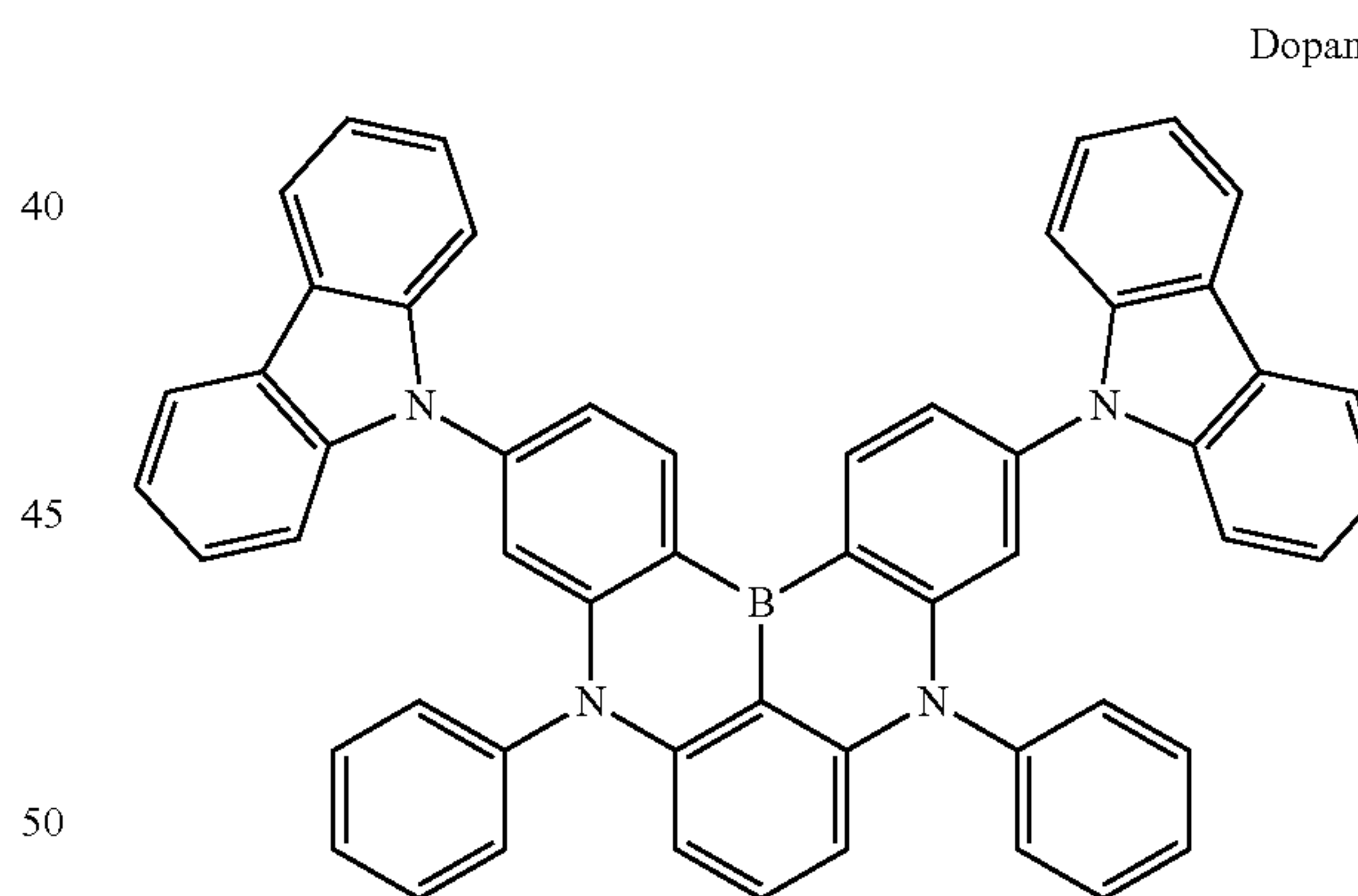
Dopant 72
