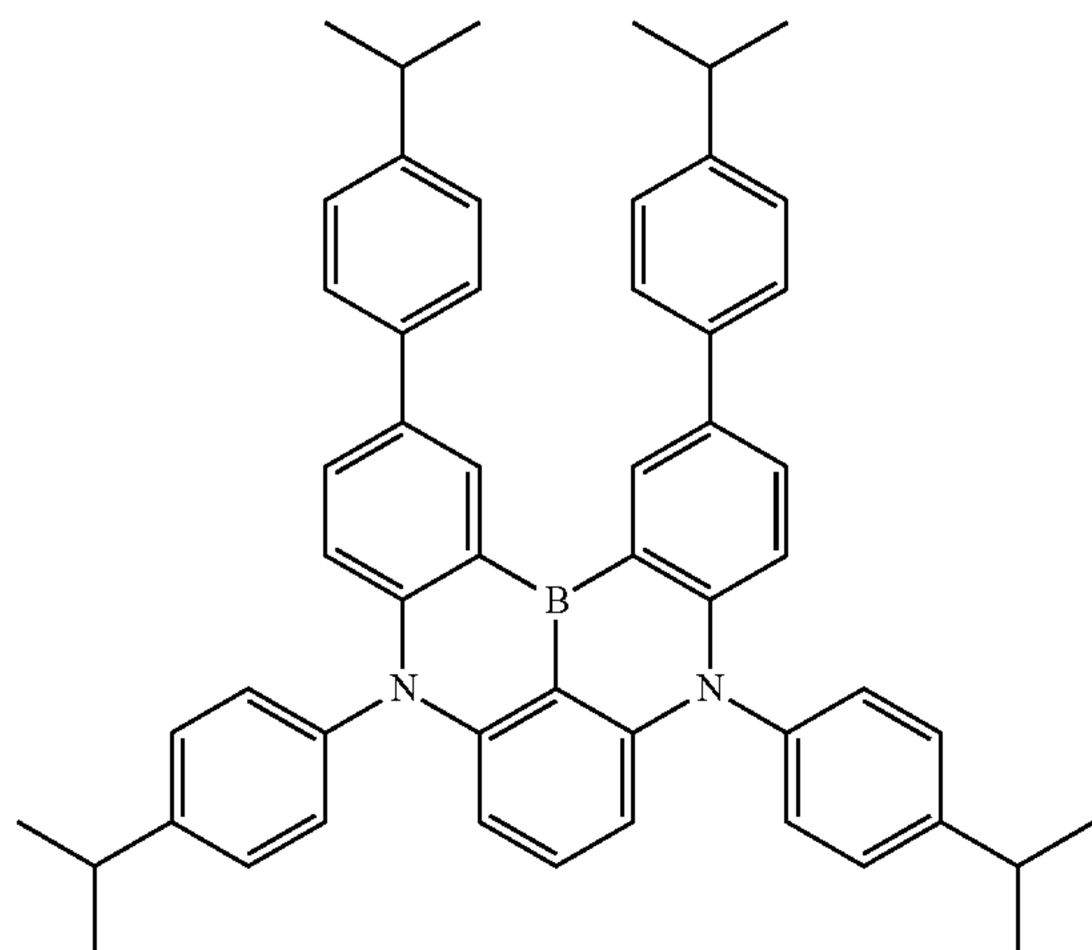
Dopant 14
