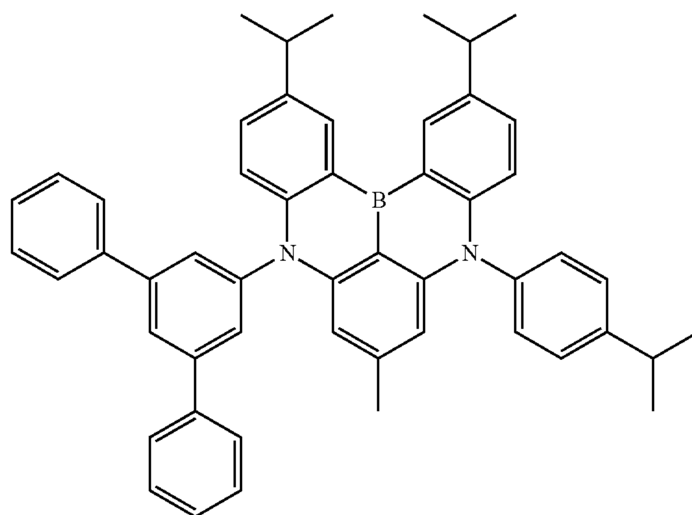
Dopant 149
