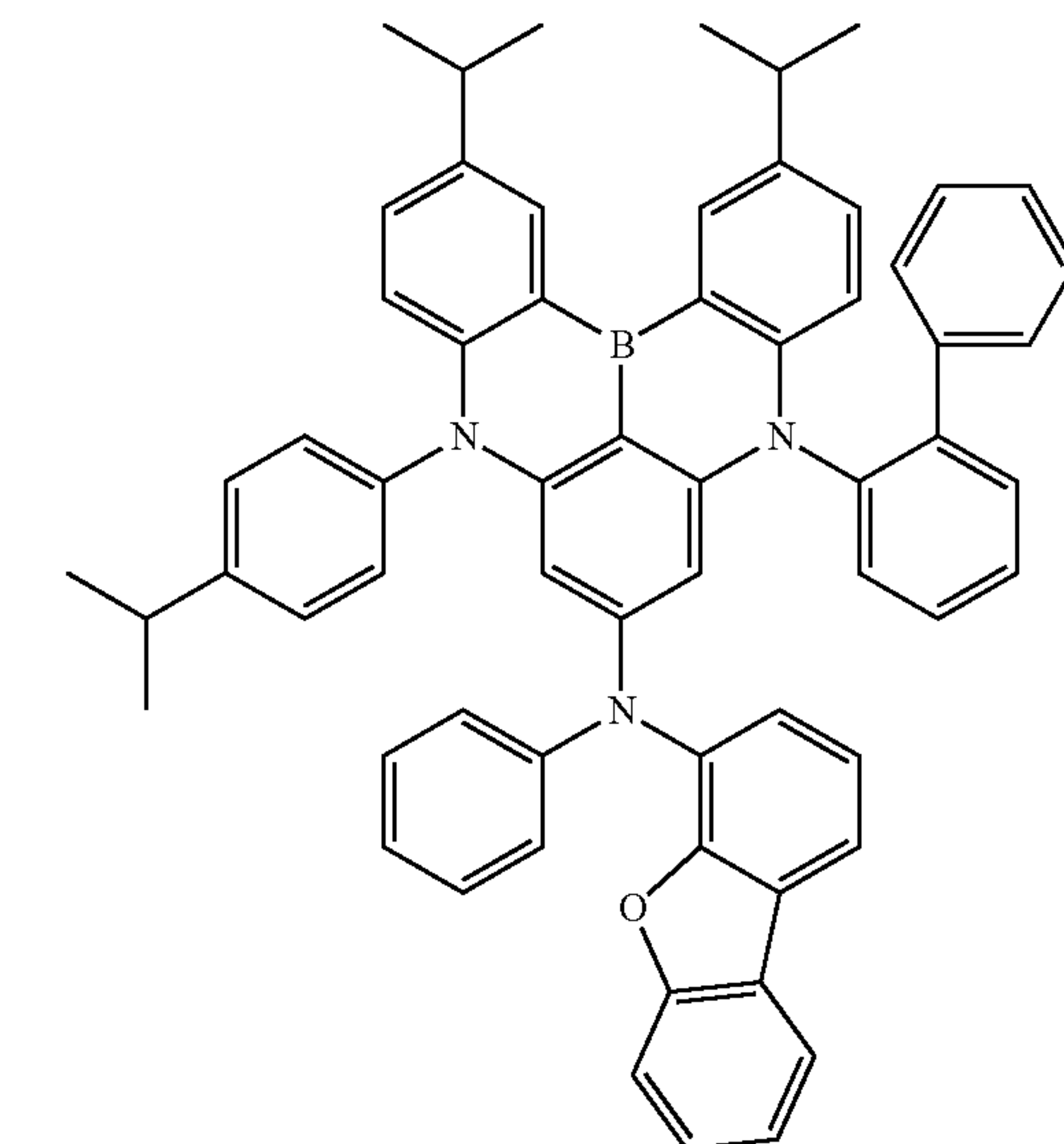
Dopant 118
