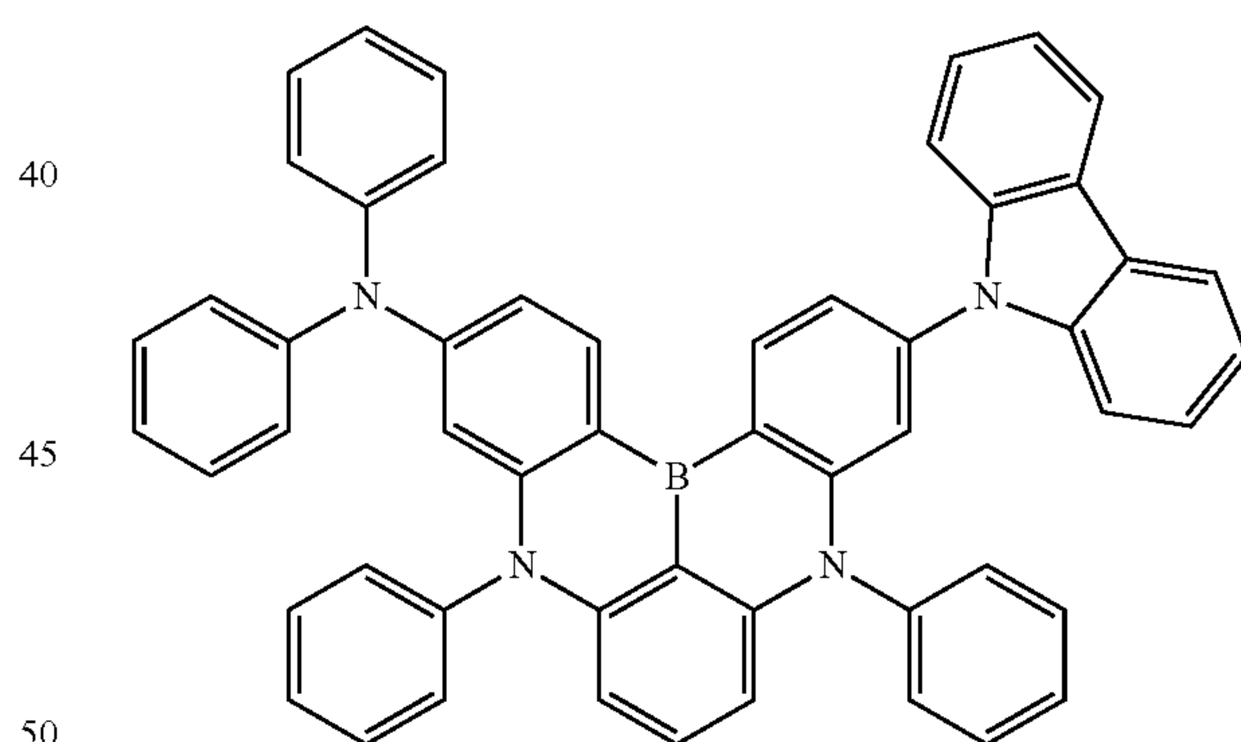
Dopant 77
