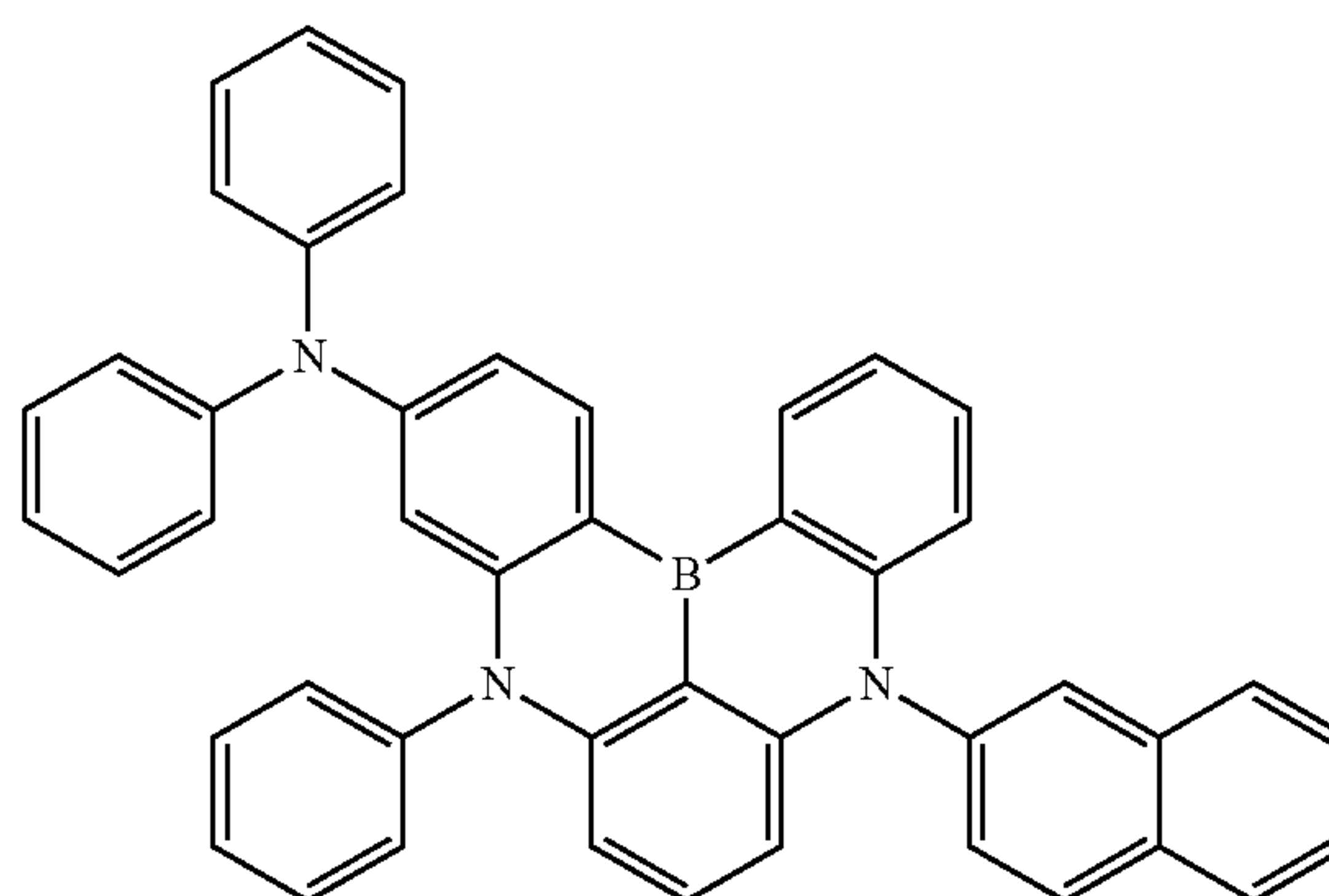
Dopant 86
