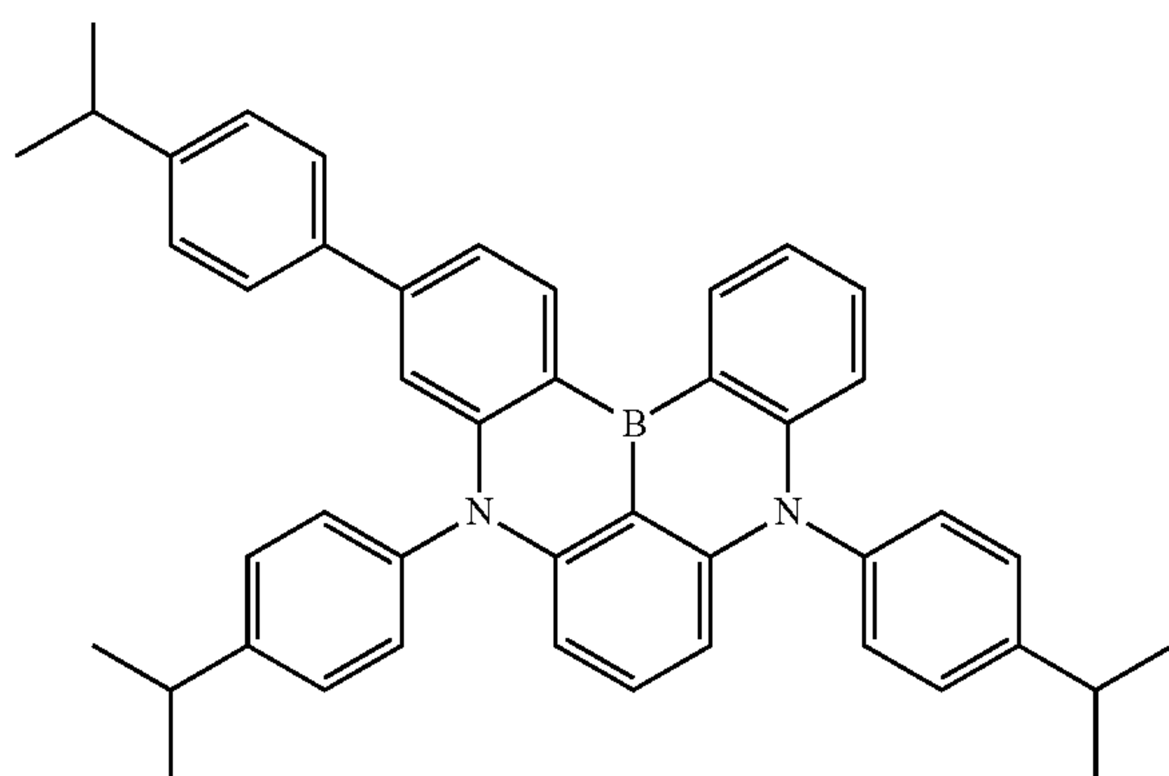
Dopant 19
