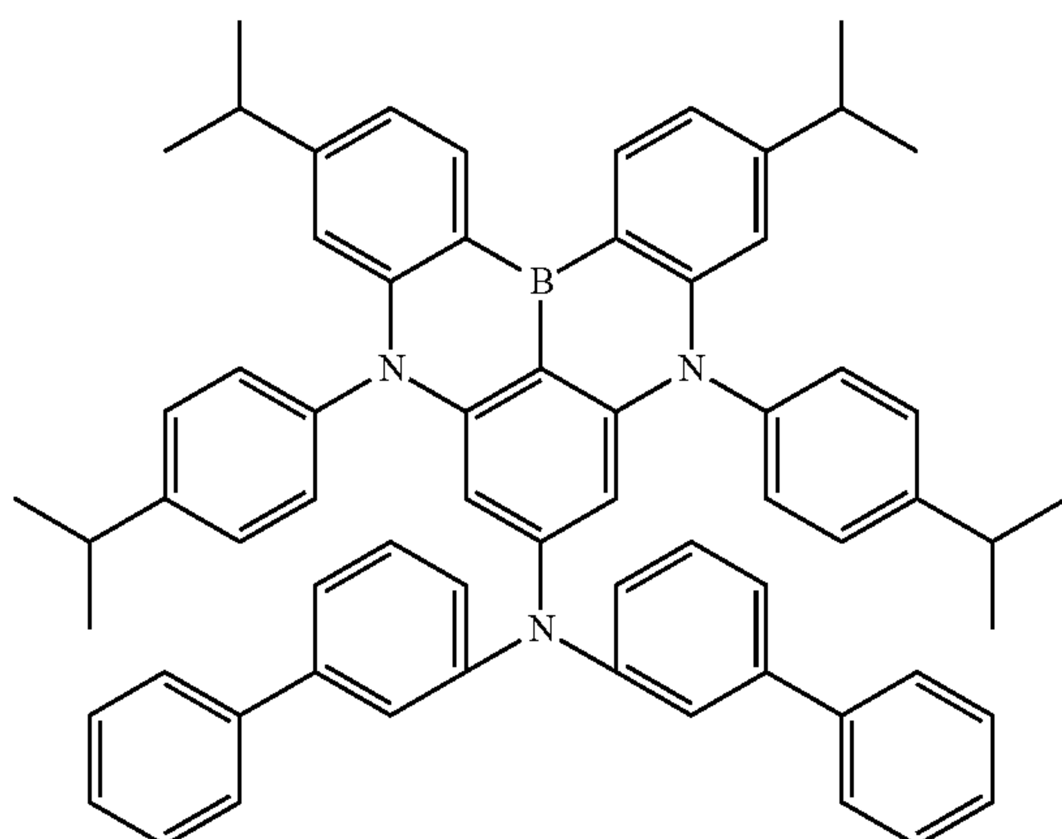
Dopant 143
