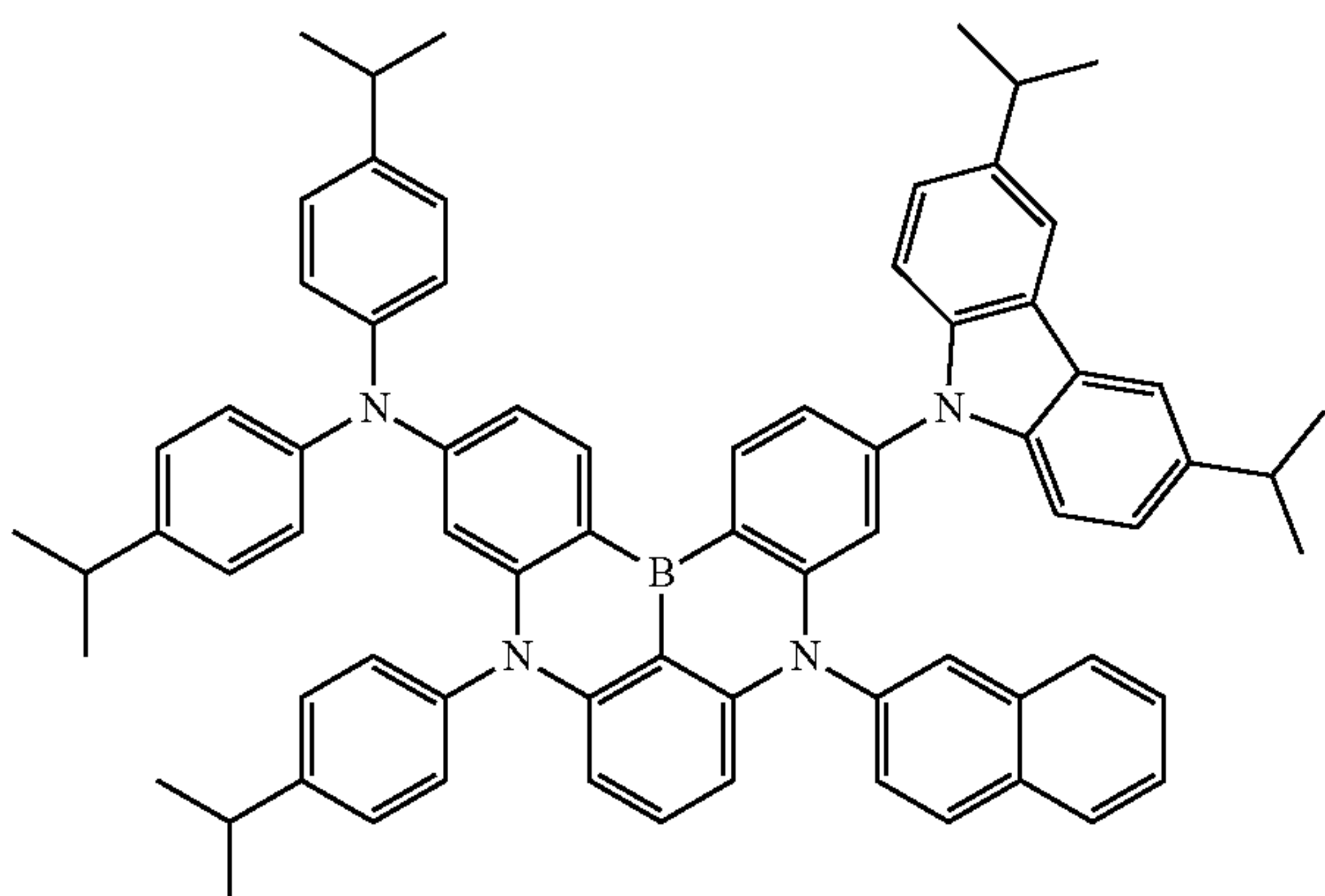
Dopant 114
