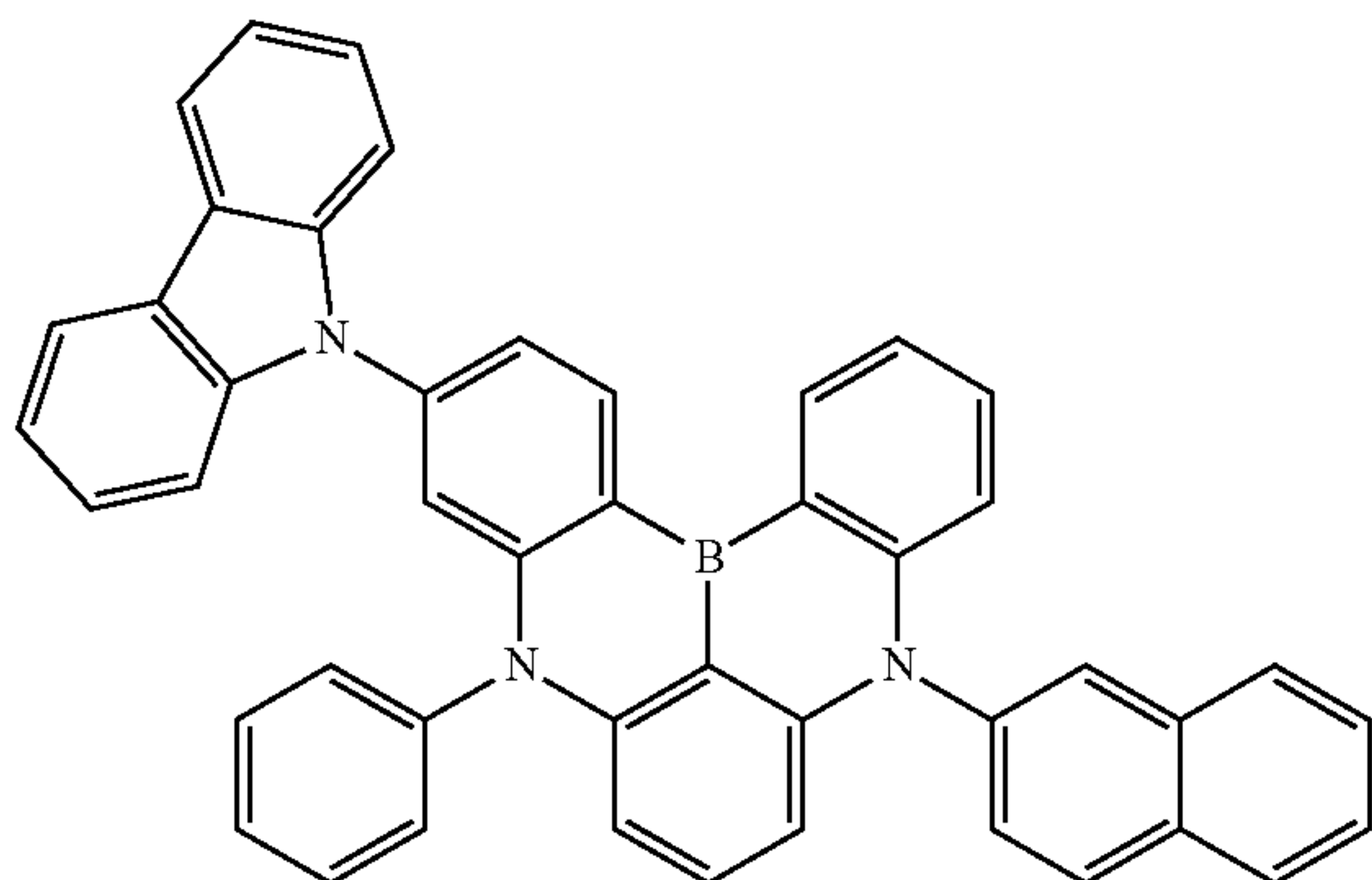
Dopant 102
