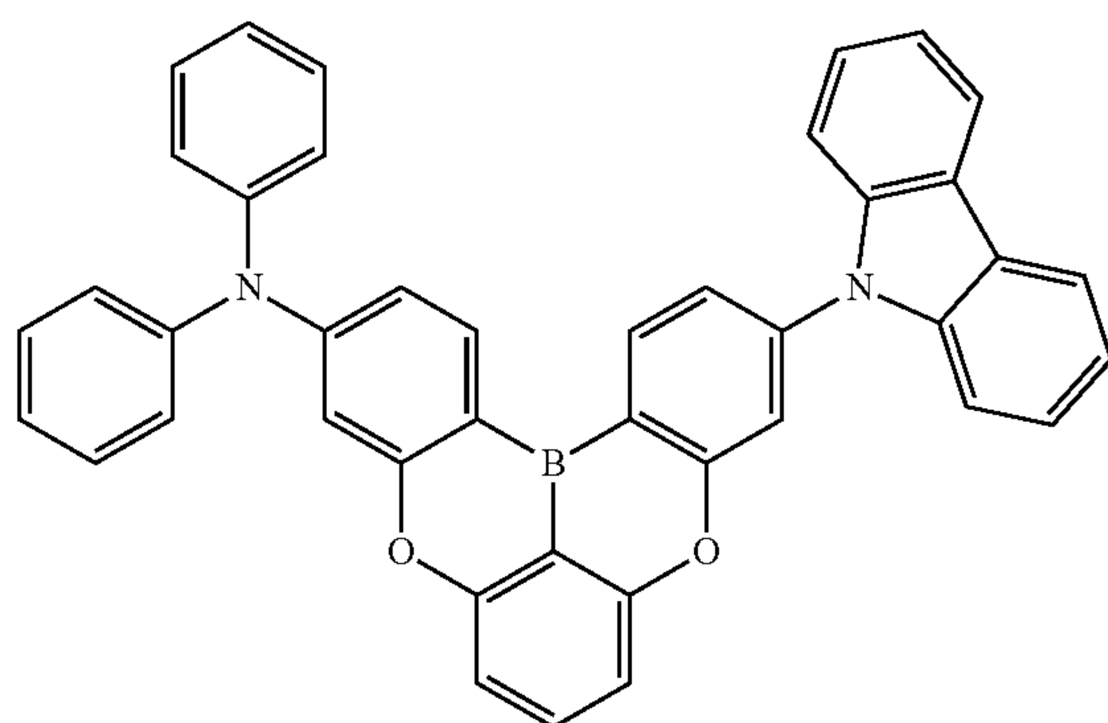
Dopant 187
