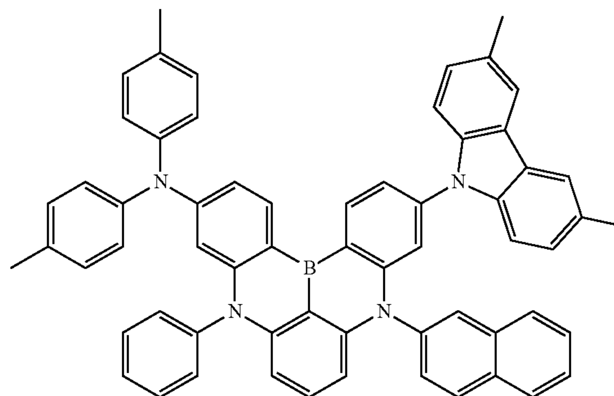
Dopant 113
