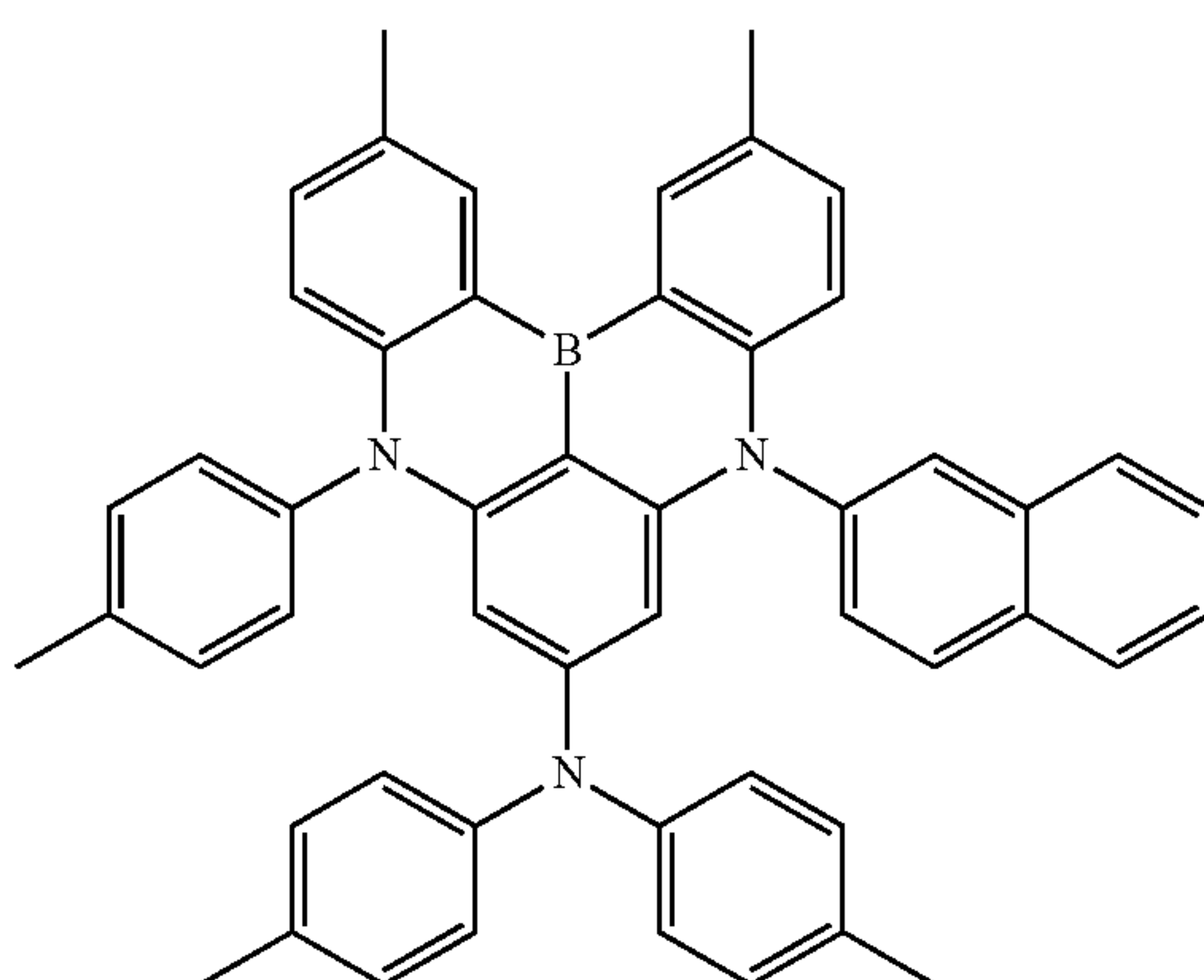
Dopant 82
