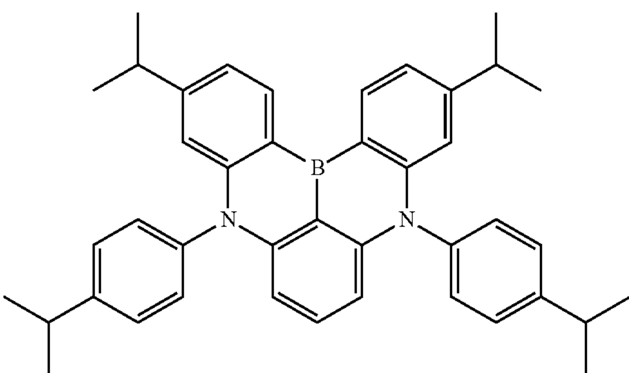
Dopant 4
