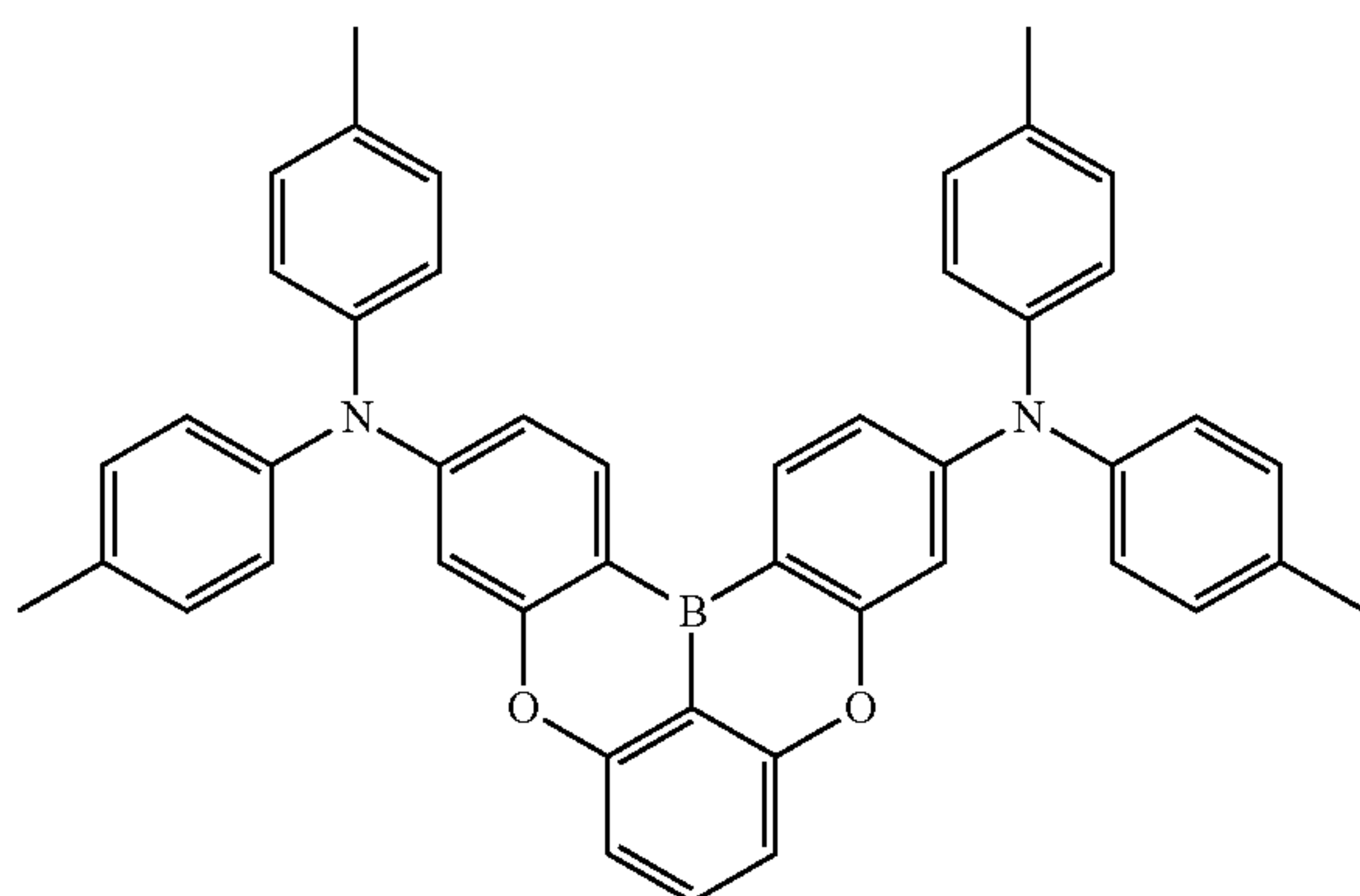
Dopant 191
