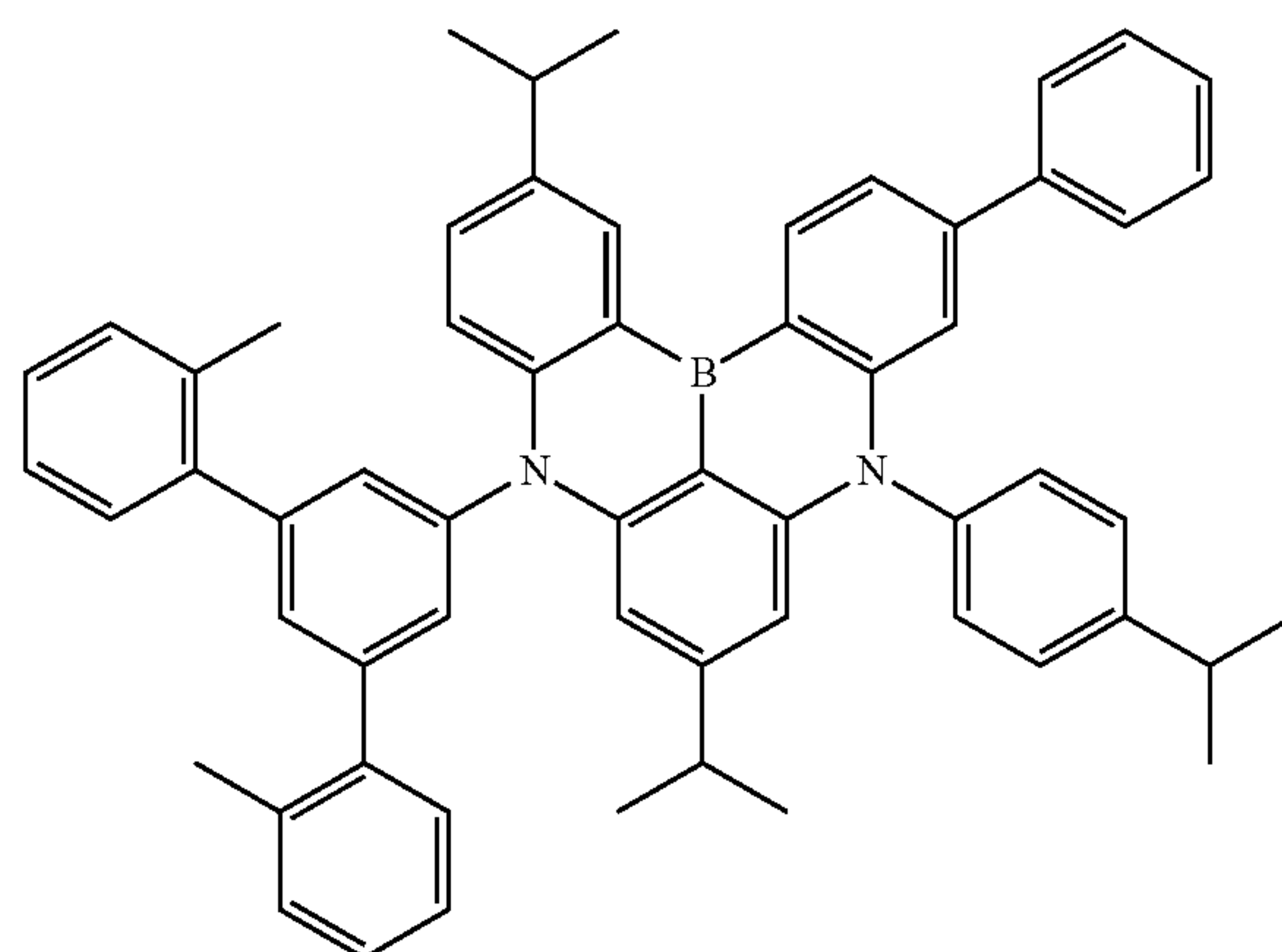
Dopant 165
