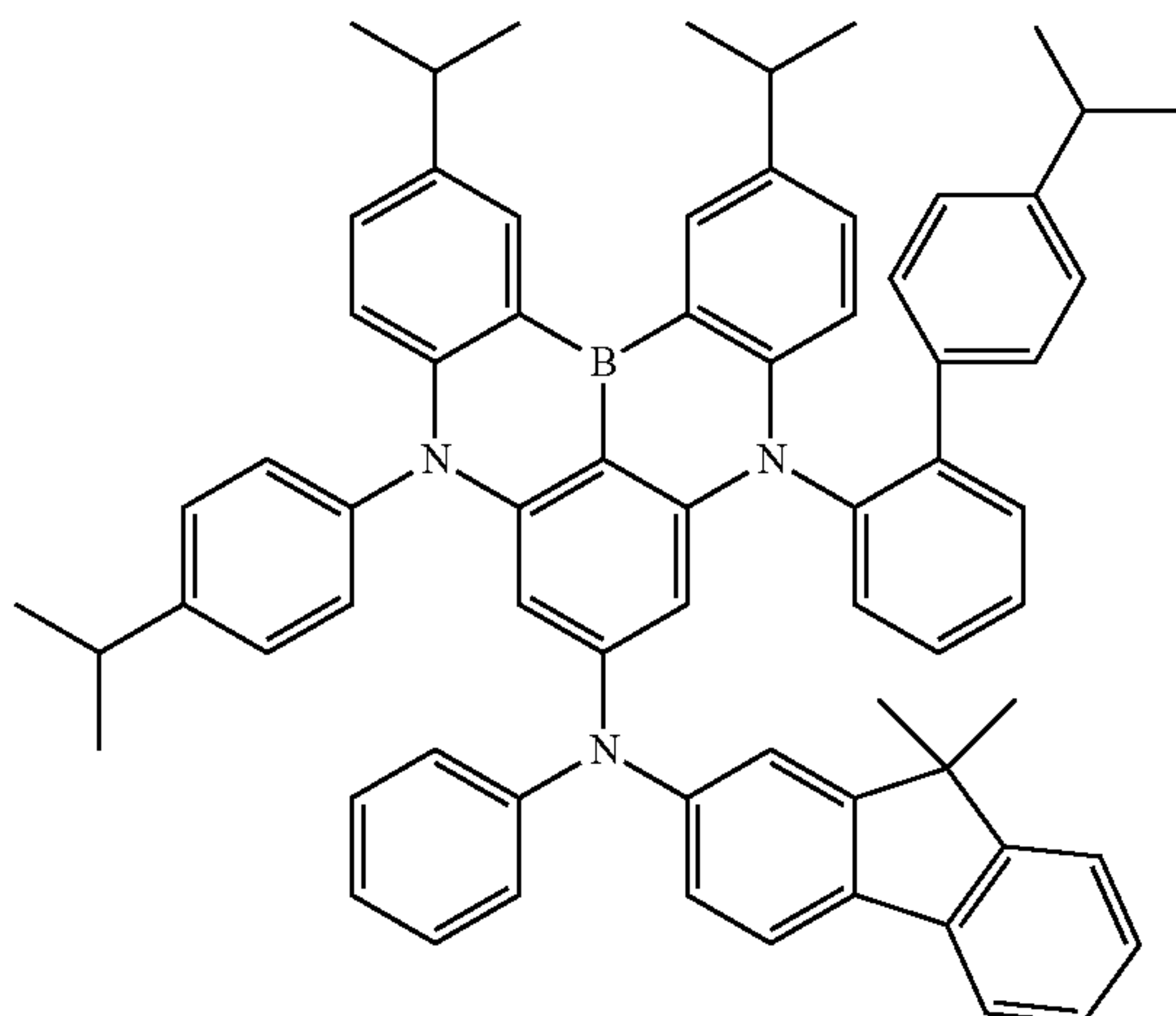
Dopant 130
