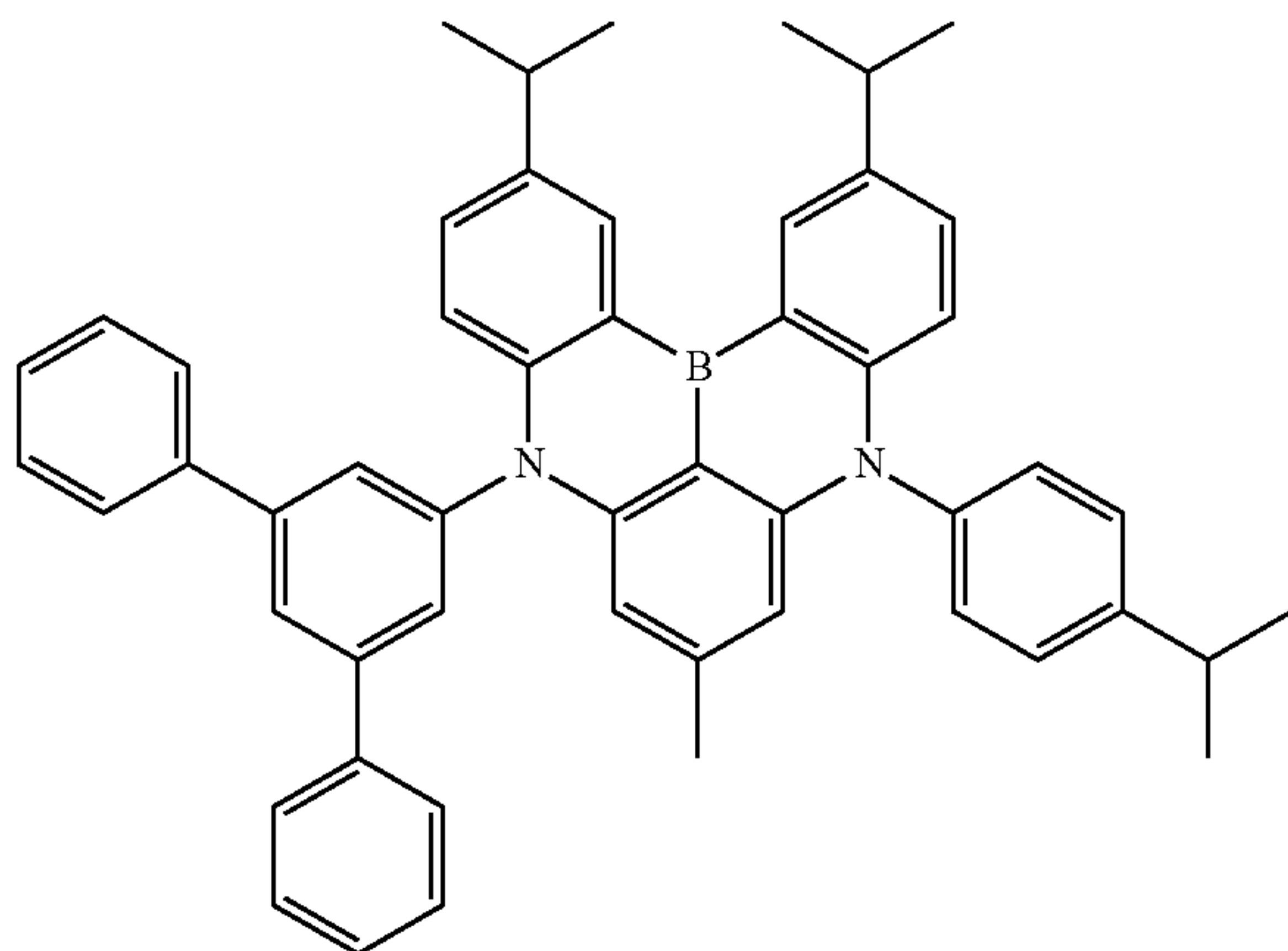
Dopant 149
