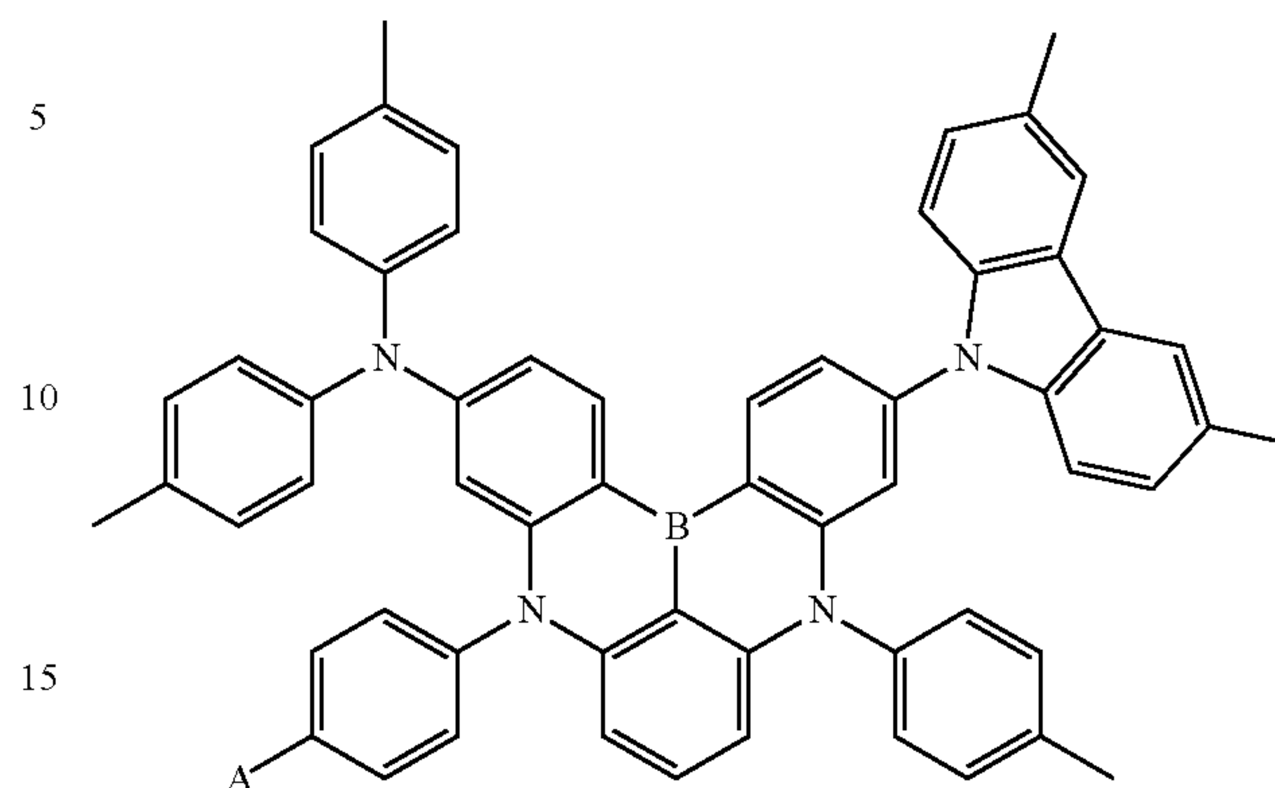
Dopant 77
