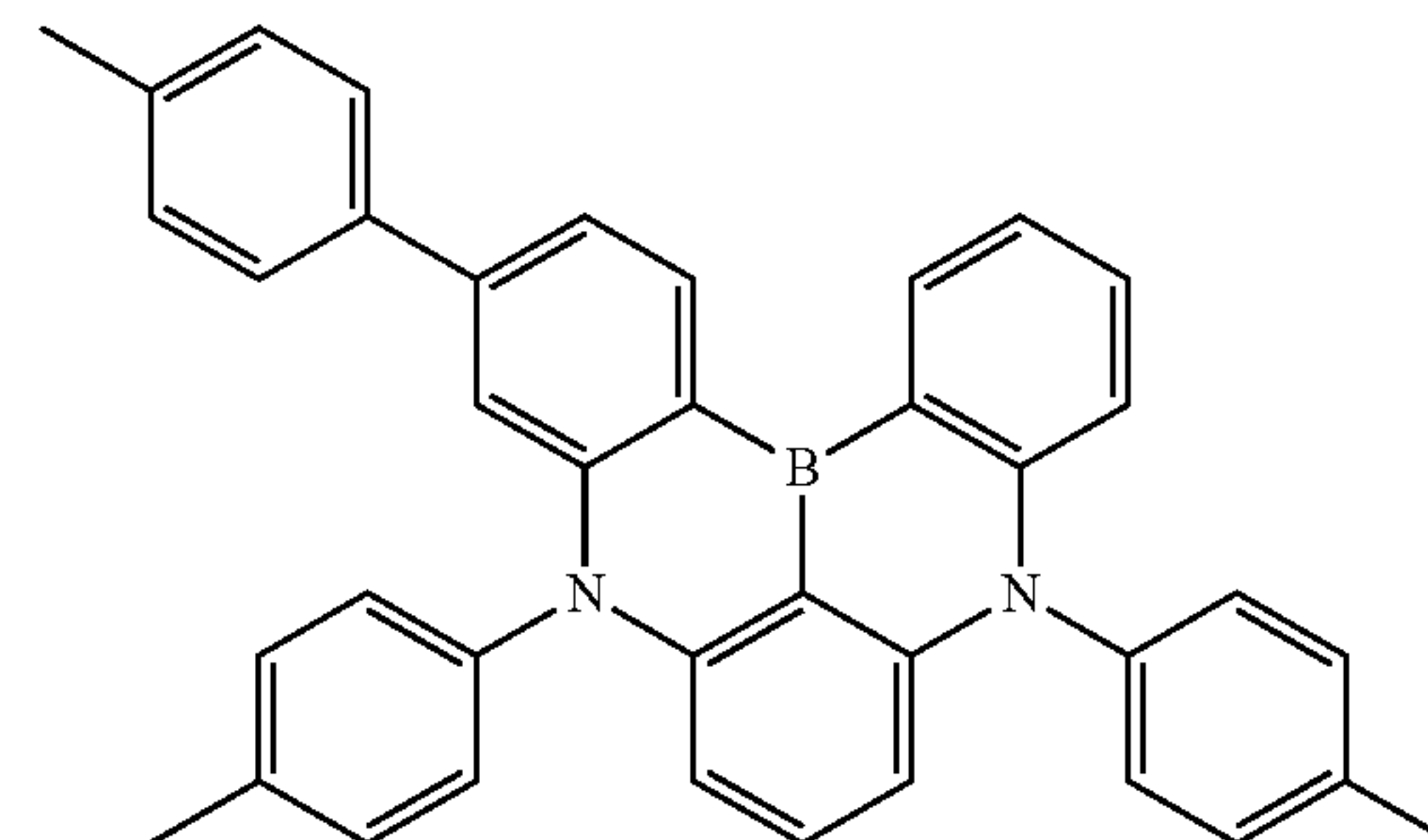
Dopant 17
