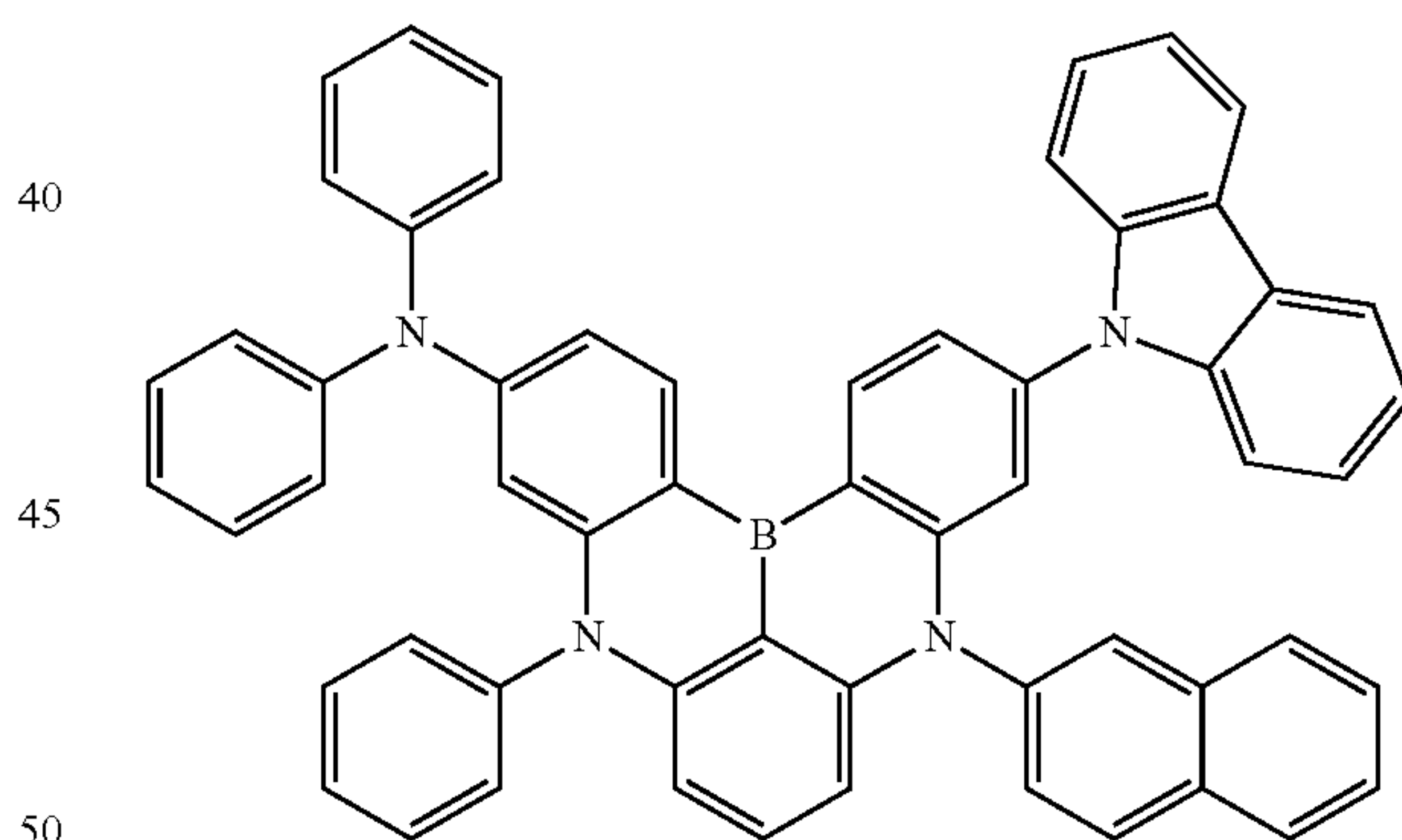
Dopant 112
