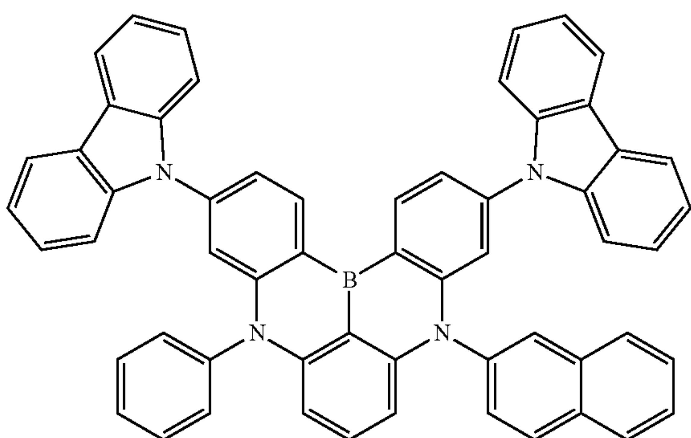
Dopant 106
