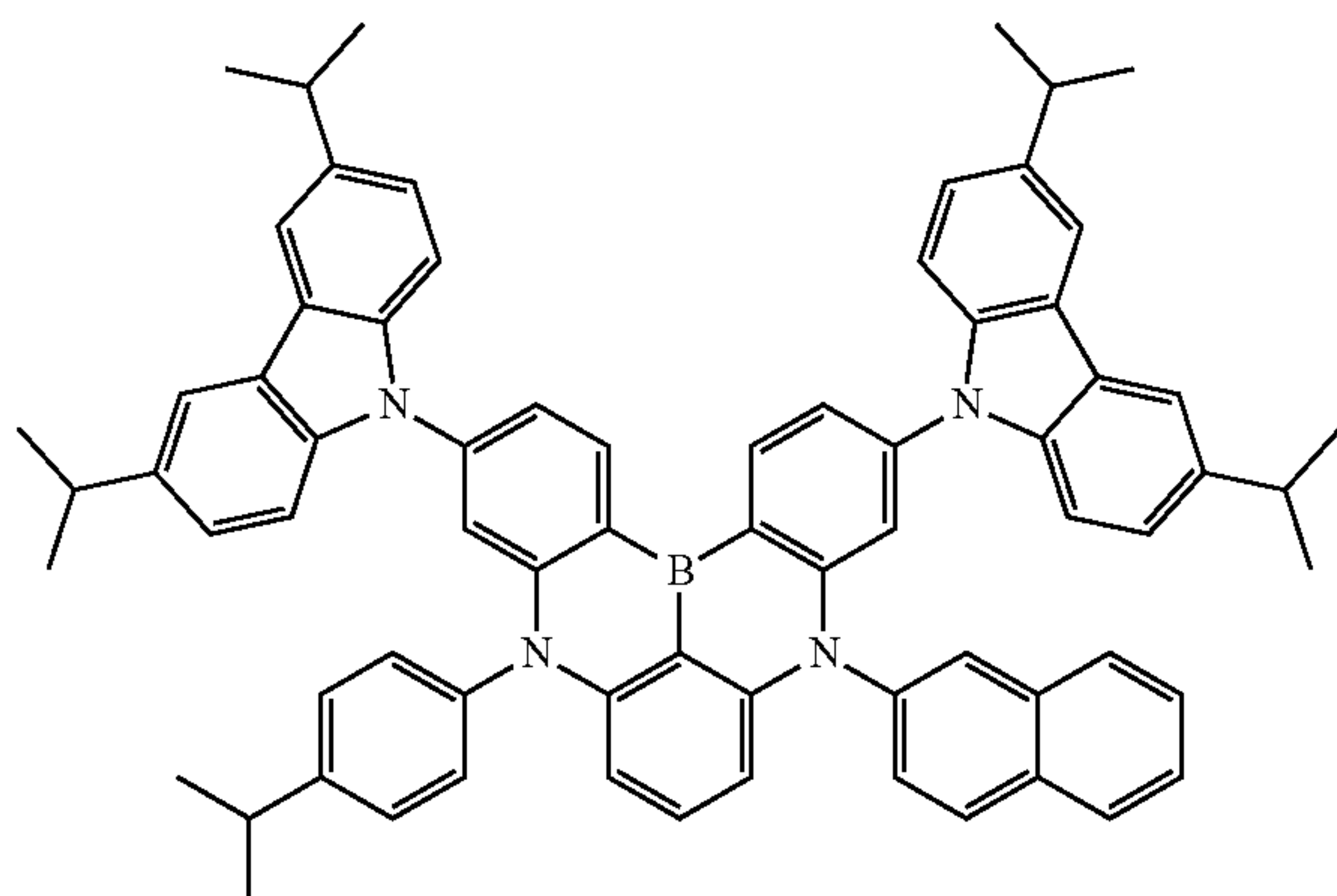
Dopant 109
