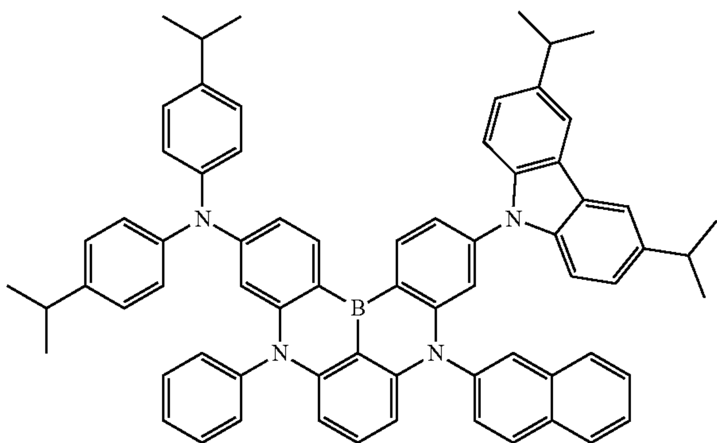
Dopant 115
