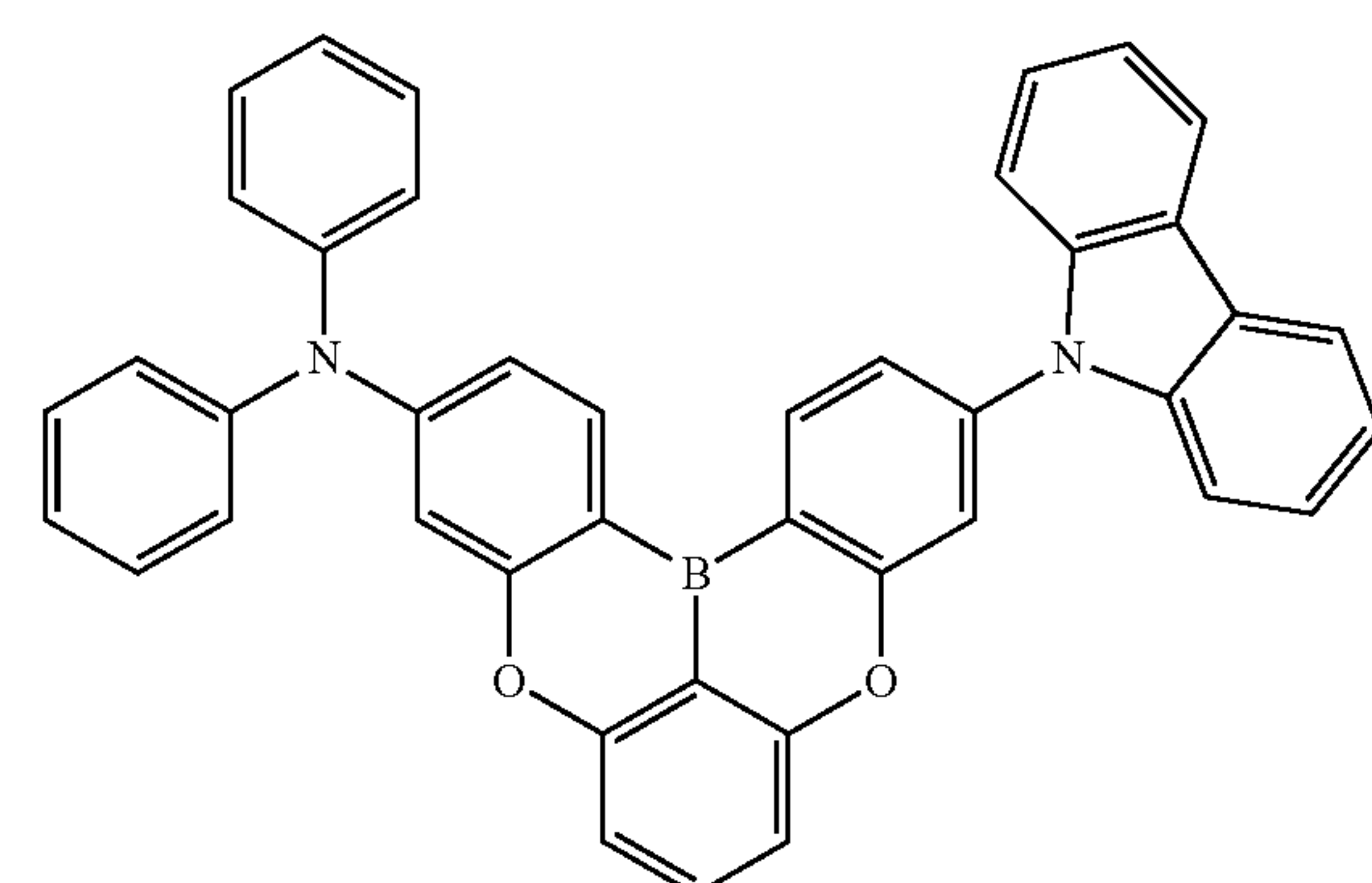
Dopant 188
