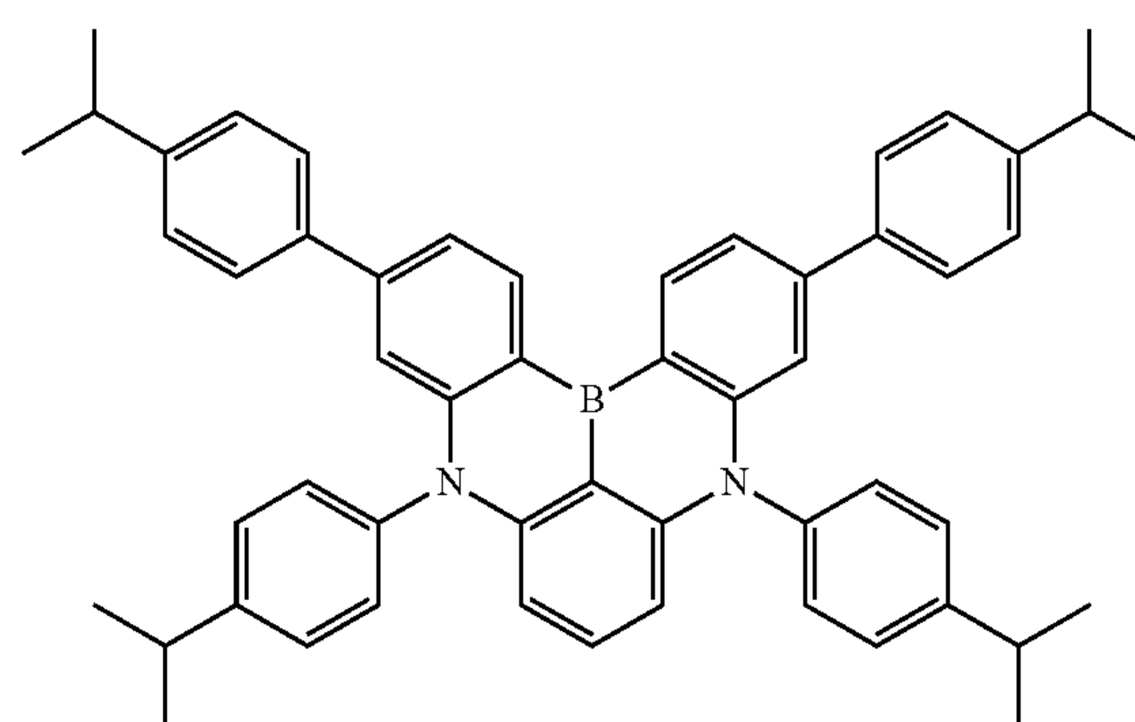
Dopant 9
