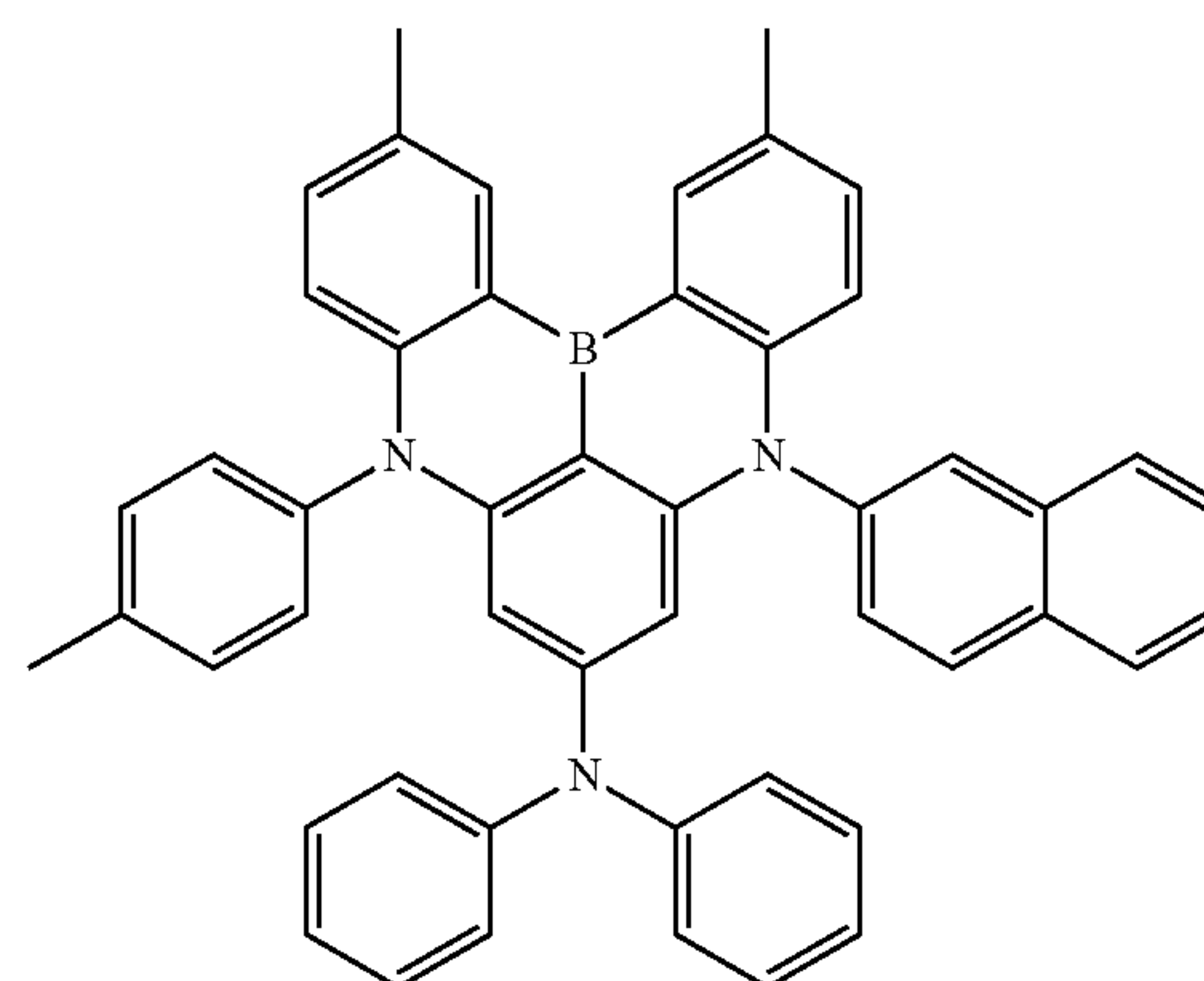
Dopant 83
