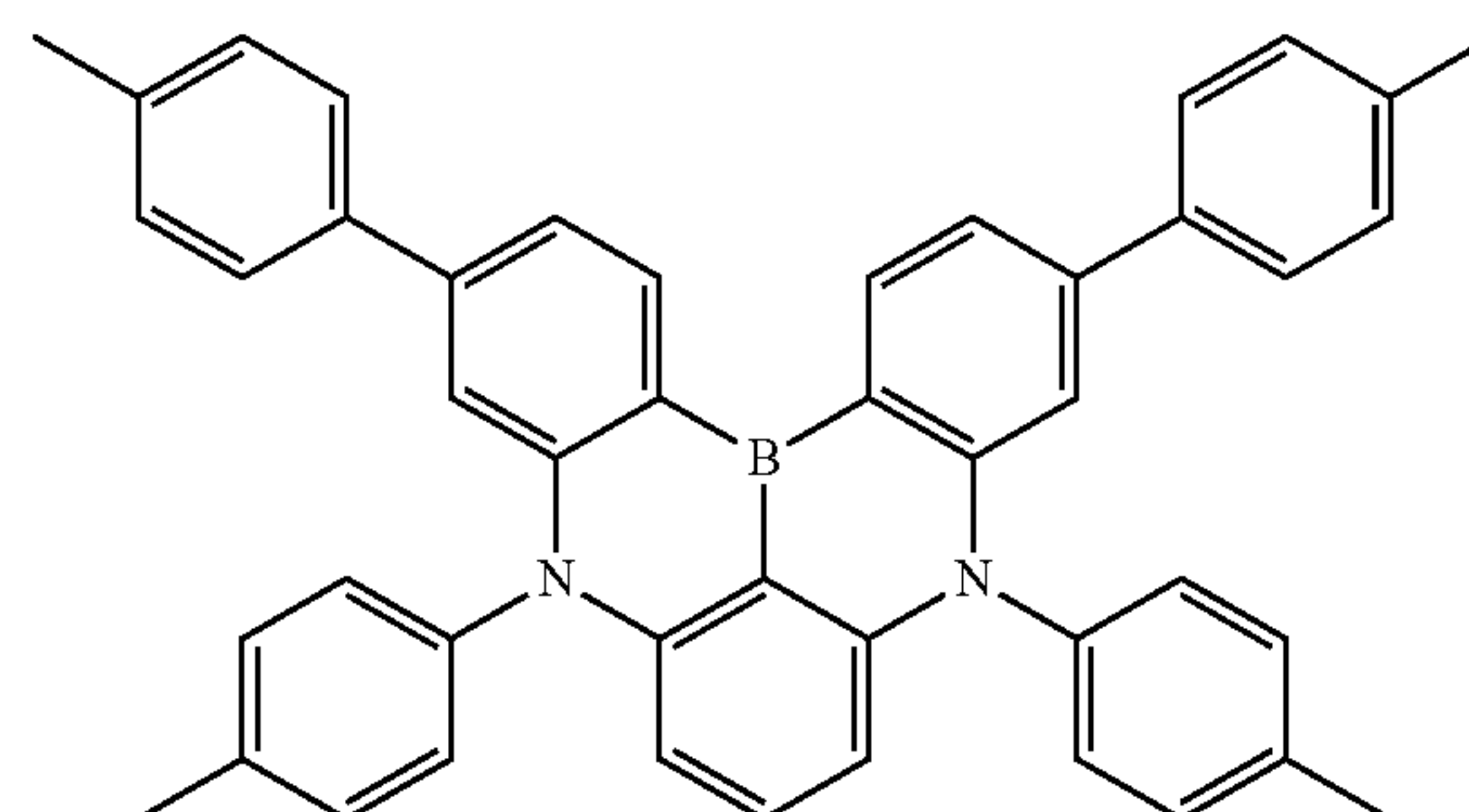
Dopant 8
