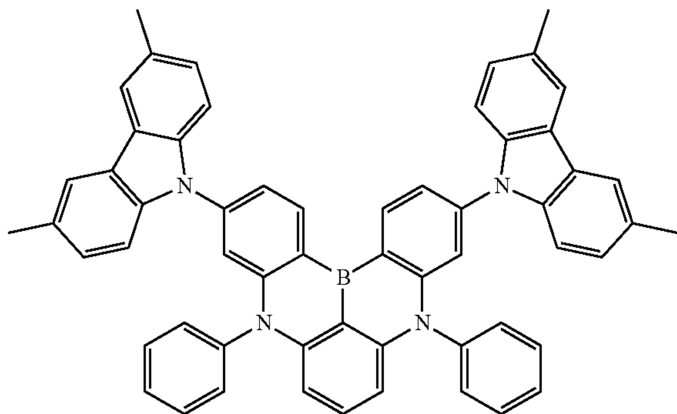
Dopant 73
