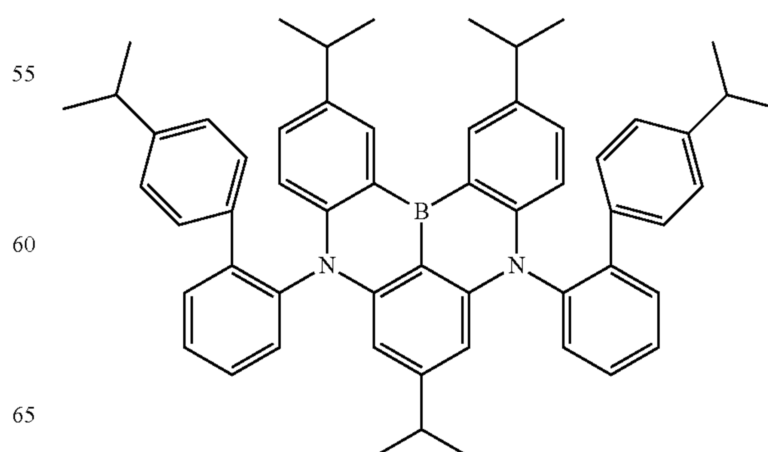
Dopant 148
