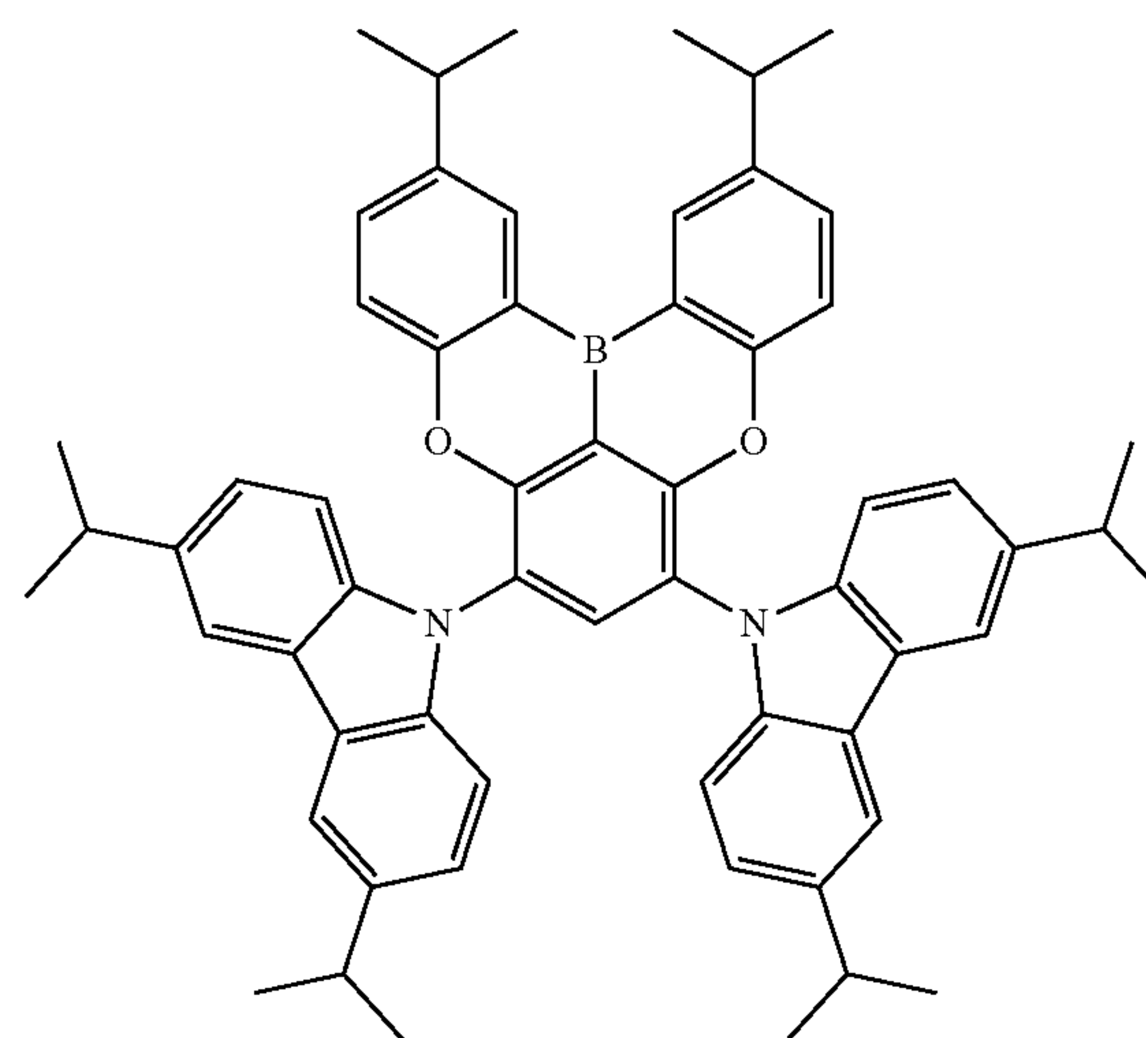
Dopant 231
