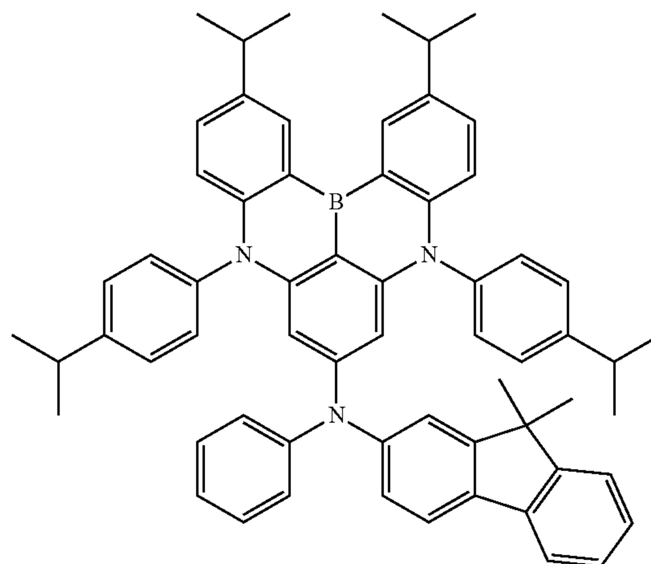
Dopant 120
