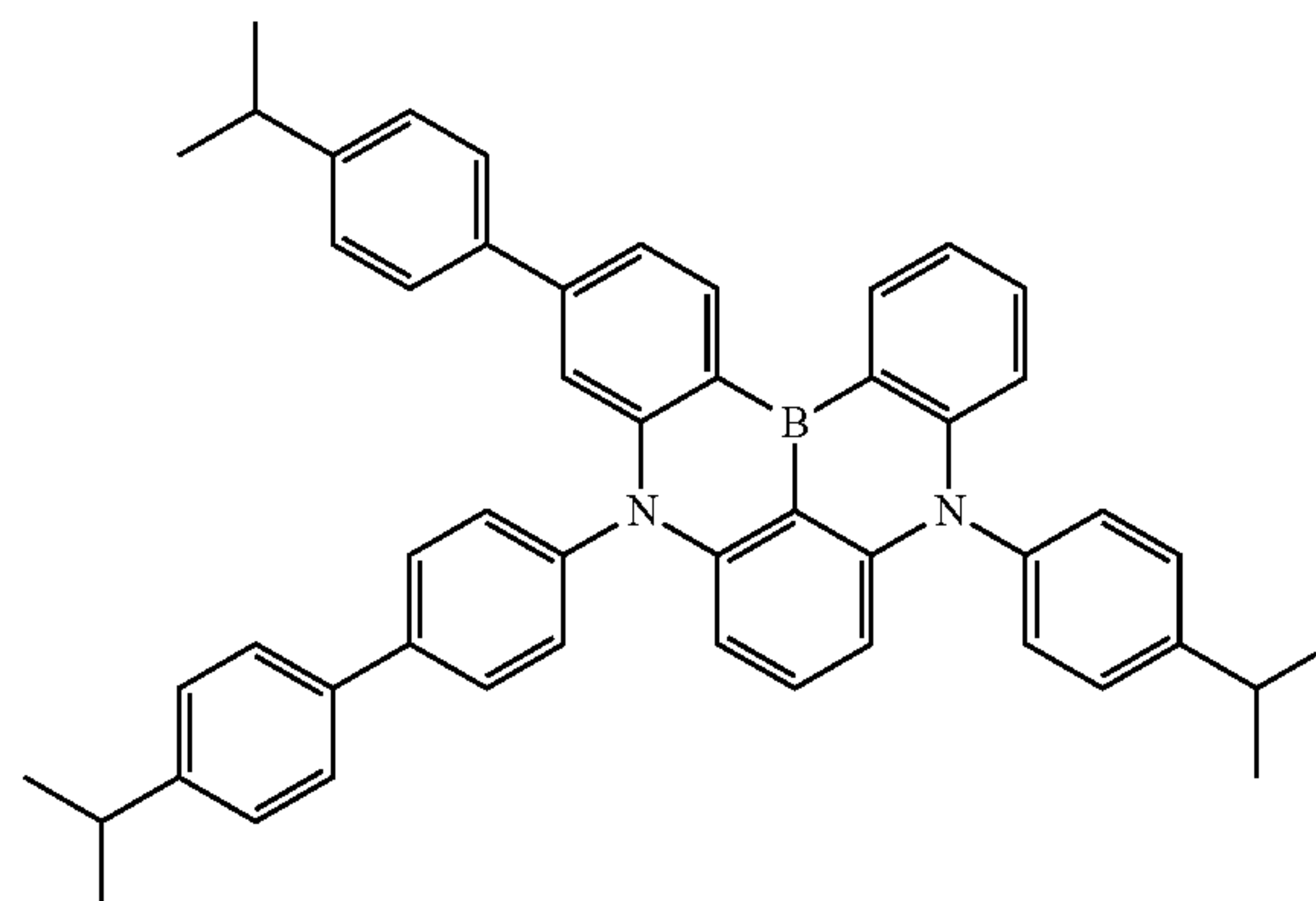
Dopant 29
