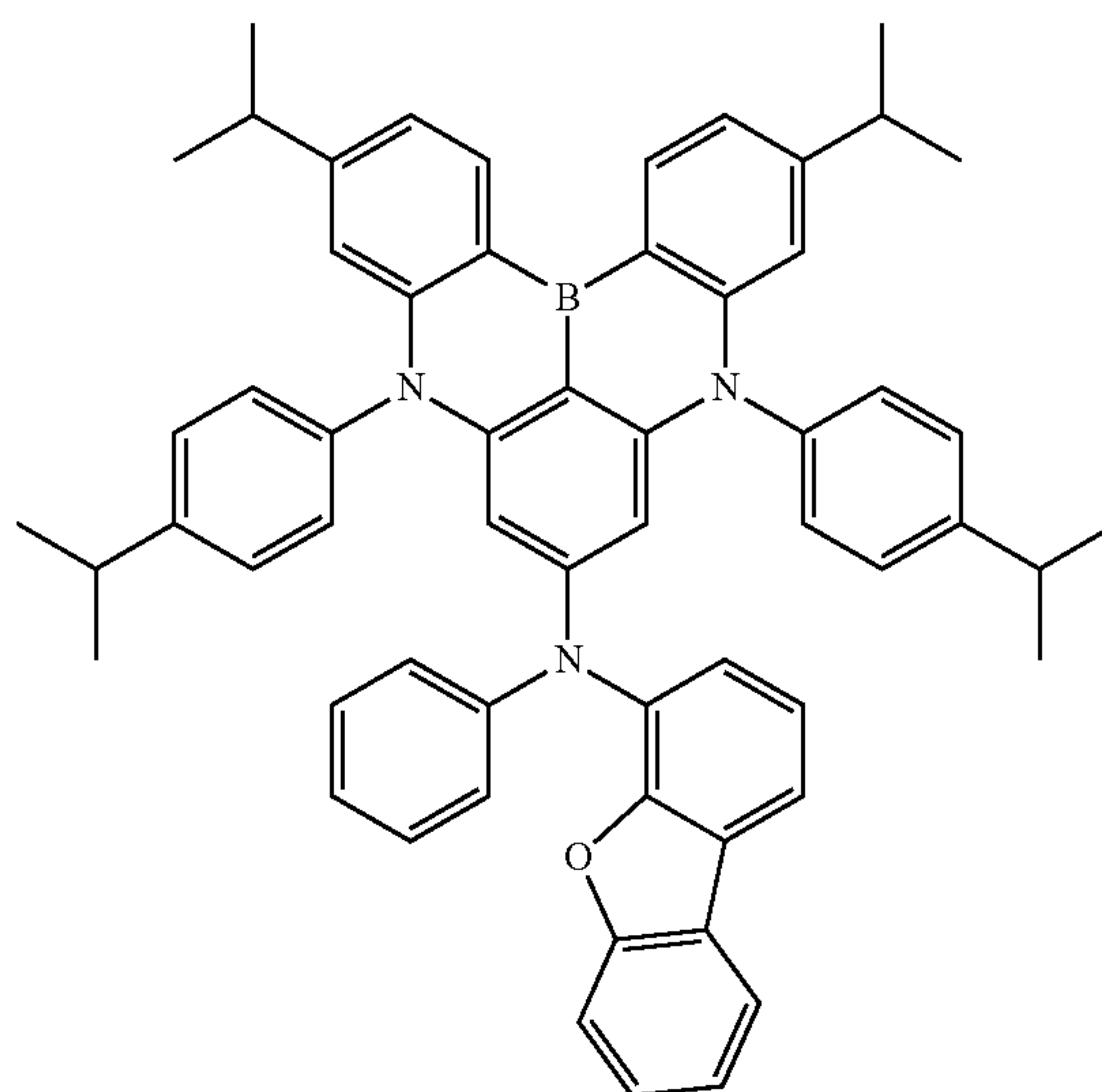
Dopant 118
