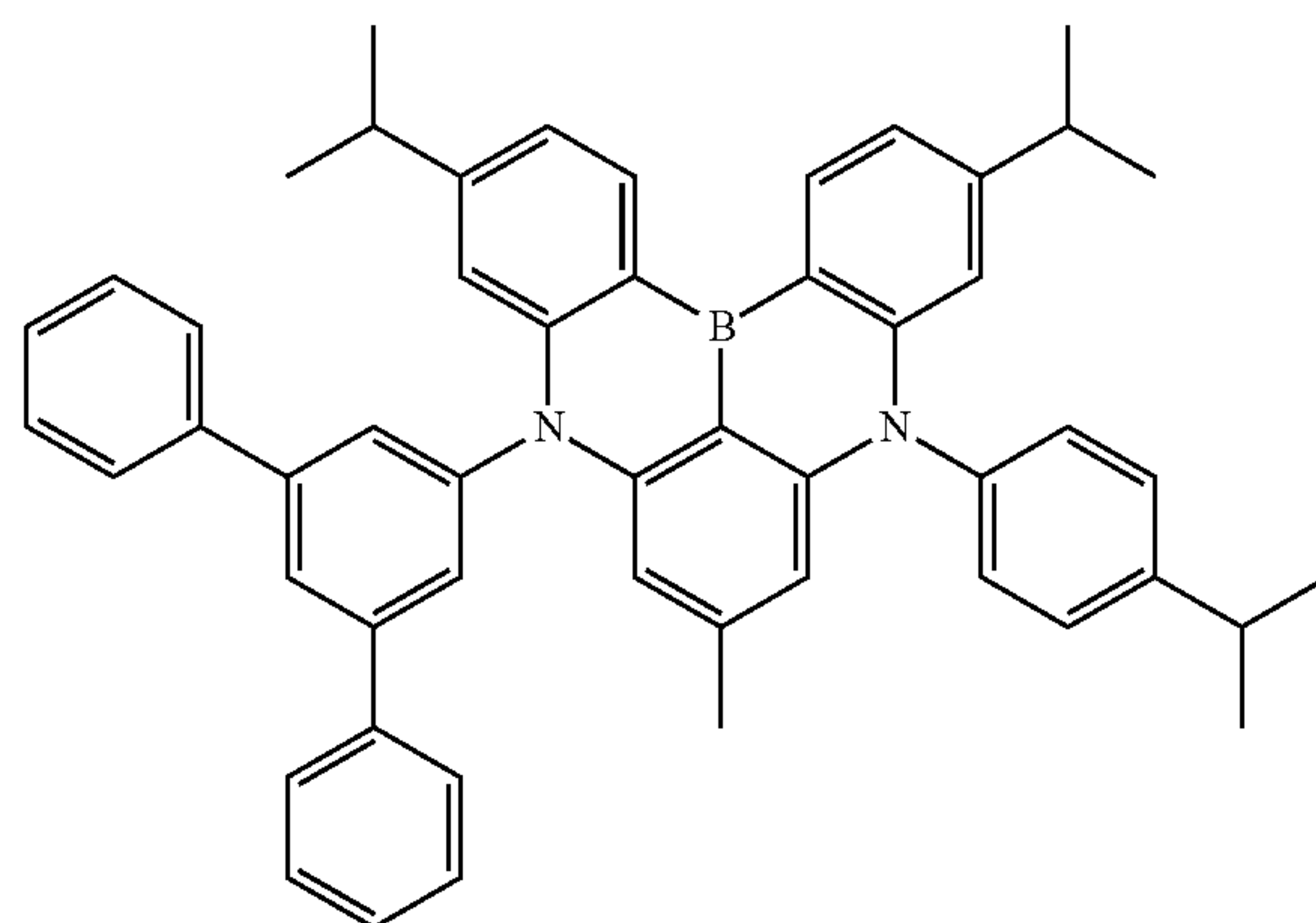
Dopant 152
