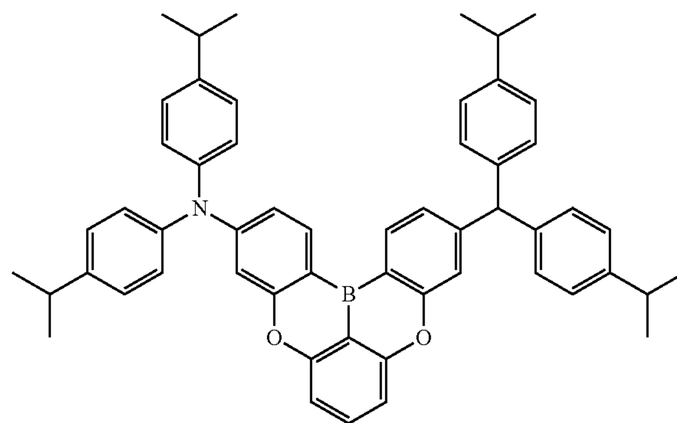
Dopant 197
