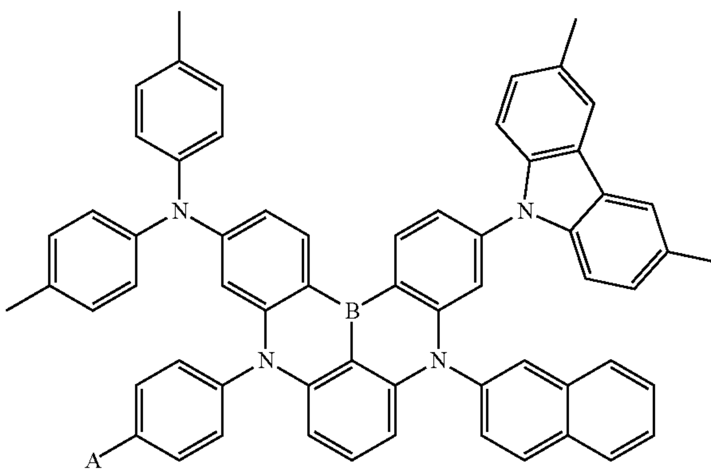
Dopant 112
