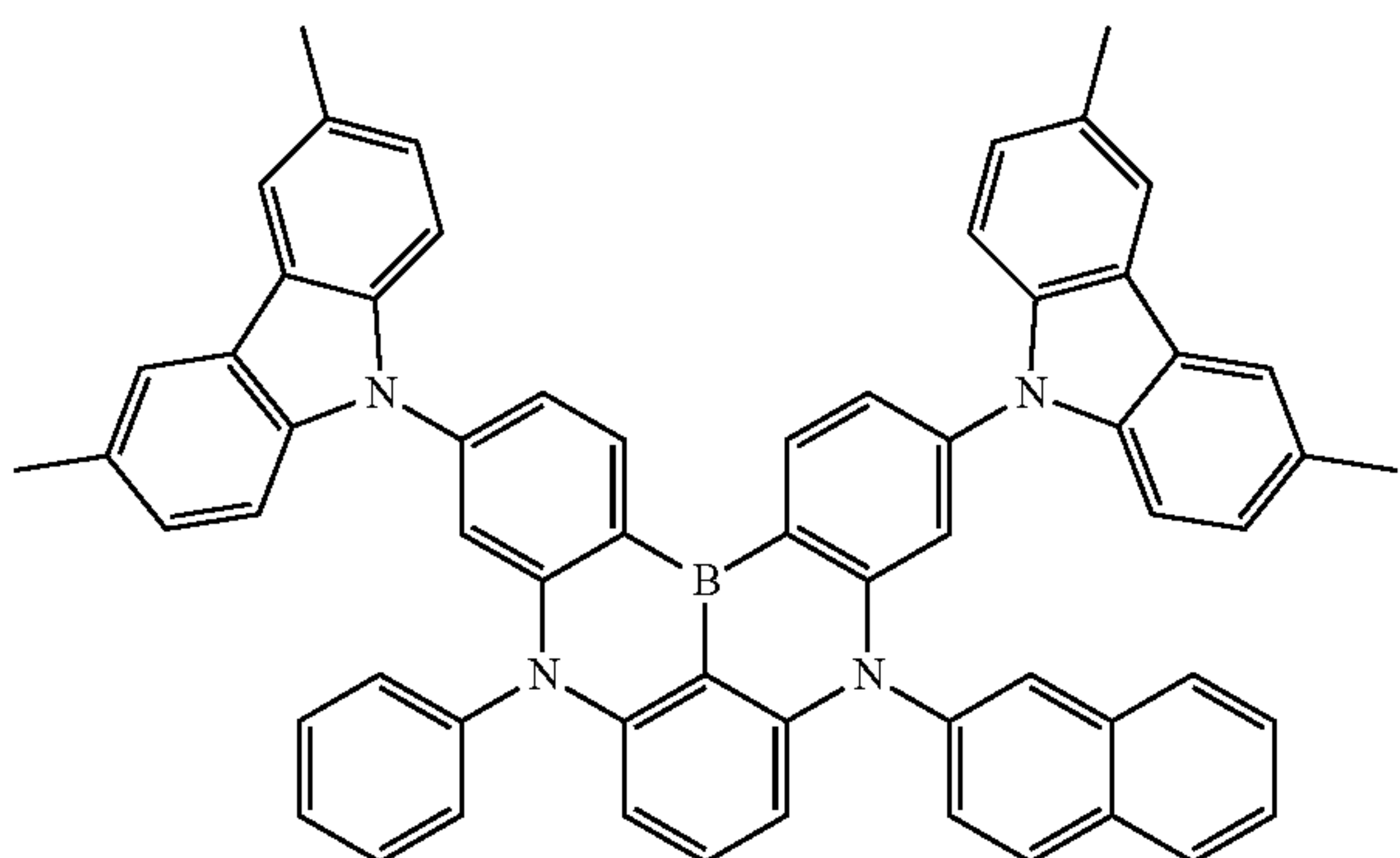
Dopant 108
