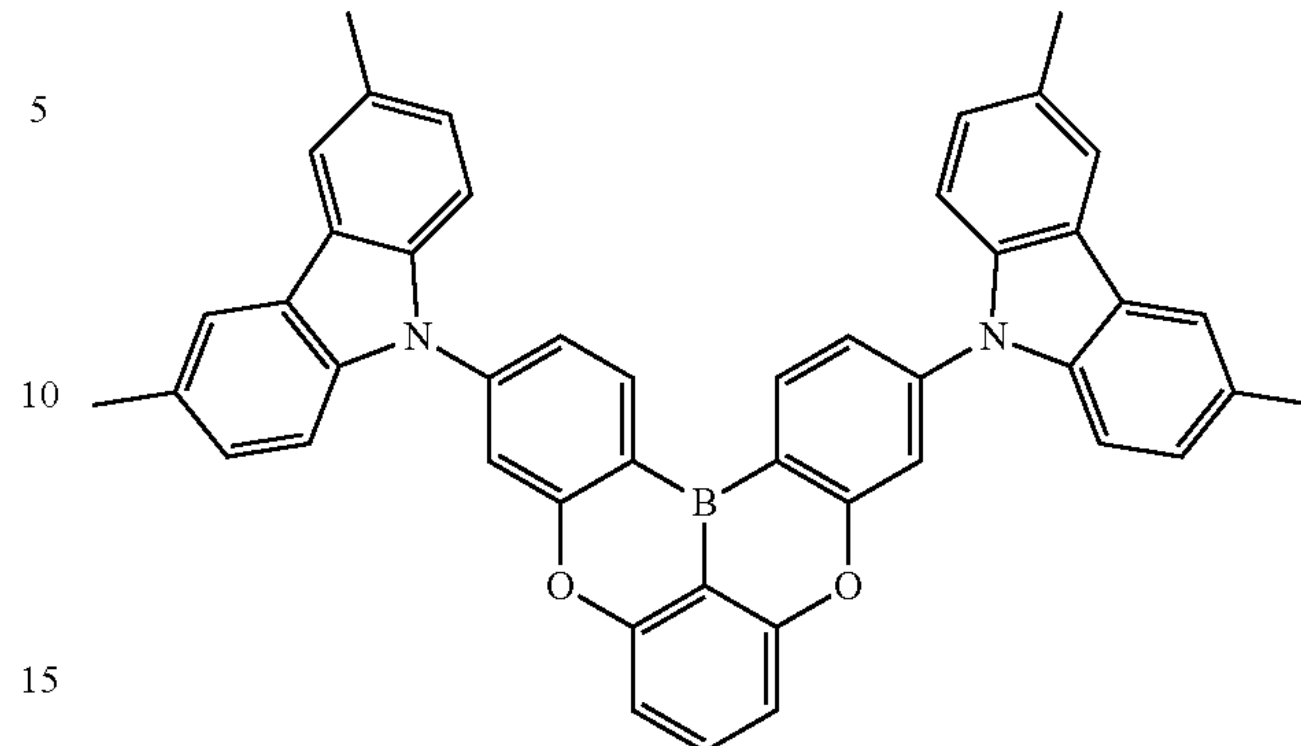
Dopant 194
