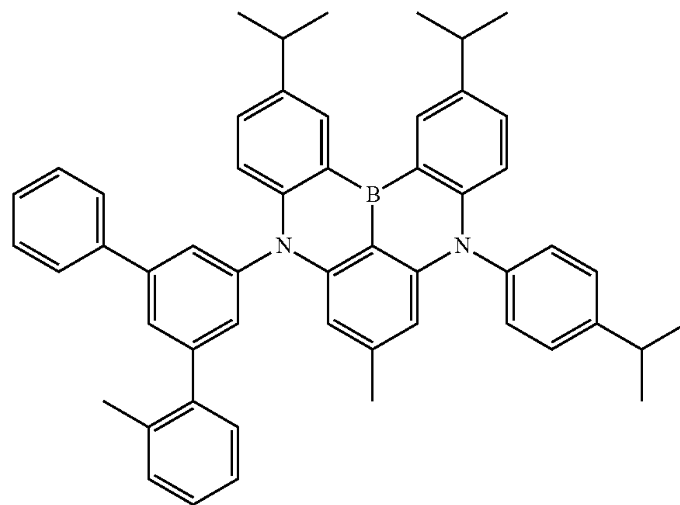
Dopant 154
