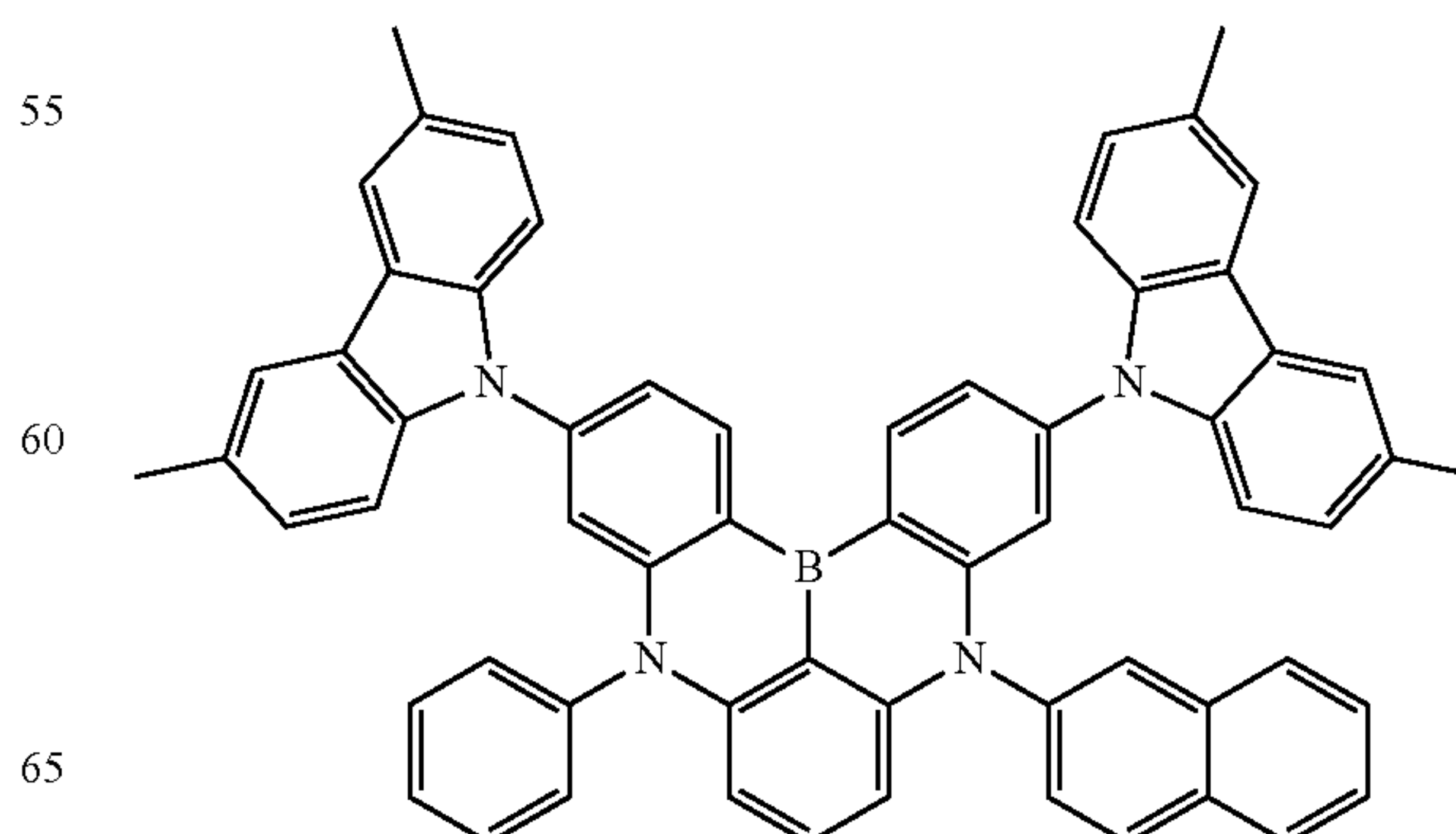
Dopant 108
