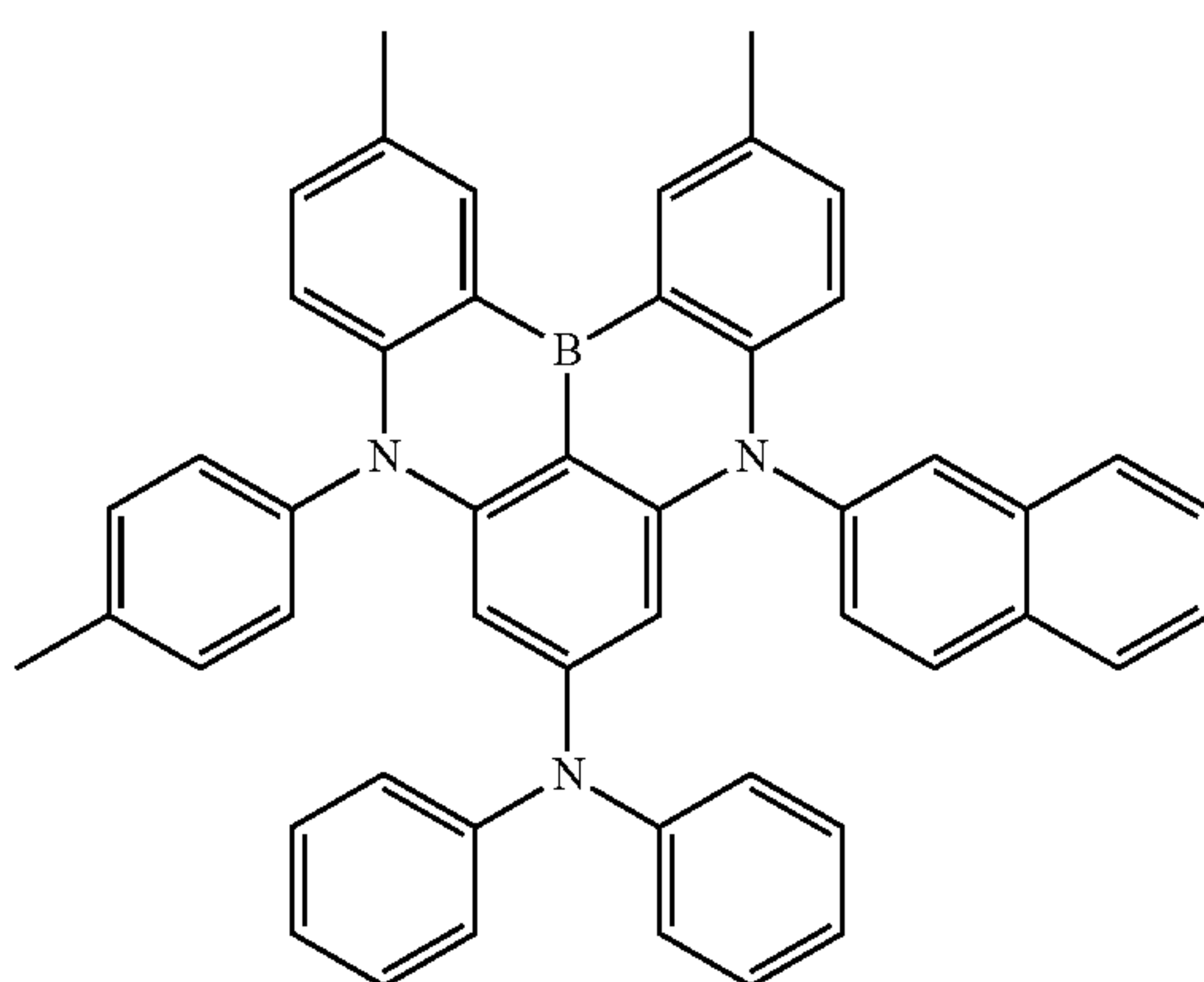
Dopant 83
