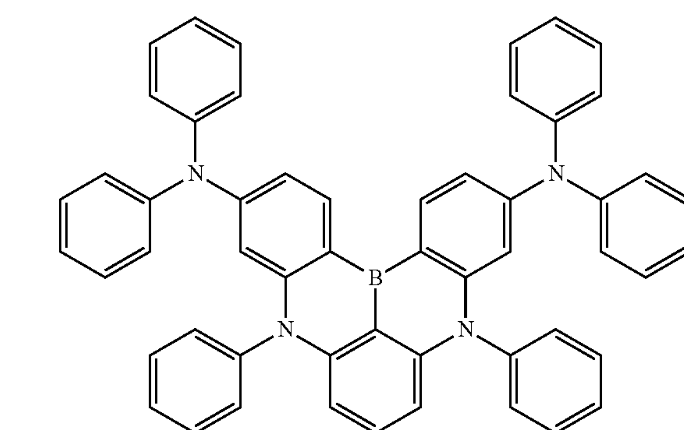
Dopant 57
