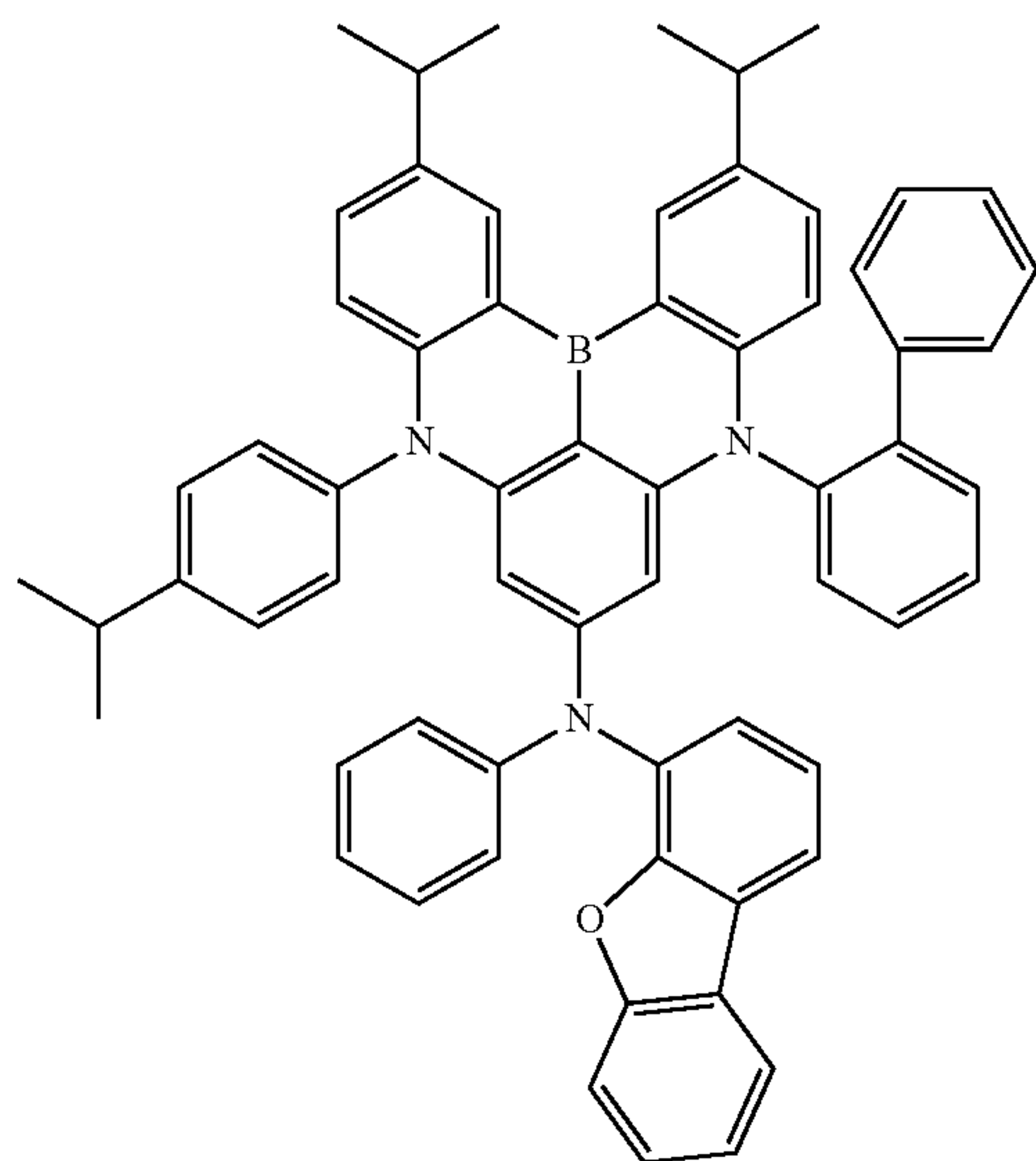
Dopant 118
