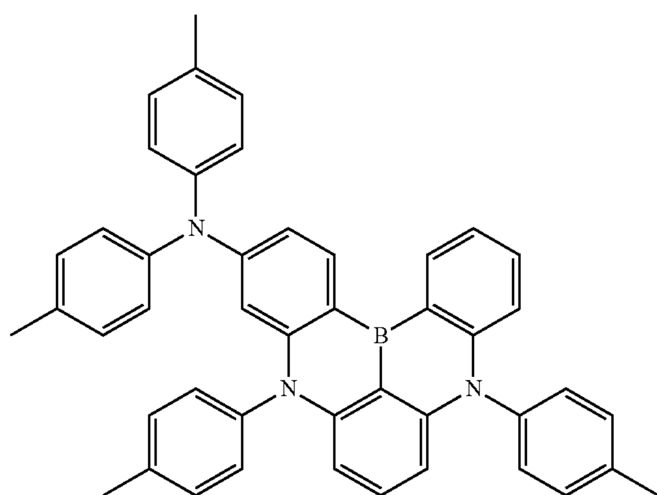
Dopant 53
