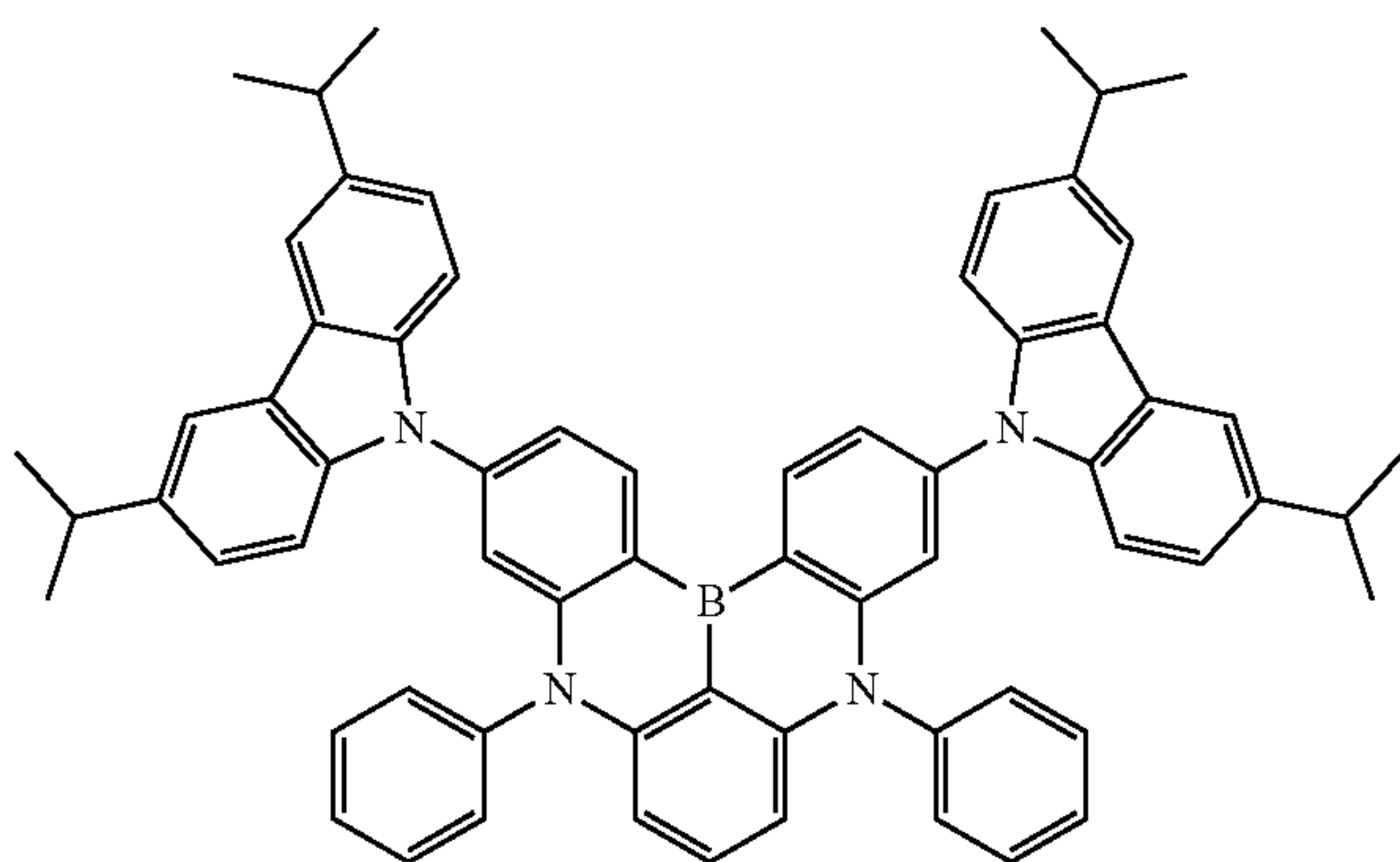
Dopant 75
