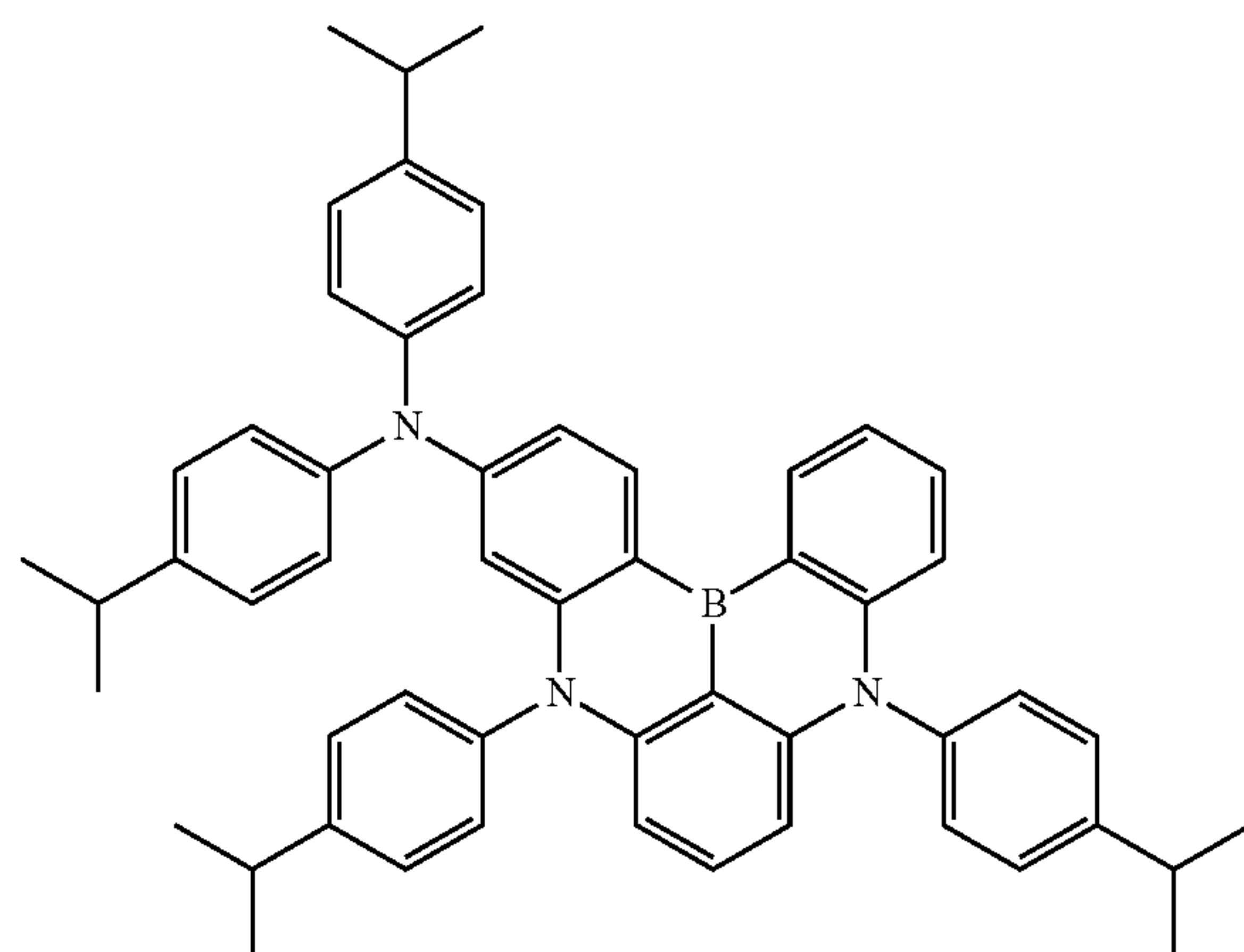
Dopant 55
