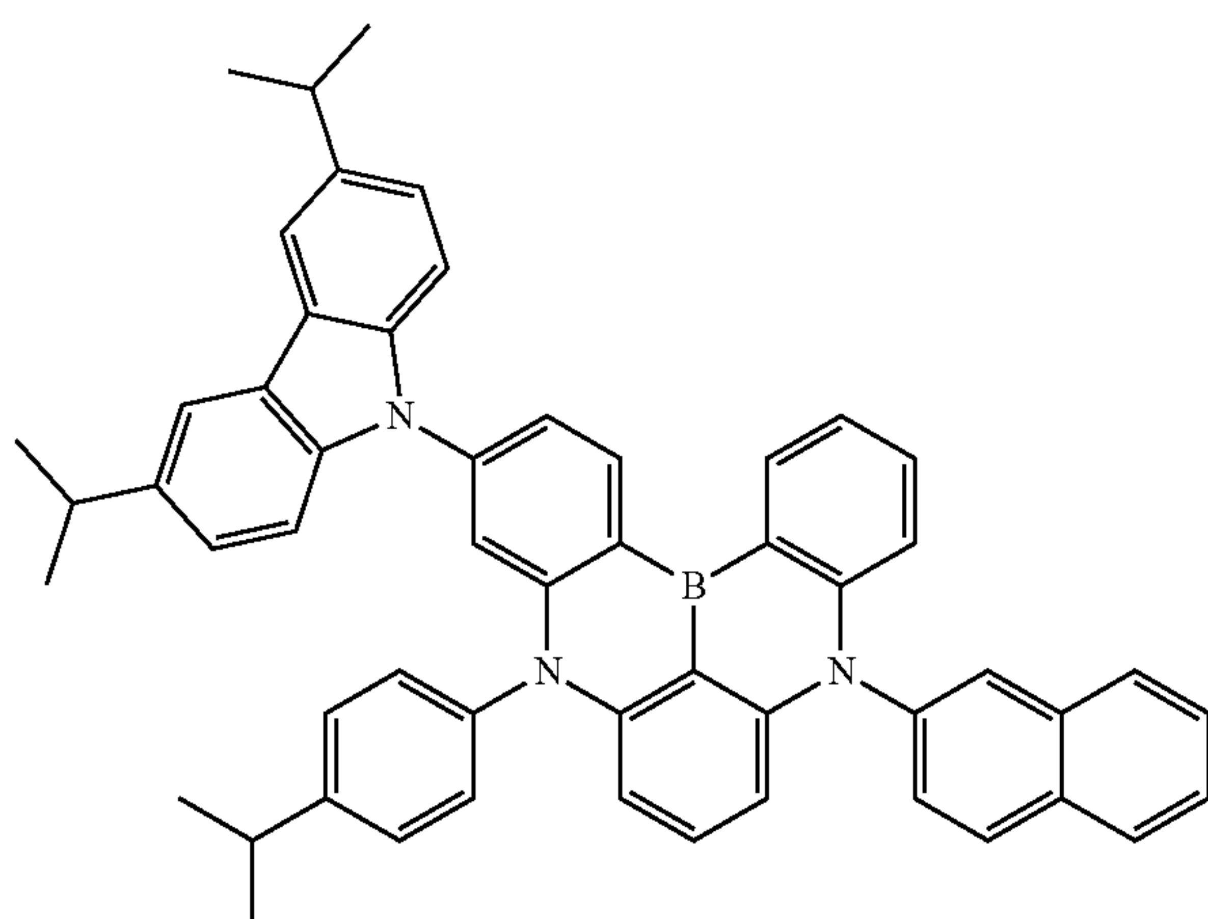
Dopant 104
