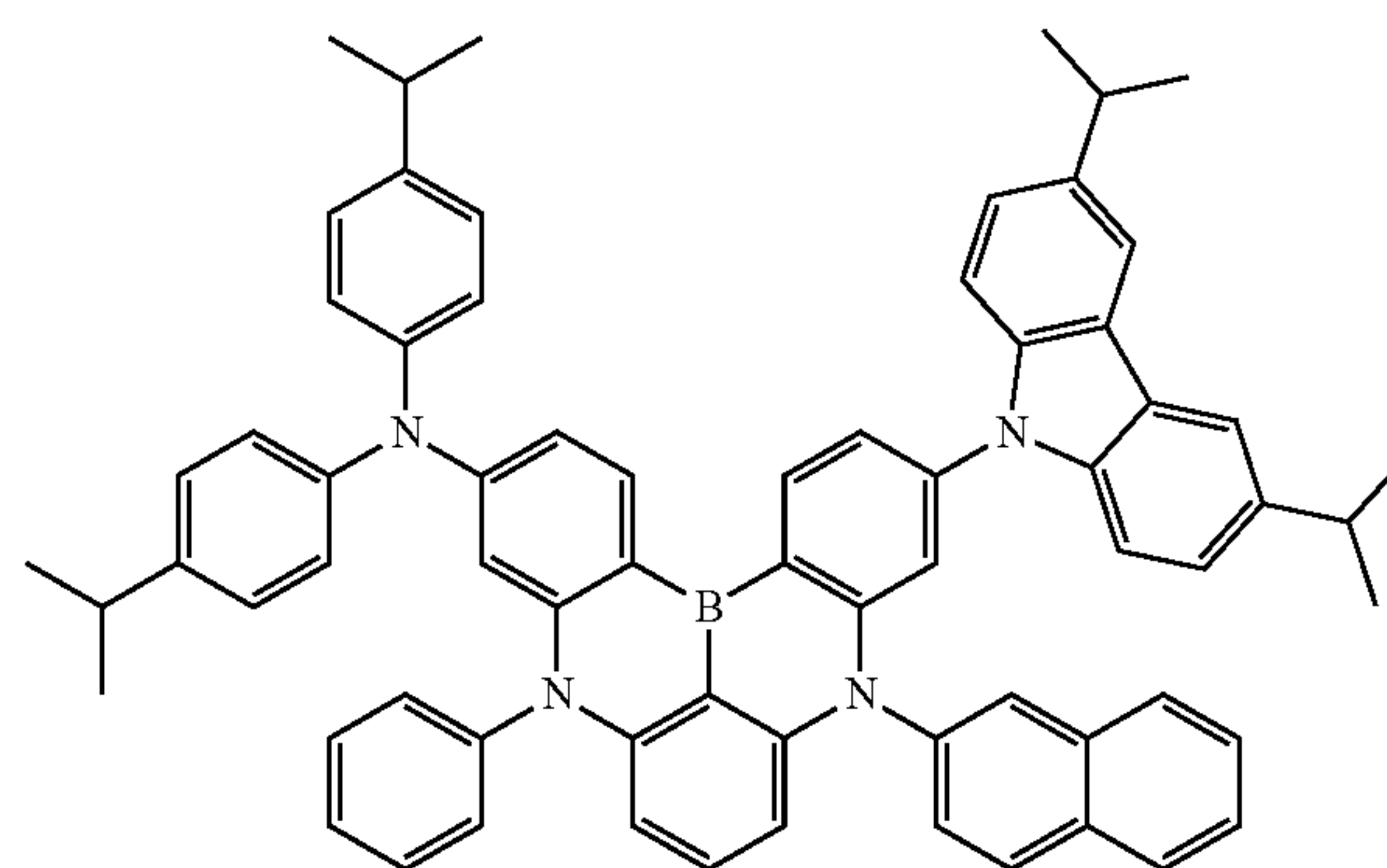
Dopant 115
