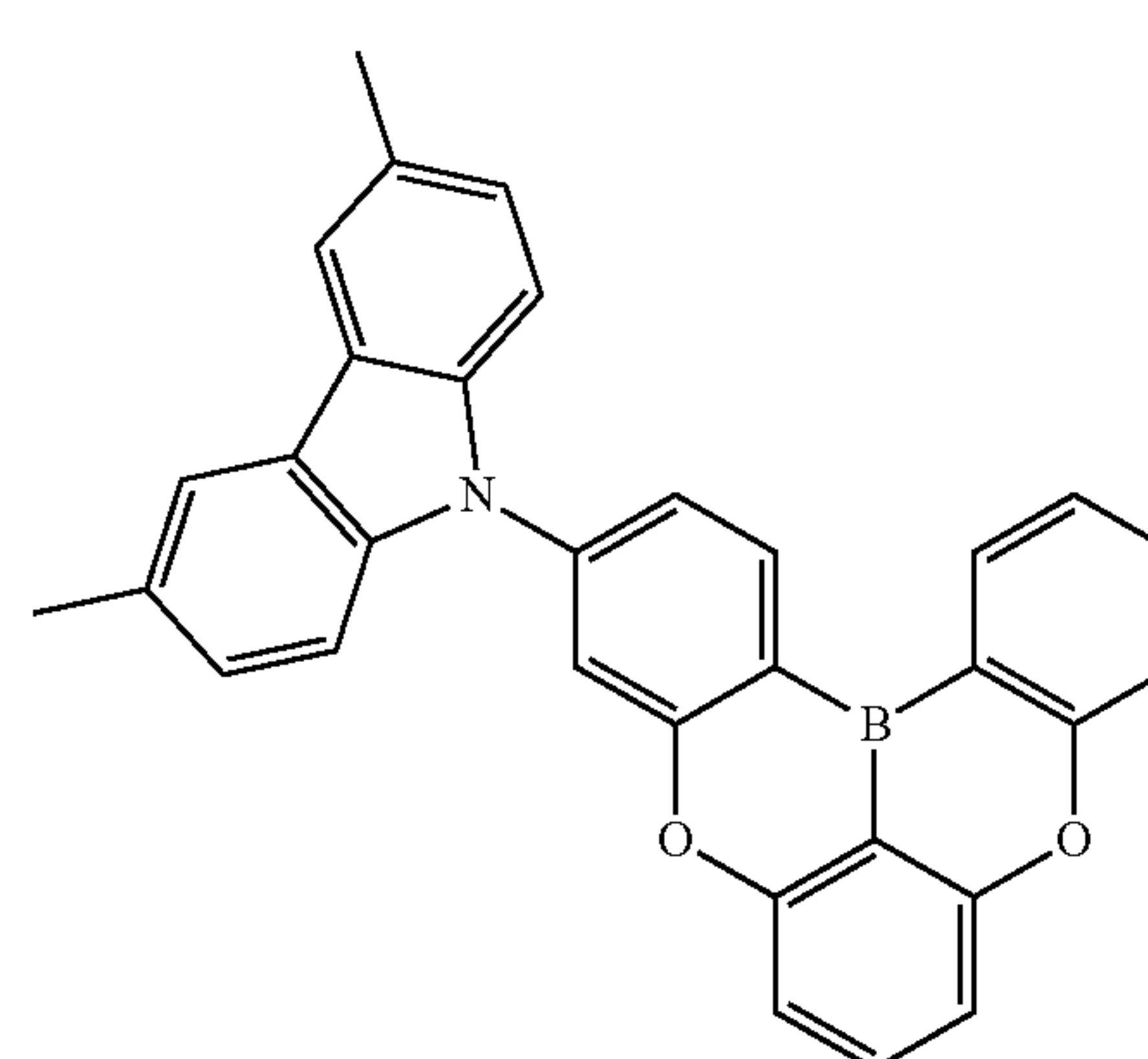
Dopant 192
