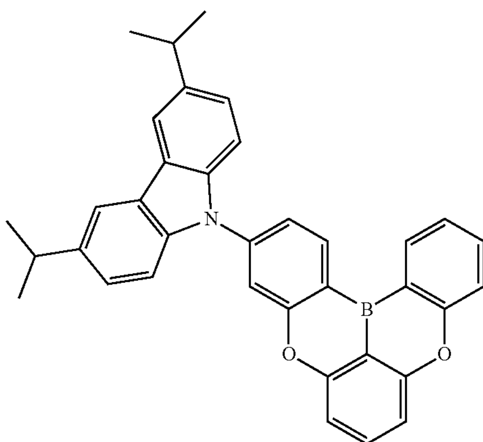
Dopant 199
