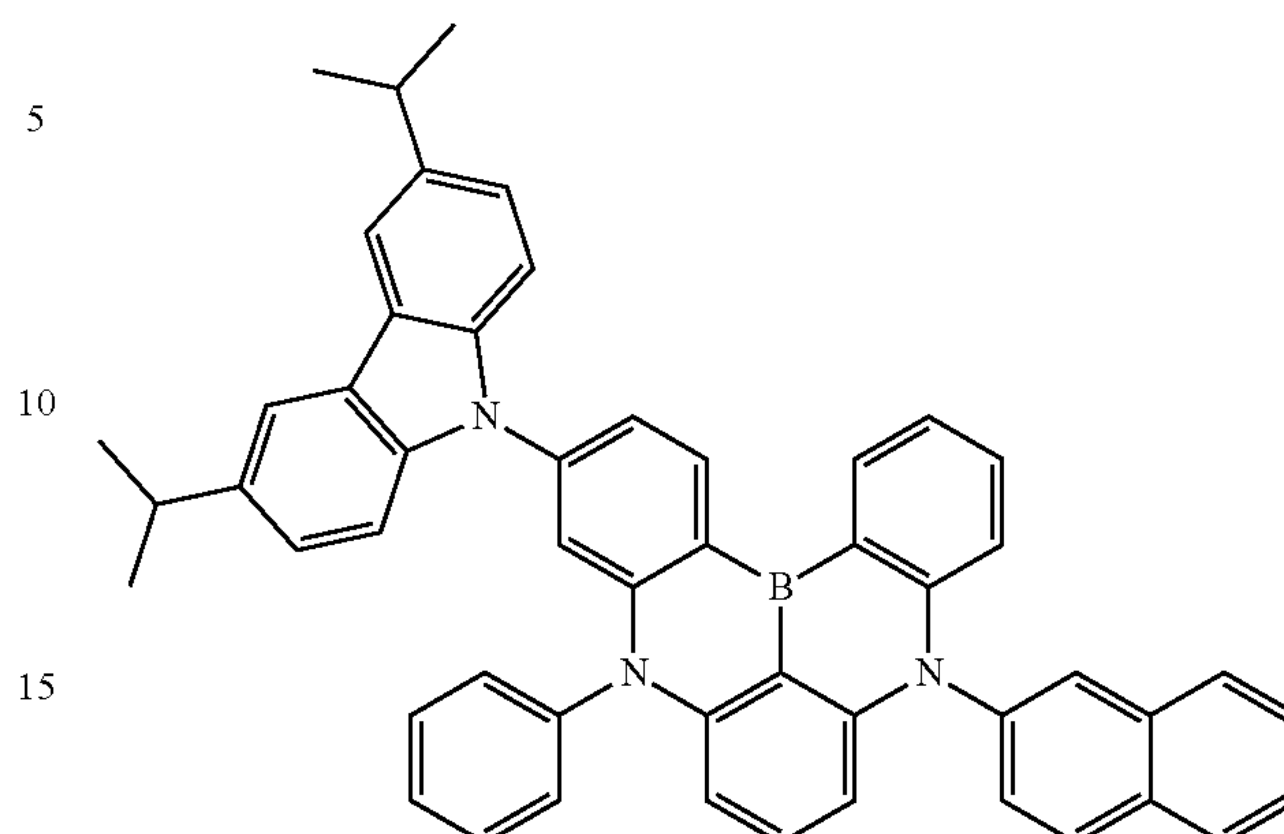
Dopant 105
