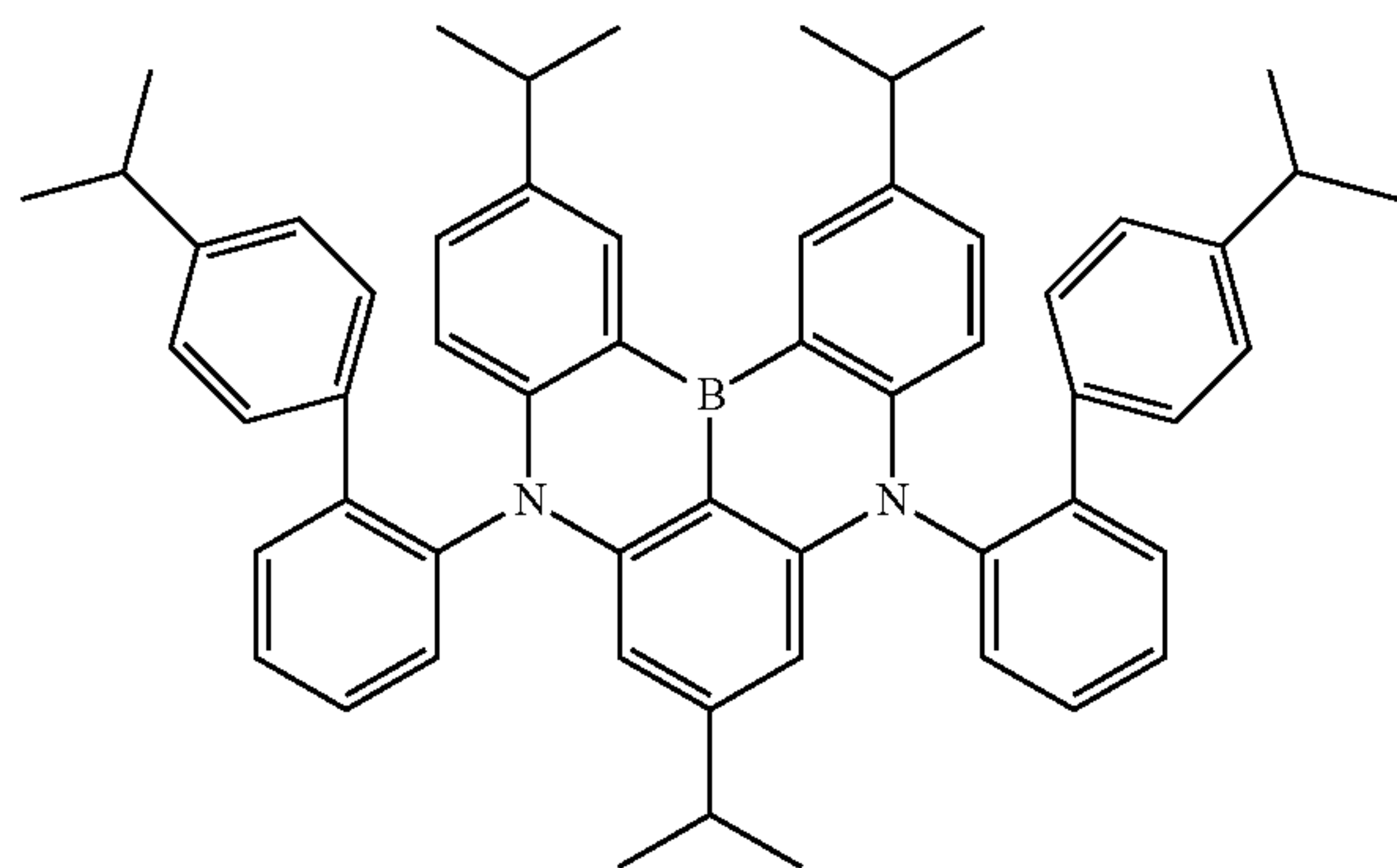
Dopant 148
