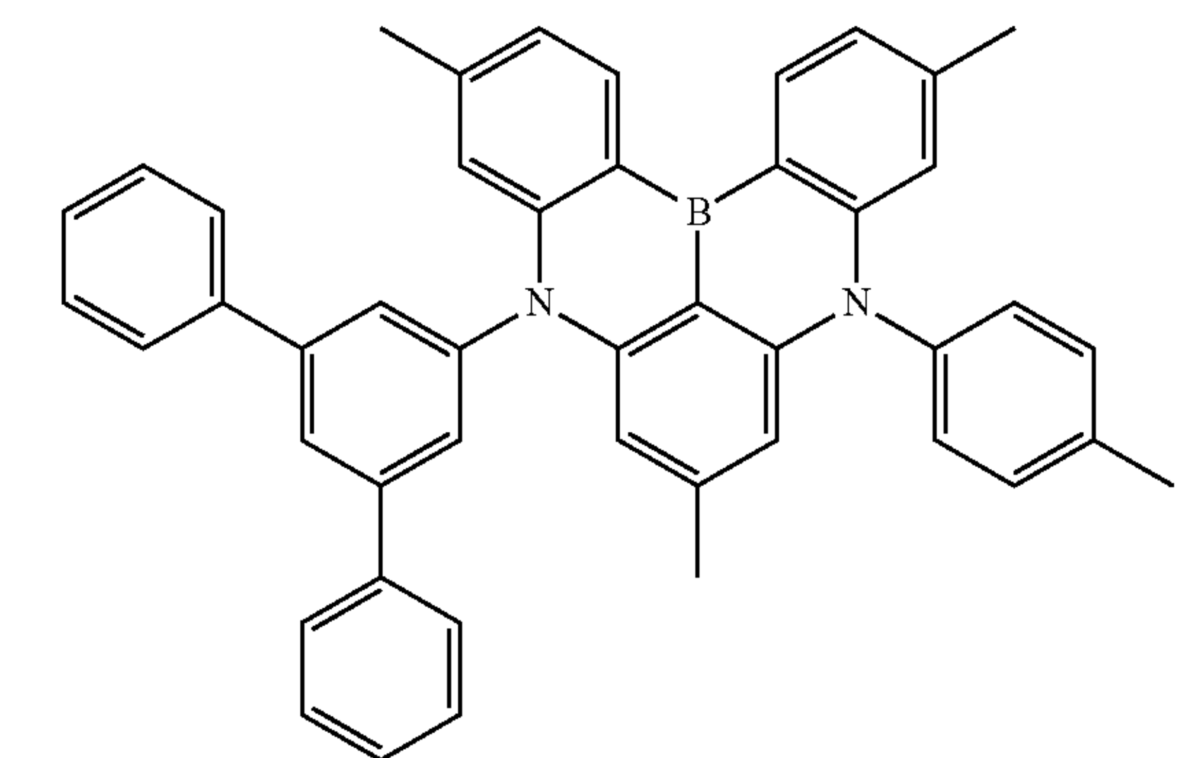
Dopant 153
