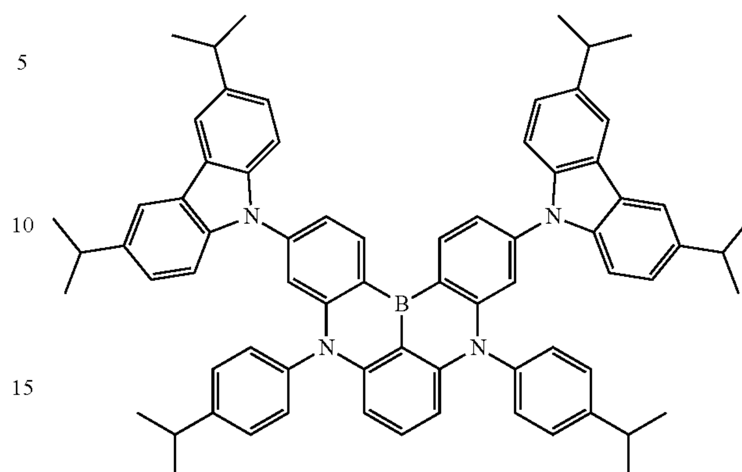
Dopant 74
