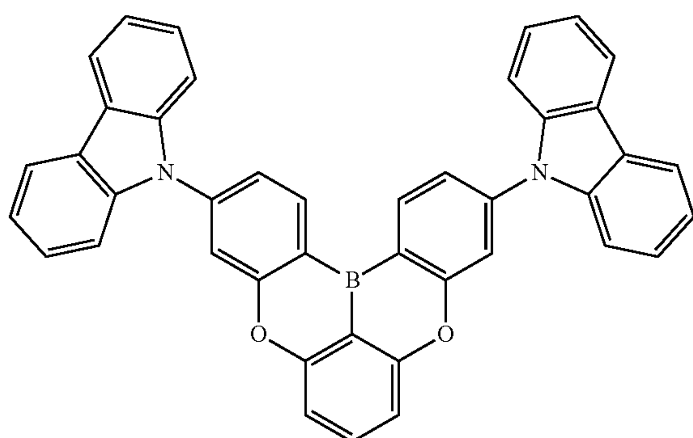
Dopant 186
