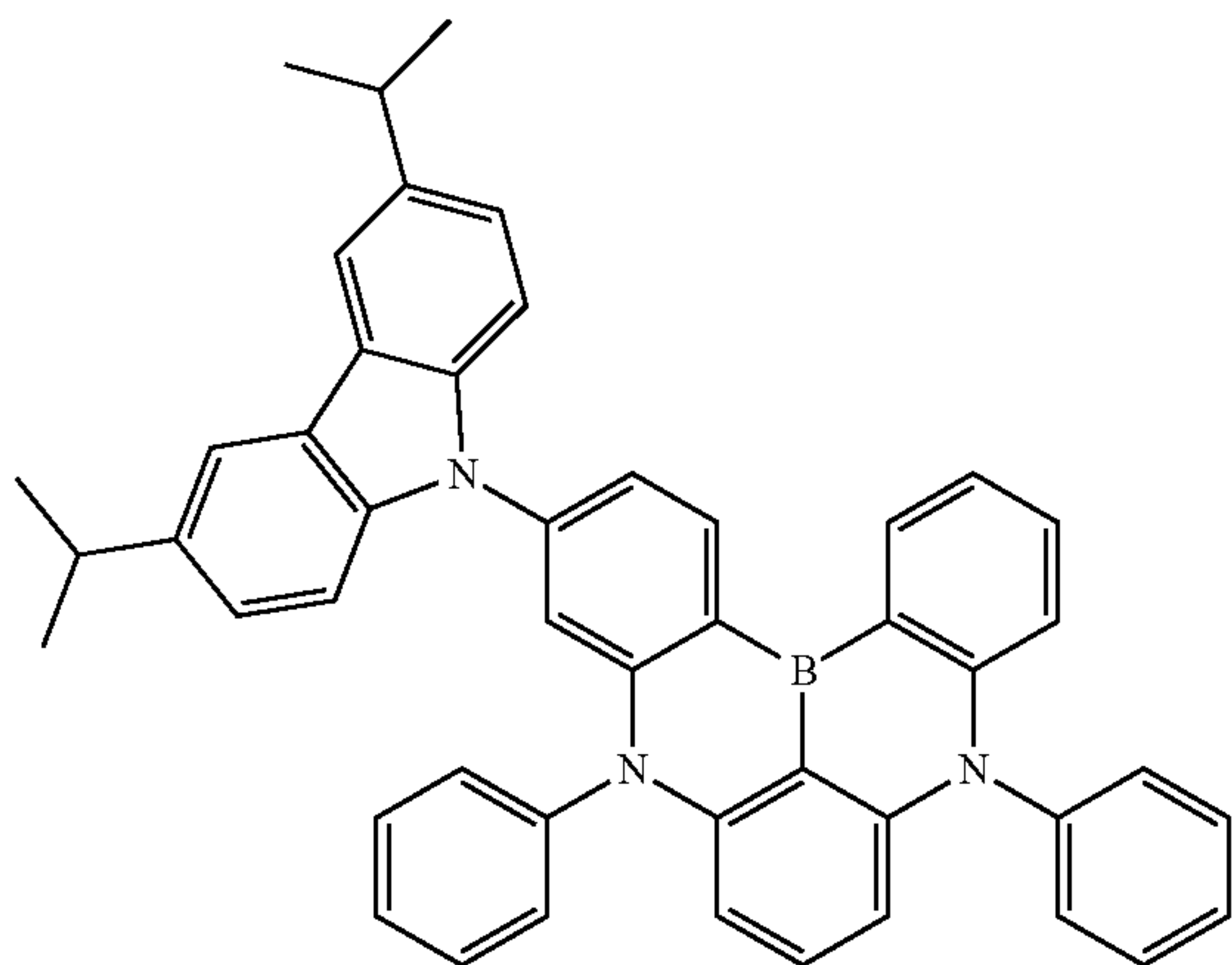
Dopant 70
