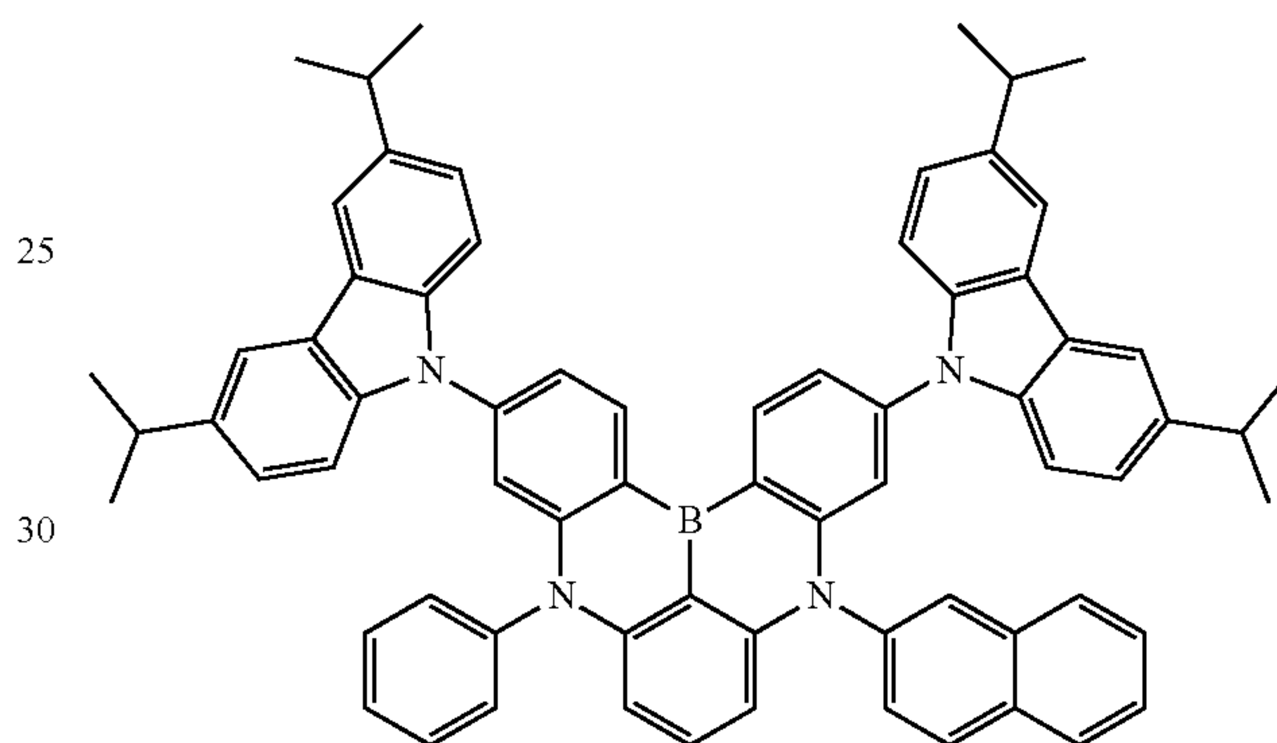
Dopant 110
