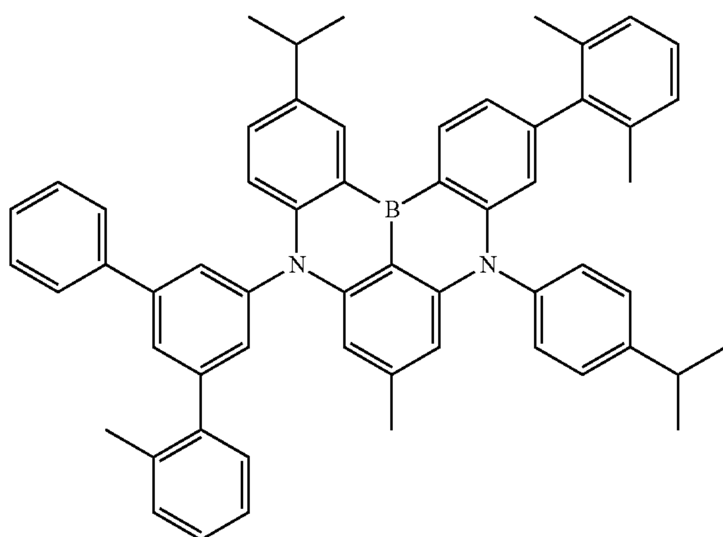
Dopant 162
