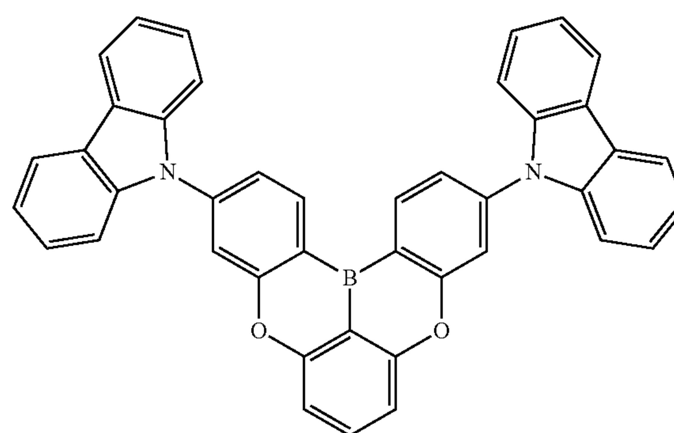
Dopant 186
