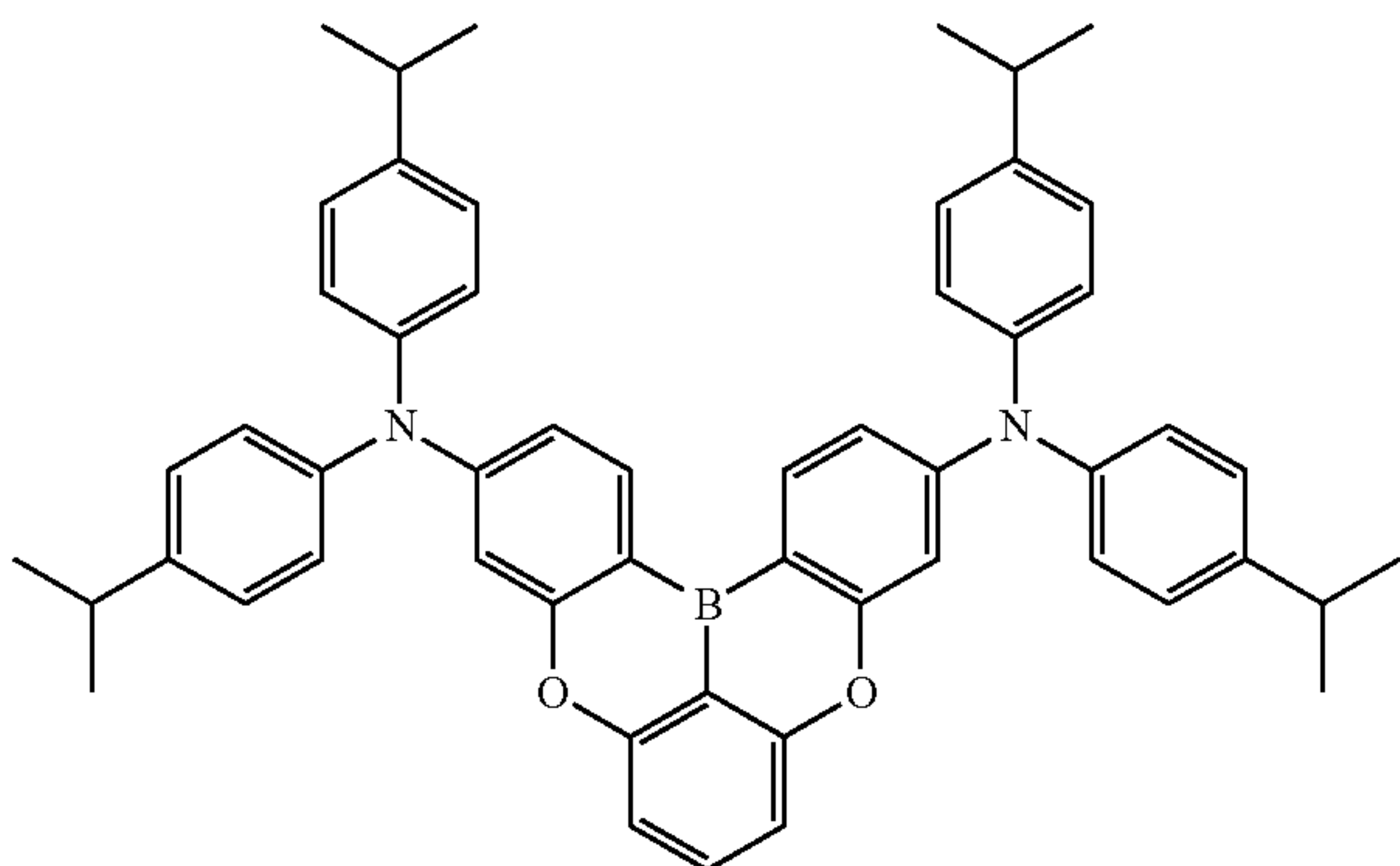
Dopant 197
