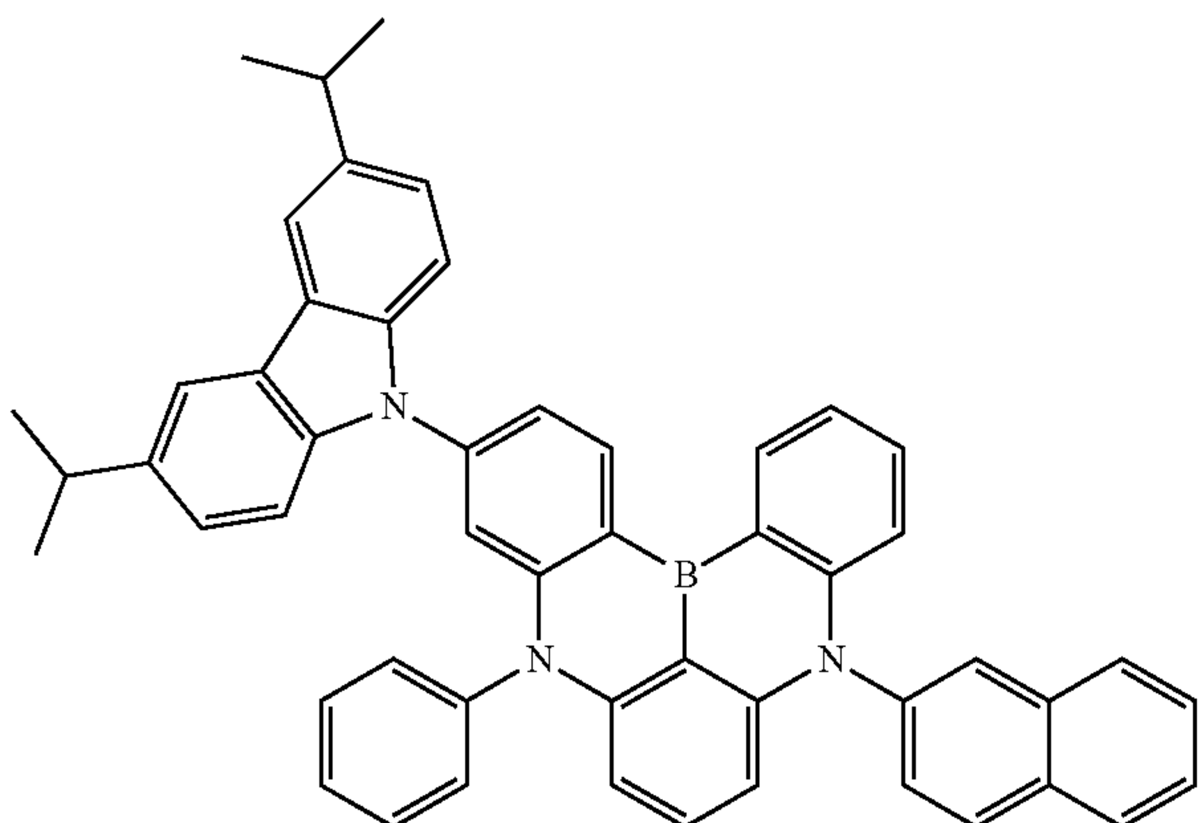
Dopant 105
