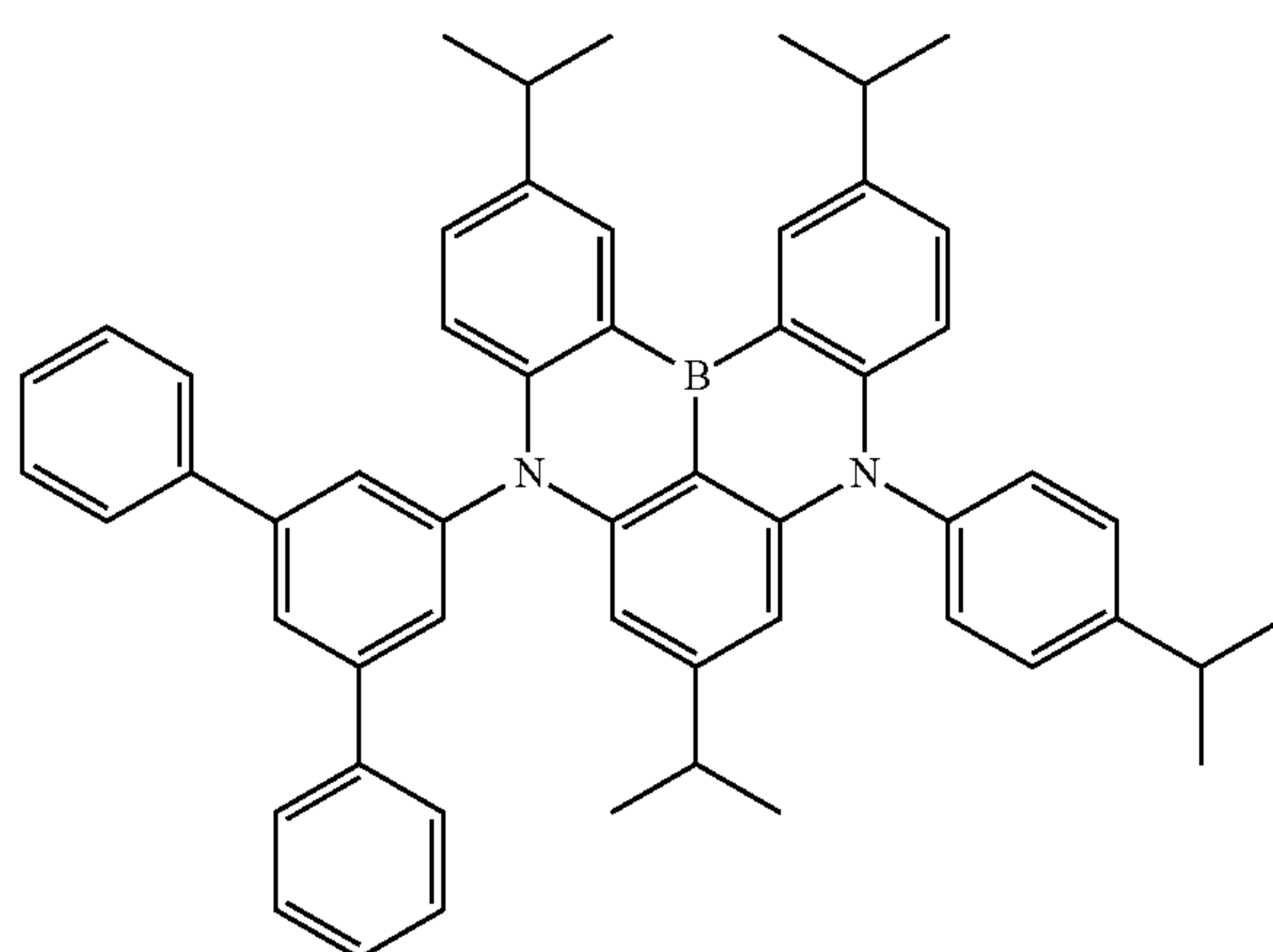
Dopant 150
