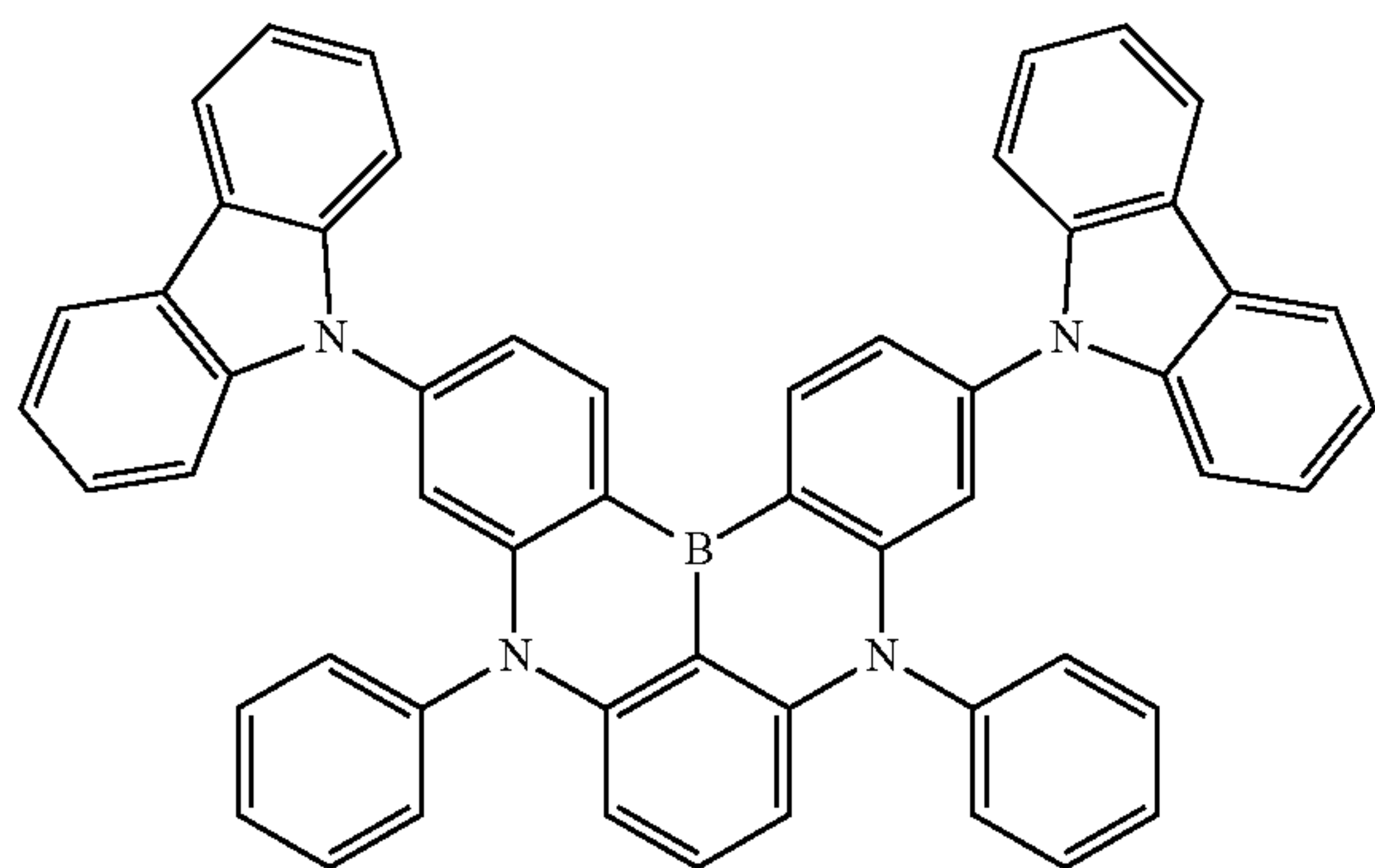
Dopant 71
