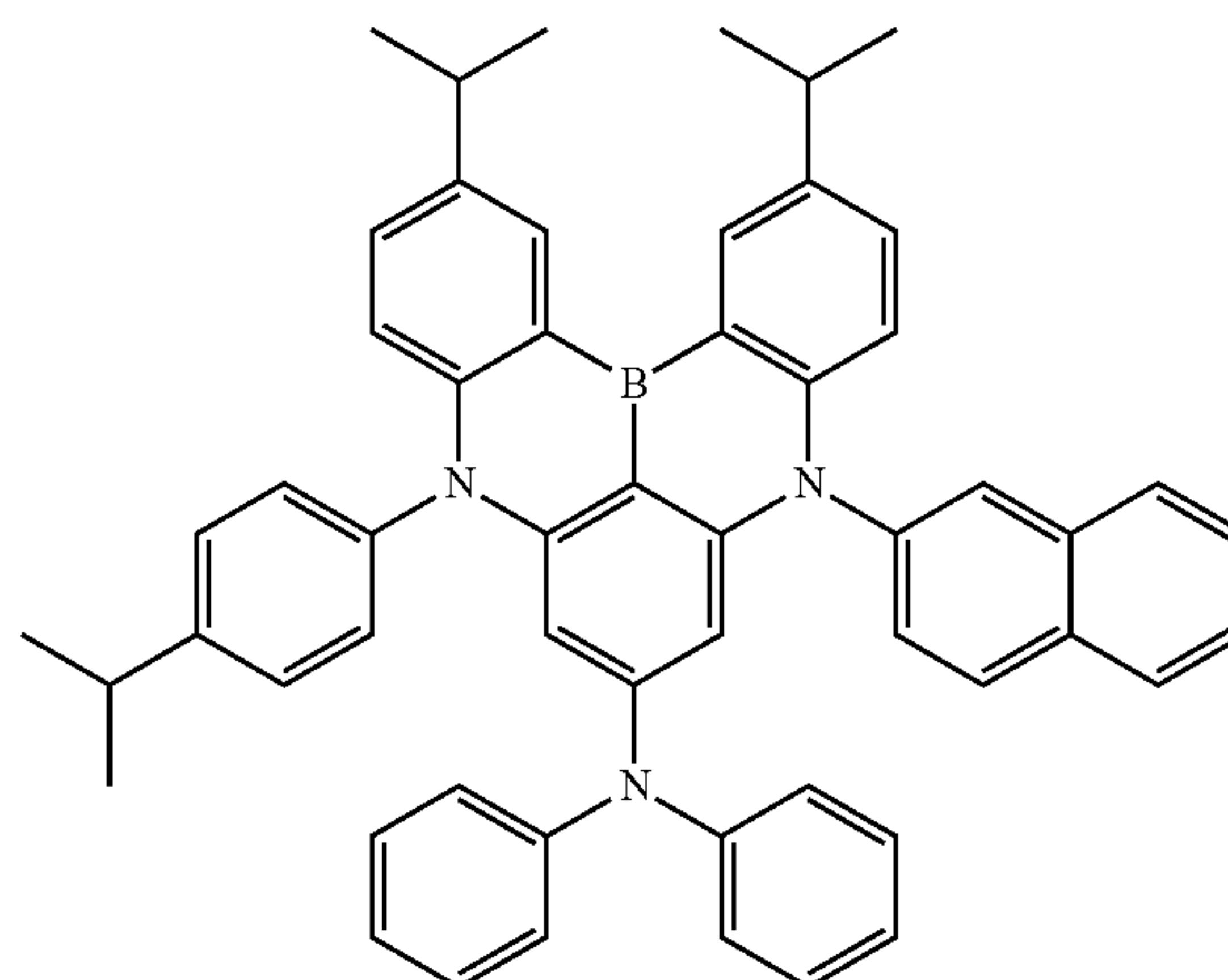
Dopant 85
