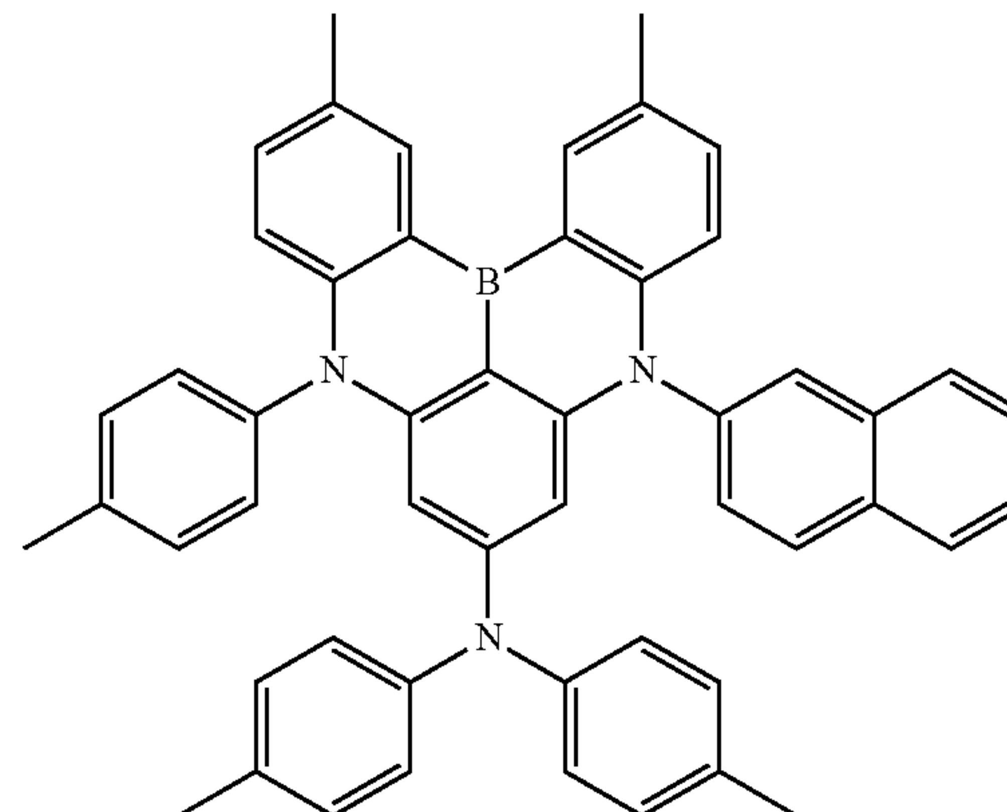
Dopant 82
