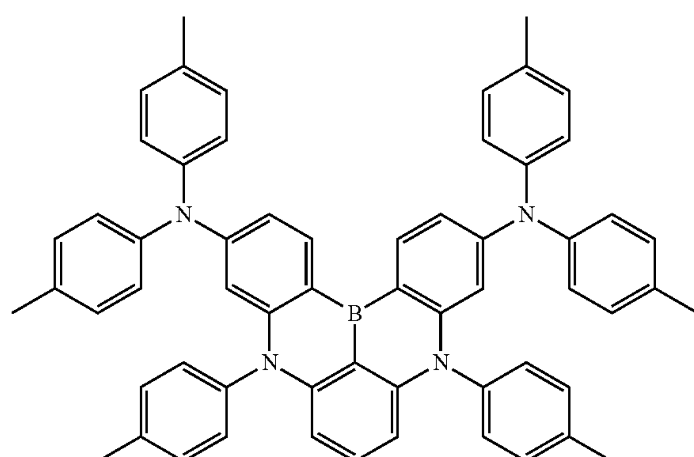
Dopant 57
