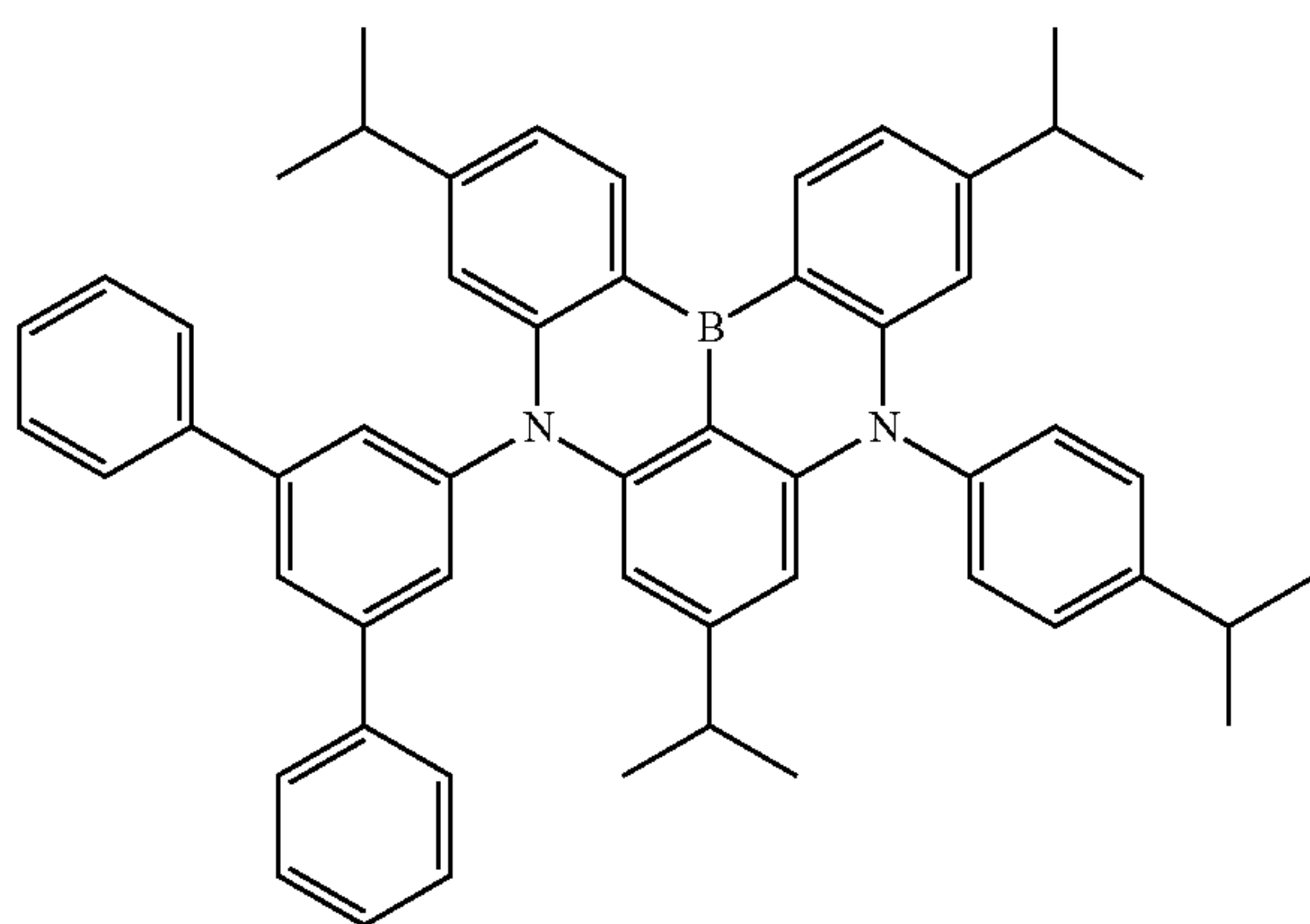
Dopant 151
