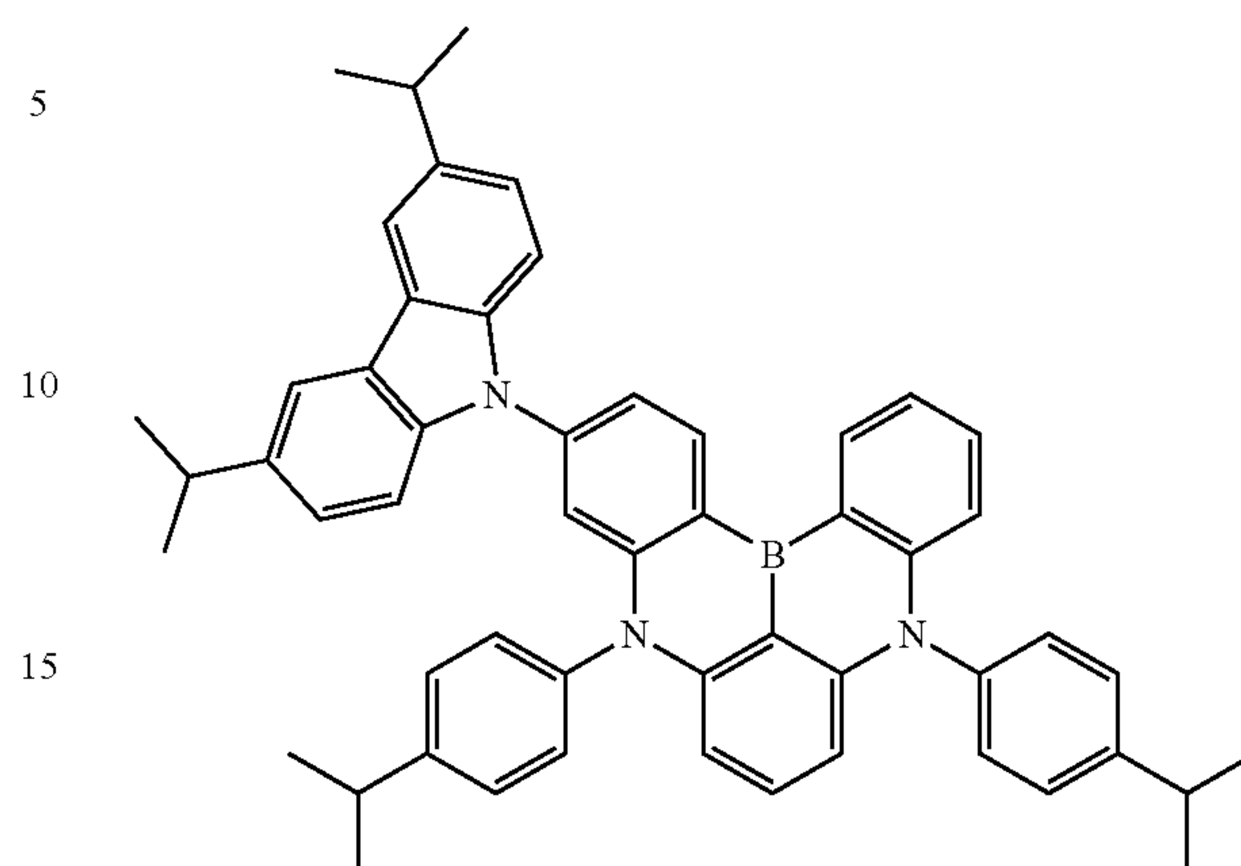
Dopant 70
