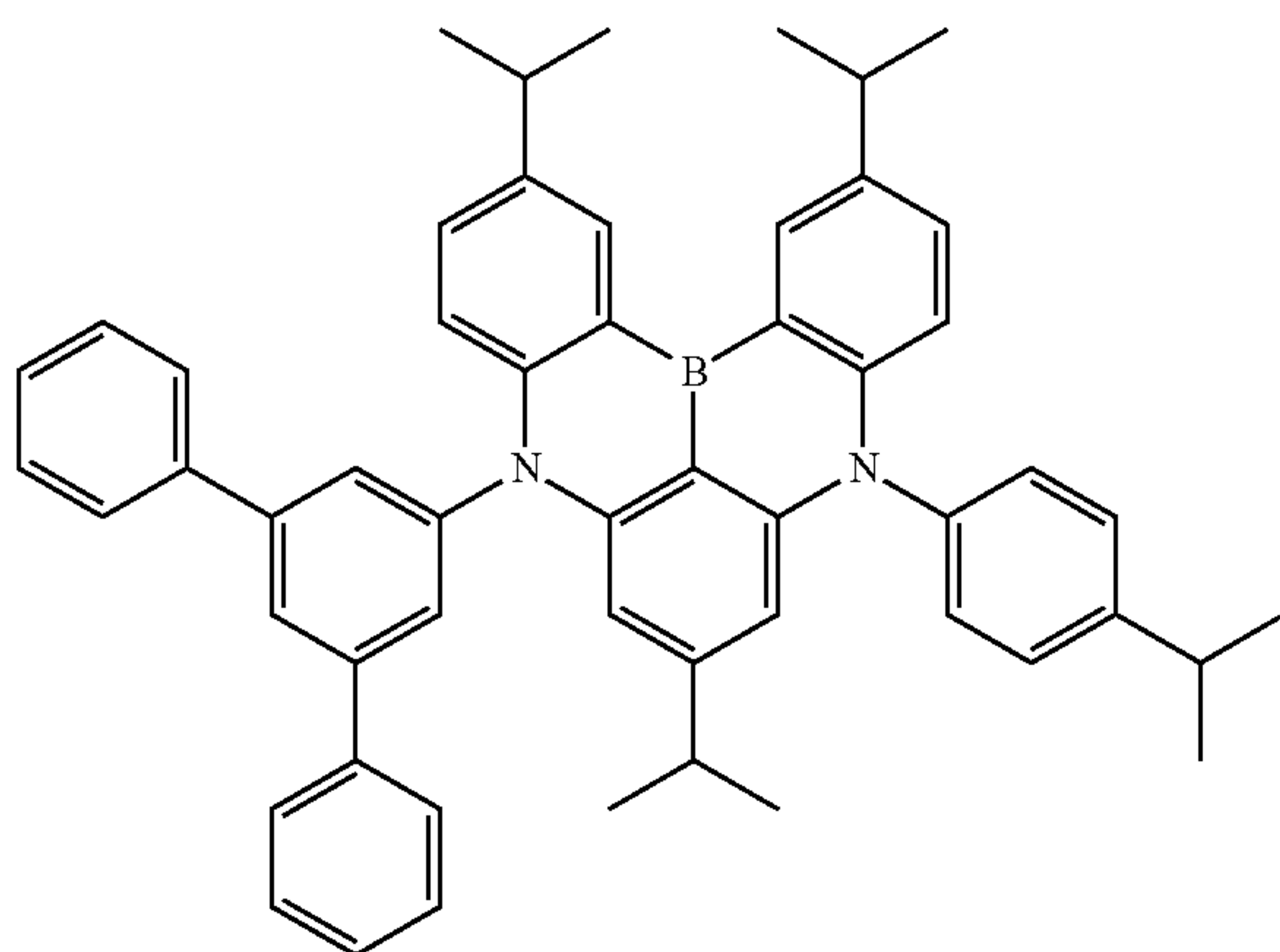
Dopant 150
