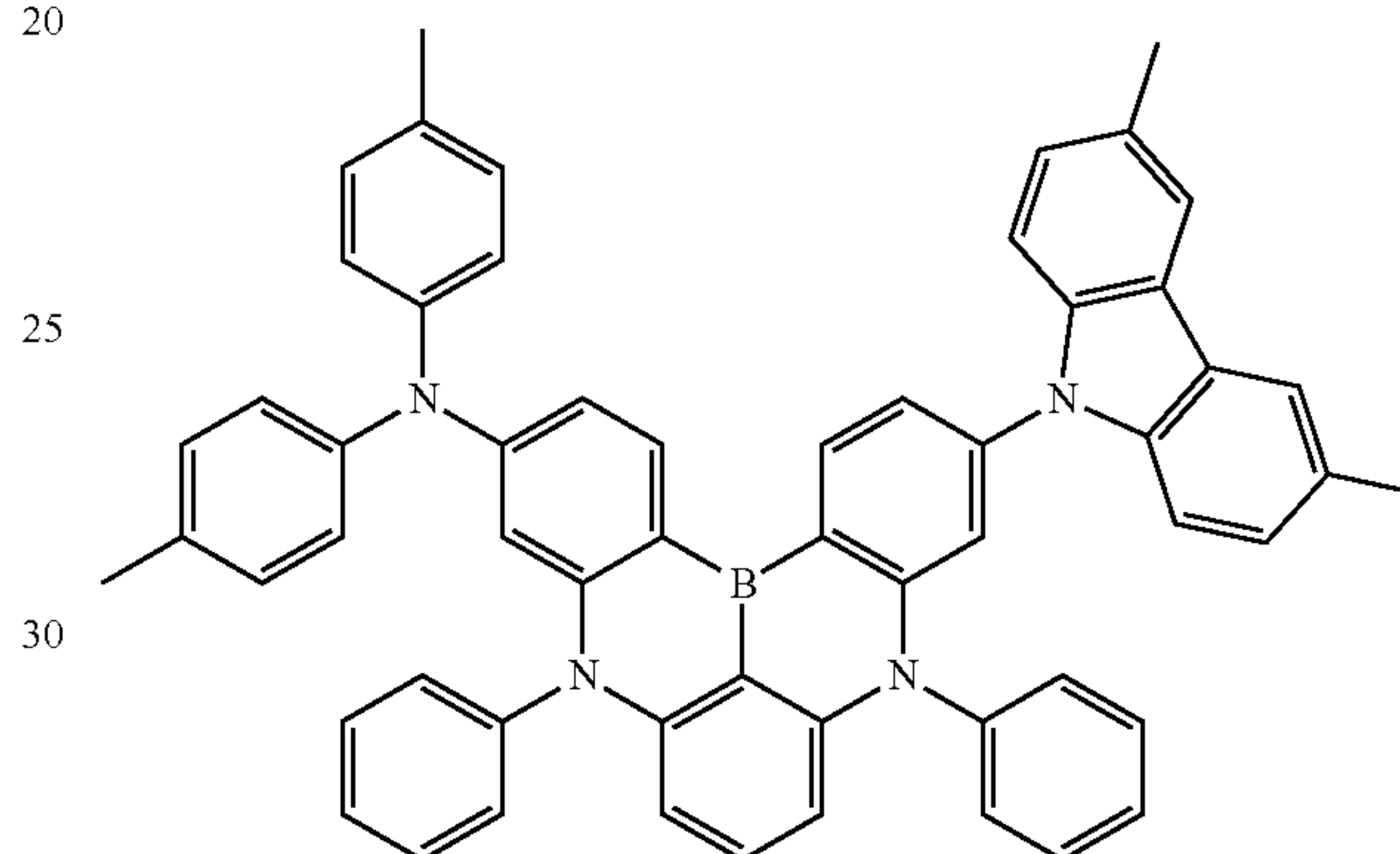
Dopant 78
