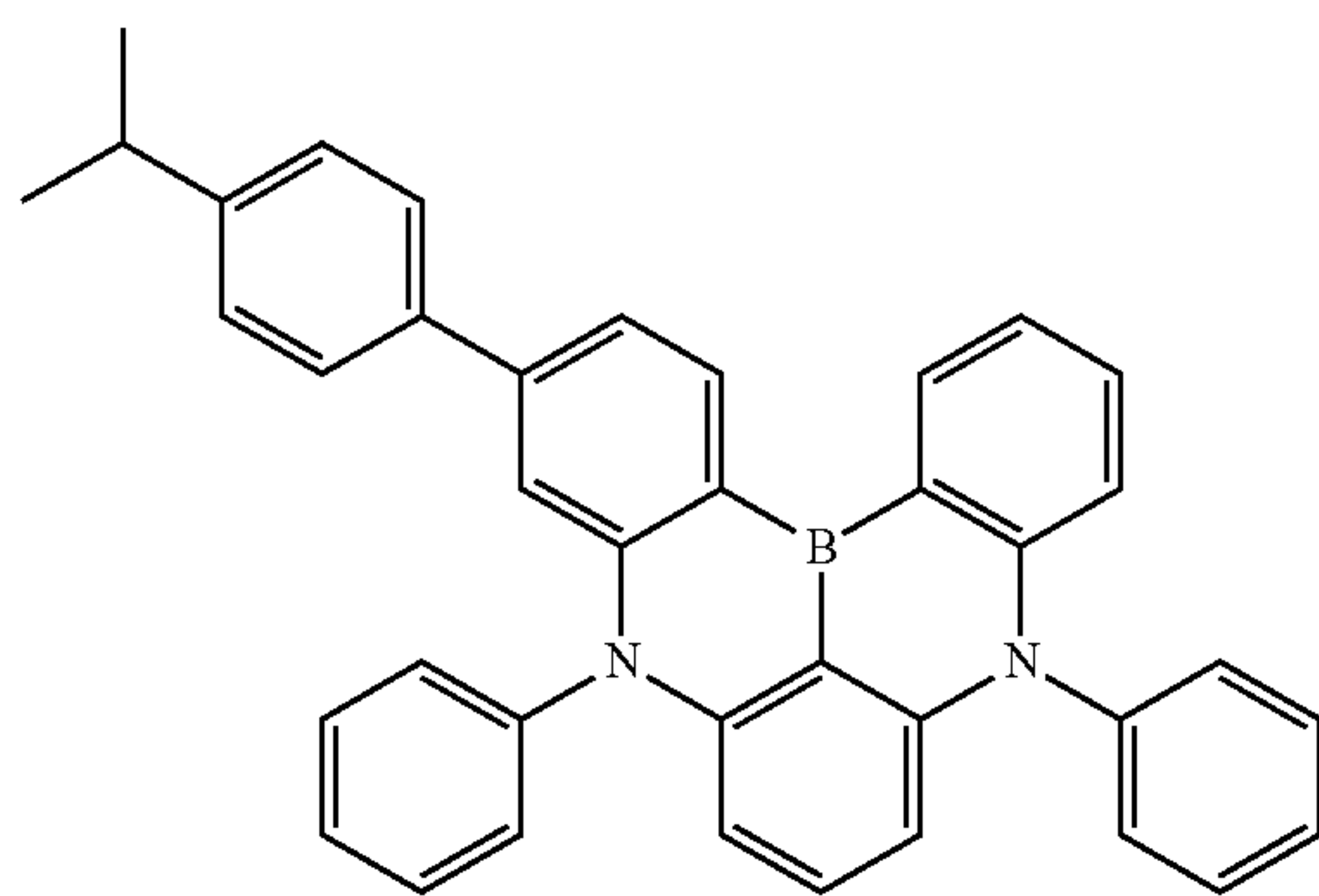
Dopant 20
