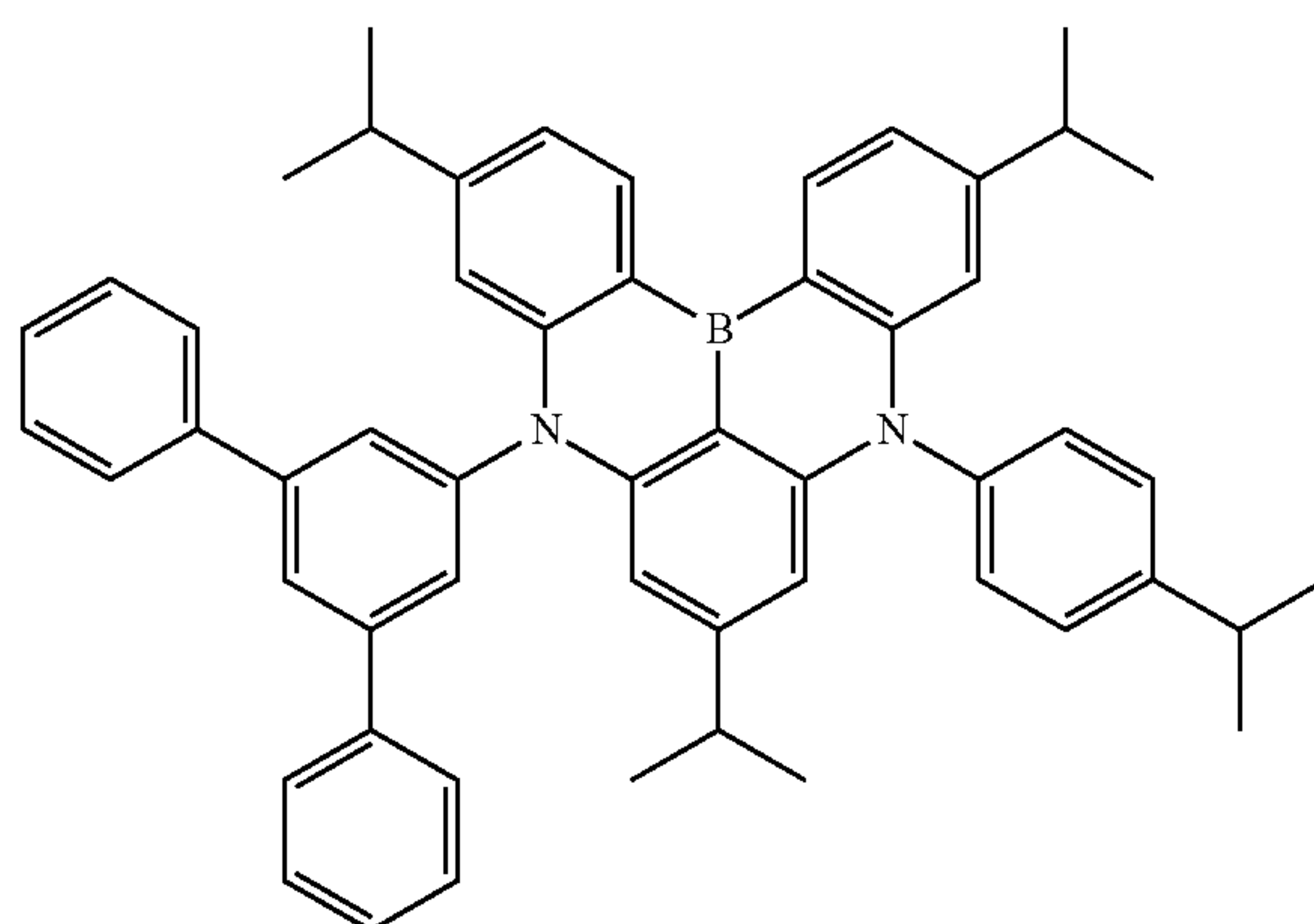
Dopant 151
