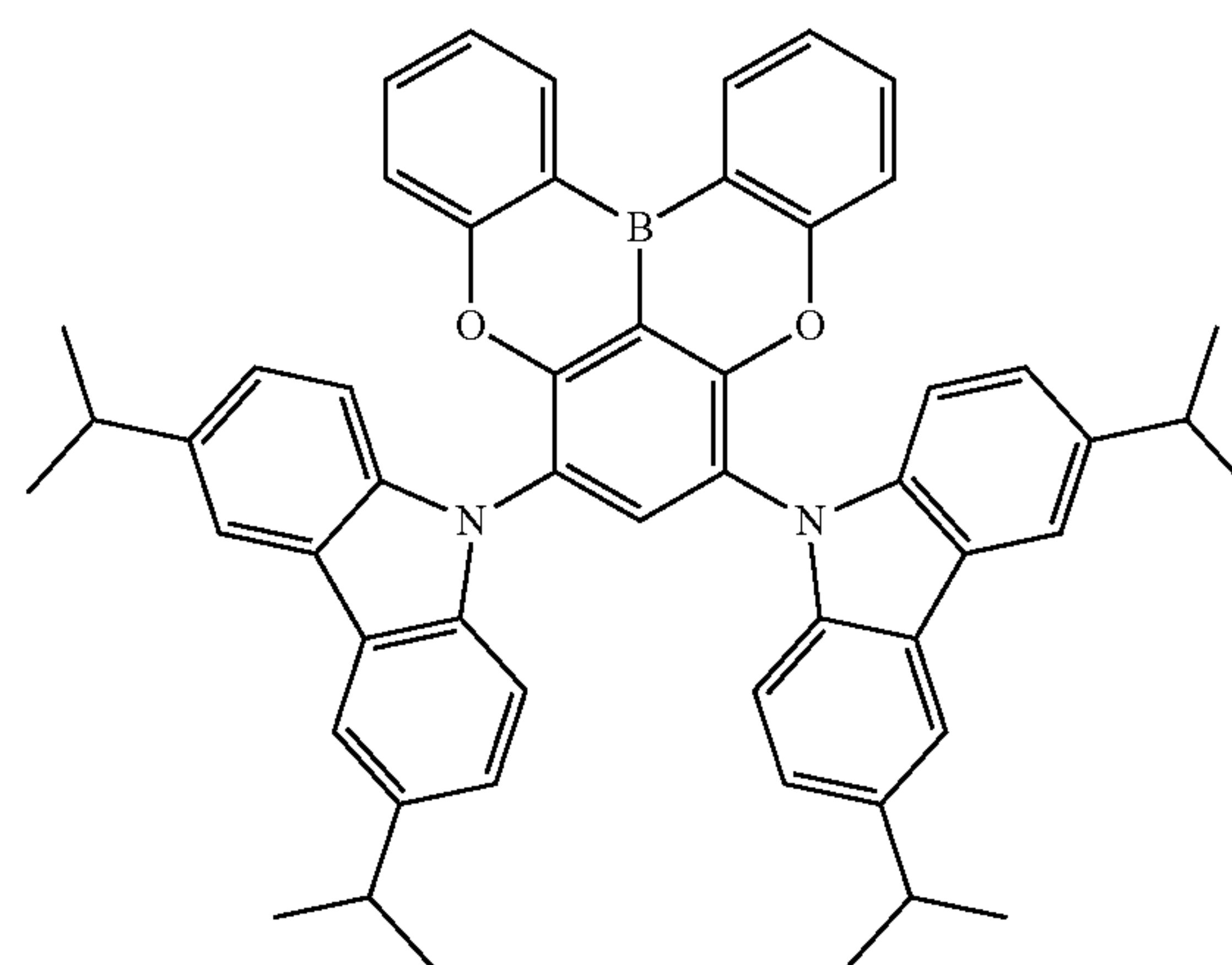
Dopant 232
