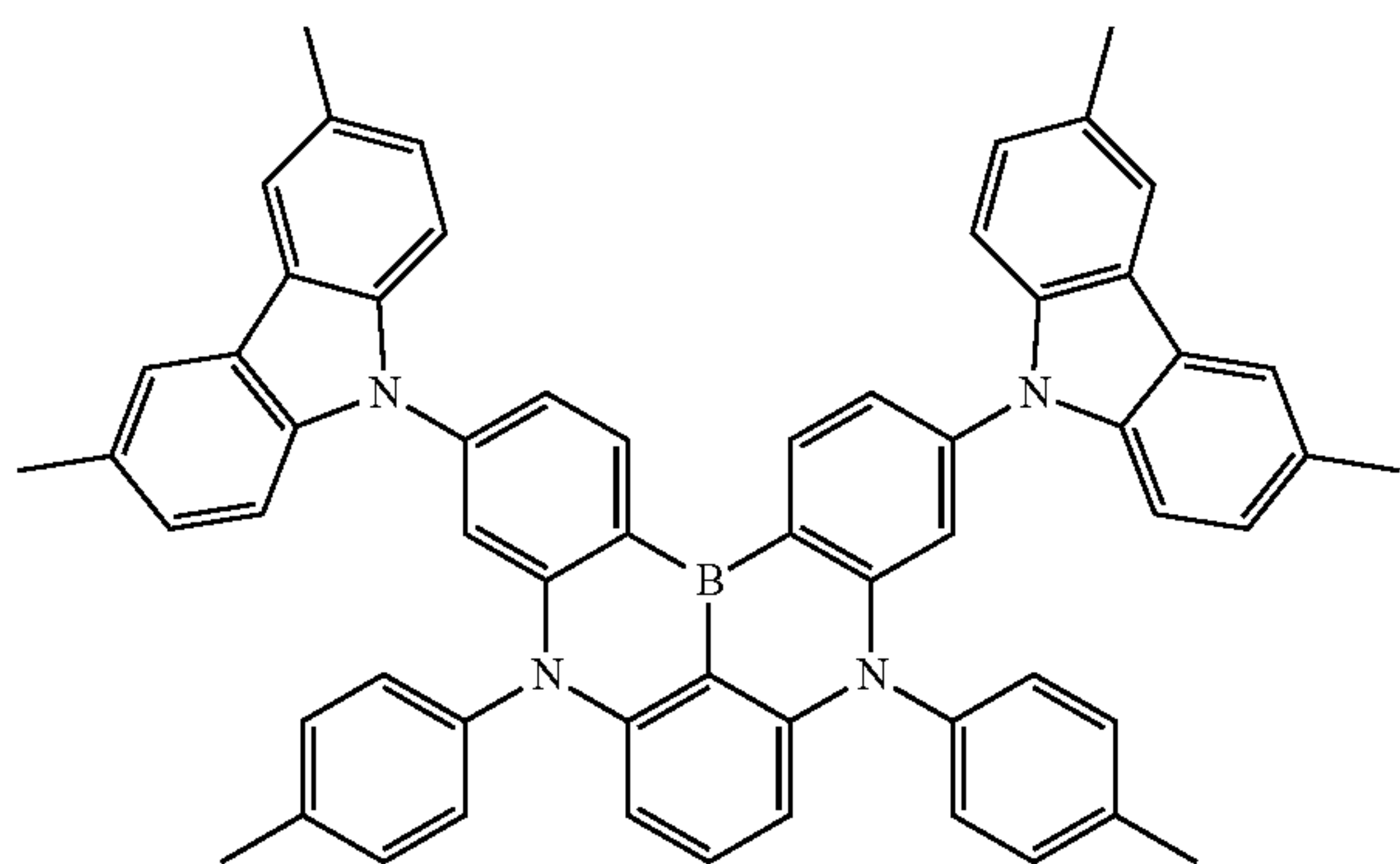
Dopant 73
