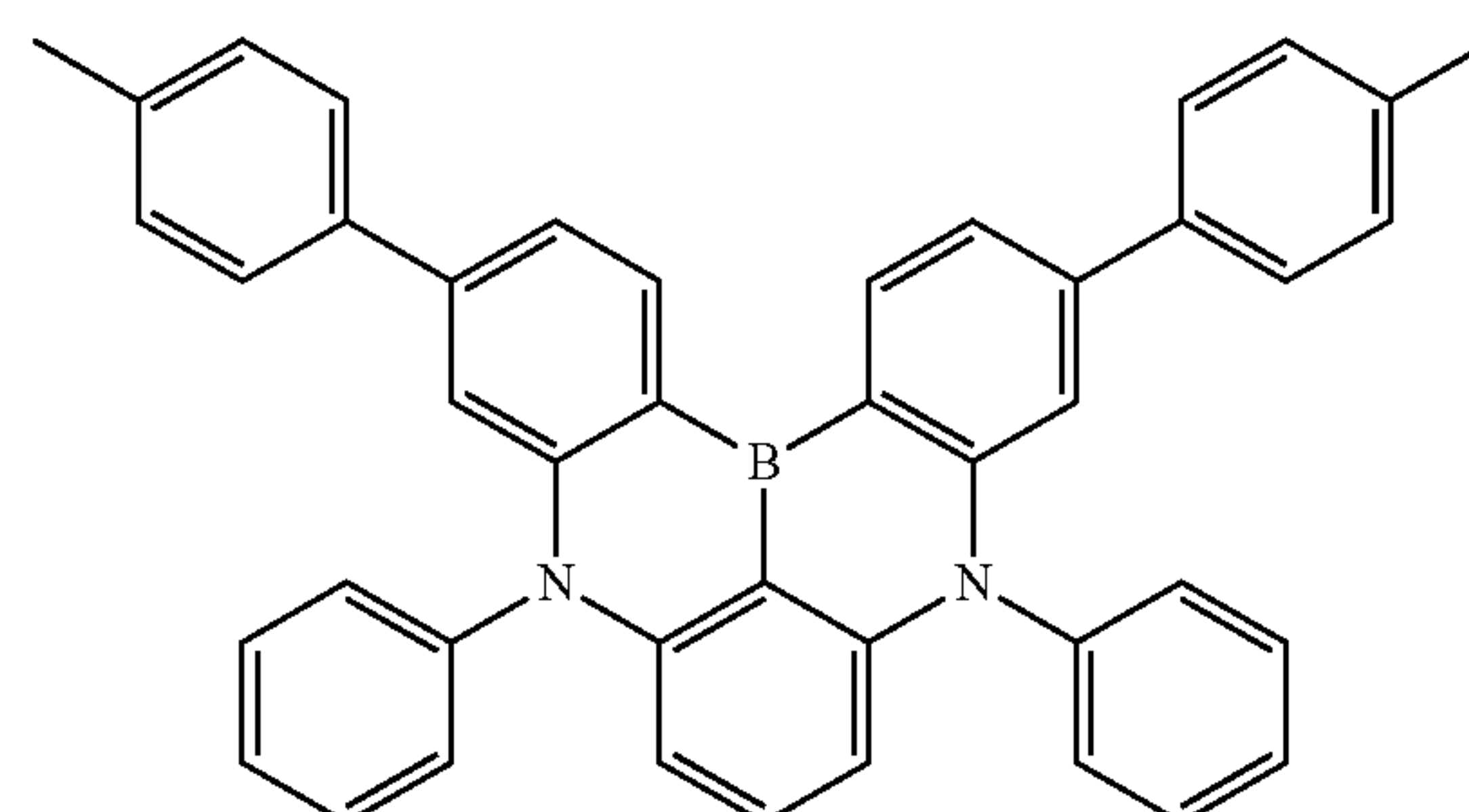
Dopant 9
