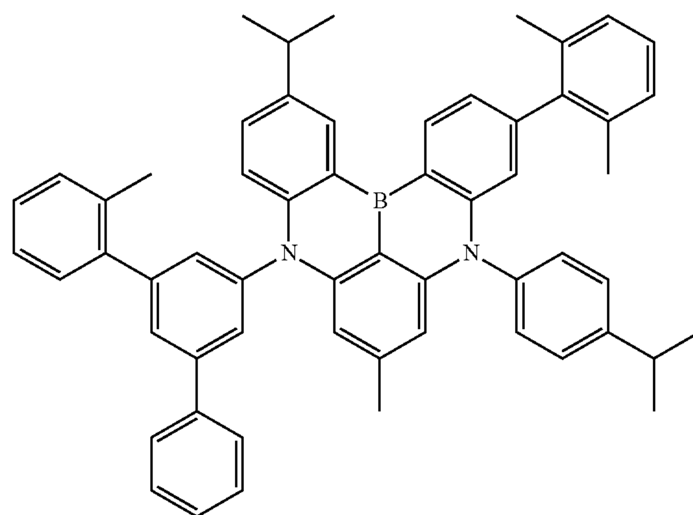
Dopant 163
