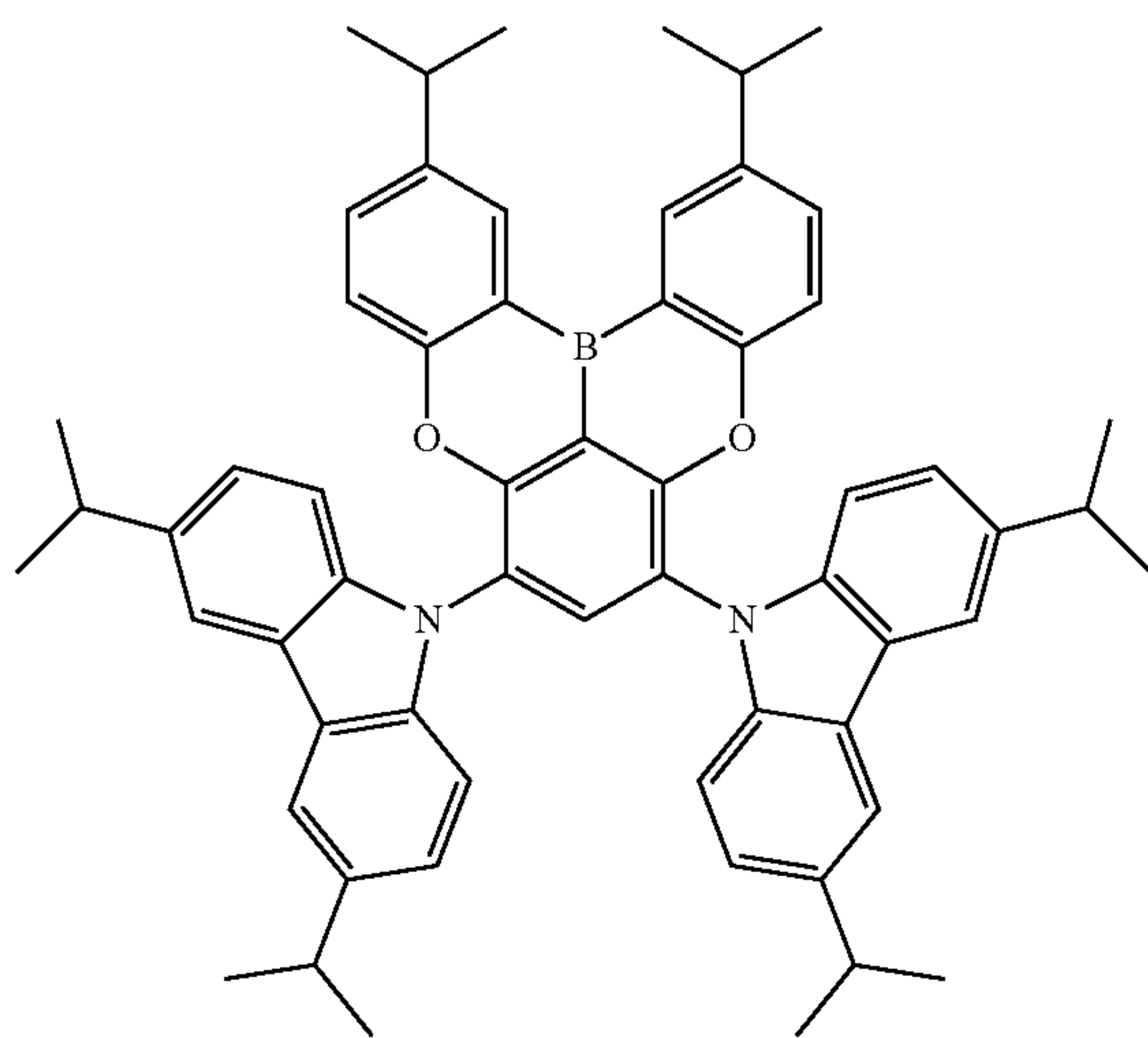
Dopant 231
