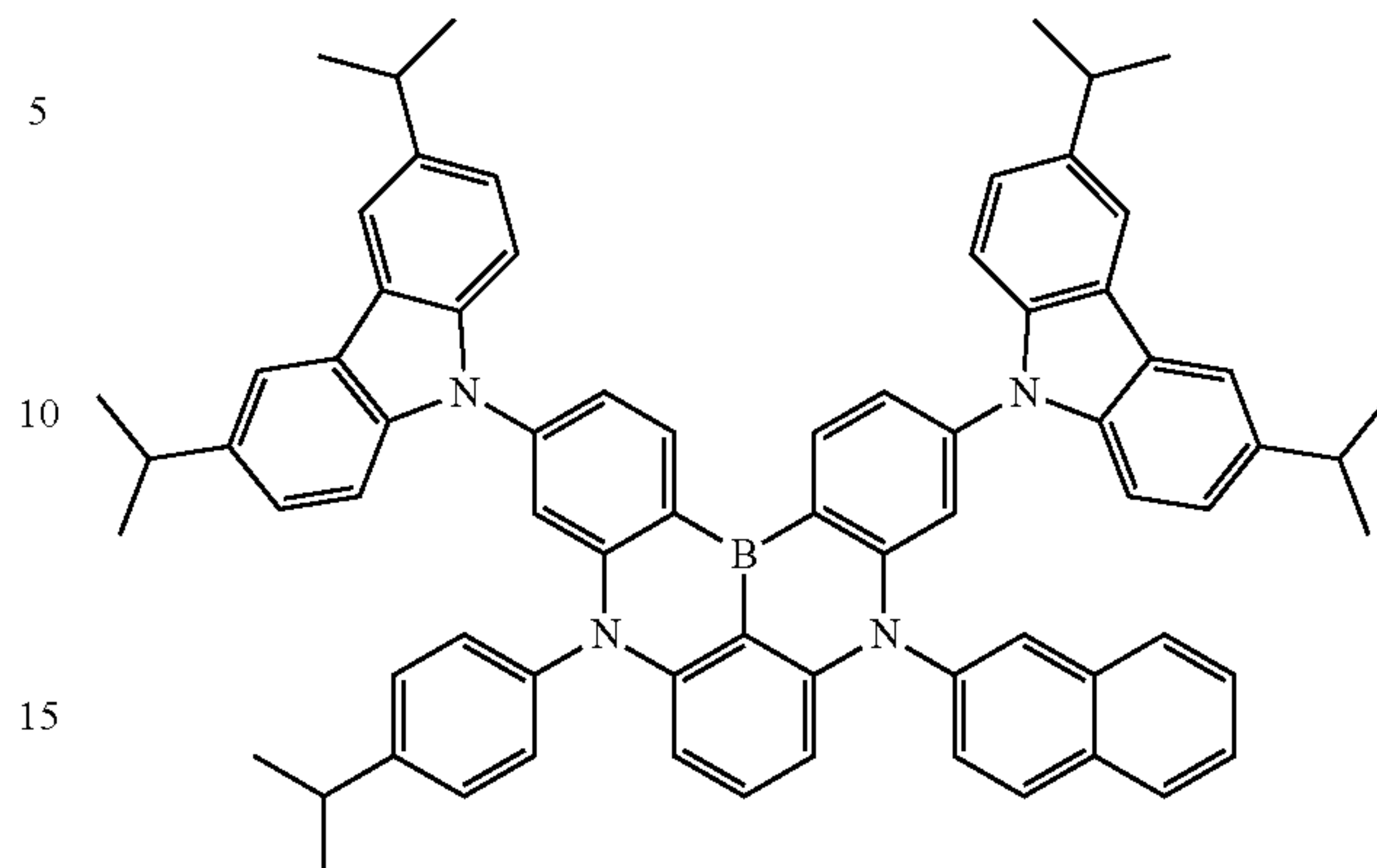
Dopant 109
