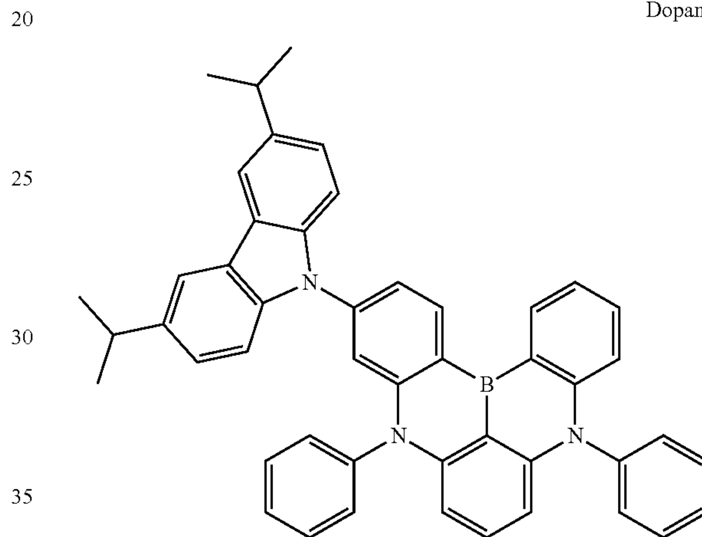
Dopant 71
