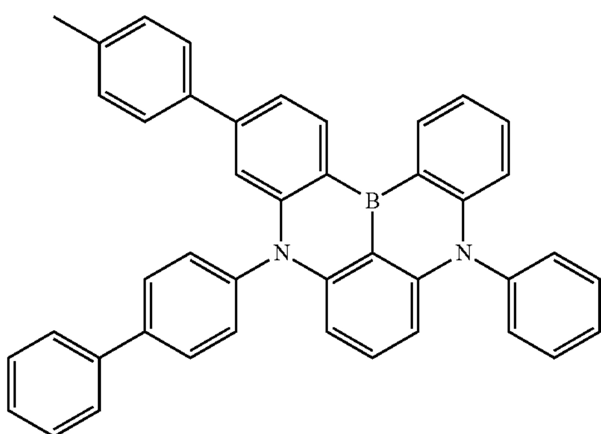
Dopant 28
