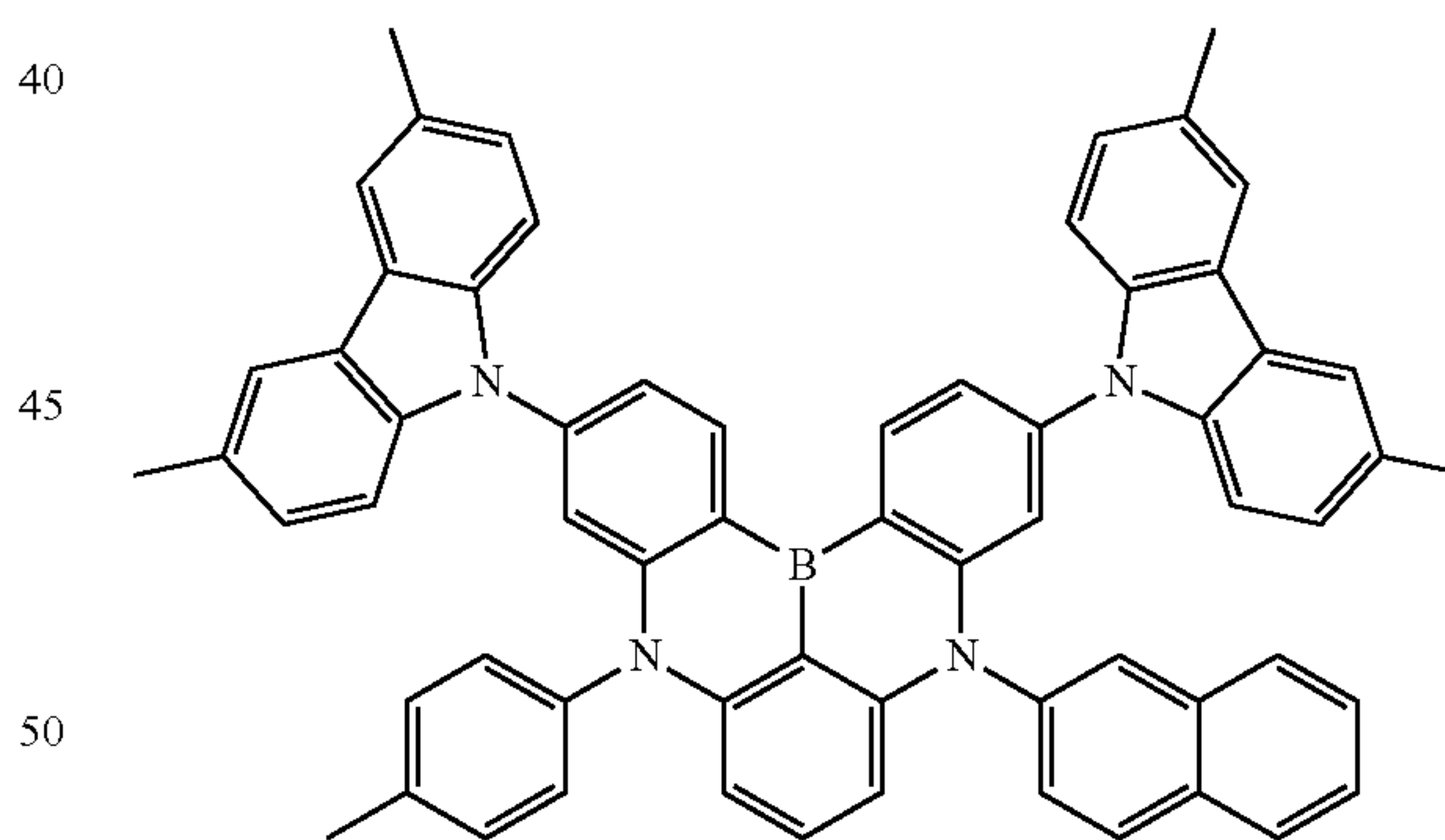
Dopant 108
