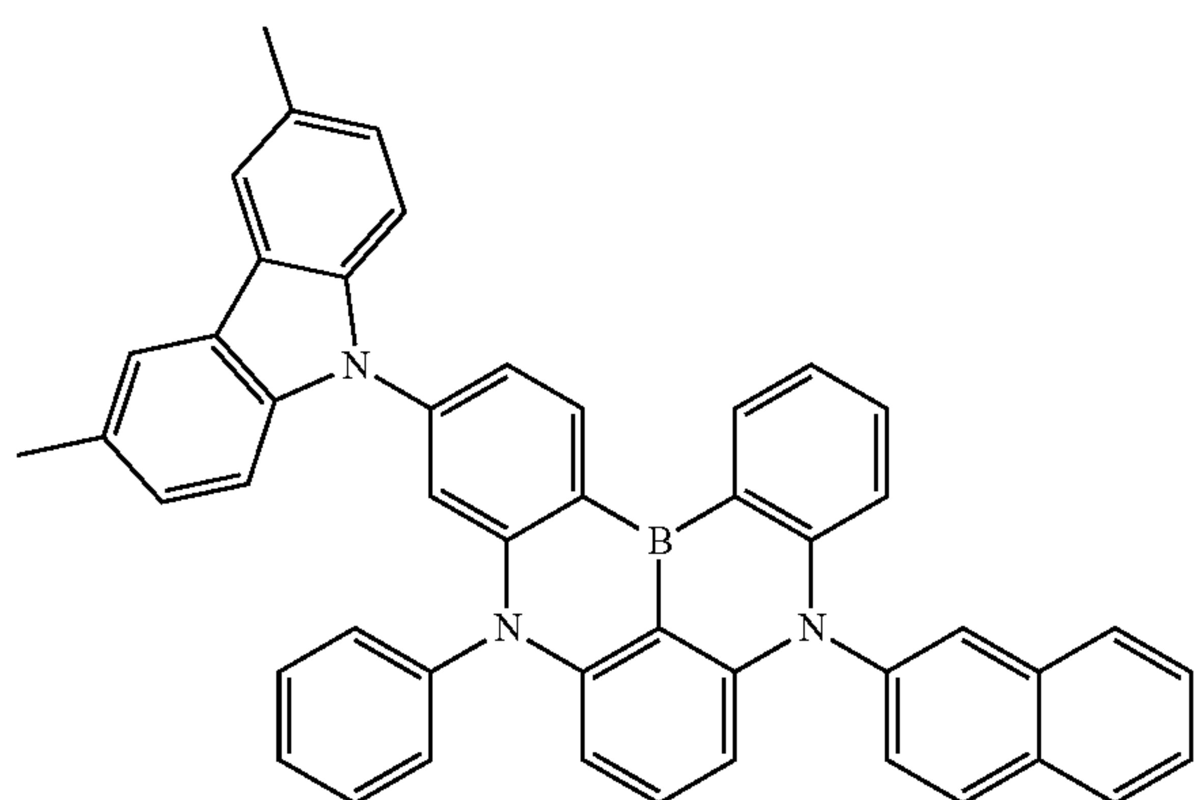
Dopant 104
