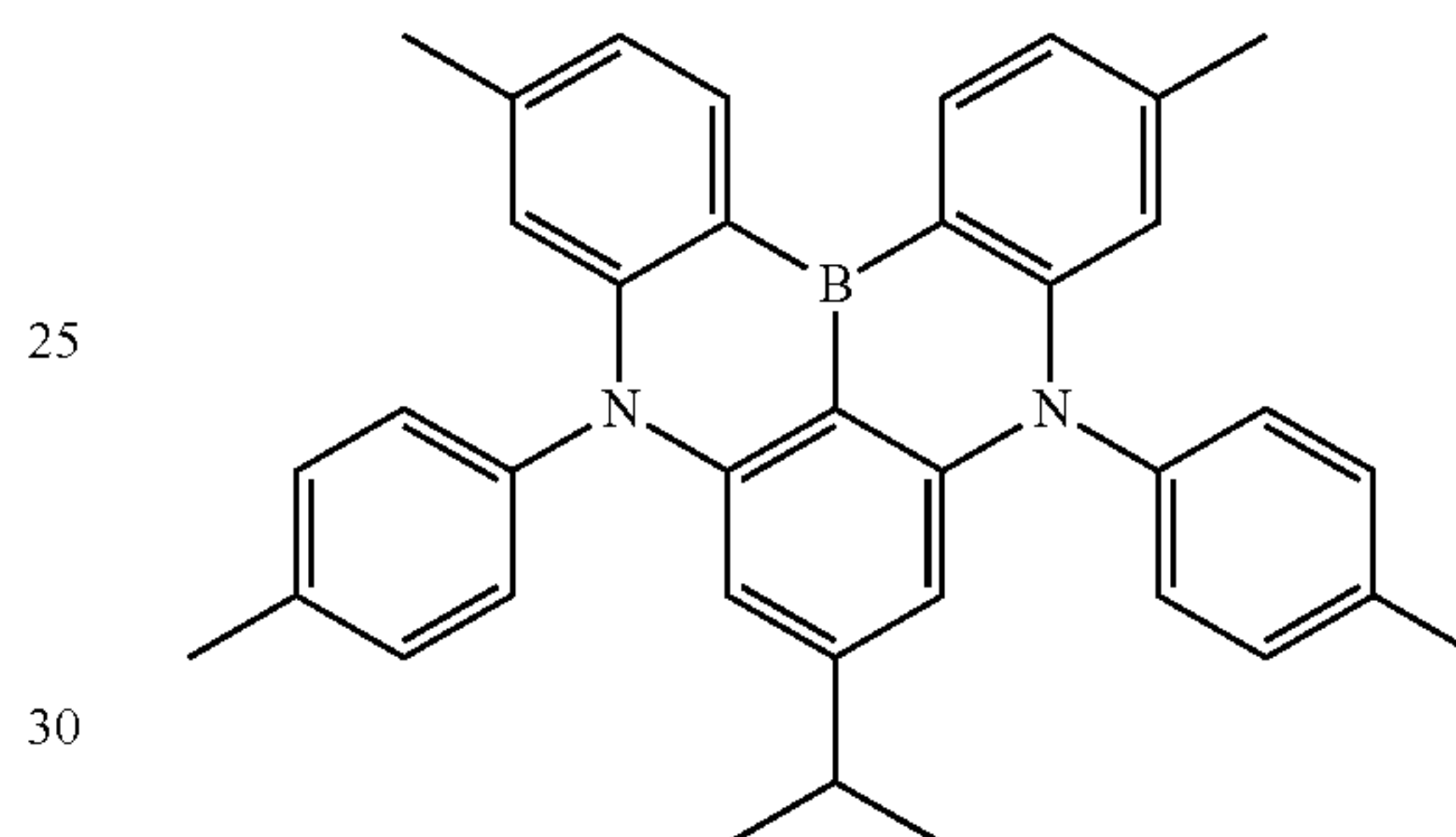
Dopant 146
