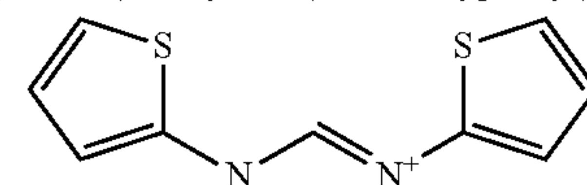
Thienyl-[(2-thienylamino)methylene]ammonium
