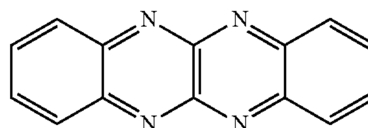
quinoxalino[2,3-b]quinoxaline
