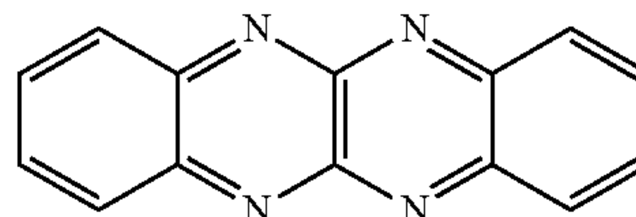
quinoxalino[2,3-b]quinoxaline
