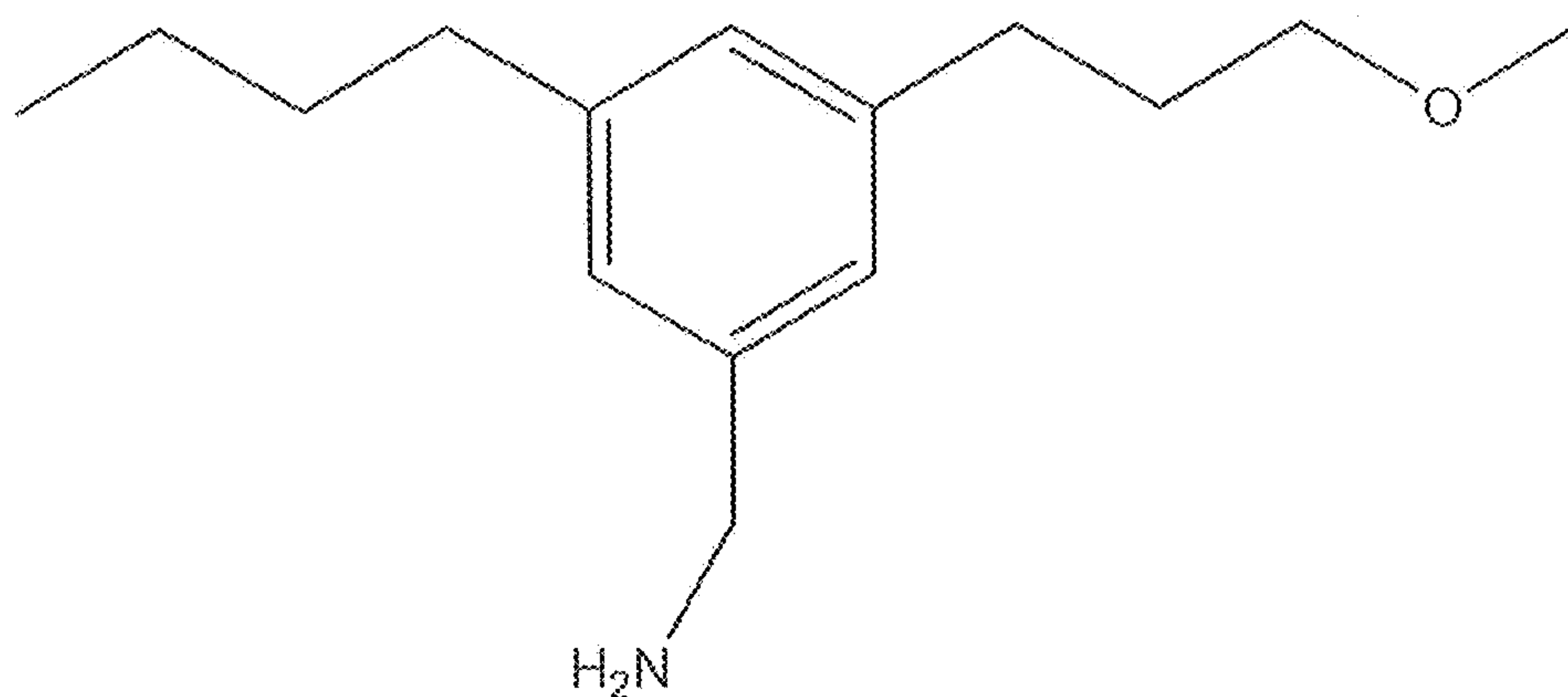
1-(3-butyl-5-methoxybutylphenyl)ethanamine
