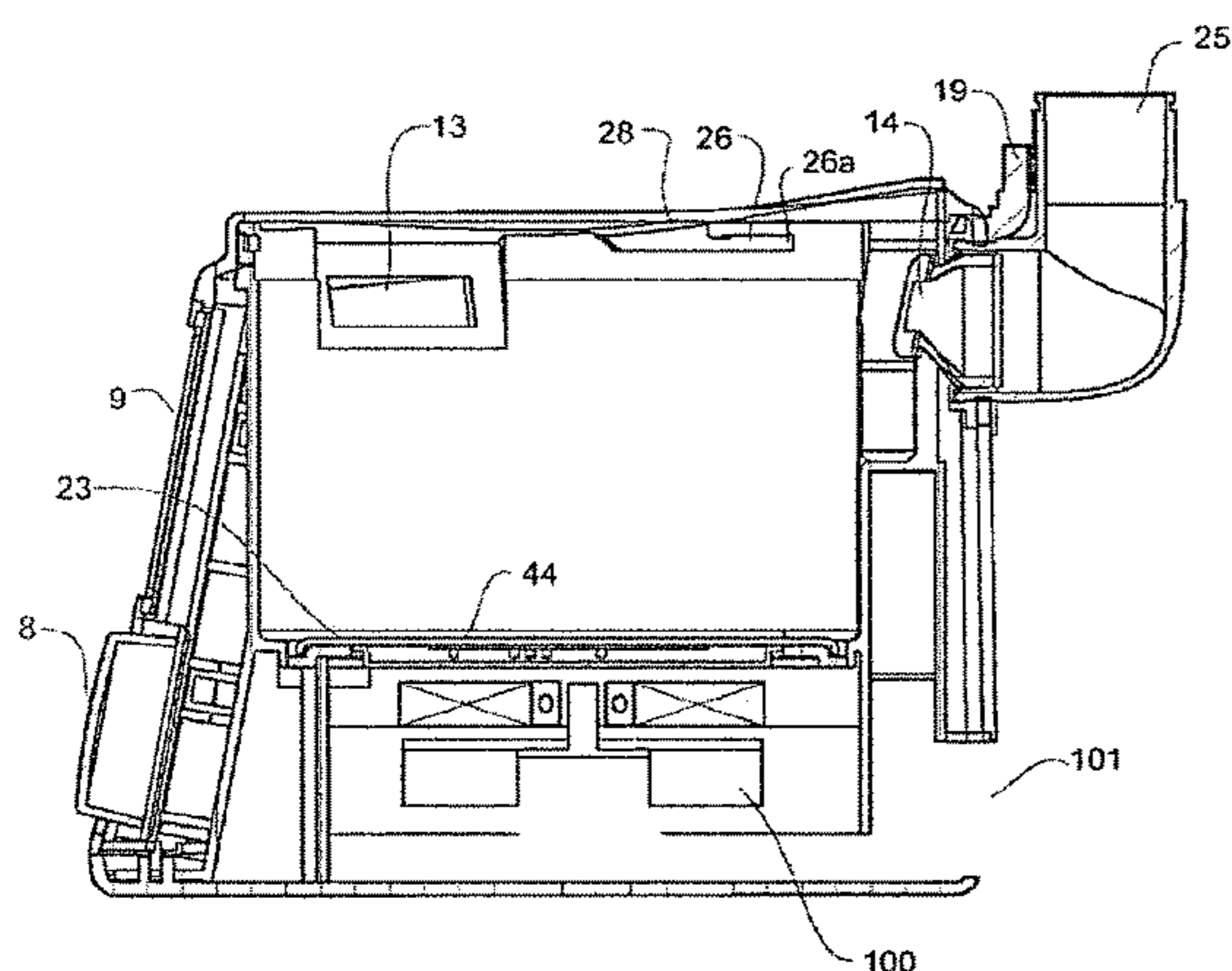
SECTION D-D
