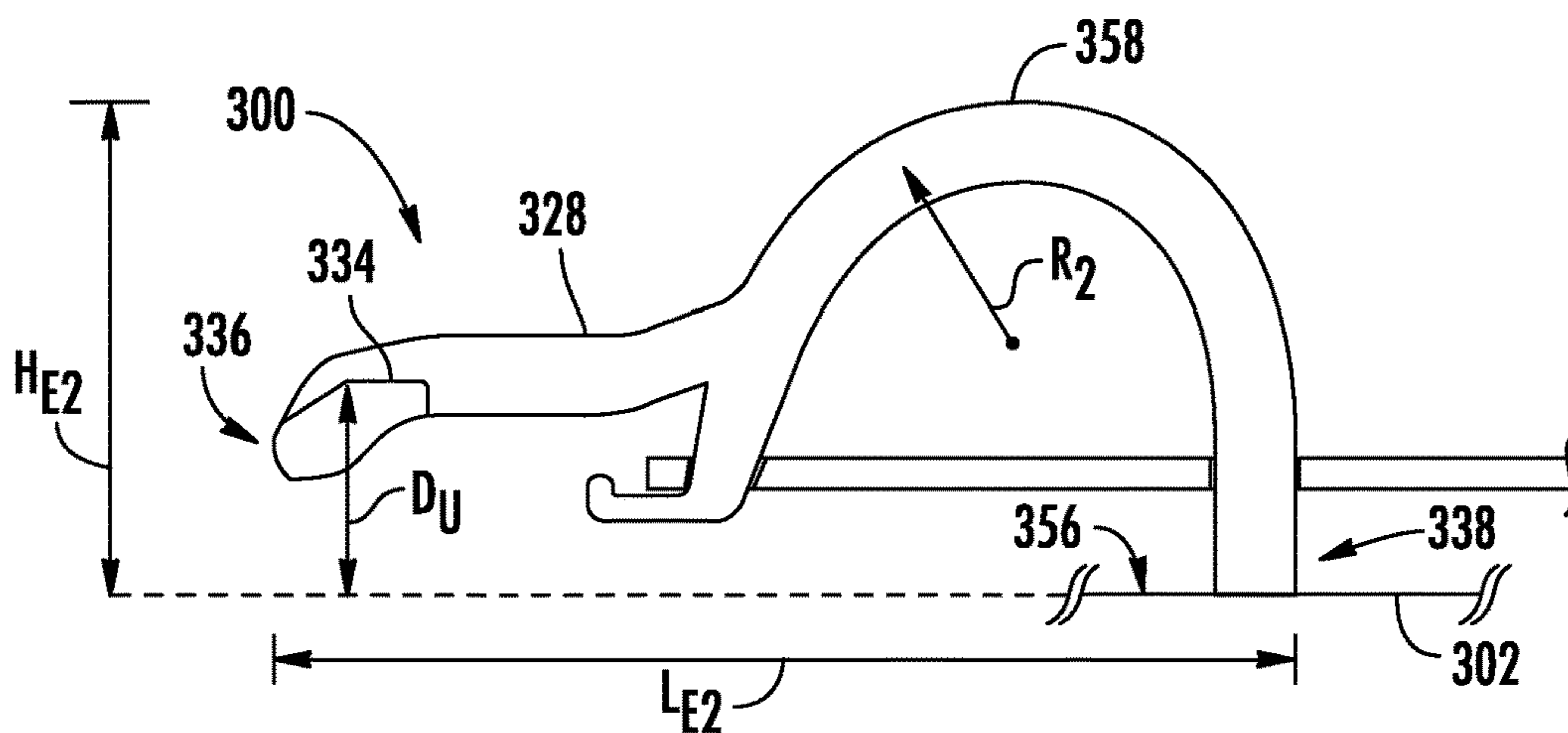
FIG. 6B
