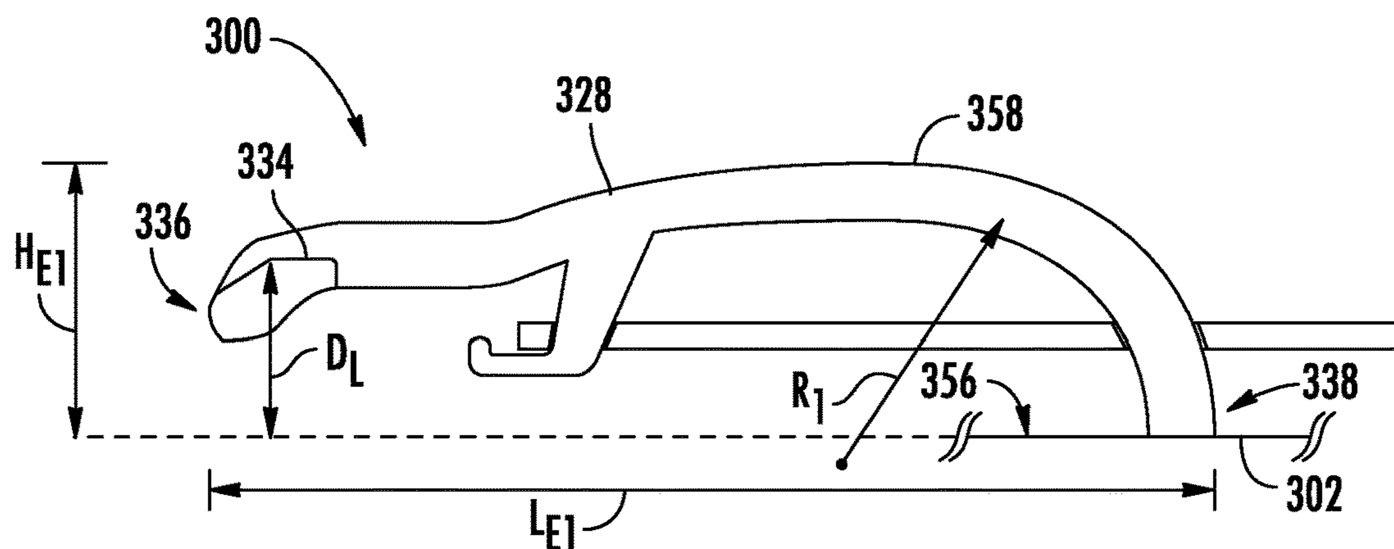
FIG. 6A
