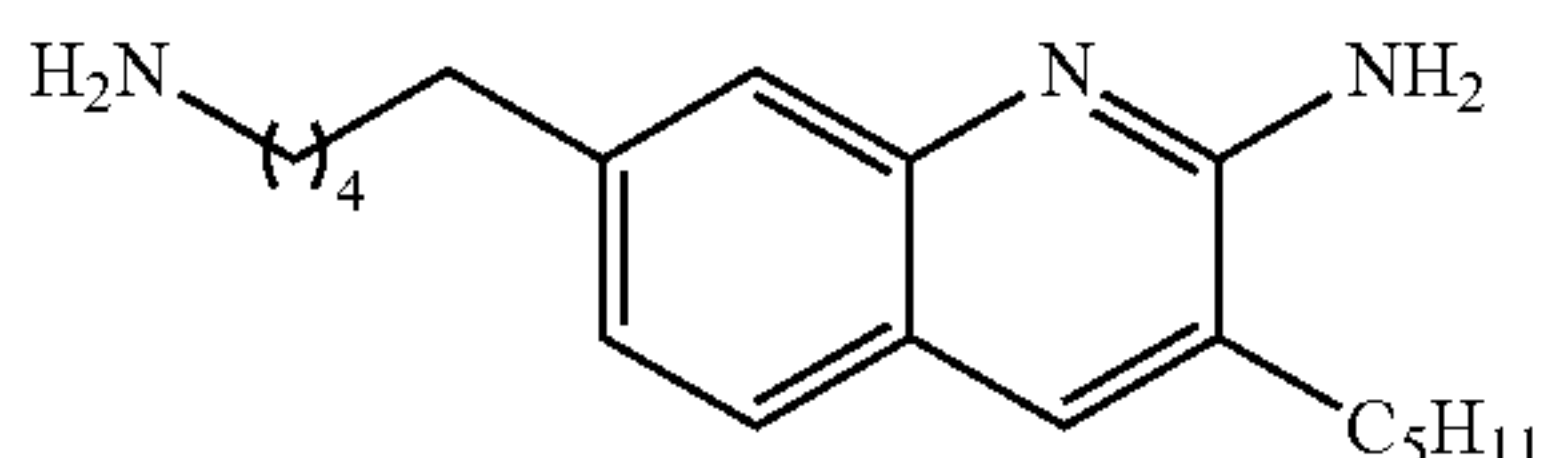
7-(5-Aminopentyl)-3-pentylquinolin-2-amine (36b)
