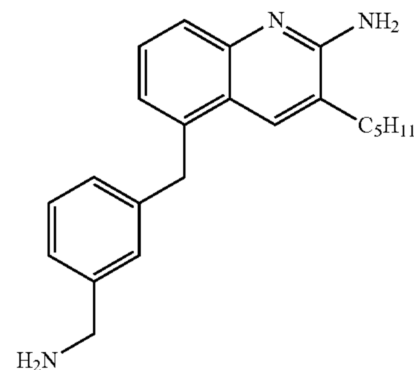
5-(3-(Aminomethyl)benzyl)-3-pentylquinolin-2-amine (18a)
