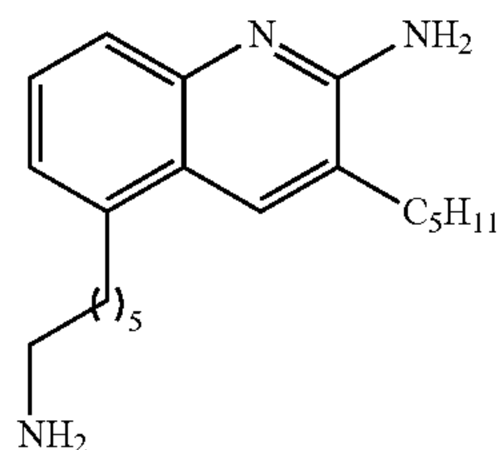
5-(6-Aminohexyl)-3-pentylquinolin-2-amine (34c)
