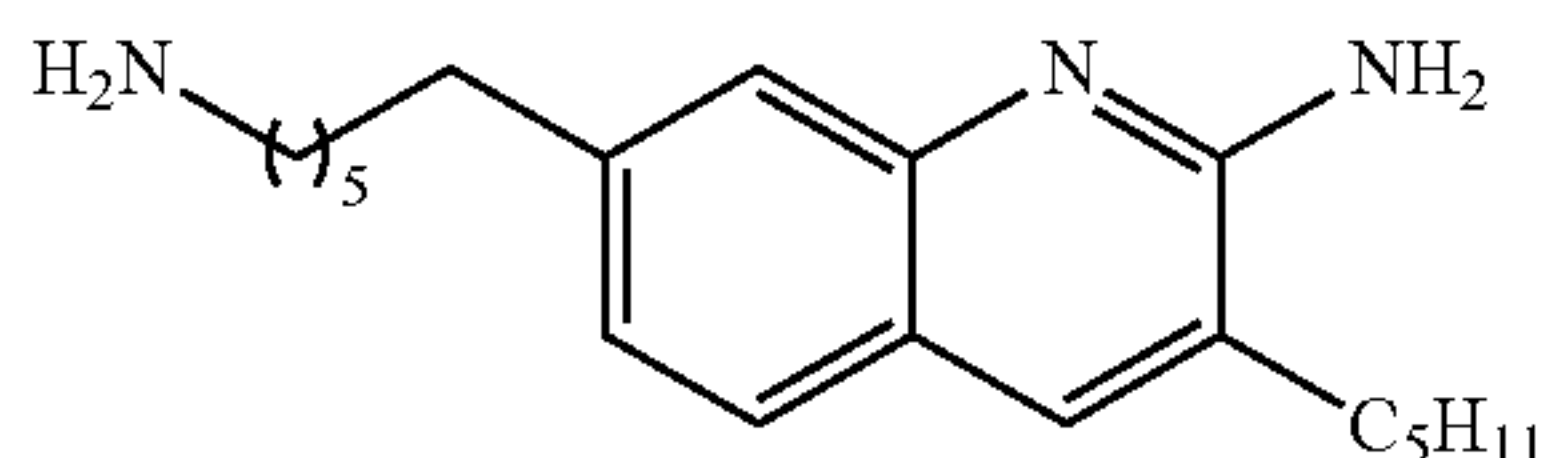
7-(6-Aminohexyl)-3-pentylquinolin-2-amine (36c)
