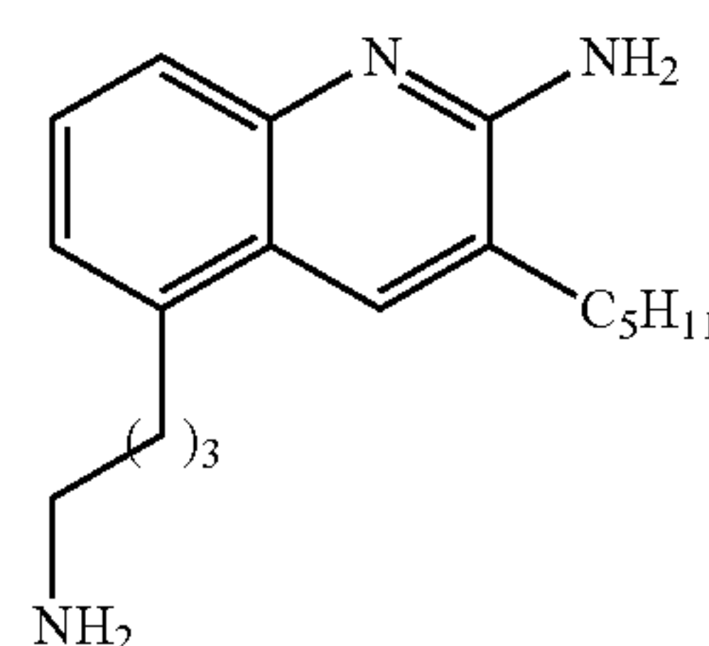
5-(4-Aminobutyl)-3-pentylquinolin-2-amine (34a)
