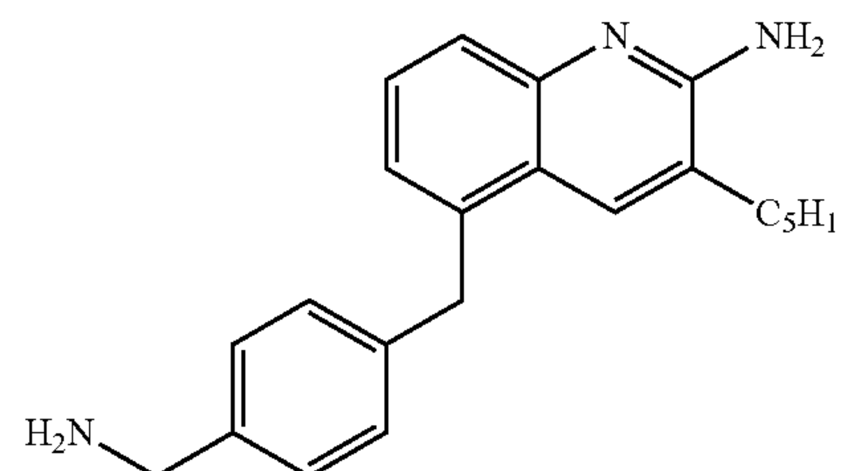
5-(4-(Aminomethyl)benzyl)-3-pentylquinolin-2-amine (18b)
