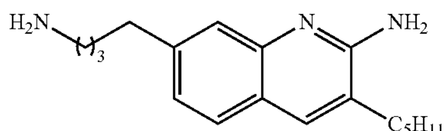
7-(4-Aminobutyl)-3-pentylquinolin-2-amine (36a)
