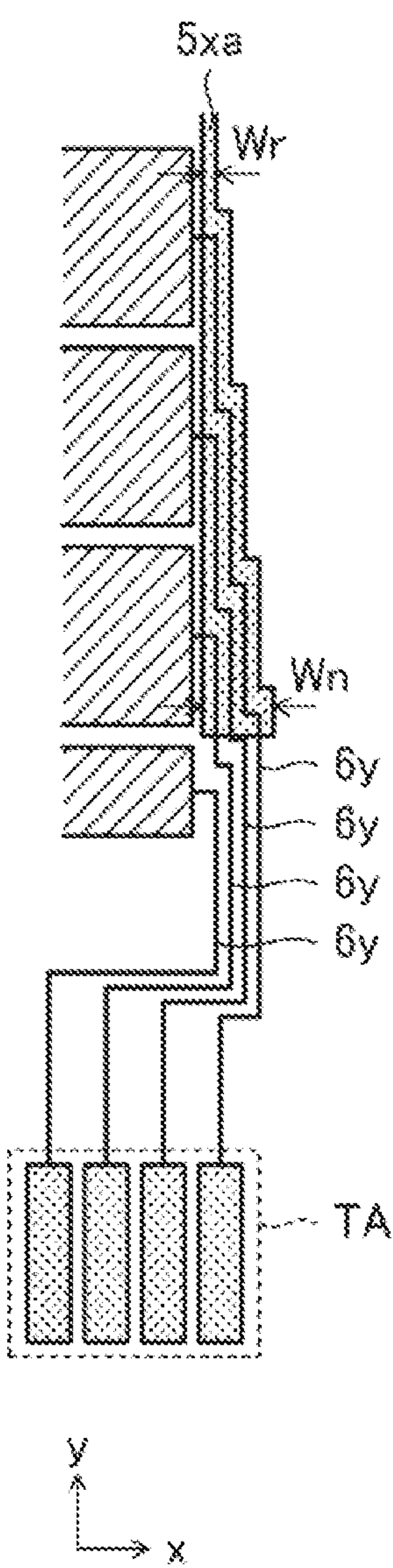
FIG. 9B
