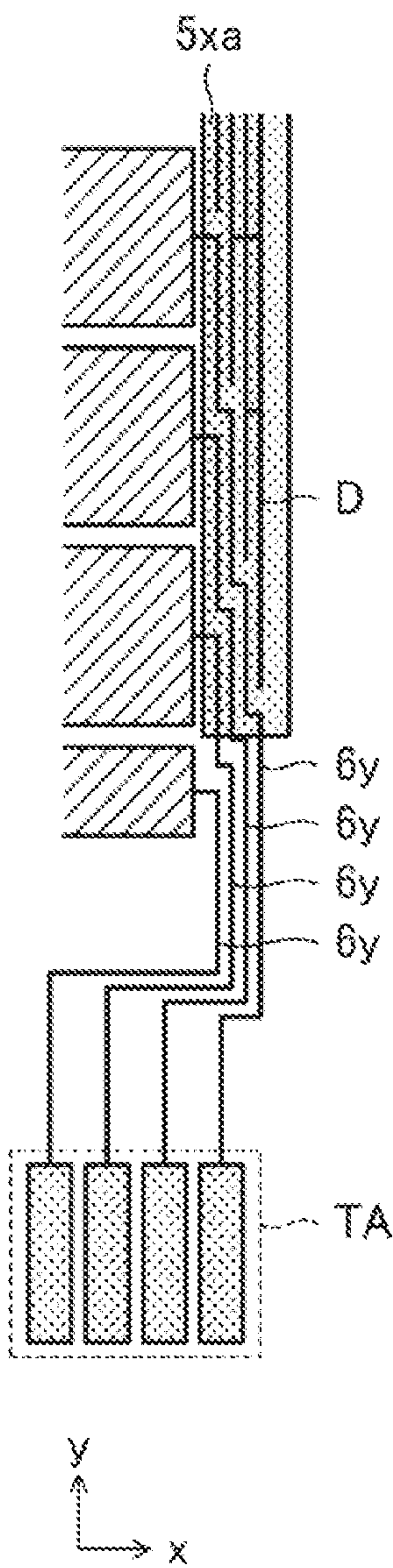
FIG. 9A
