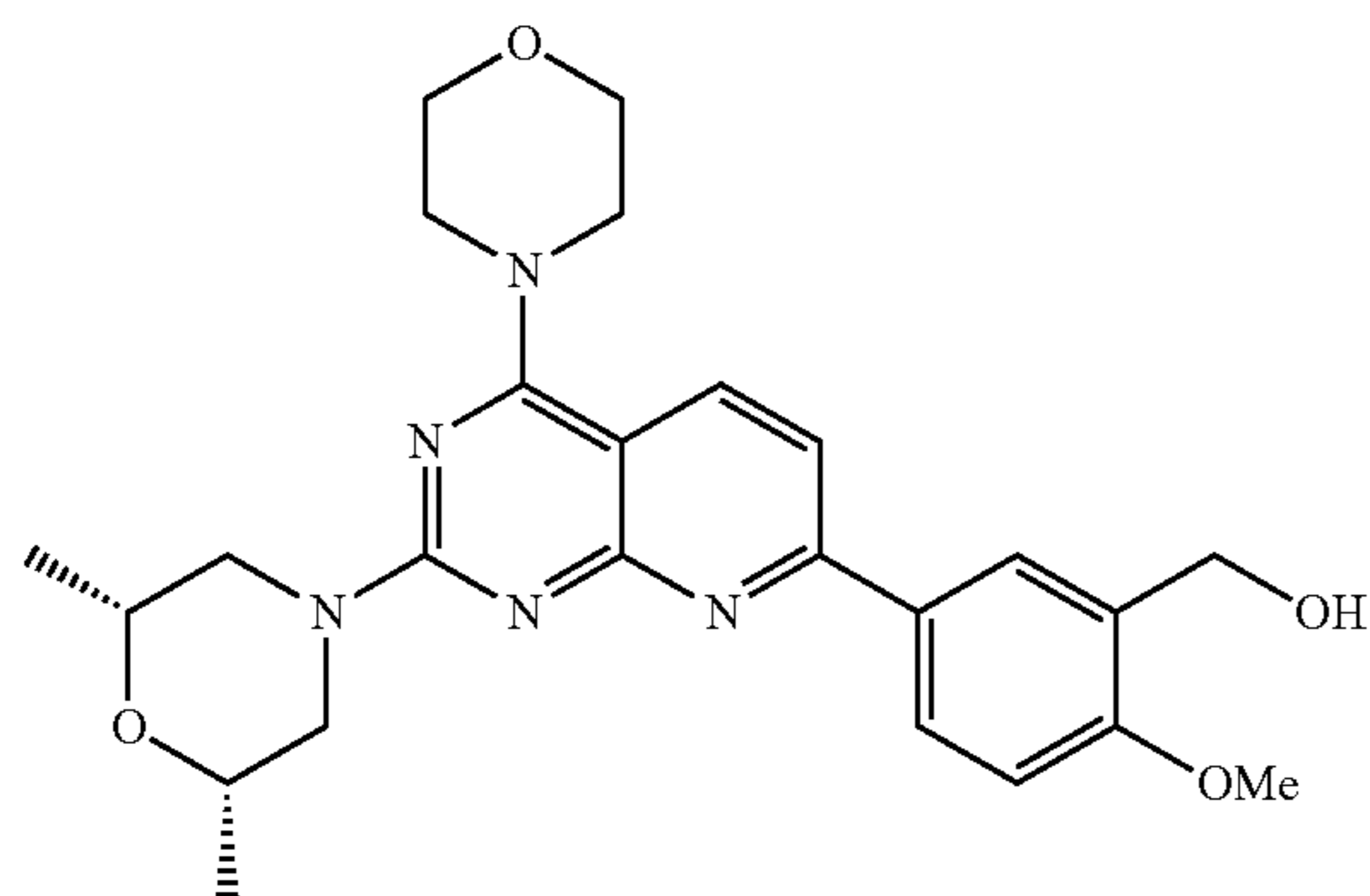
KU-0063794
