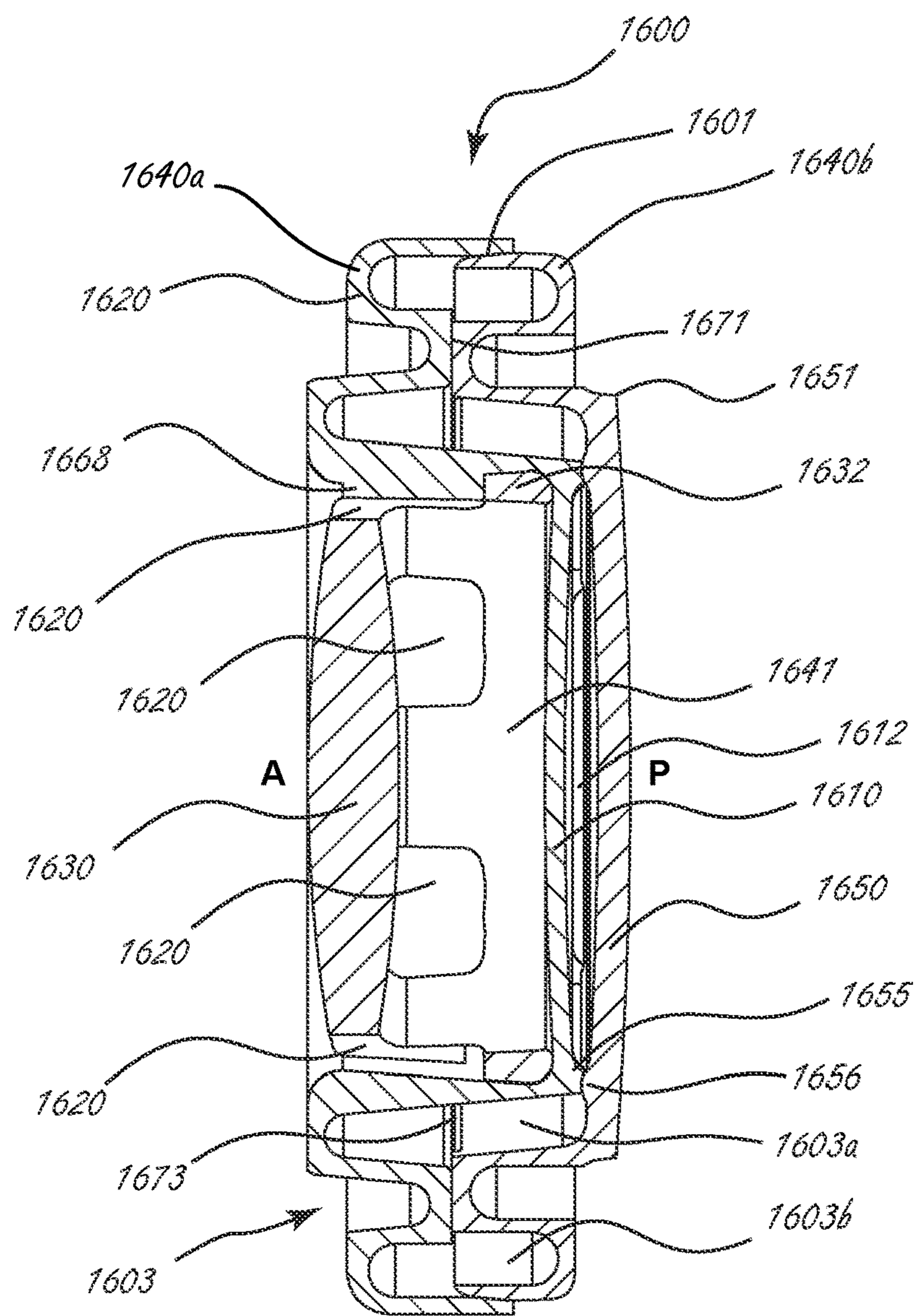
SECTION A-A
