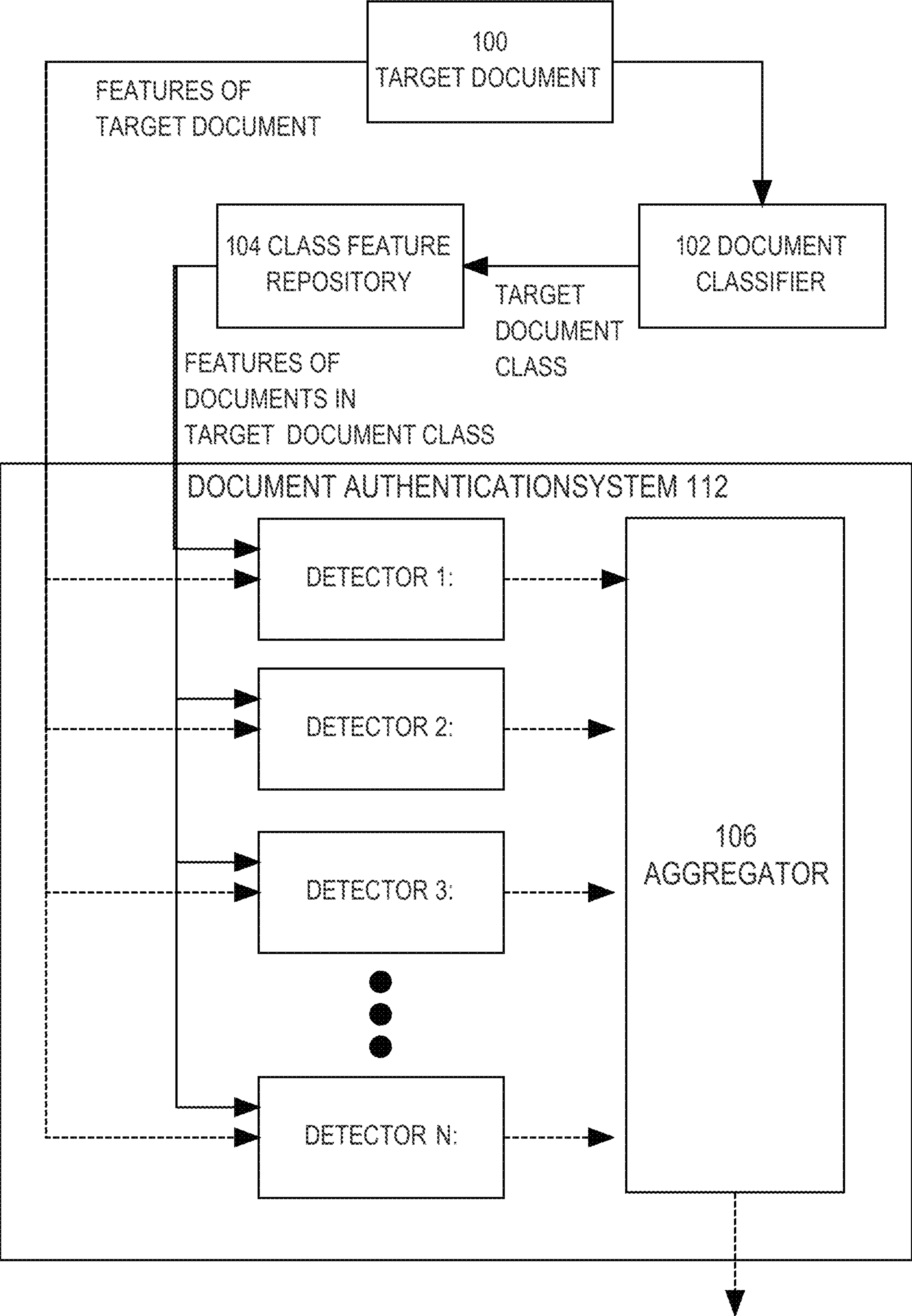
FIG. 1 DOCUMENT ANOMALY SCORE 110
