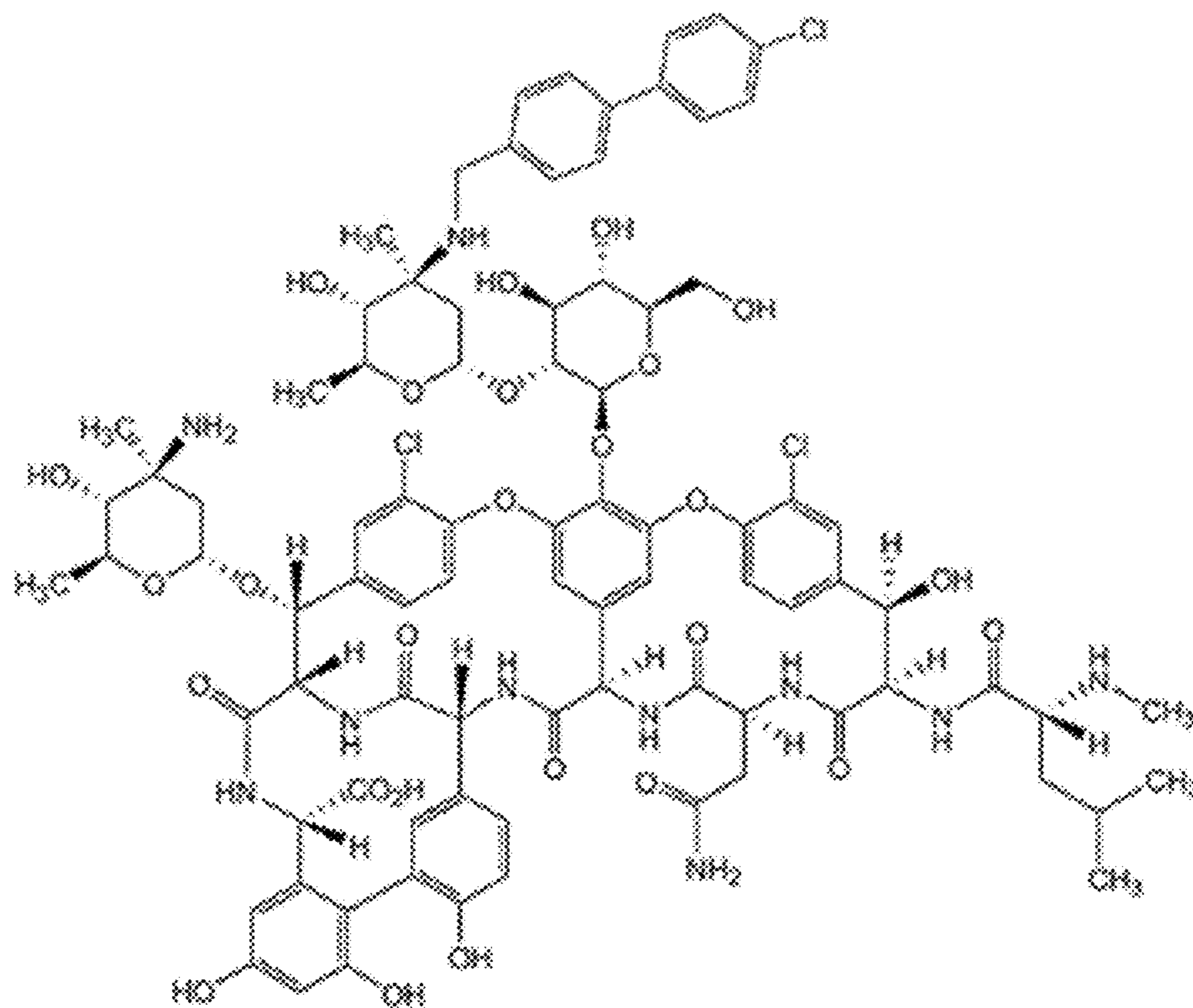
Oritavancin
