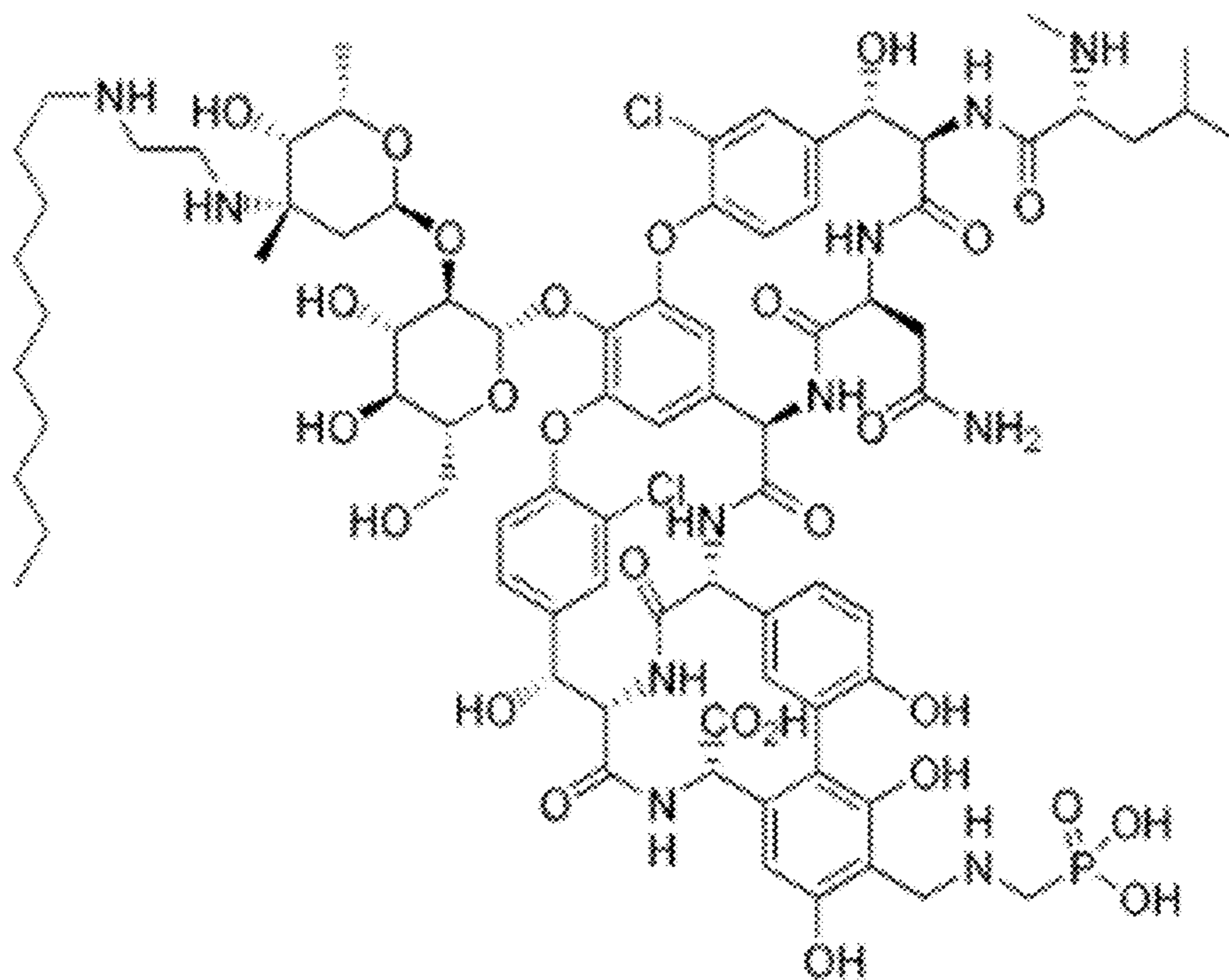
Telavancin
