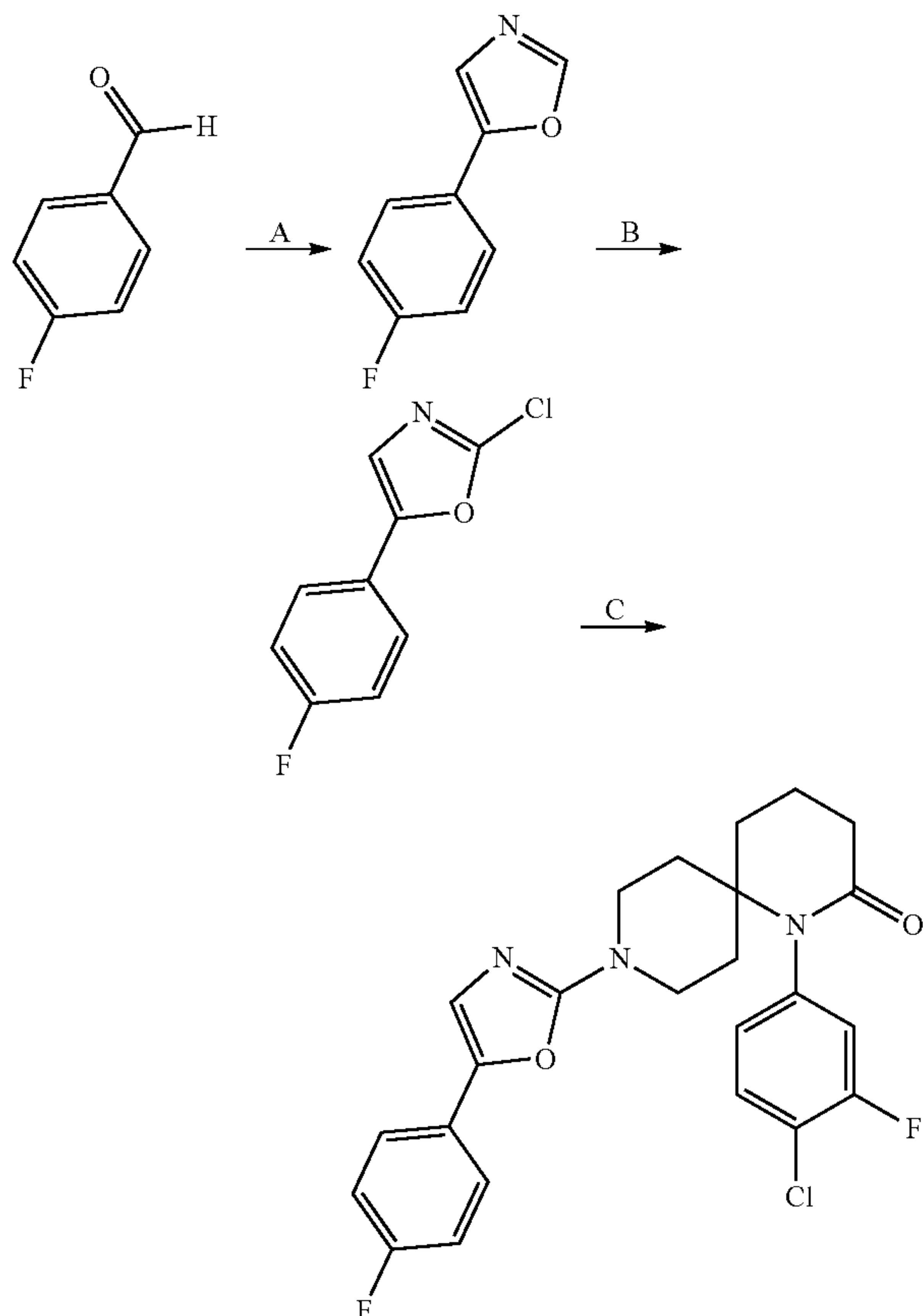
Step A: 5-(4-fluorophenyl)oxazole
