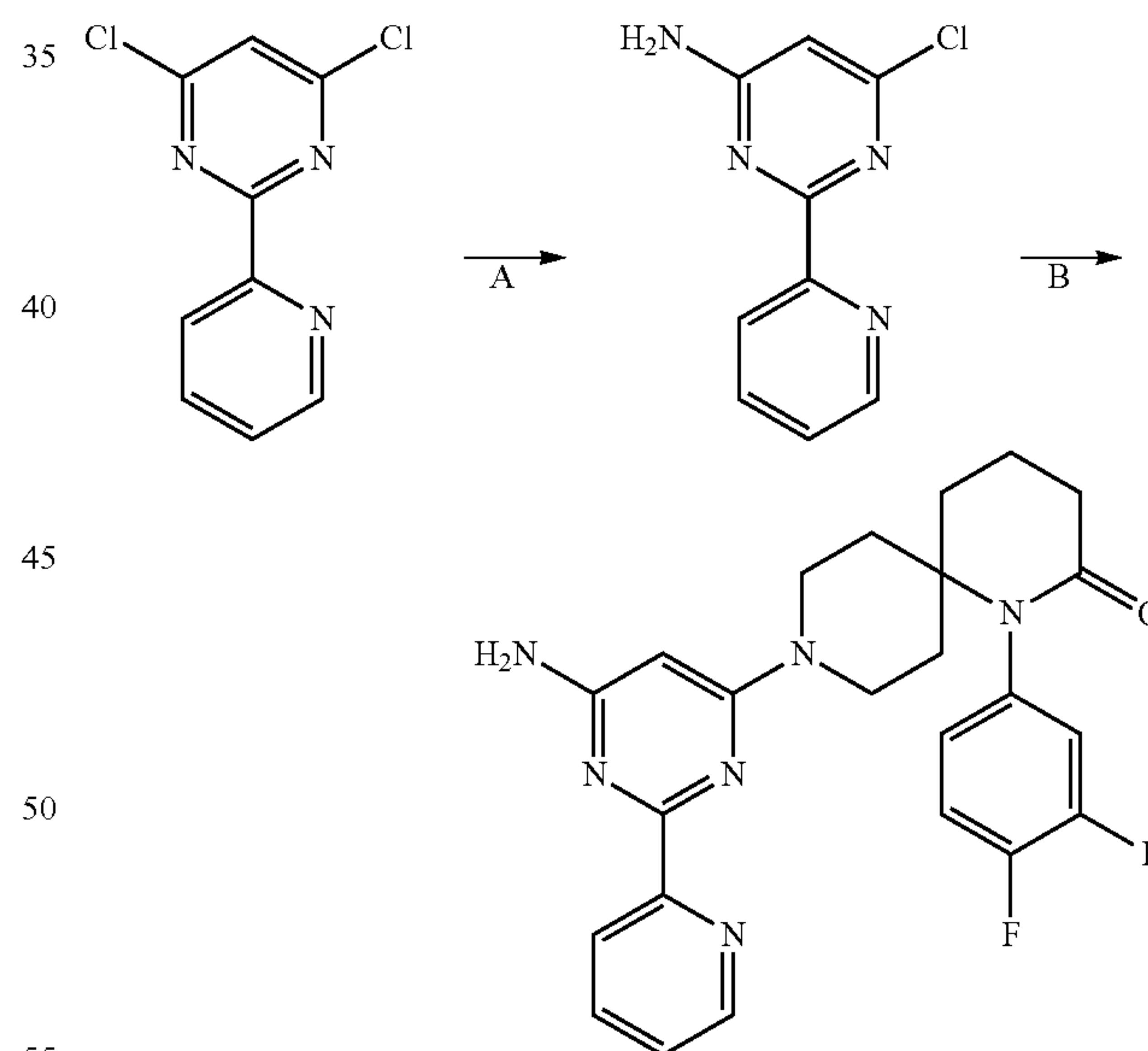
Step A: 6-chloro-2-(pyridin-2-yl)pyrimidin-4-amine
