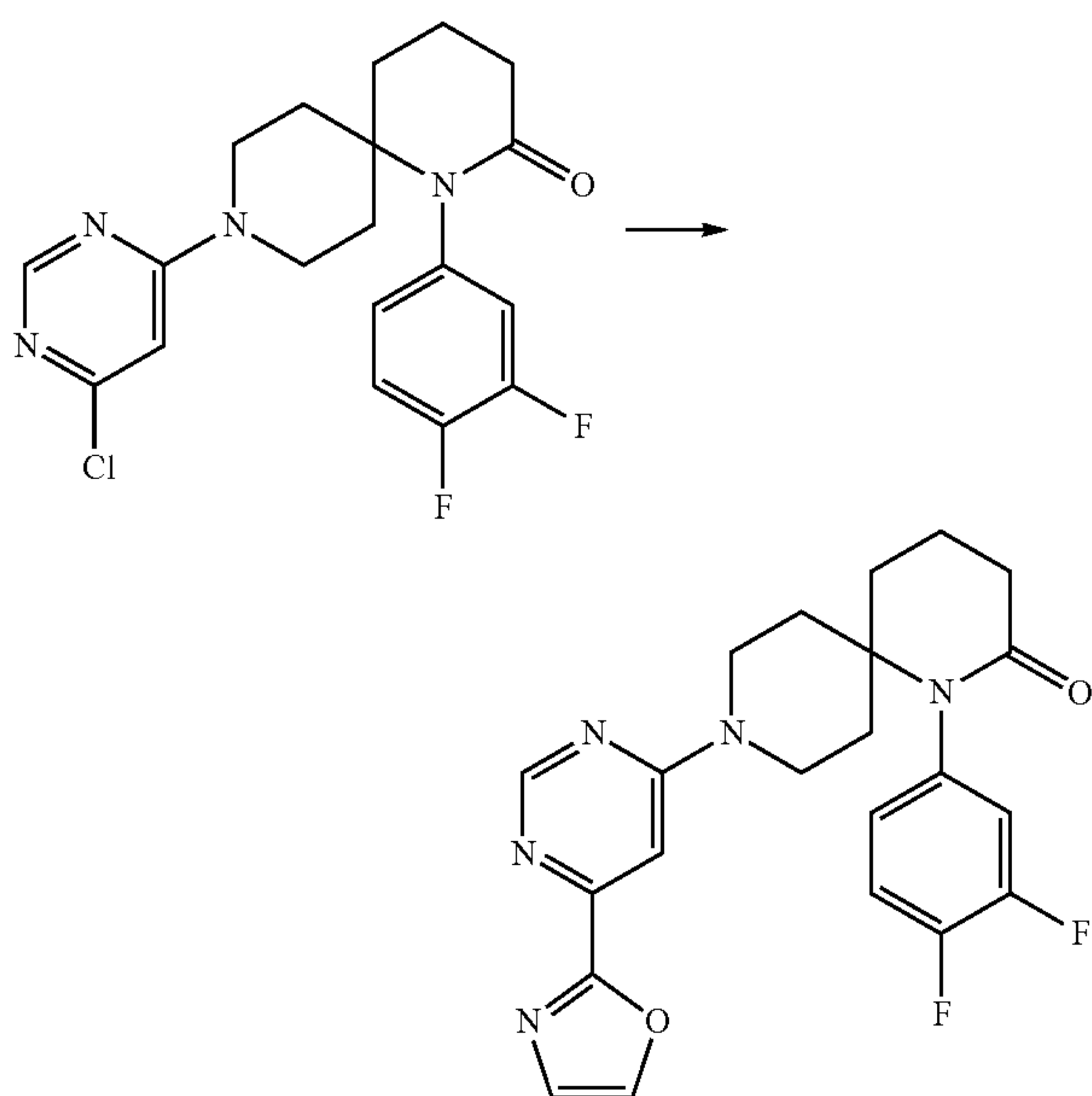
Example 63: 9-(6-amino-2-(pyridin-2-yl)pyrimidin-4-yl)-1-(3,4-difluorophenyl)-1,9-diazaspiro[5.5]undecan-2-one
