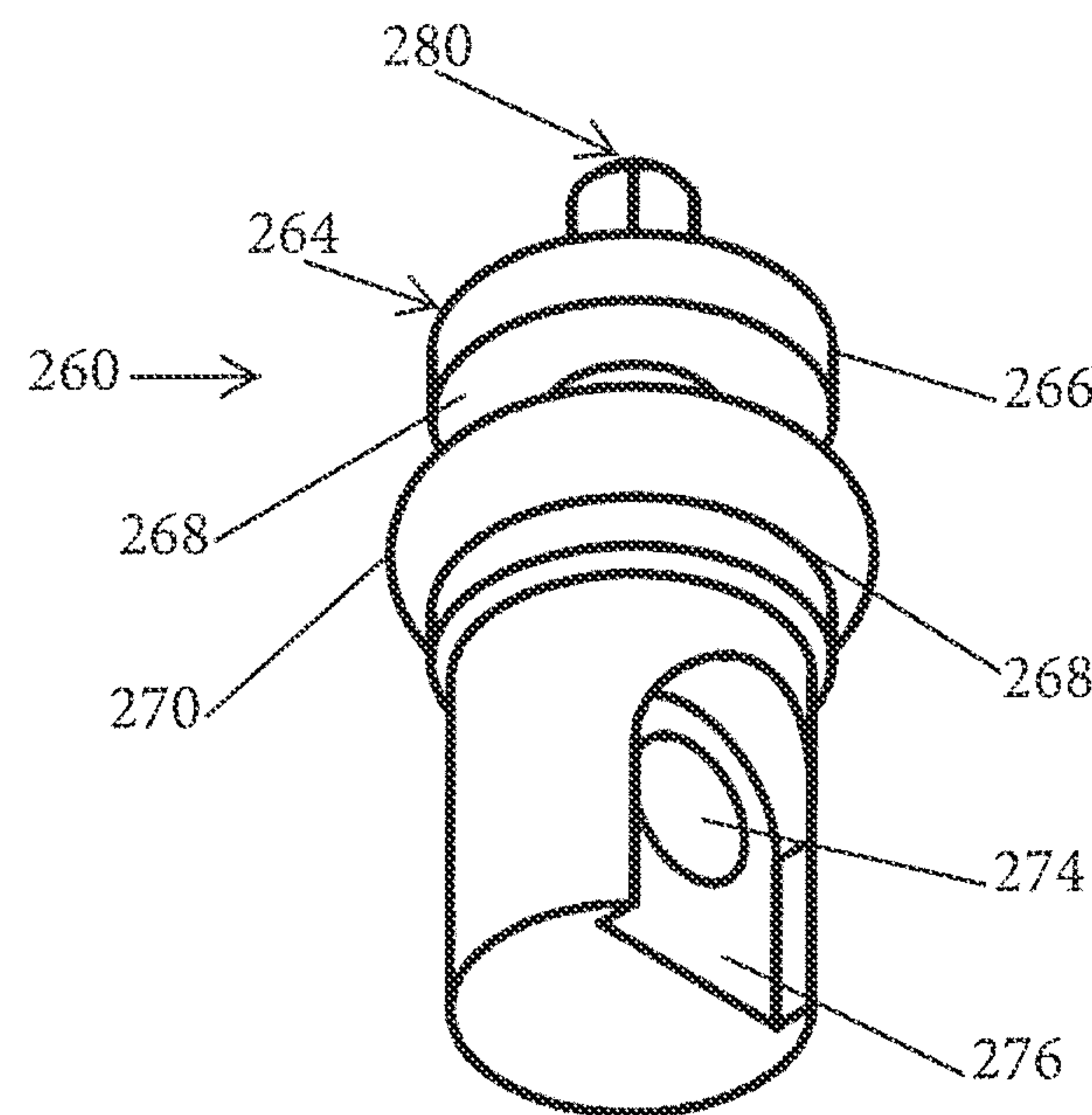
FIG. 20
