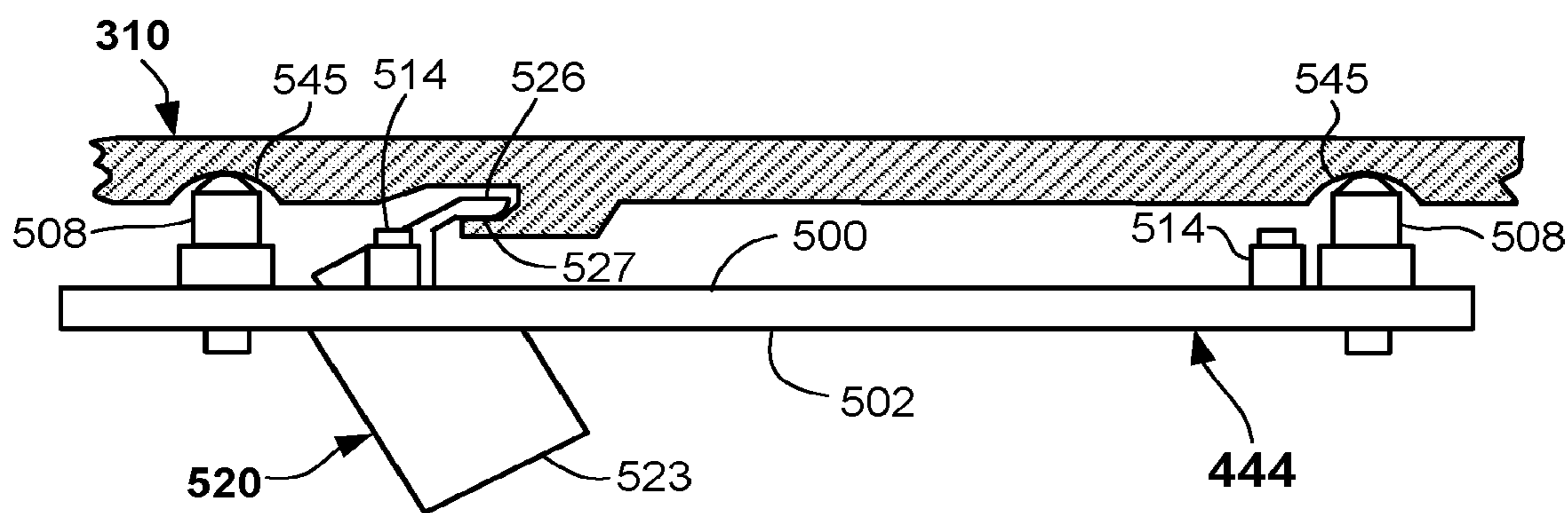
FIG. 5B
