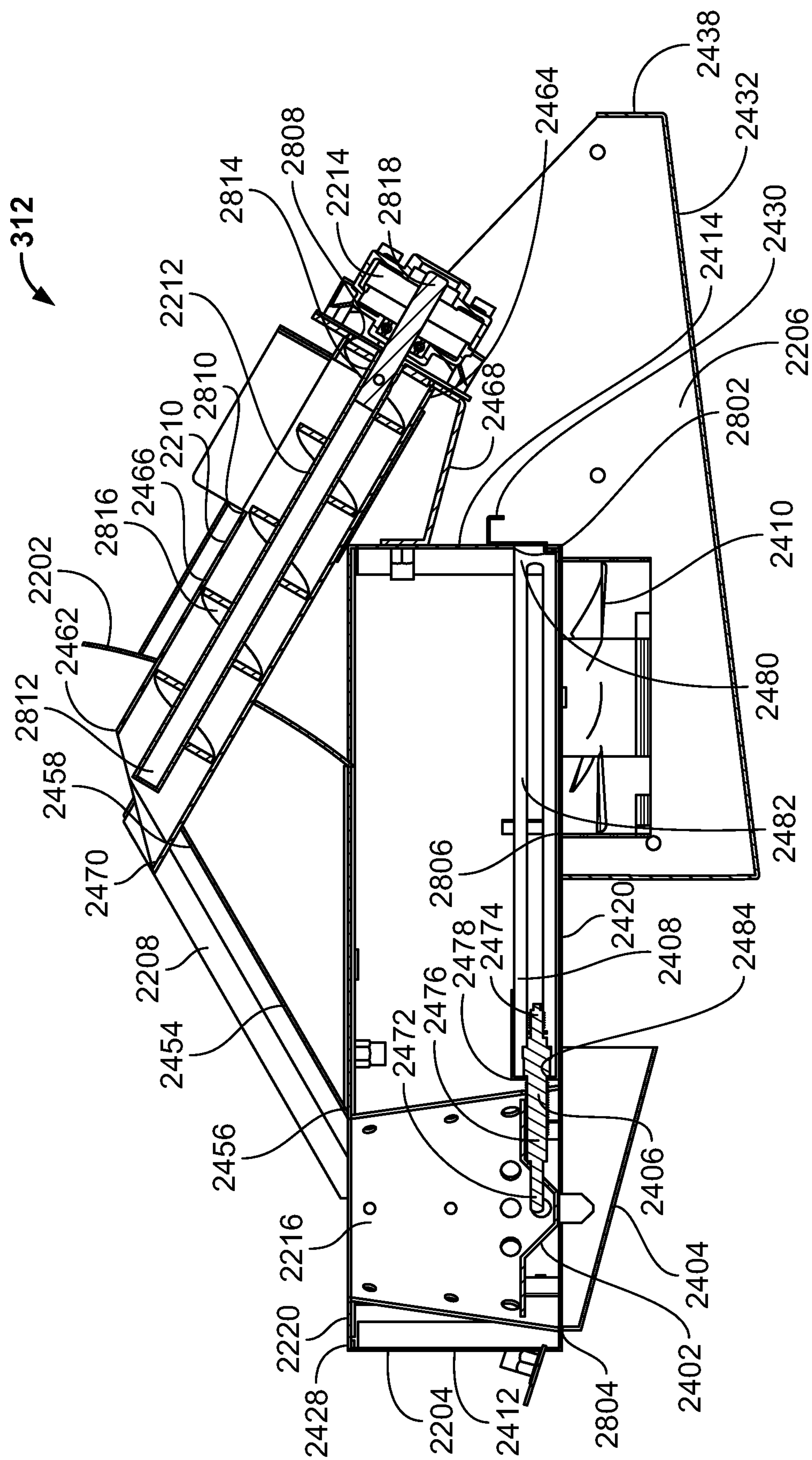
SECTION D-D
