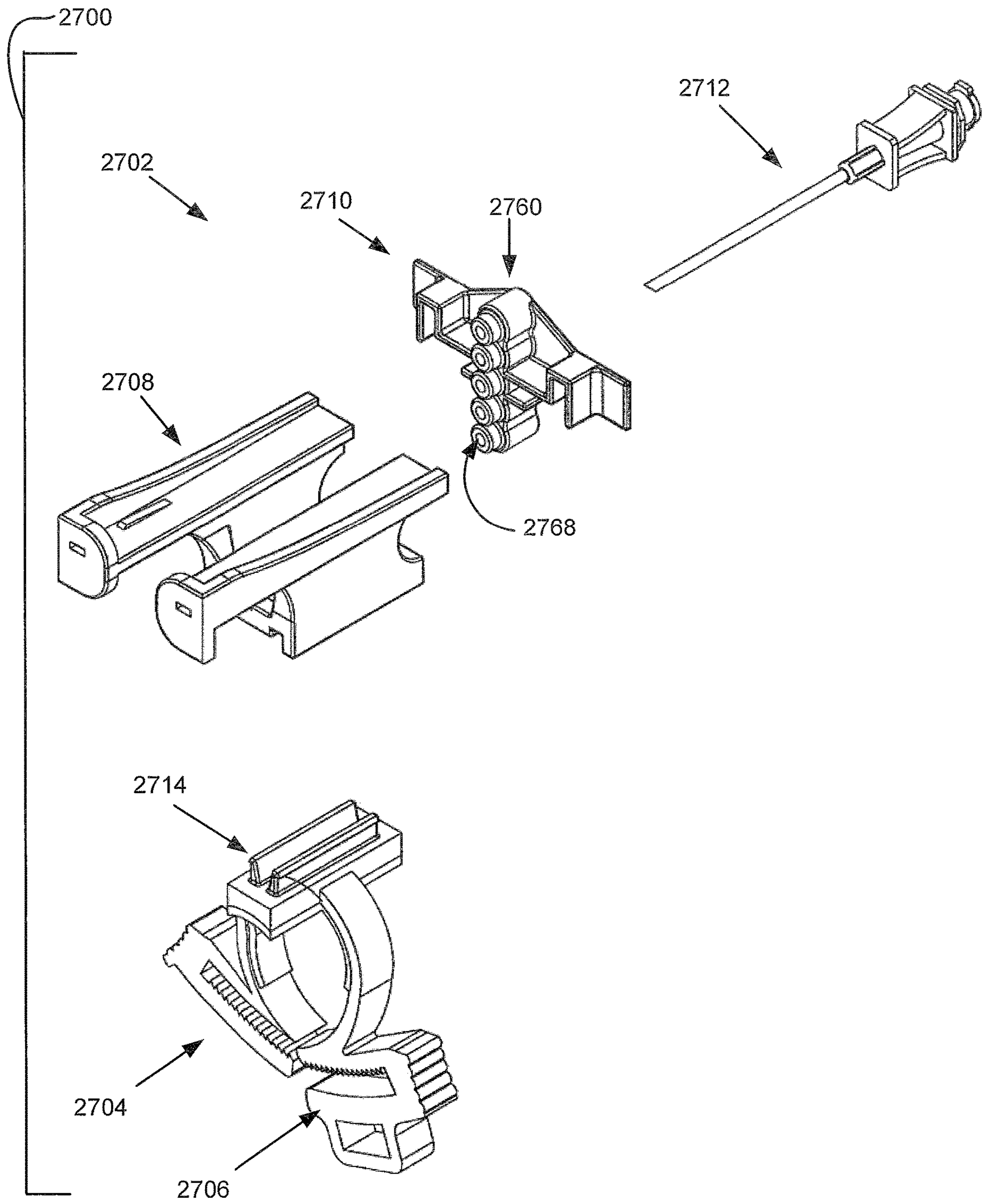
FIG. 30
