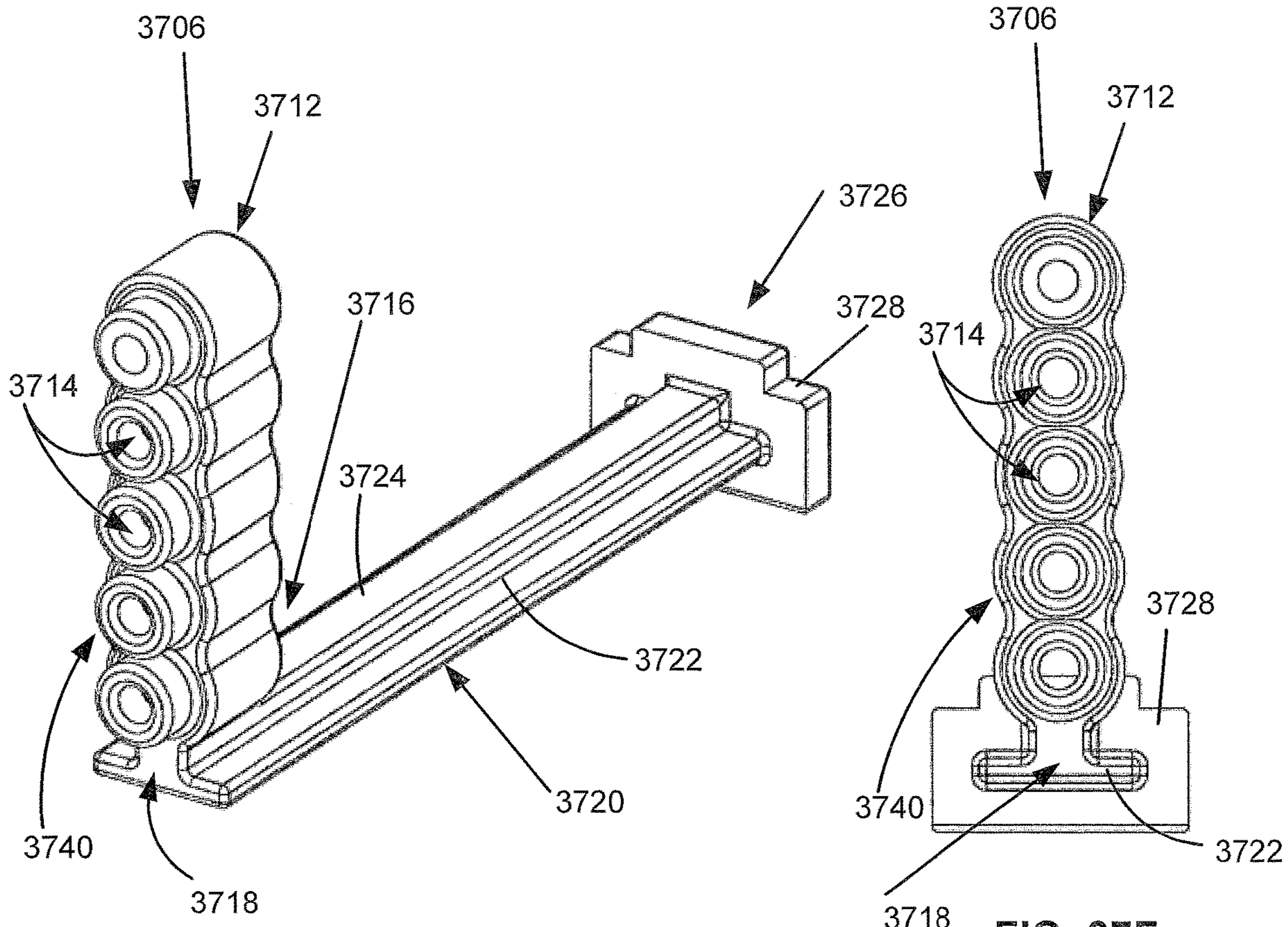
FIG. 37E
