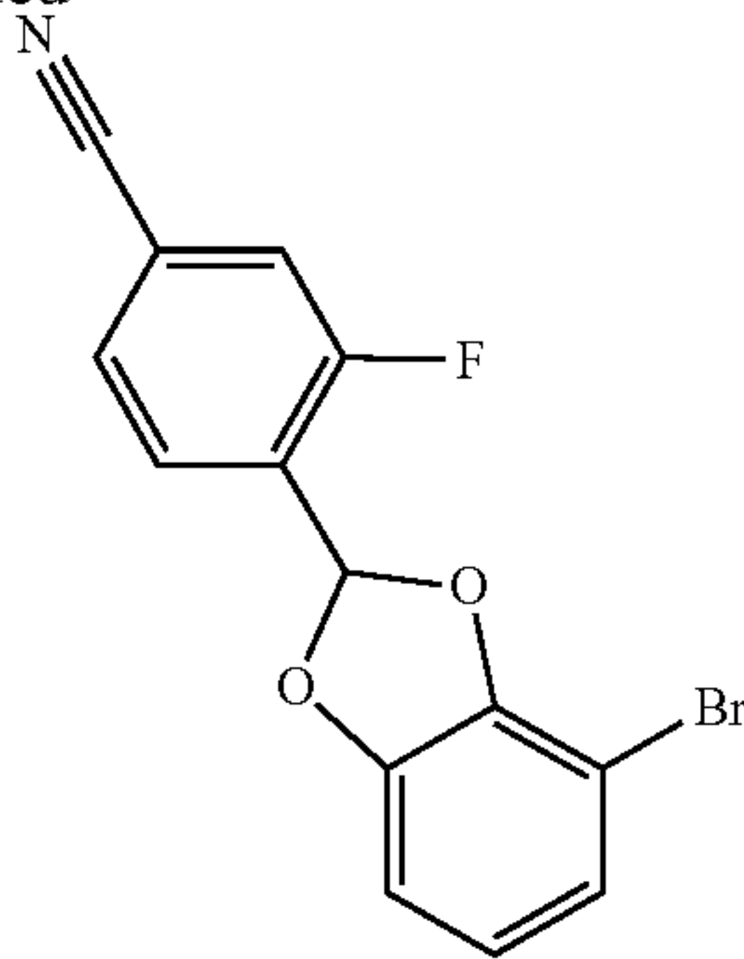
I-1
