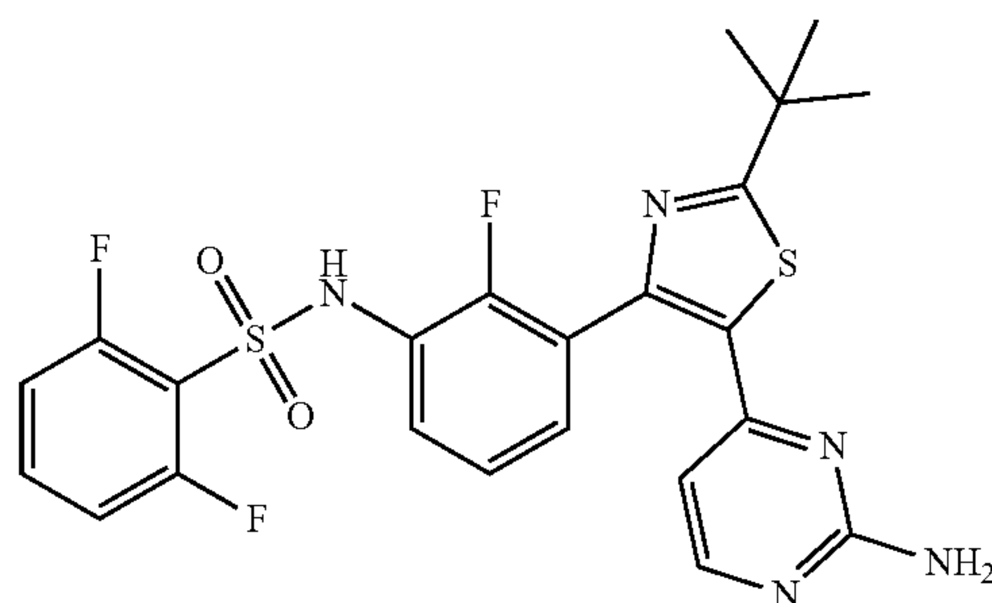
dabrafenib
