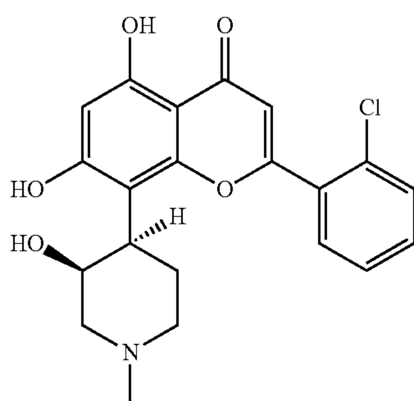
alvocidib
