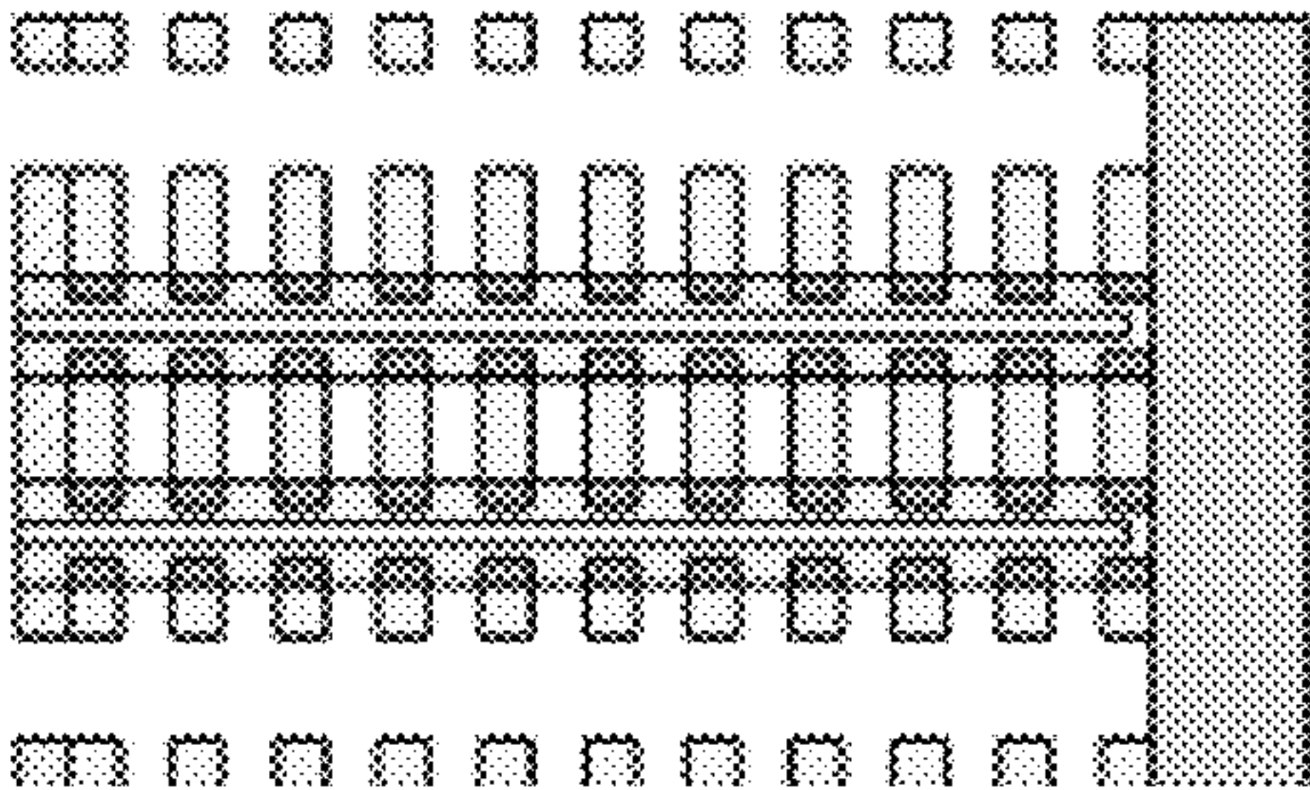
Fig. 4E Nitride removal
