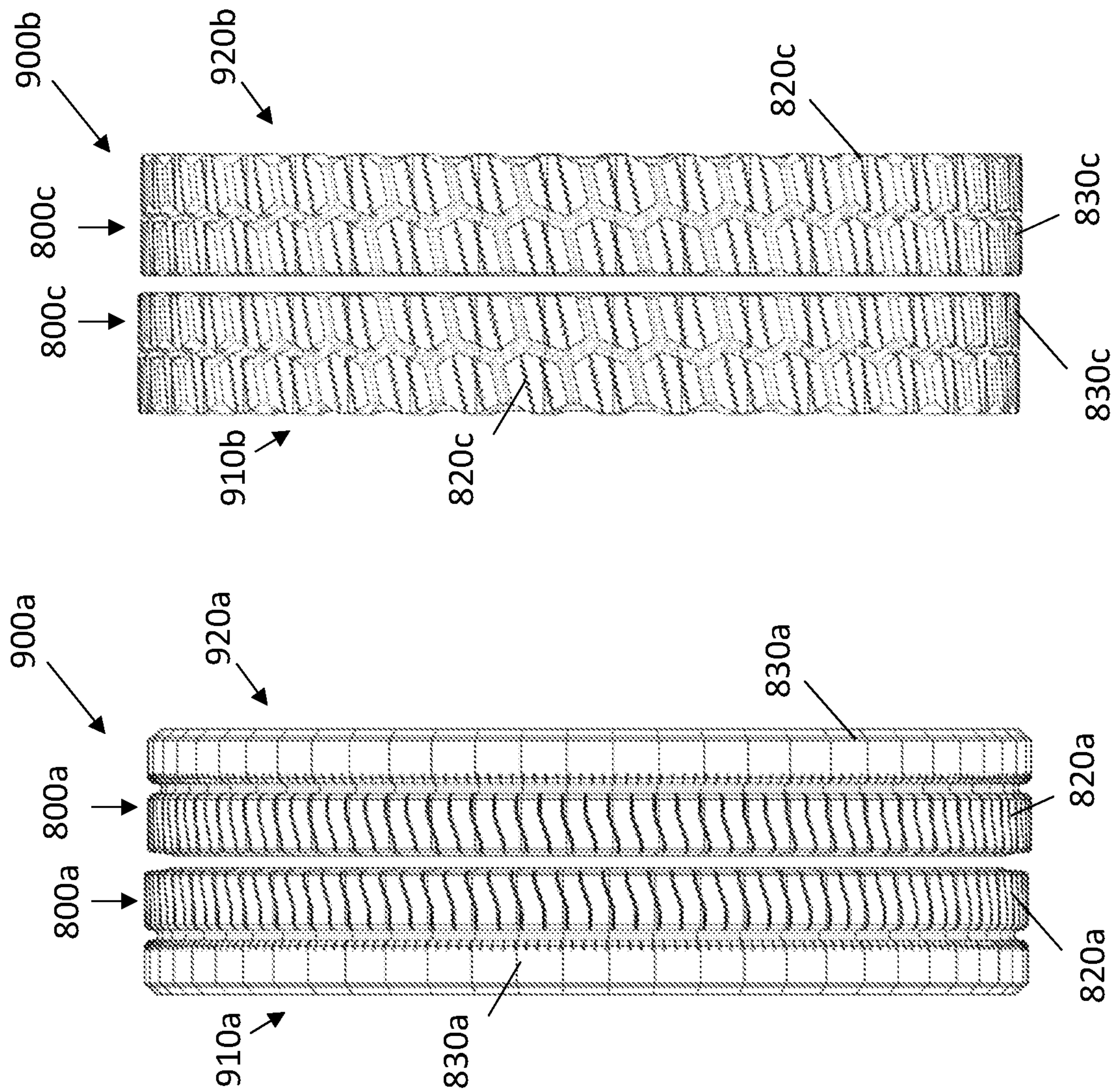
Fig. 9B
