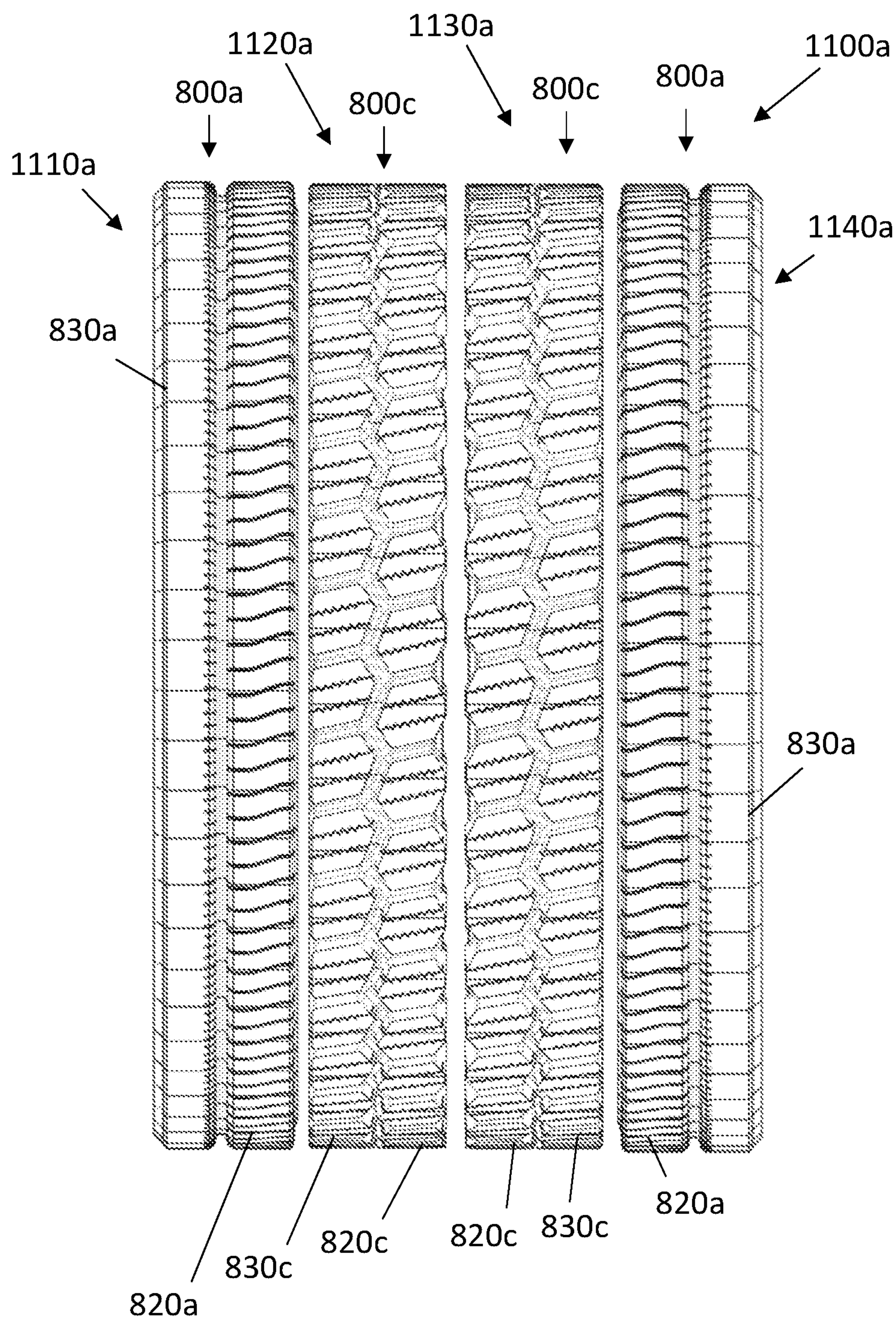
Fig. 11A
