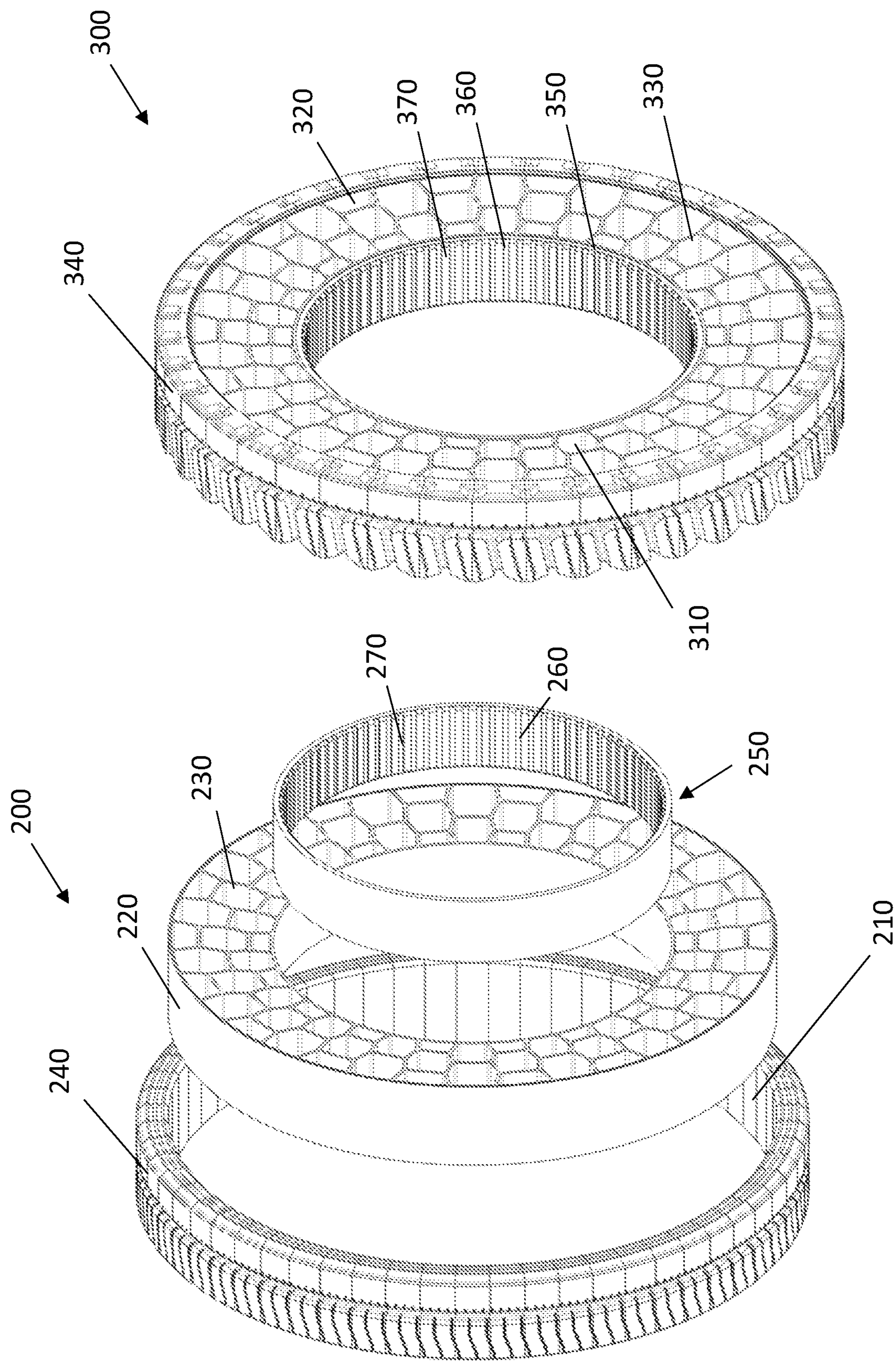
Fig. 4B
