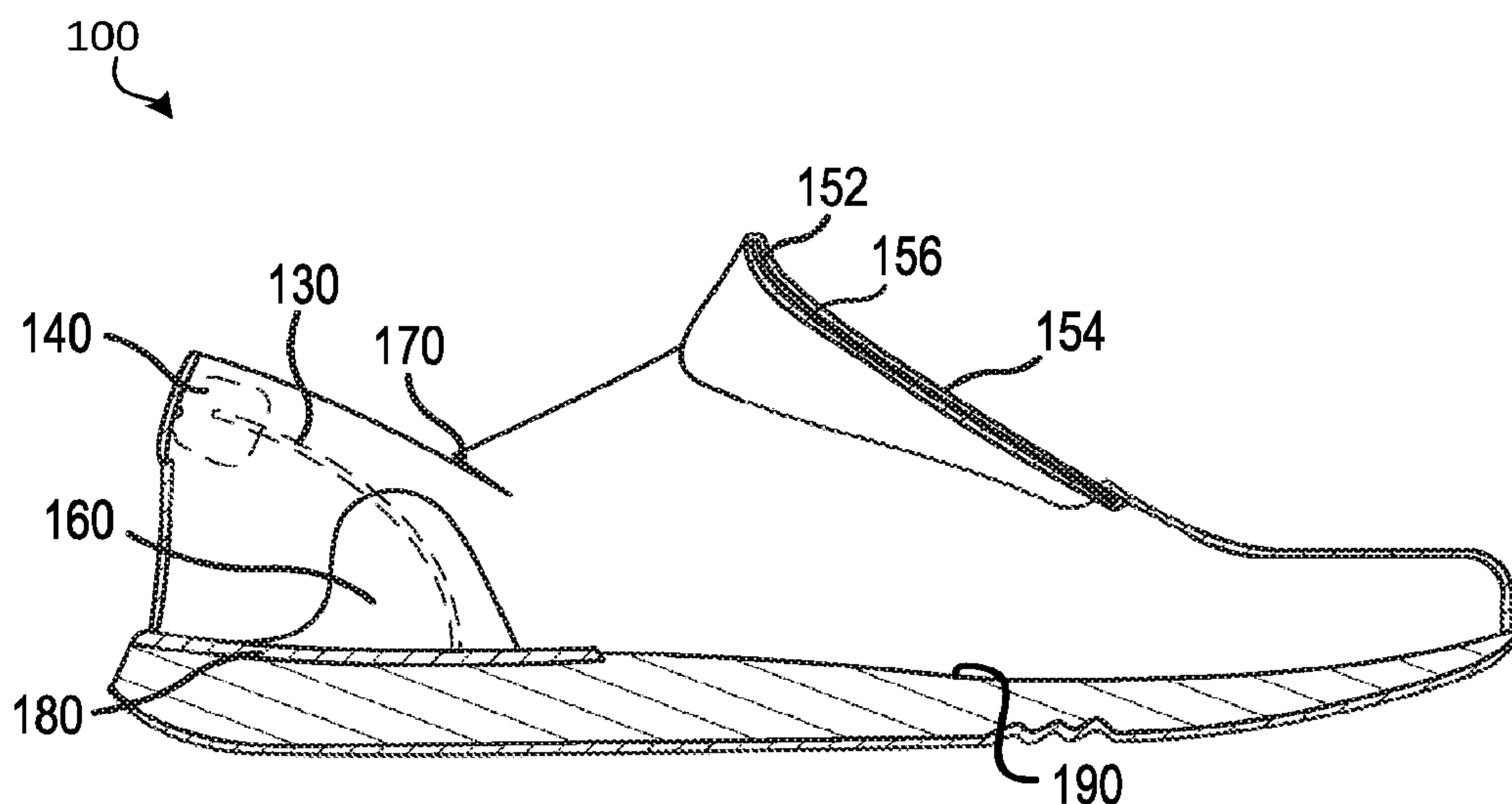
FIG. 6A
