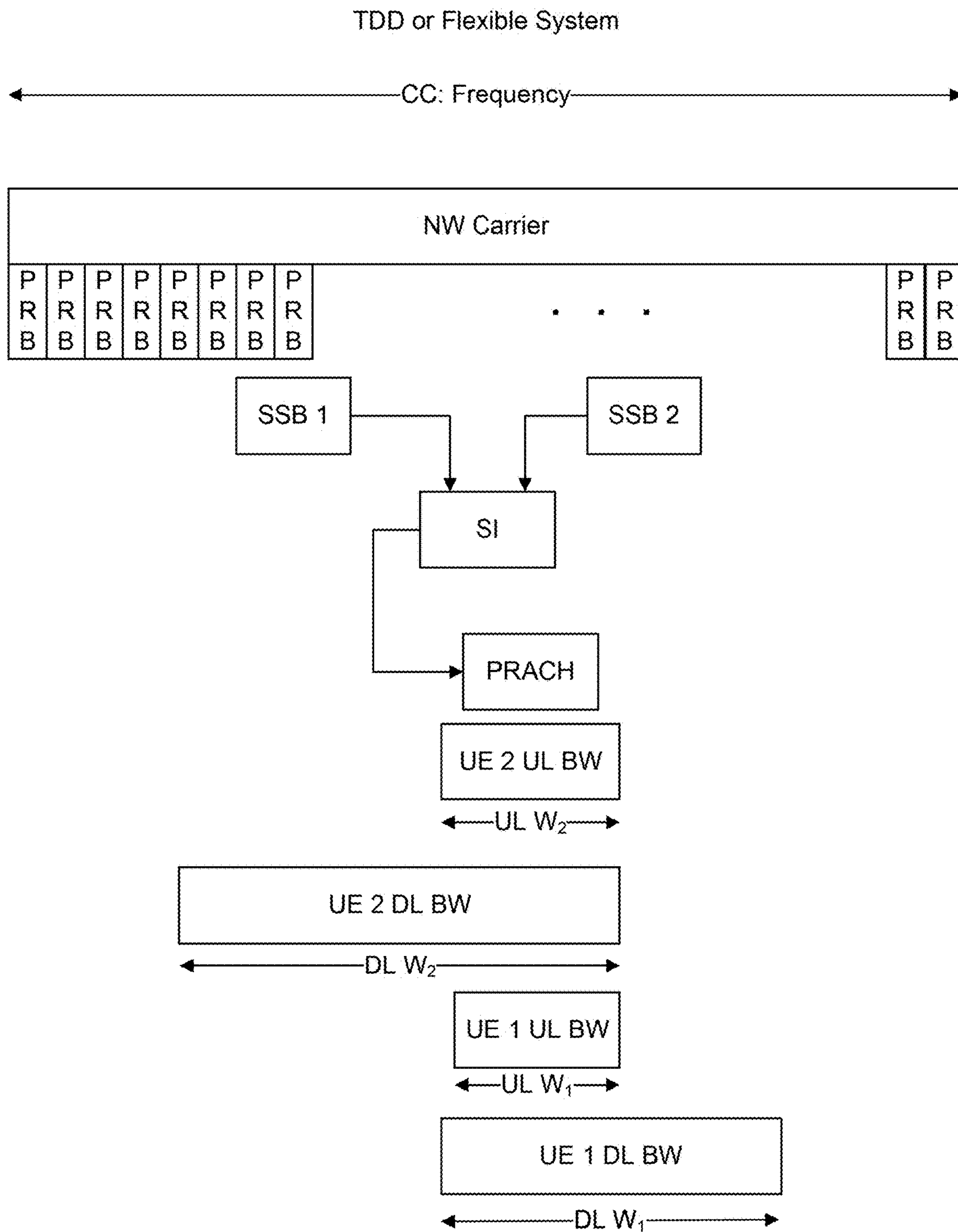
FIG. 16-A2
