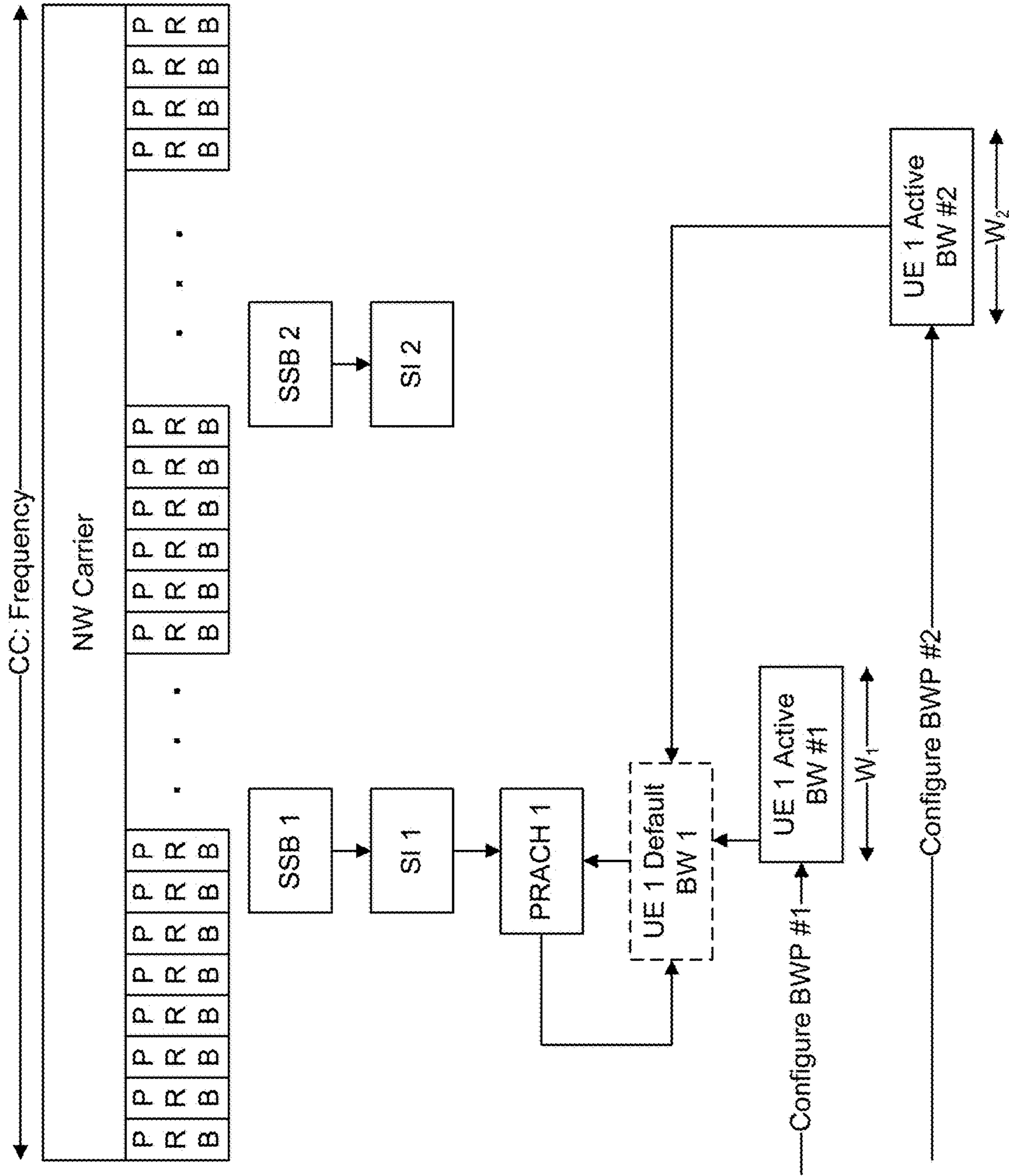
FIG. 28A
