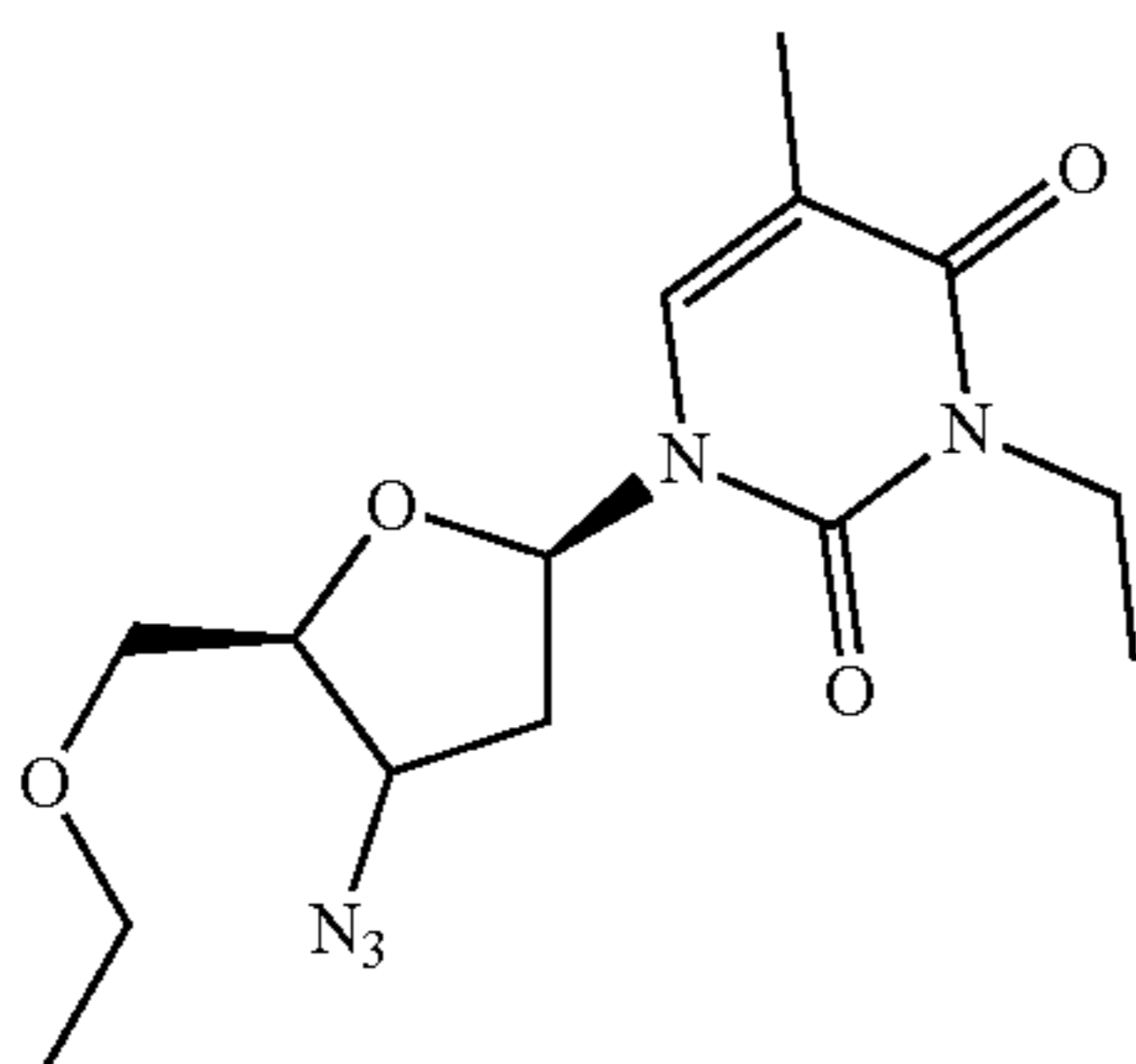
2-Et-AZT
