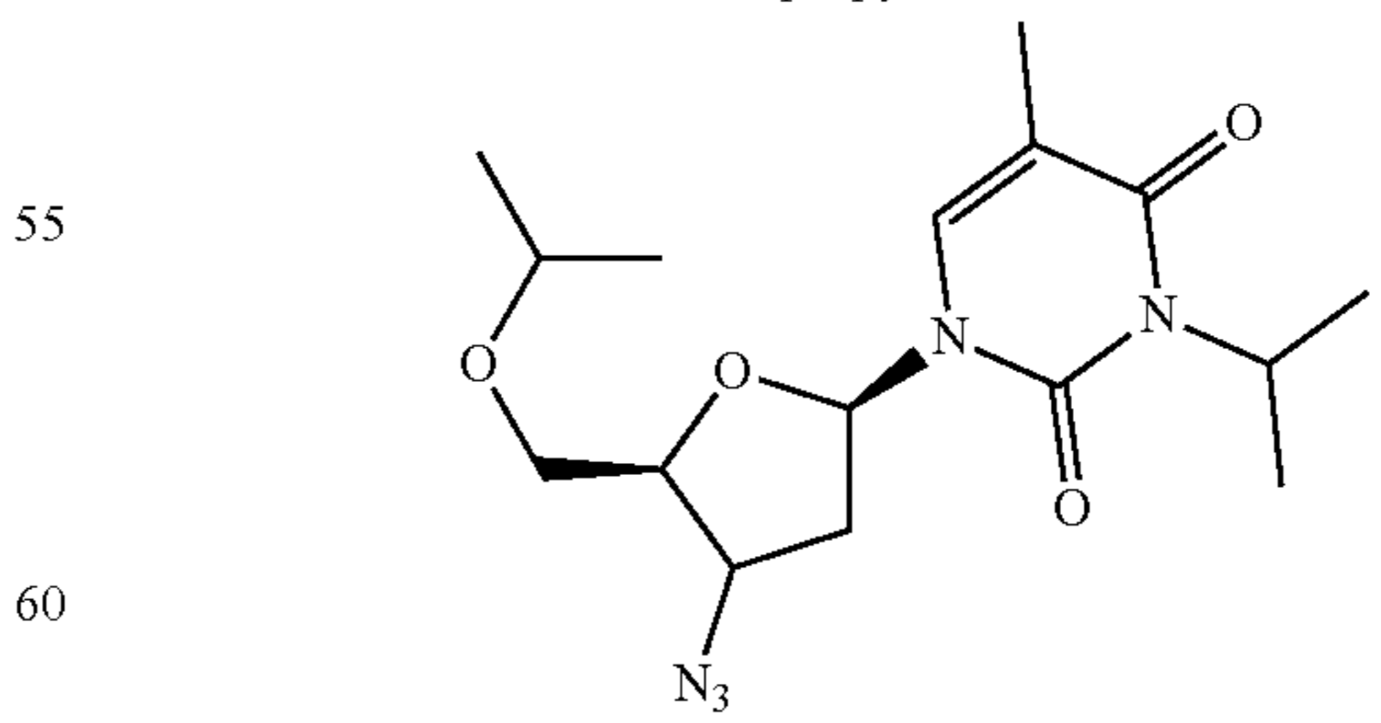
2-isopropyl-AZT
