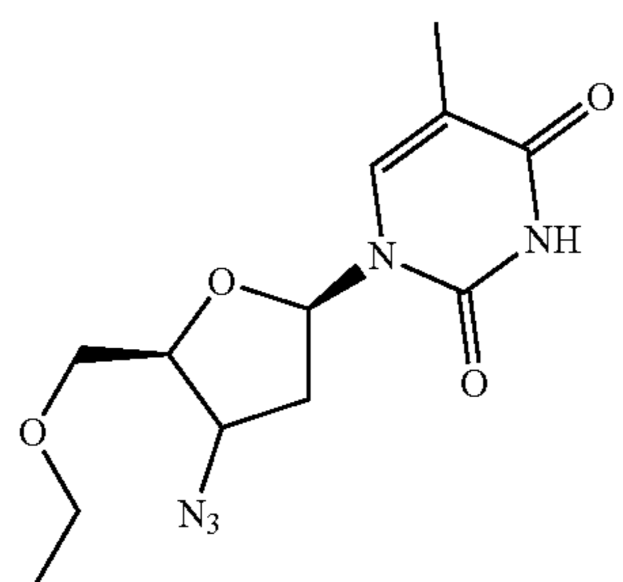
O-Et-AZT
