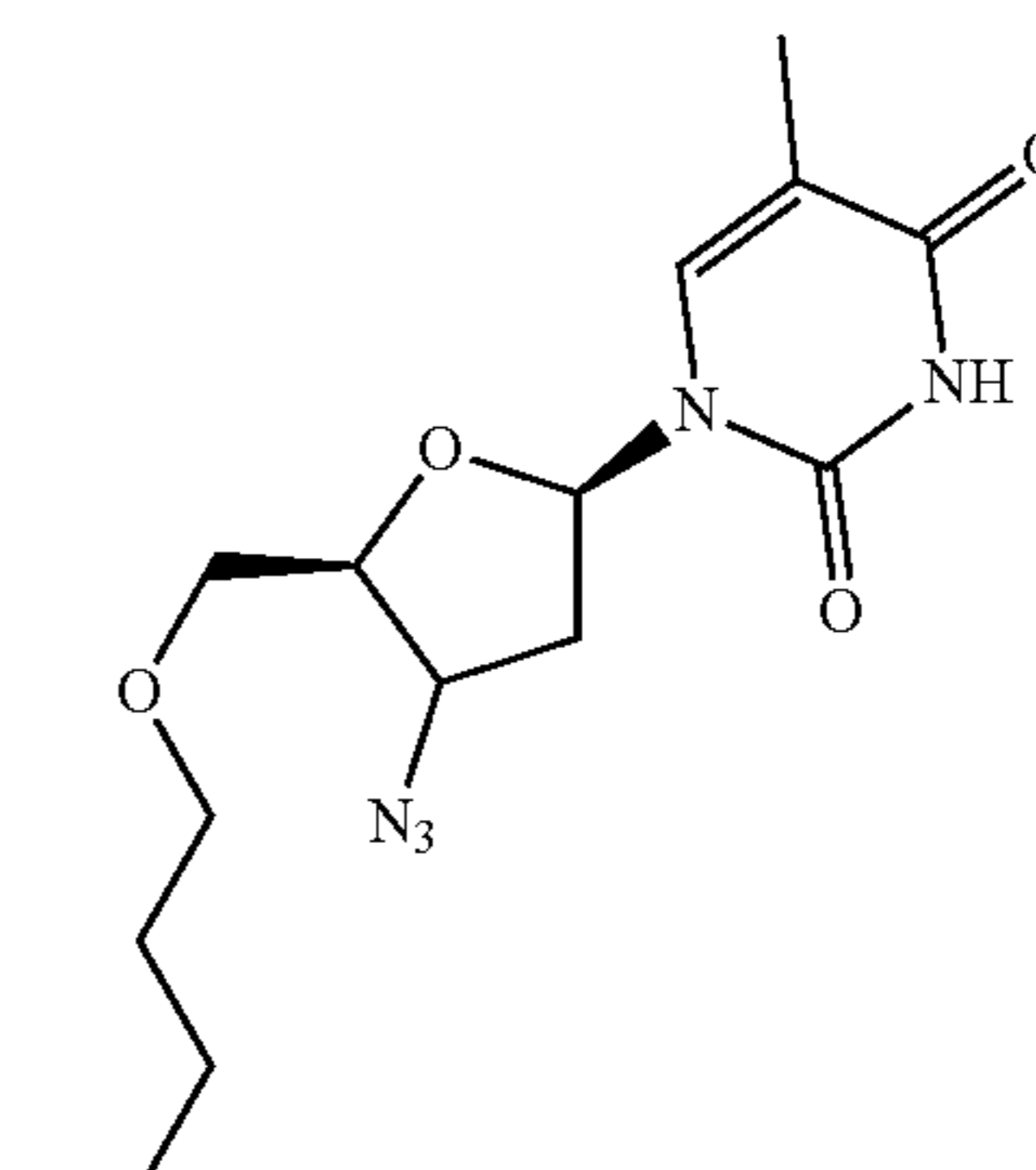
O-Butyl-AZT
