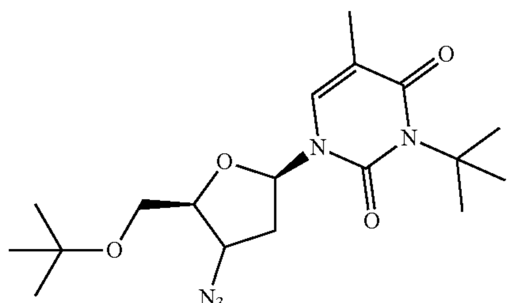
2-tert-butyl-AZT
