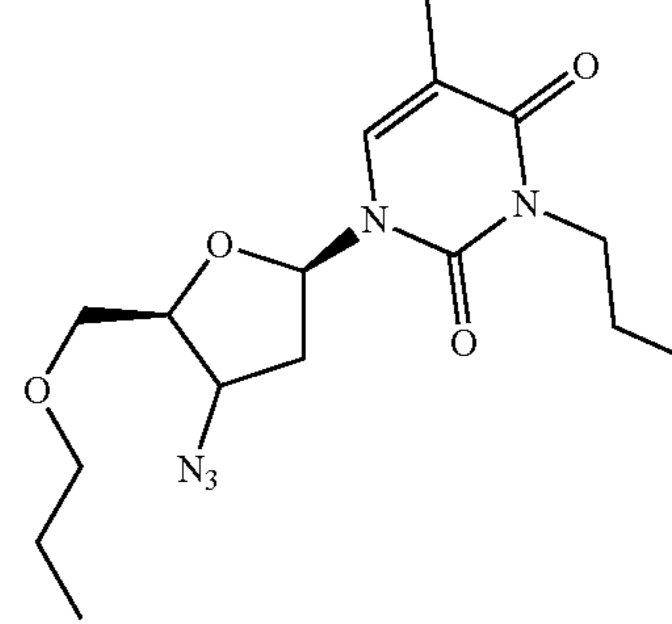
2-Propyl-AZT
