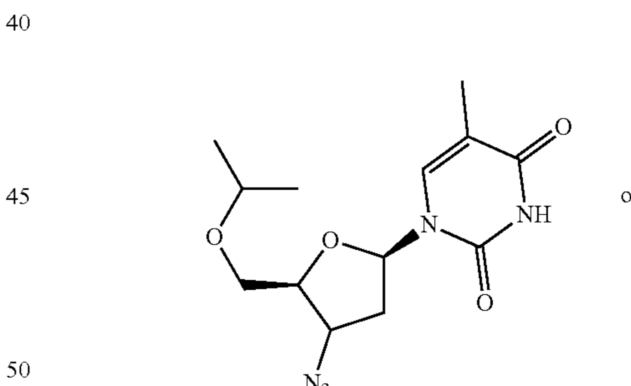
O-isopropyl-AZT
