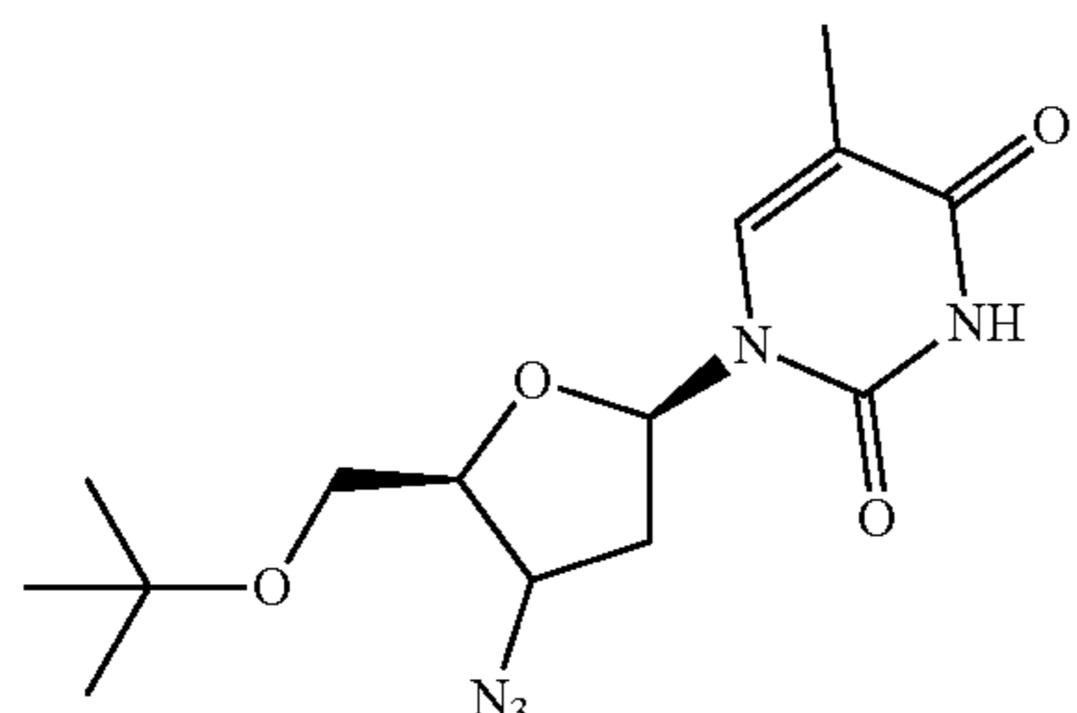
O-tert-butyl-AZT
