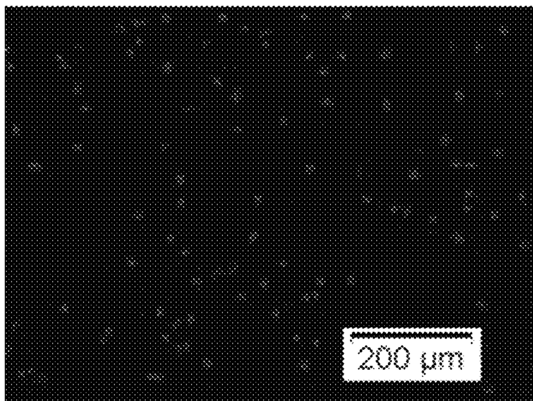
pUC19
