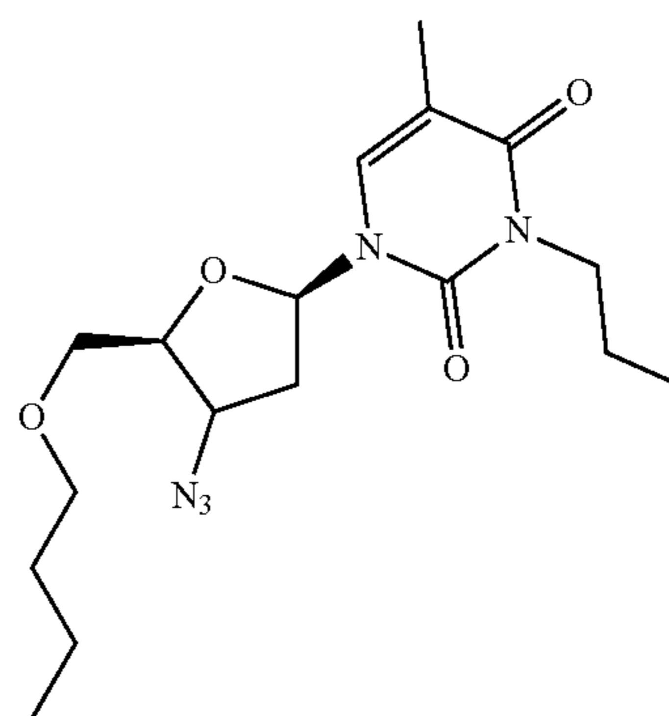
2-Butyl-AZT
