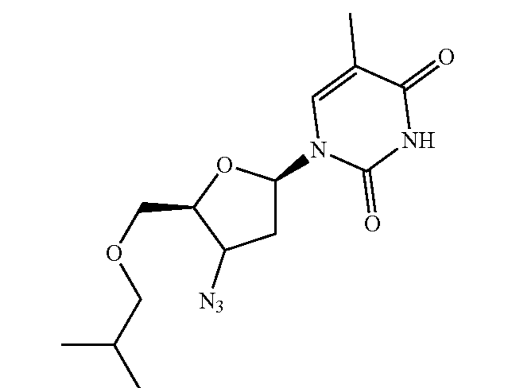
O-isobutyl-AZT
