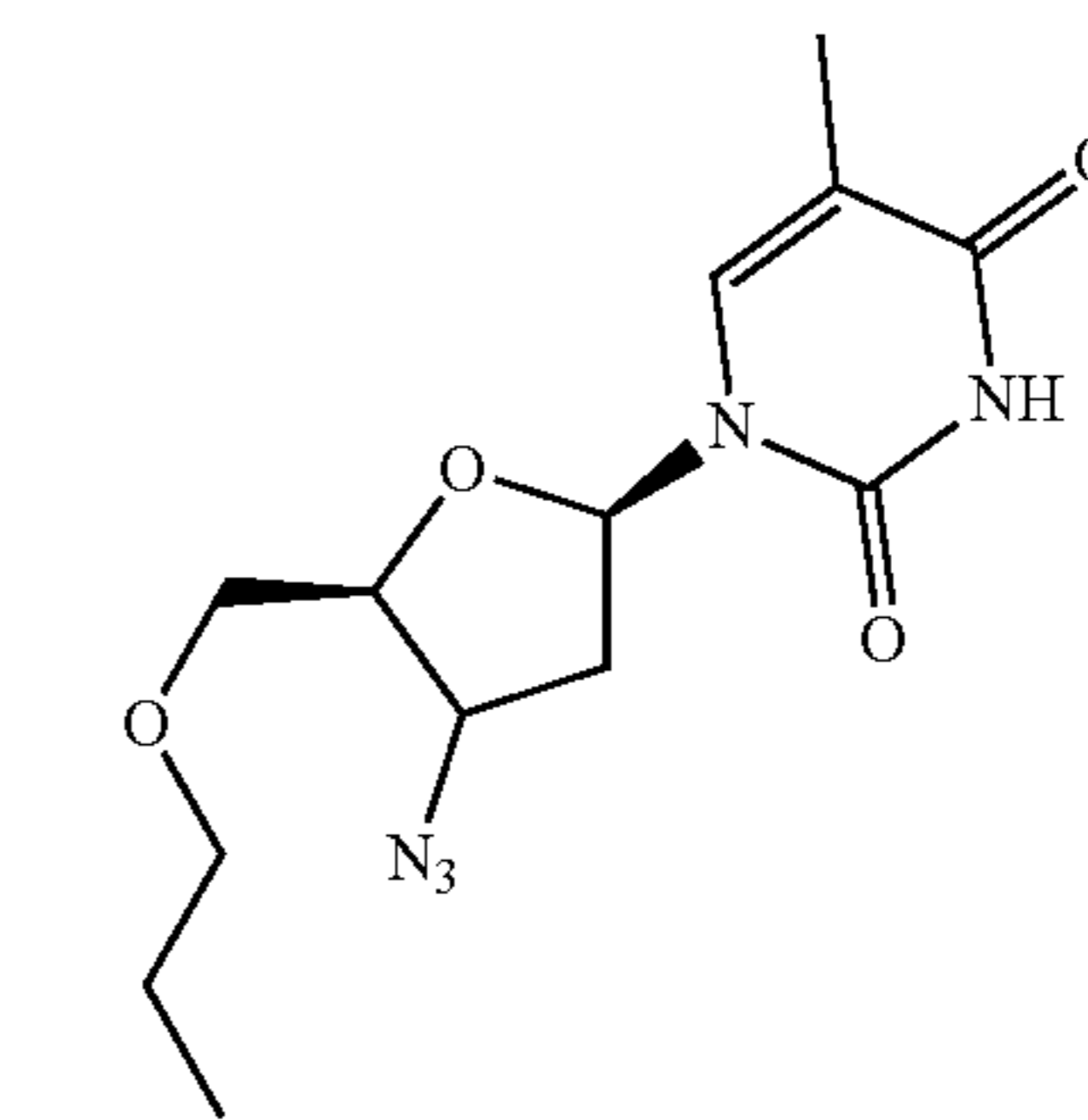
O-Propyl-AZT
