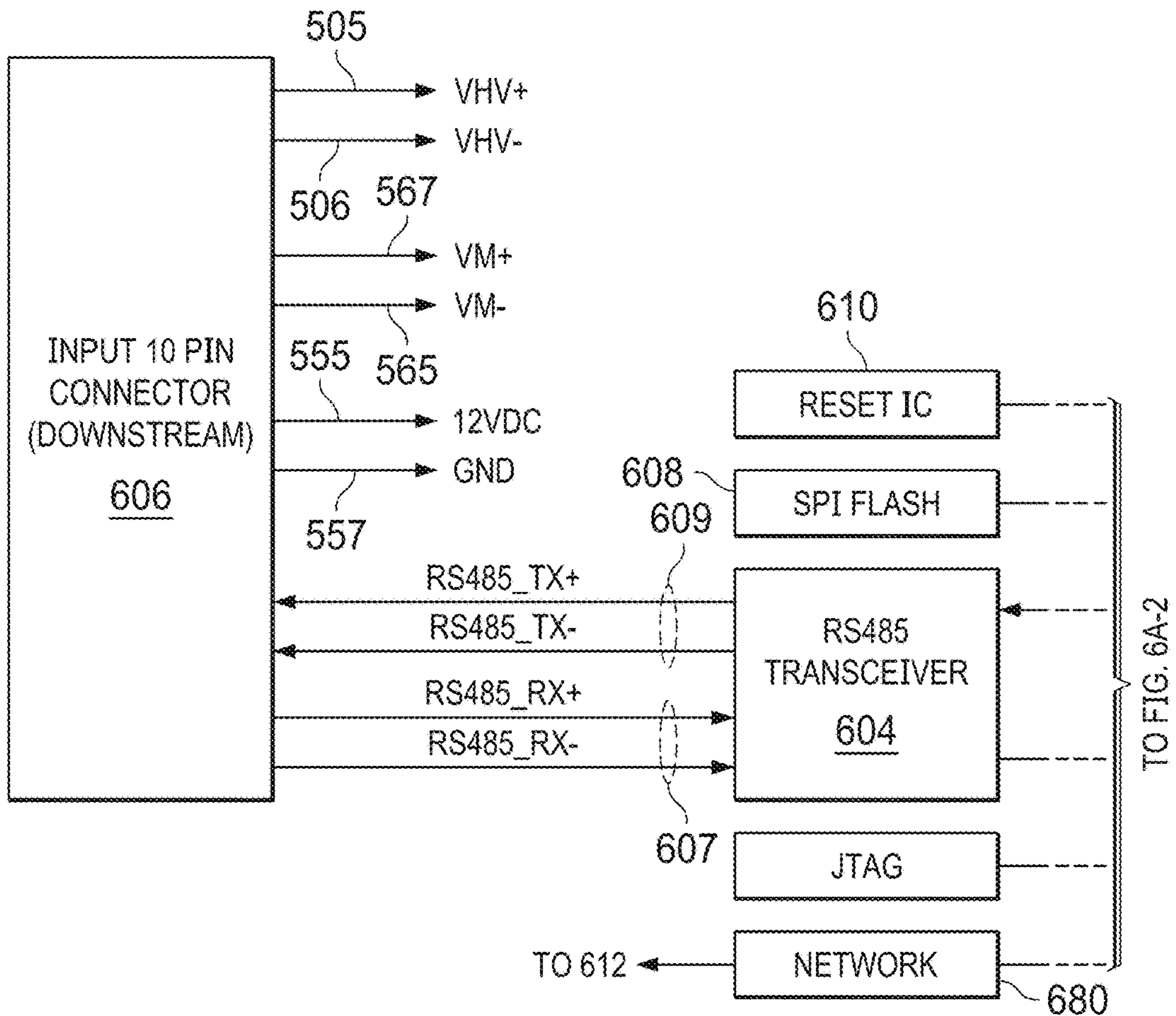
FIG. 6A-1
