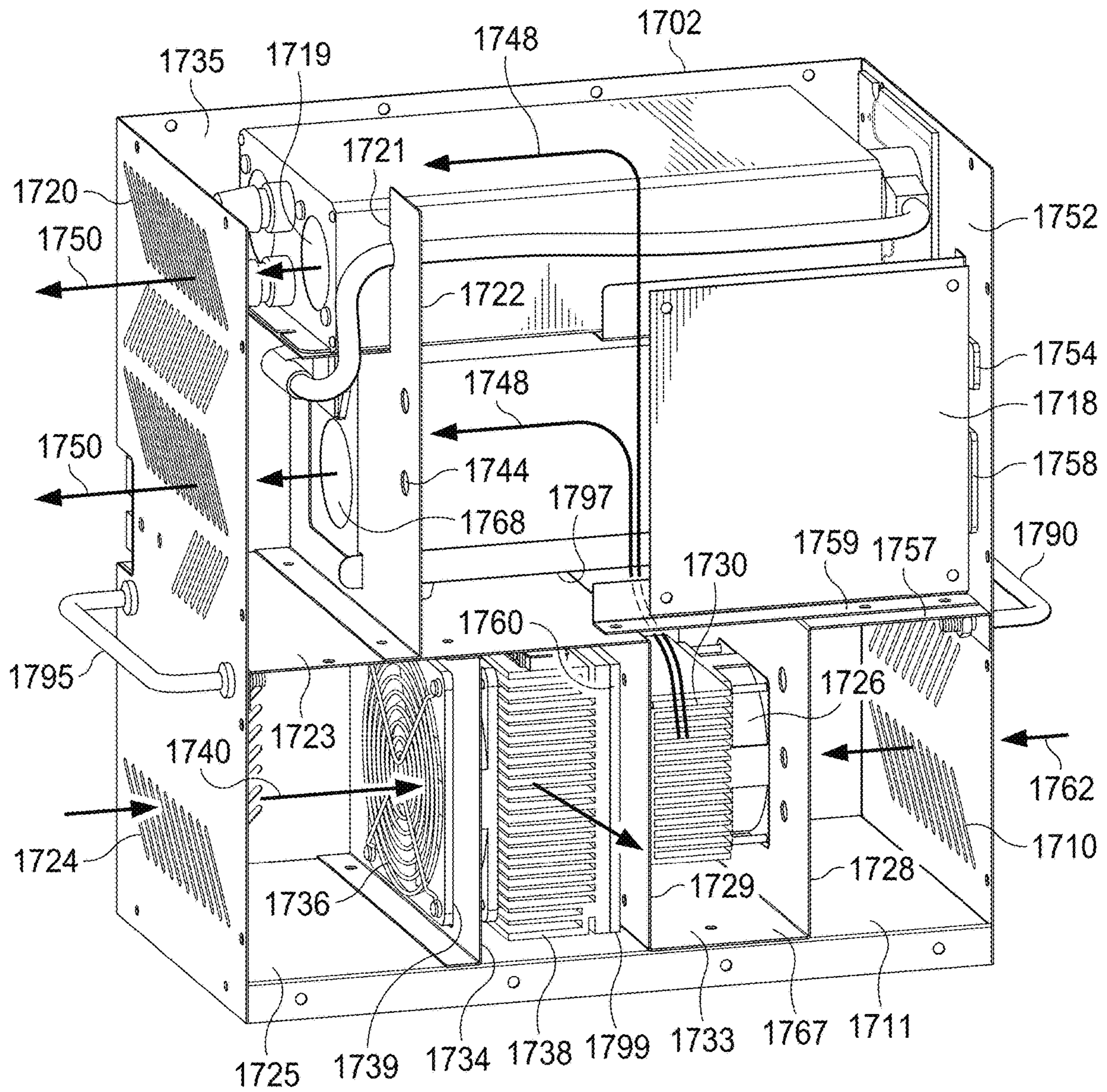
FIG. 17C
