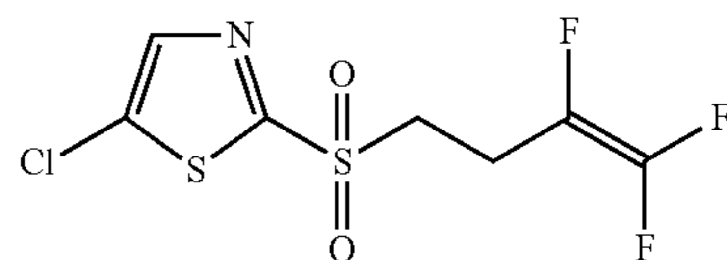
fluensulfone
