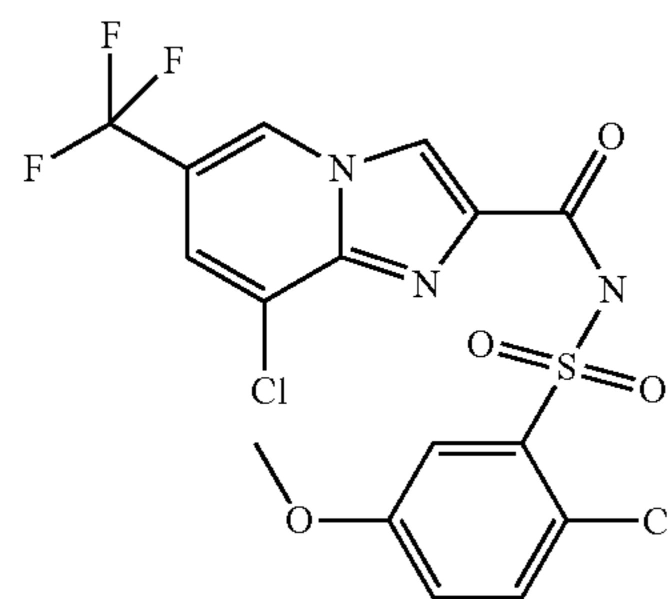
fluazaindolizin
