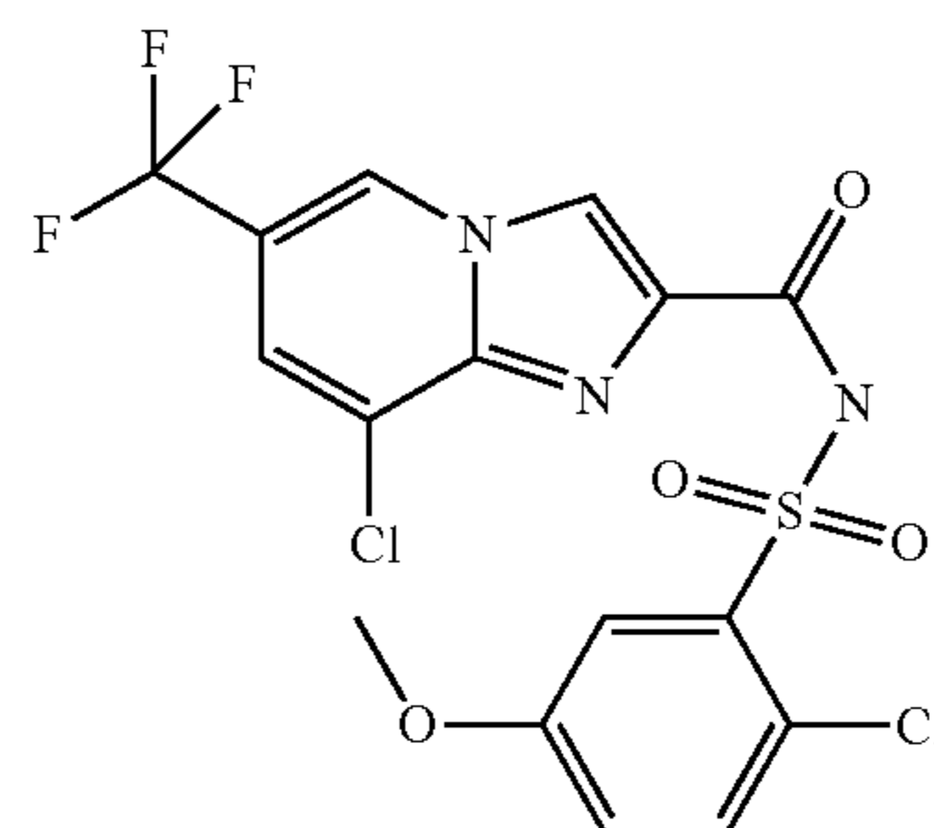
fluazaindolizin
