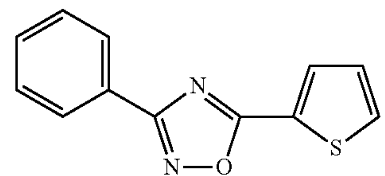
tioxazafen
