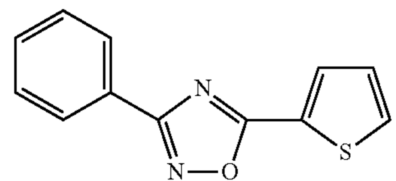
tioxazafen
