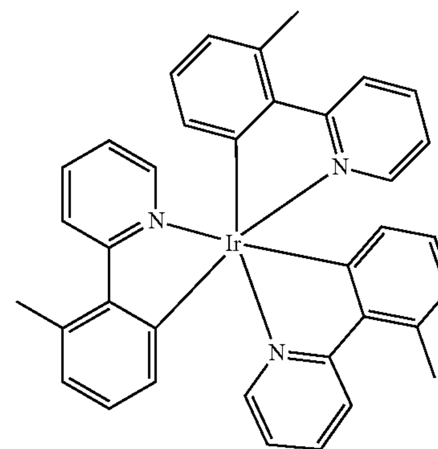
Dopant 1
