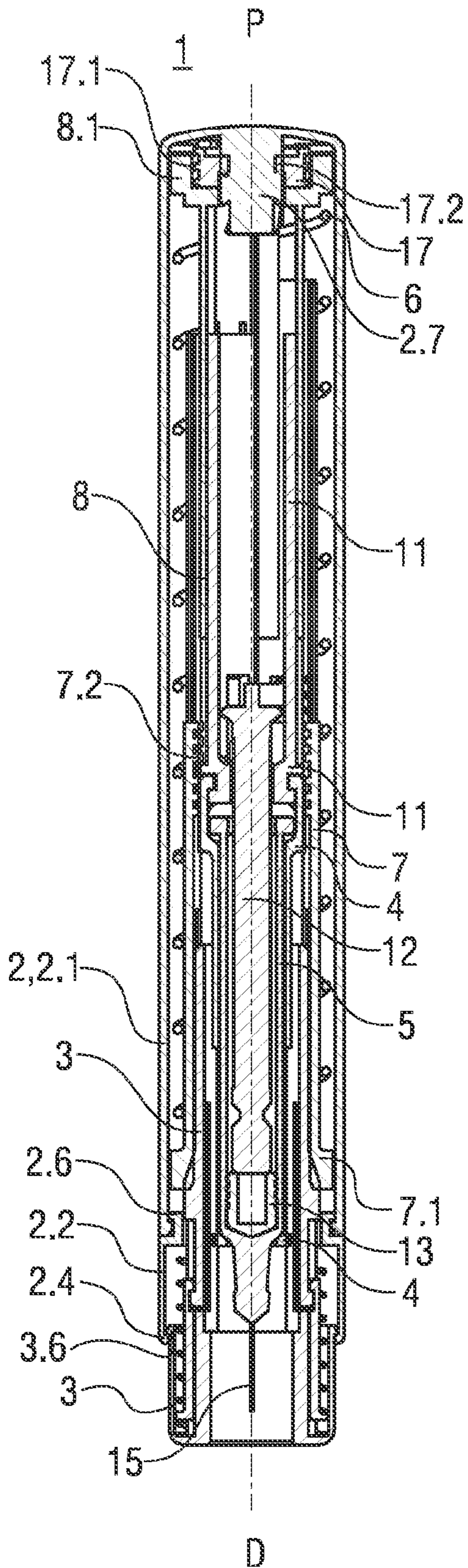
FIG 10A
