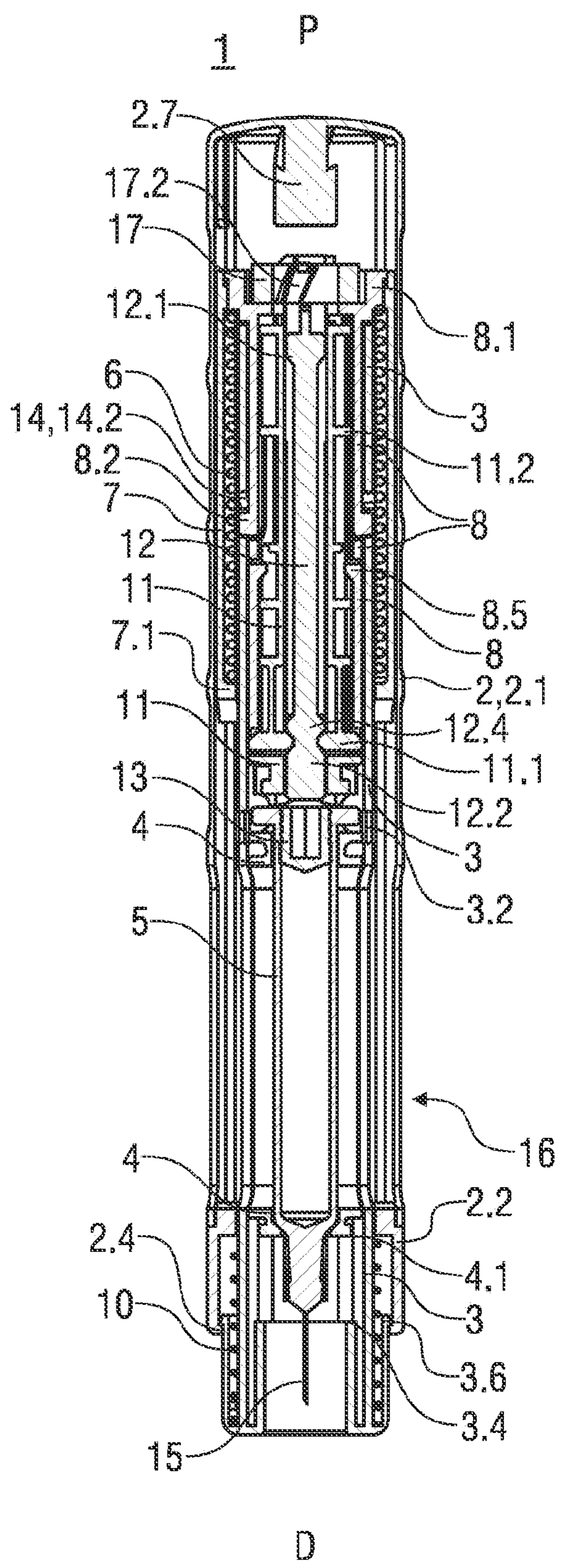
FIG 1B
