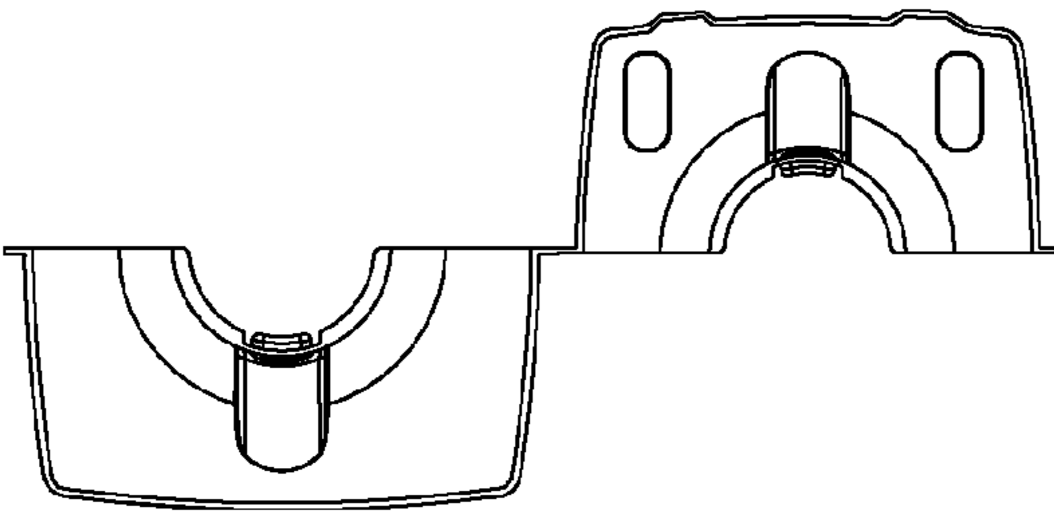
Section B-B FIG. 29F
