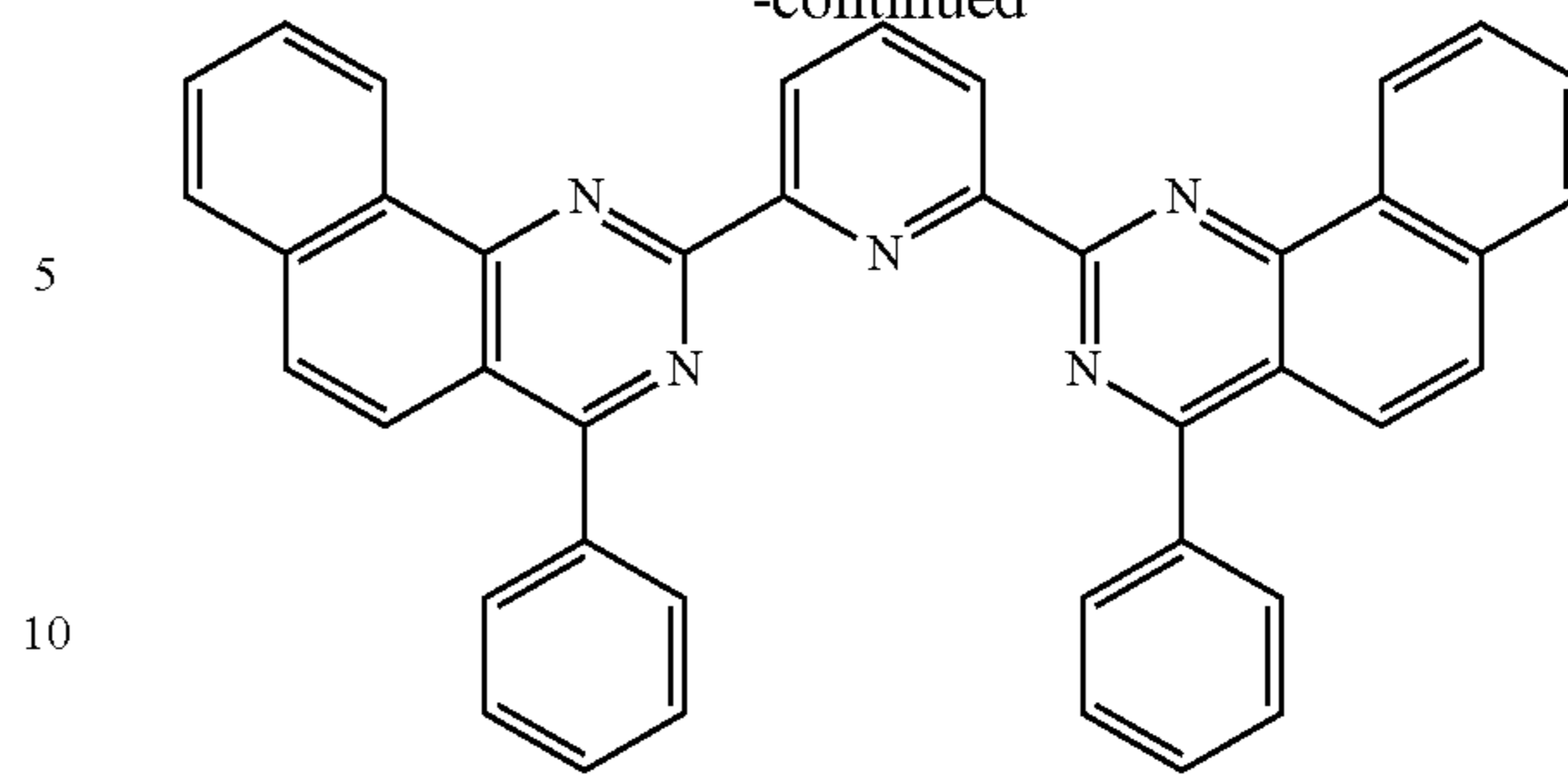
2,6(P-Bqn)2Py
