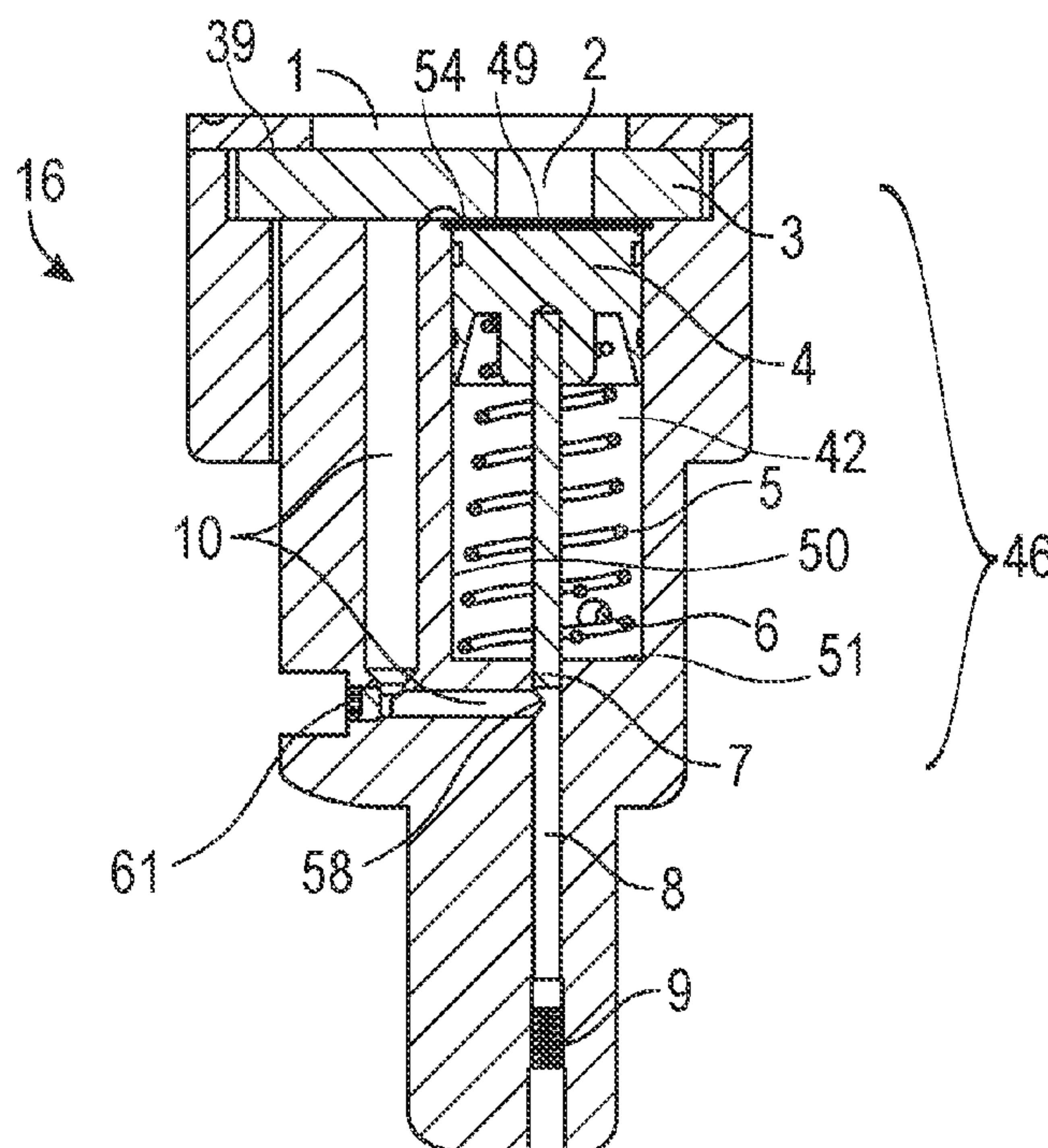
Section A-A
