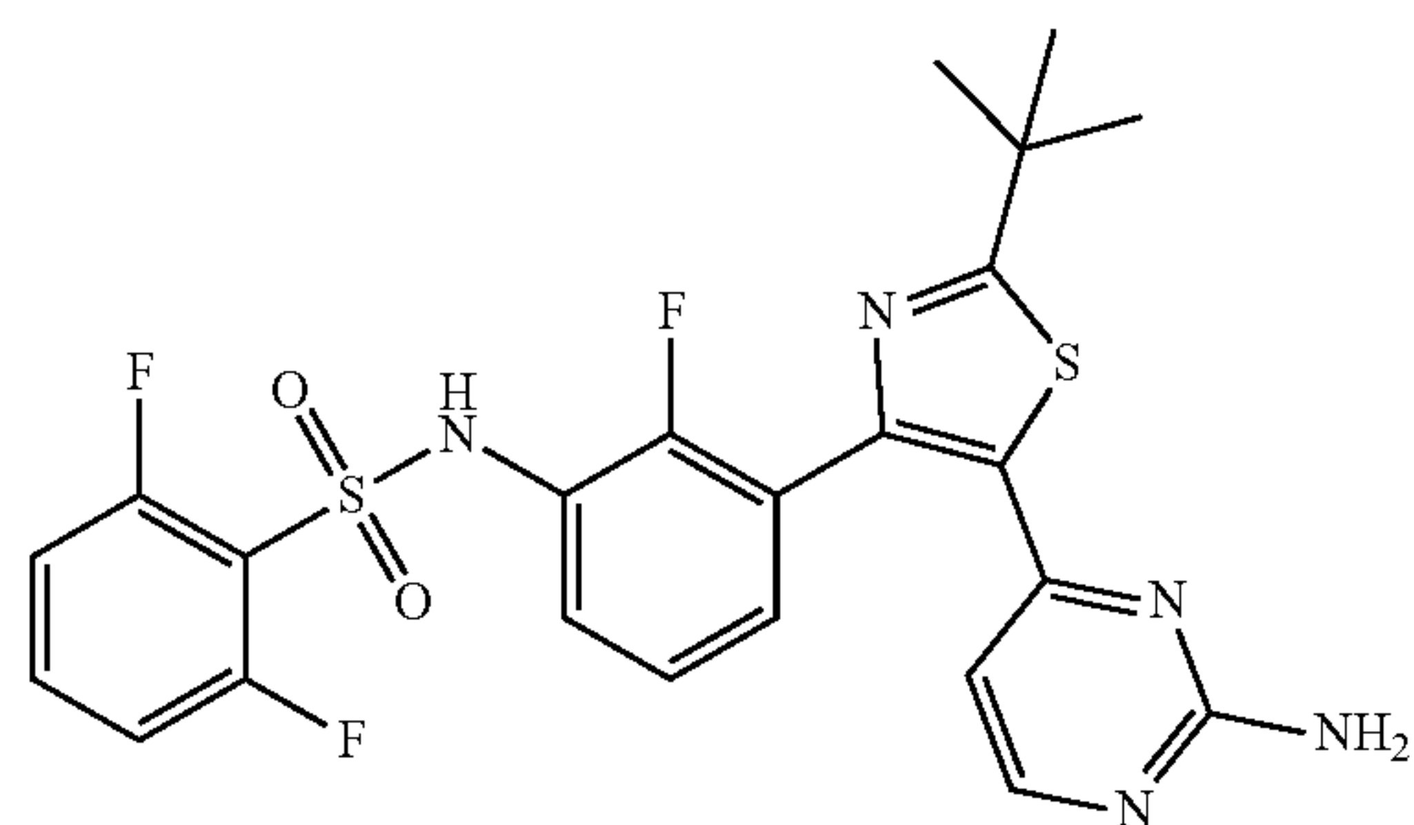
dabrafenib
