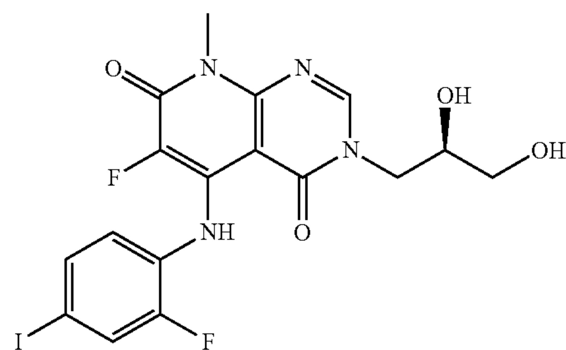
TAK-733
