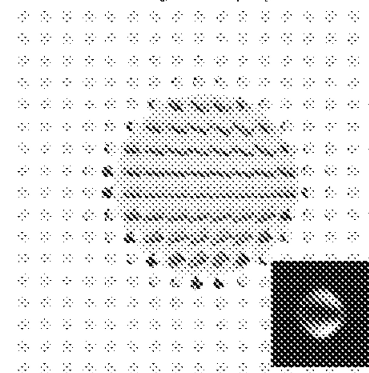
FIG. 1E Boojum (B)
