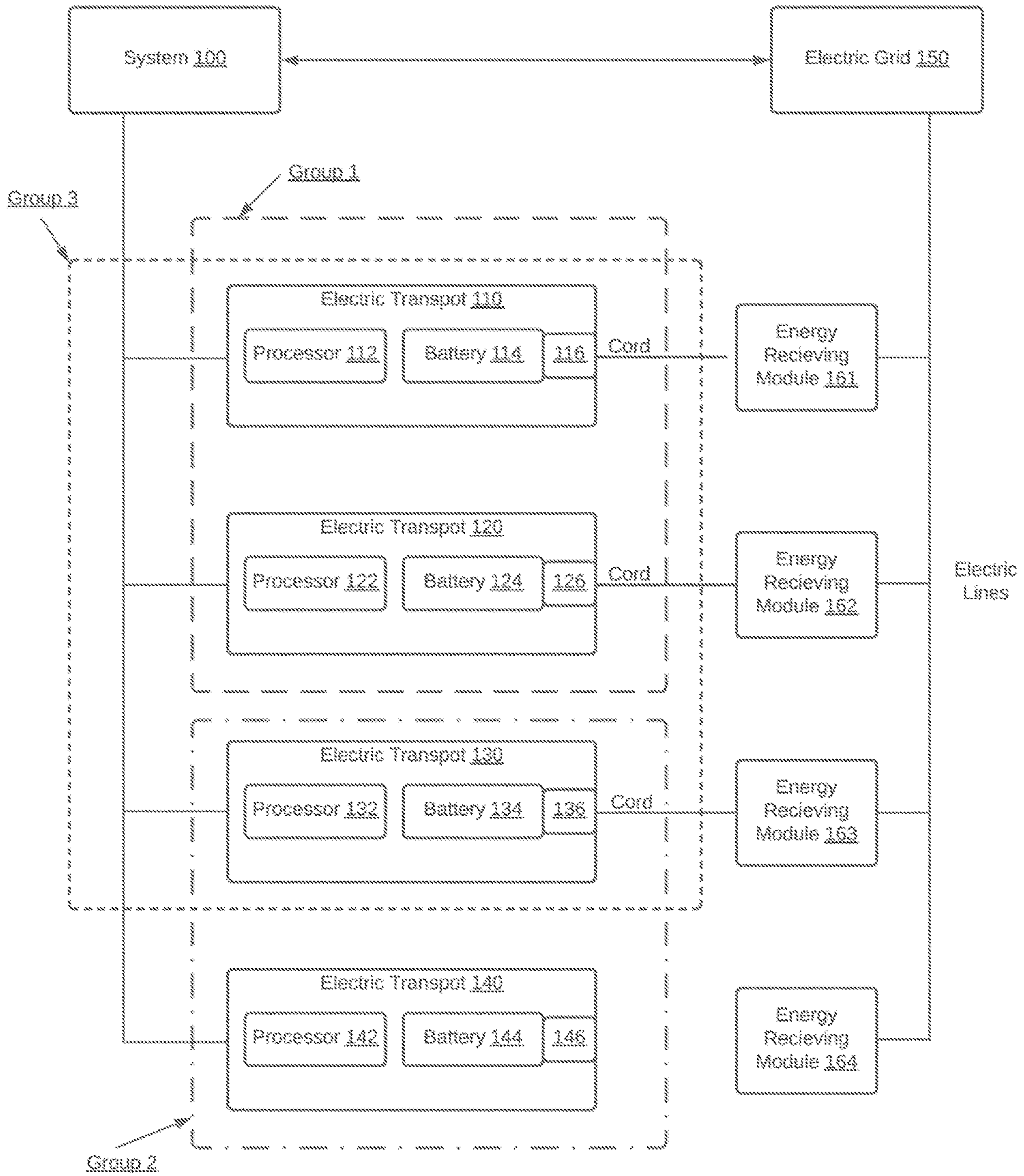
FIG. 1B
